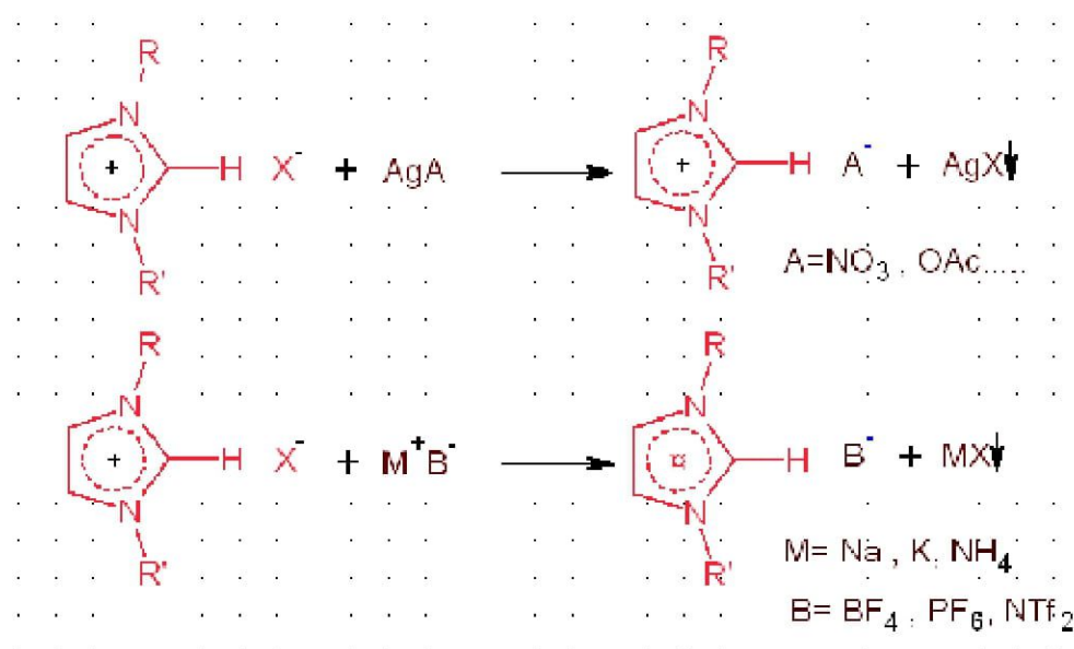
Schéma I. 9. Préparation des sels d'imidazolium par échange d'ions
