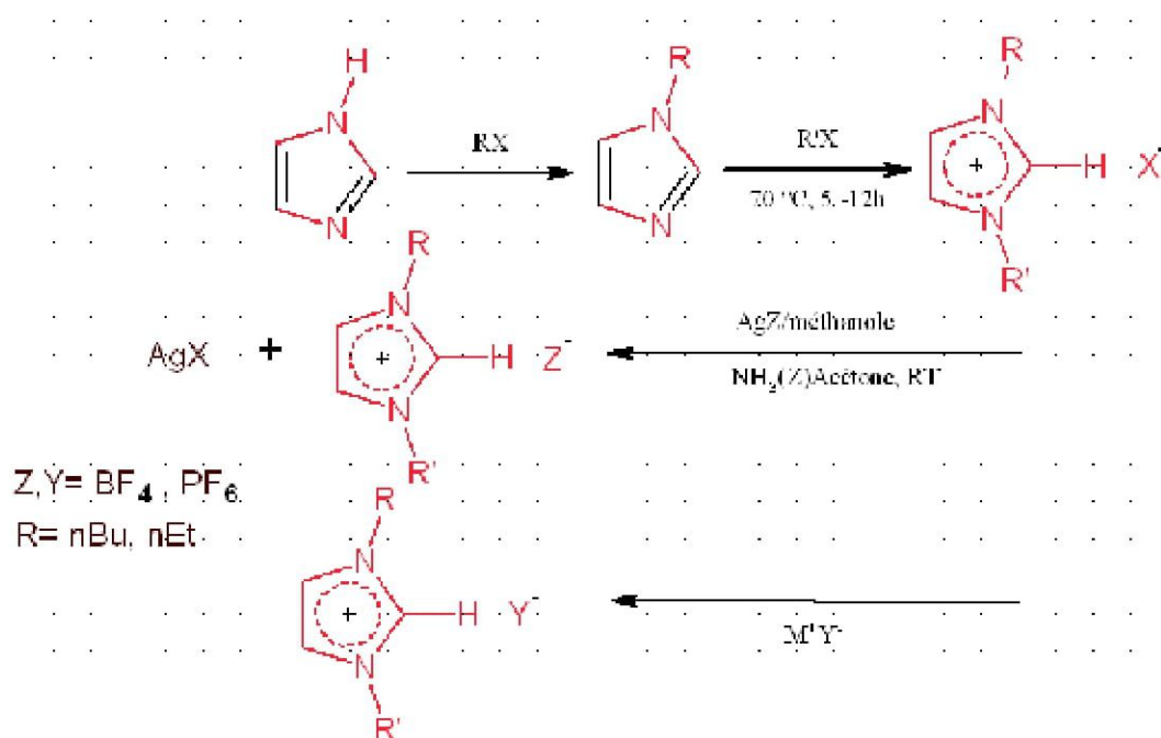
Schéma I. 10. Synthèse des liquides ioniques de sels de N,N'-dialkyl imidazolium
