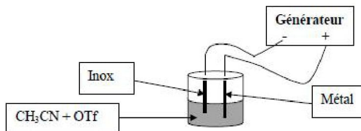
Figure VI. 1. Montage expérimentale
