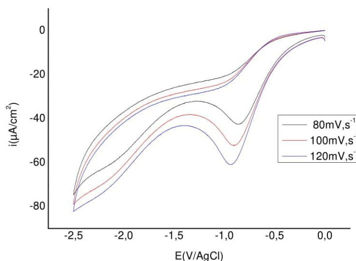
Figure VI. 23. Voltammogrammes cycliques sur l'électrode decarbone vitreux de \text{Ln}(\text{OTf})_3 (0.1mmol), en milieu \text{CH}_3\text{CN} (10ml) en présence de \text{Bu}_4\text{NBF}_4 (33mg), vitesses de balayage ( v=80, 100, 120\text{mV}\cdot\text{s}^{-1} )
