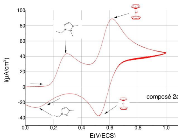
Figure V. 3. Voltammogramme cyclique du composé 2a dans ( 0.1 \text{ M CH}_3\text{CN//Bu}_4\text{NBF}_4 ), \nu = 100 \text{ mV s}^{-1}
