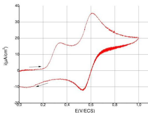
Figure V. 4. Voltammogramme cyclique du composé 2b dans ( 0.1 \text{ M CH}_3\text{CN//Bu}_4\text{NBF}_4 ), sur électrode carbone vitreux, \nu = 100 \text{ mV s}^{-1}
