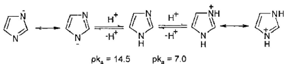
Figure I.2. Équilibres de transfert de protons de l'imidazole
