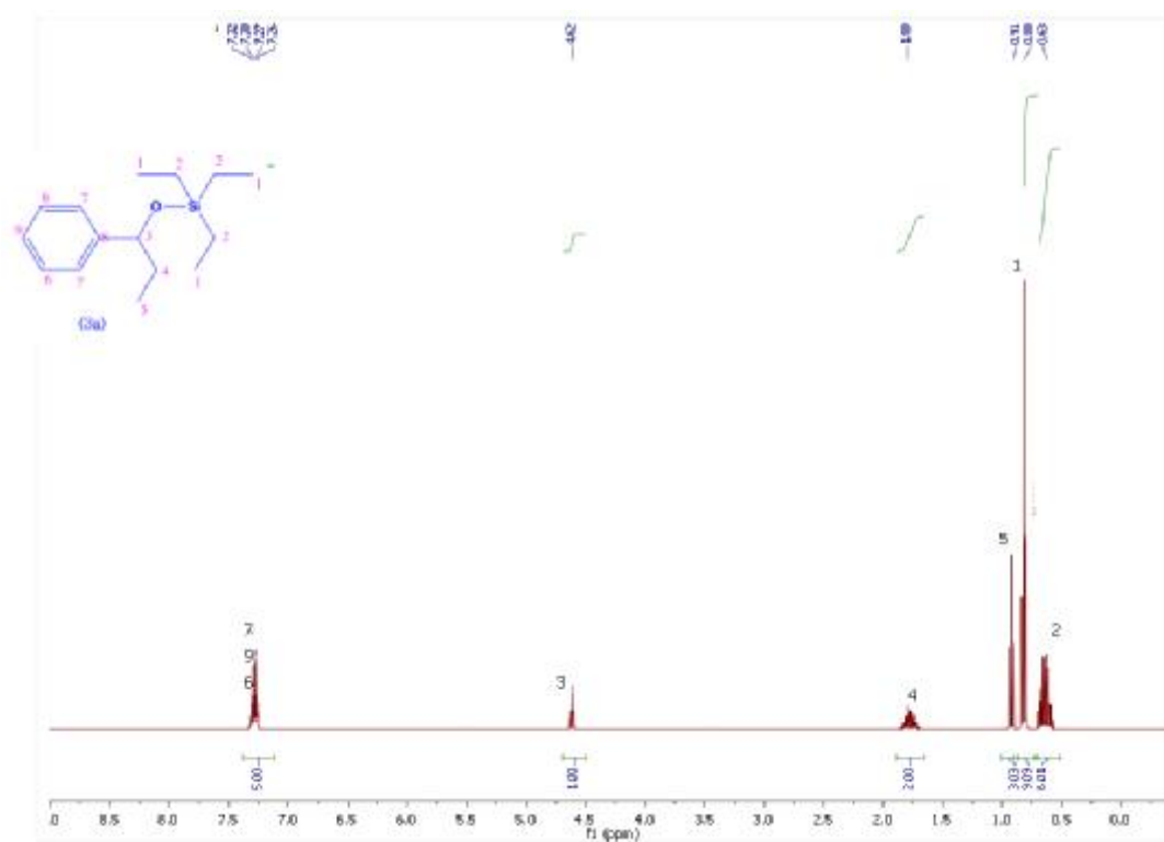
Figure 24. Spectre RMN ^1\text{H} de composé 3a en \text{CDCl}_3
