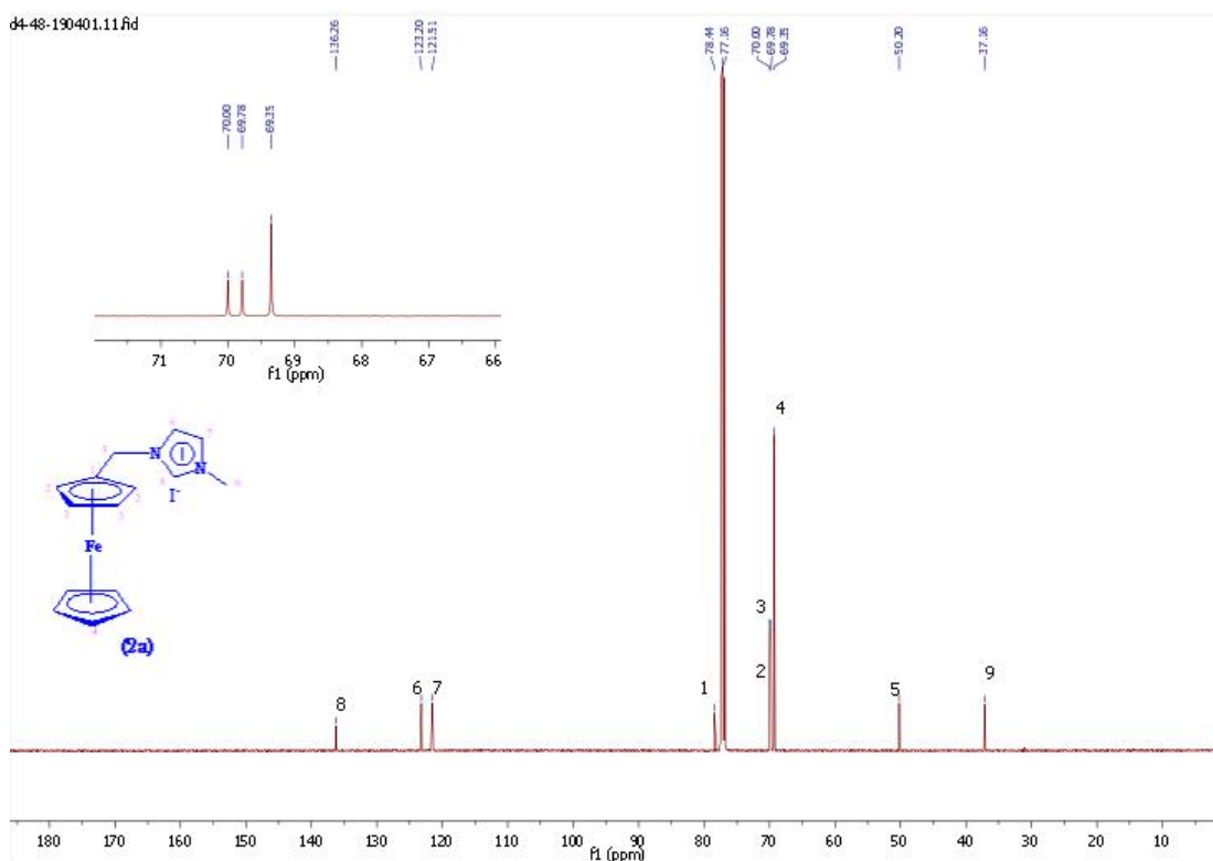
Figure 10. Spectre RMN ^{13}\text{C} de composé 2a en \text{CDCl}_3
