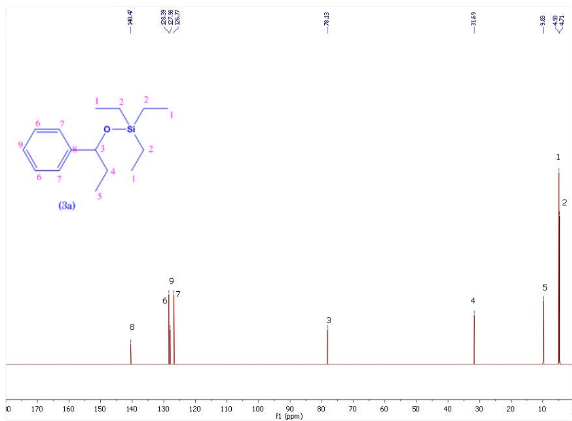
Figure 25. Spectre RMN ^{13}\text{C} de composé 3a en \text{CDCl}_3
