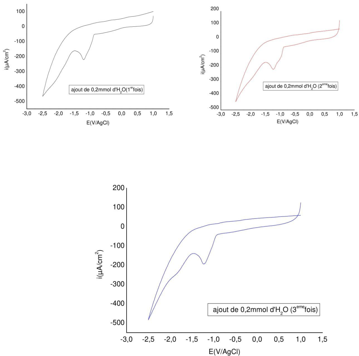
Figure VI. 12. Voltammogrammes cycliques de \text{Fe}(\text{OTf})_2 (0.1mmol) sur électrode de carbone vitreux après ajout d'eau(3 fois), en milieu DMF (10ml) en présence de \text{Bu}_4\text{NBF}_4 (33mg), vitesse de balayage 100\text{mV}\cdot\text{s}^{-1}
