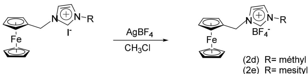
Schéma IV. 6. Synthèse de (2d) (2e) par échange d'anions
