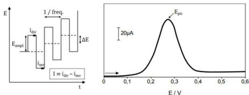
Figure III. 5. Séquence de balayage de potentiel utilisée en SWV (gauche) et exemple de courbe courant-potentiel obtenue (droite).
