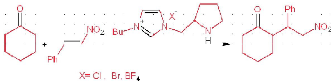
Schéma I. 22. Addition asymétrique de Michael des cétones avec des nitroalcènes
