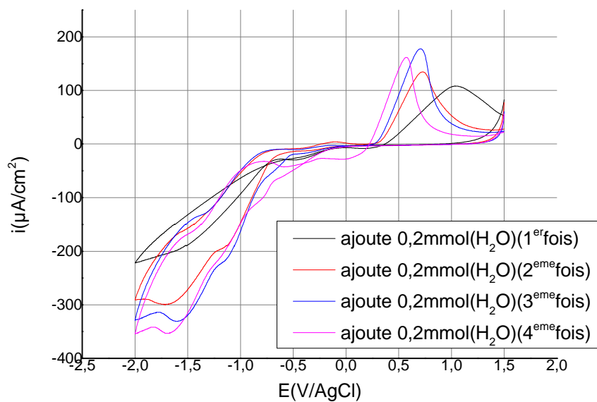
Figure.2. Voltammogrammes cycliques à l'électrode de carbone vitreux de Bi(OTf) 3 (0.1mmol) Après chaque ajout d'eau, en milieu organique ( Bu 4 NBF 4 (33mg) ; l'électrolyte support, CH 3 CN (10ml)), vitesses de balayage 100\text{mV}\cdot\text{s}^{-1}
