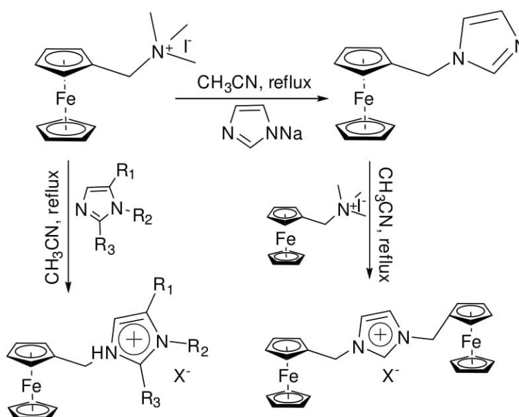
Schéma I. 14. Synthèse de sels de 1-ferrocényl-3-alkyle et de 1,3-di (ferrocénylméthyl) imidazolium
