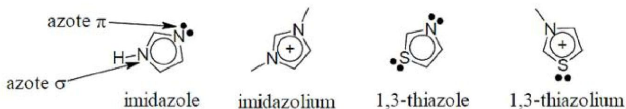
Figure I.3. Quelques azoles et sels d'azolium dérivés
