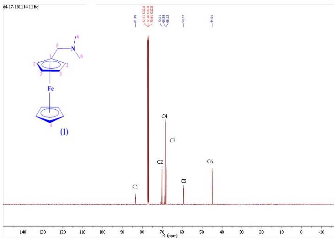
Figure 1. Spectre RMN 1 H de diméthylaminométhylferrocène(1)
