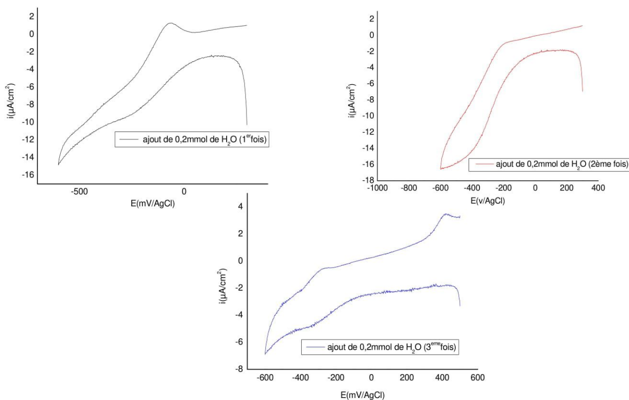
Figure VI. 6. Voltammogramme cyclique de l' \text{In}(\text{OTf})_3 (0.1mmol) sur l'électrode de carbone vitreux après chaque ajout d'eau, en milieu organique \text{CH}_3\text{CN} (10ml) en présence de l'électrolyte support \text{Bu}_4\text{NBF}_4 (33mg) , vitesse de balayage 100\text{mV}\cdot\text{s}^{-1}
