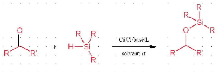
Schéma I. 26. Hydrosilylation de cétones catalysée par un sel d'imidazolium
