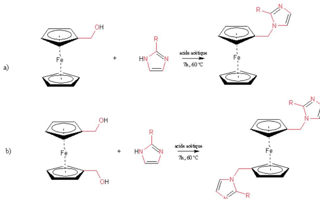
Schéma I. 15. Schémas de réaction du (a) ferrocénéméthanol et (b) du 1,1'-diferrocénéméthanol
