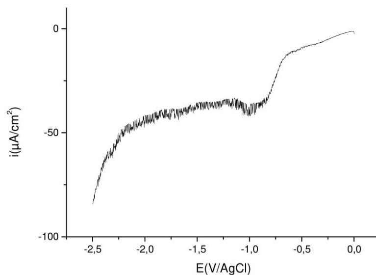
Figure VI. 5. Résultats typiques de voltampérométrie d'impulsion normale pour 0.2 mmol de In[OTf] 3 dans Bu 4 NBF 4 / MeCN
