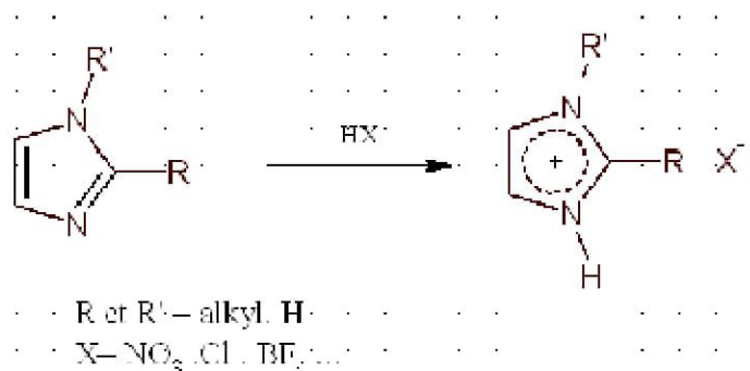
Schéma I. 8. Préparation de sels d'imidazolium par réaction acido-basique
