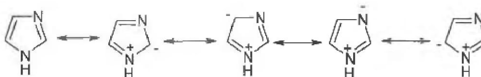
Schéma I. 1. Système délocalisé de l'anneau imidazole
