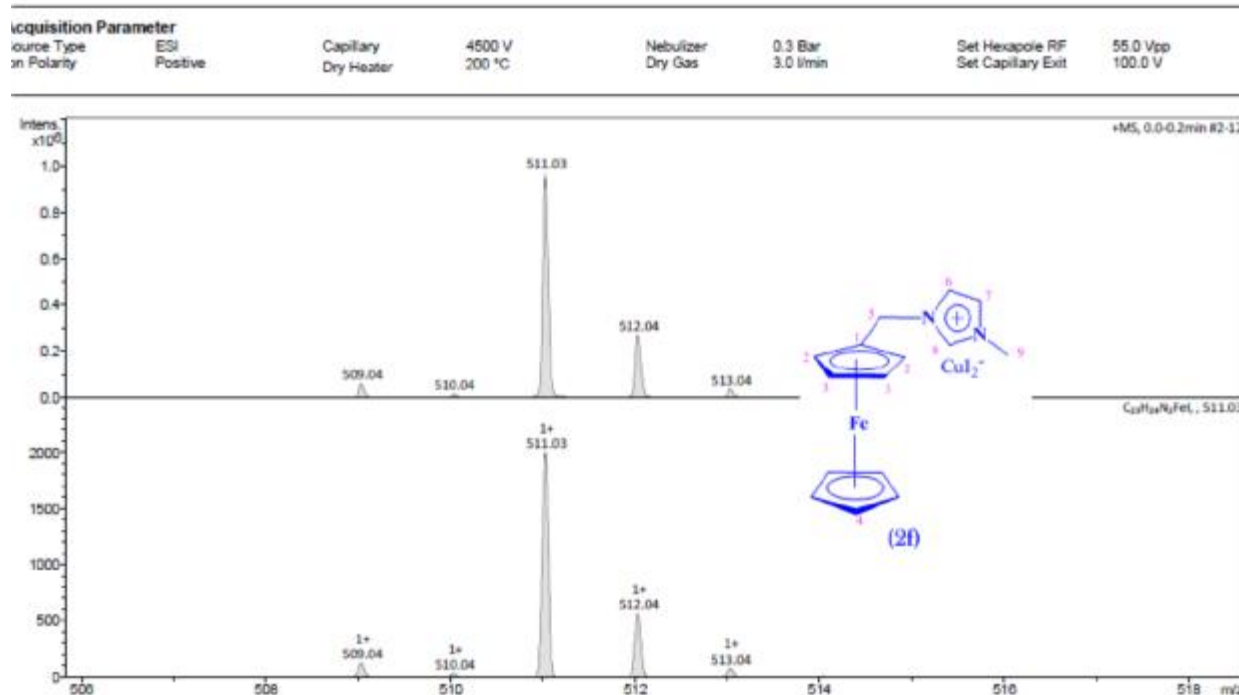
Figure 8. Spectre de masse du d'iodure du 1-(Ferrocénylméthyl)-3-méthyl-imidazolium \text{CuI}_2 (2f) (Electrospray) en mode positif (zoom et simulation2).
