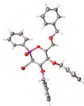
Figure 3.4 : Structure cristallographique de phosphine bromée 3.8 à configuration glucose-like .
