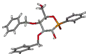
Figure 2.6 : Structure cristallographique de la phostine 2.54 .
