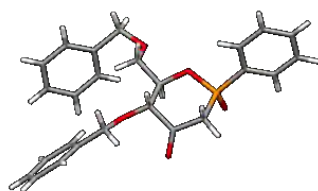
Figure 3.13 : Structure cristallographique du \beta -cétophosphinate 3.18 .
