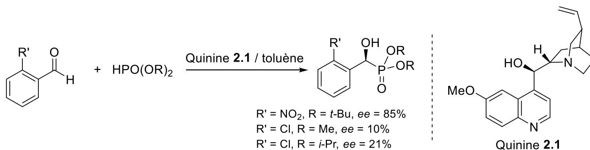
Schéma 2.3 : Hydrophosphonylation asymétrique d'aldéhydes catalysée par la quinine 2.1 .
