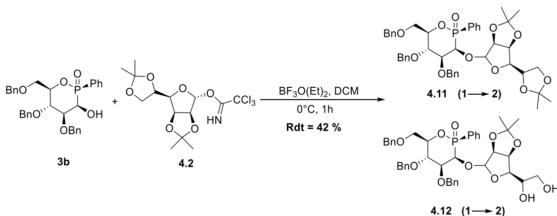
Schéma 4.10 : Couplage entre la phostine 3b et le sucre donneur 4.2 catalysé par le trifluorure de bore.
