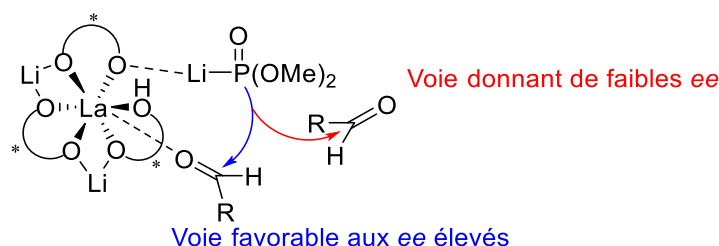
Figure 2.2 : État de transition proposé dans l'hydrophosphonylation d'aldéhydes par le R -LLB.
