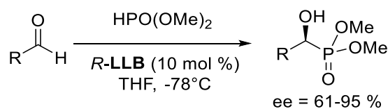
Schéma 2.10 : Effet de l'addition lente de l'aldéhyde dans l'hydrophosphonylation catalysée par le R -LLB.
