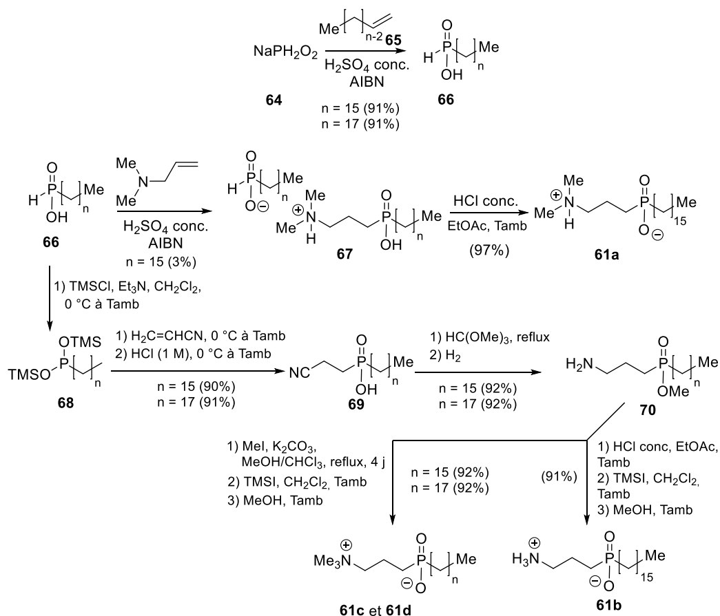
Schéma 1.8 : Synthèse d'analogues phosphinates 61a-d de la miltéfosine.
