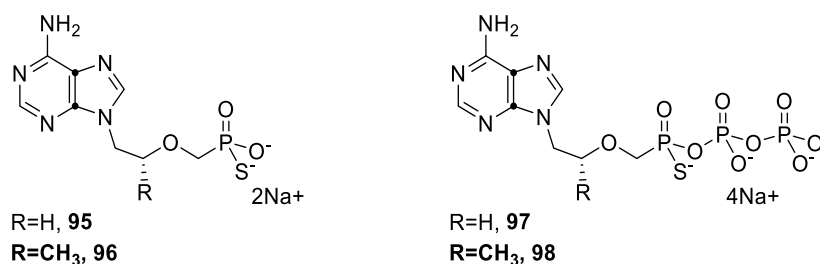
Figure 1.14 : Analogues thiophosphonates dérivés de l'Adéfovir et Ténofovir à activité antirétrovirale.
