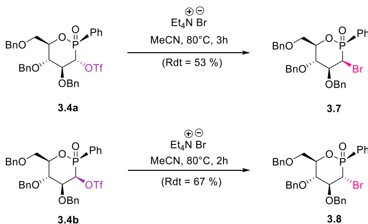
Schéma 3.10 : Synthèse des dérivés bromés 3.7 et 3.8 .
