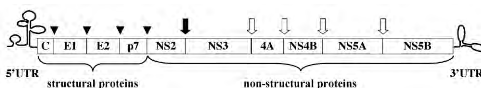
Figure 1.15 : Diagramme schématique du génome du VHC.
