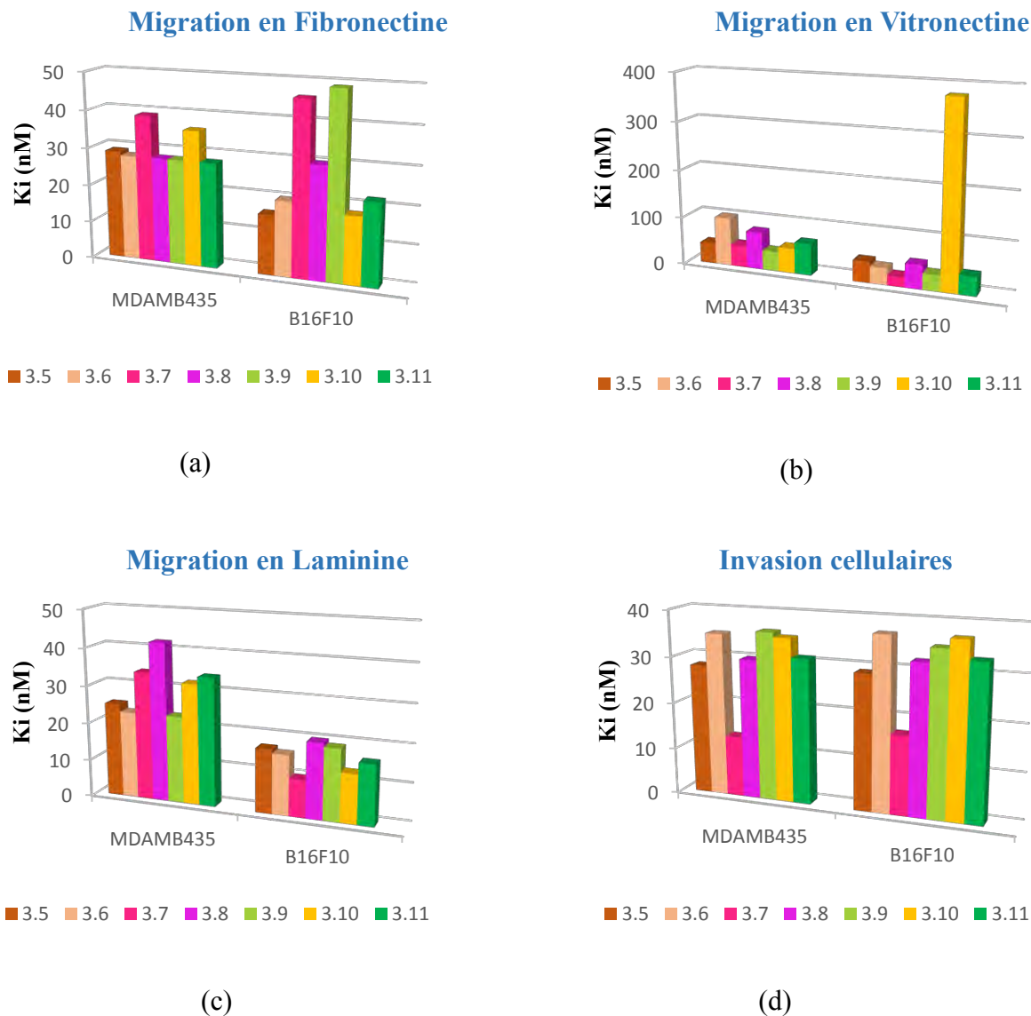
Figure 3.10 : Valeurs de Ki pour la migration et l'invasion des cellules « MDAMB435 » et « B16F10 ».
