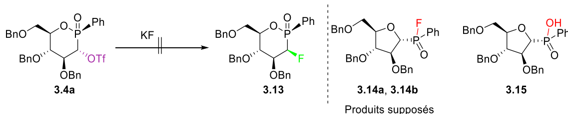
Schéma 3.15 : Fluoration du triflate 3.4a .
