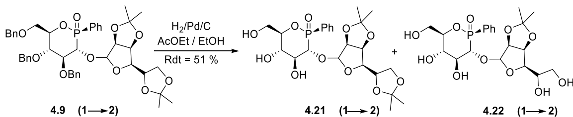
Schéma 4.19 : Hydrogénation catalytique du pseudo-disaccharide 4.9 (1→2).
