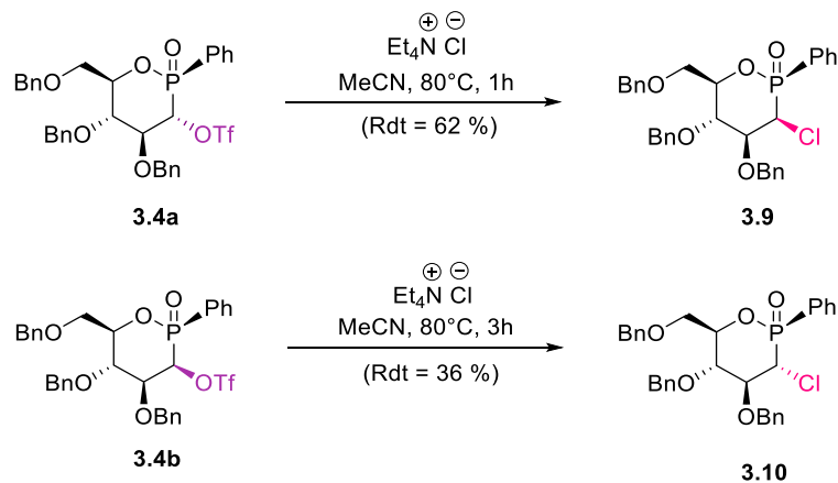
Schéma 3.11 : Synthèse des dérivés chlorés 3.9 et 3.10 .
