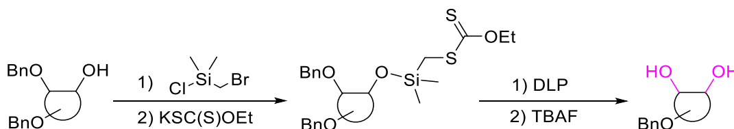
Schéma 2.27 : Débénylation régiosélective par transfert 1,7 d'hydrogène.
