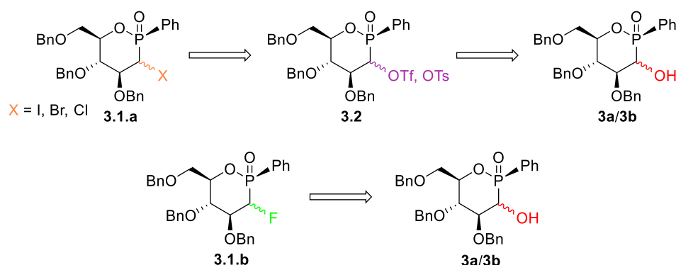
Schéma 3.3 : Séquence rétrosynthétique pour la préparation des dérivés halogénés de 3a et 3b .
