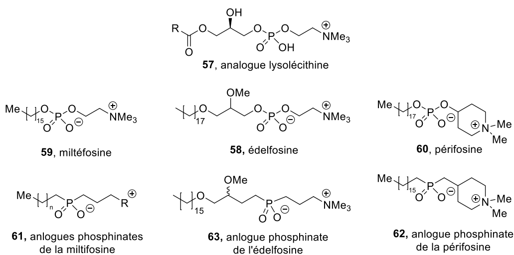
Figure 1.12 : Structure de lysocéithin, quelques alkyl- lysophospholipides et ses analogues phosphinates.
