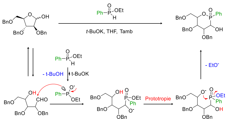
Schéma 2.2 : Mécanisme réactionnel pour la formation des phosphinosucres 3a-d .
