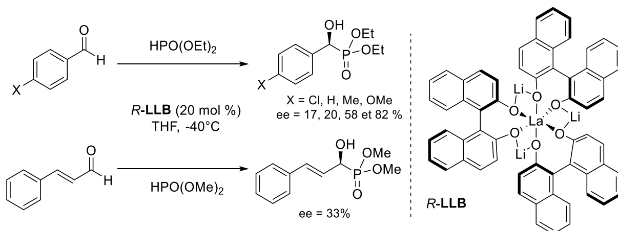
Schéma 2.9 : Utilisation du R -LLB dans l'hydrophosphonylation asymétrique d'aldéhydes.
