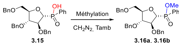
Schéma 3.16 : Réaction d'estérification de l'acide phénylphosphinique 3.15 .
