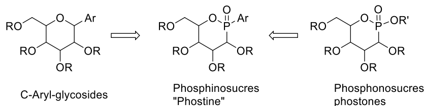
Figure 4 : Phosphinosucres ou « Phostines »
