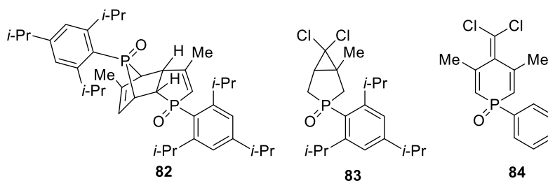
Figure 1.13 : Oxydes de phosphines synthétisés et testés comme agents antiprolifératifs.
