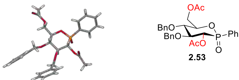
Figure 2.5 : Structure cristallographique de la phostine 2.53 .
