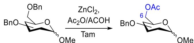
Schéma 2.19 : Débenzylation régiosélective de glycopyranoside catalysée par le chlorure de zinc.
