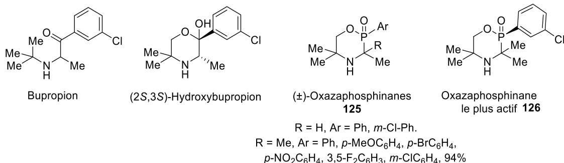
Figure 1.18 : Structure de Bupropion, son métabolite et ses analogues 1,4,2-oxazaphosphinanes.
