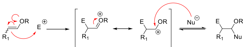
Schéma 3.24 : Réactivité des éthers d'énol.
