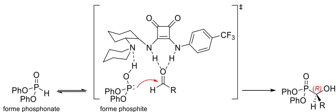
Figure 2.1 : État de transition schématisé par Herrera.
