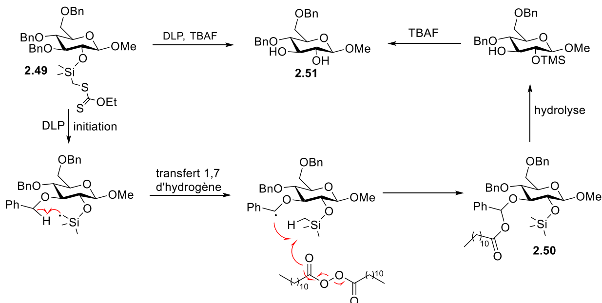
Schéma 2.28 : Mécanisme réactionnel proposé pour la débenzylation régiosélective selon Attouche.
