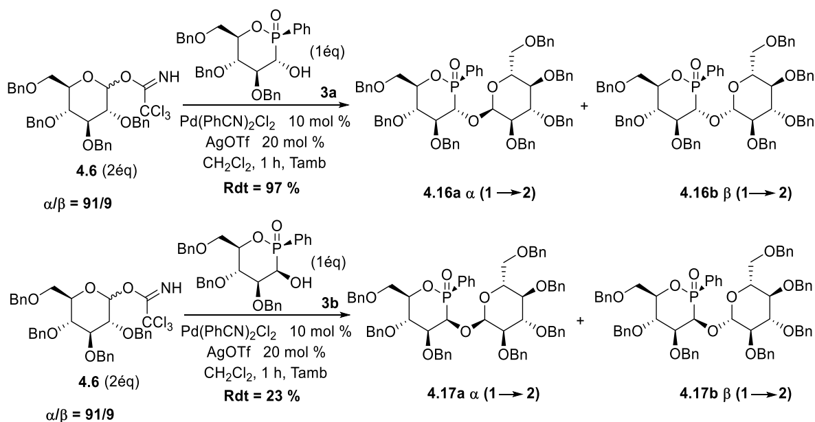
Schéma 4.15 : Synthèse des pseudo-disaccharides 4.16a \alpha ( 1 → 2 ), 4.16b \beta ( 1 → 2 ) et 4.17a \alpha ( 1 → 2 ).
