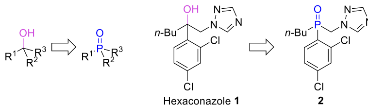
Figure 1.5 : L'analogue phosphoré « oxyde de phosphine » de hexaconazole.
