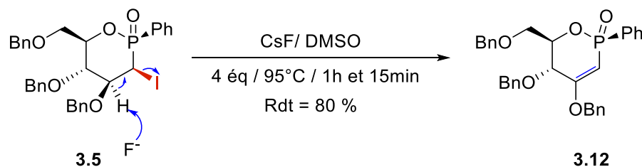
Schéma 3.14 : Mécanisme de la réaction d'élimination.
