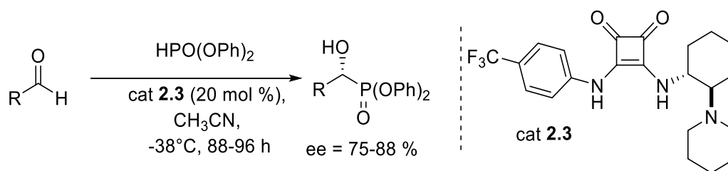
Schéma 2.5 : Hydrophosphonylation asymétrique d'aldéhydes catalysée par le squaramide 2.3 .
