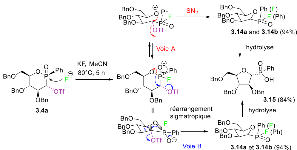
Schéma 3.17 : Proposition pour la formation du composé 3.15 .
