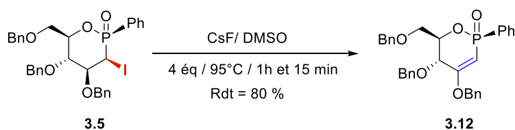
Schéma 3.14 : Synthèse de la phosphine insaturée 3.12 .
