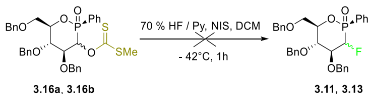
Schéma 3.22 : Fluoration des xanthates.
