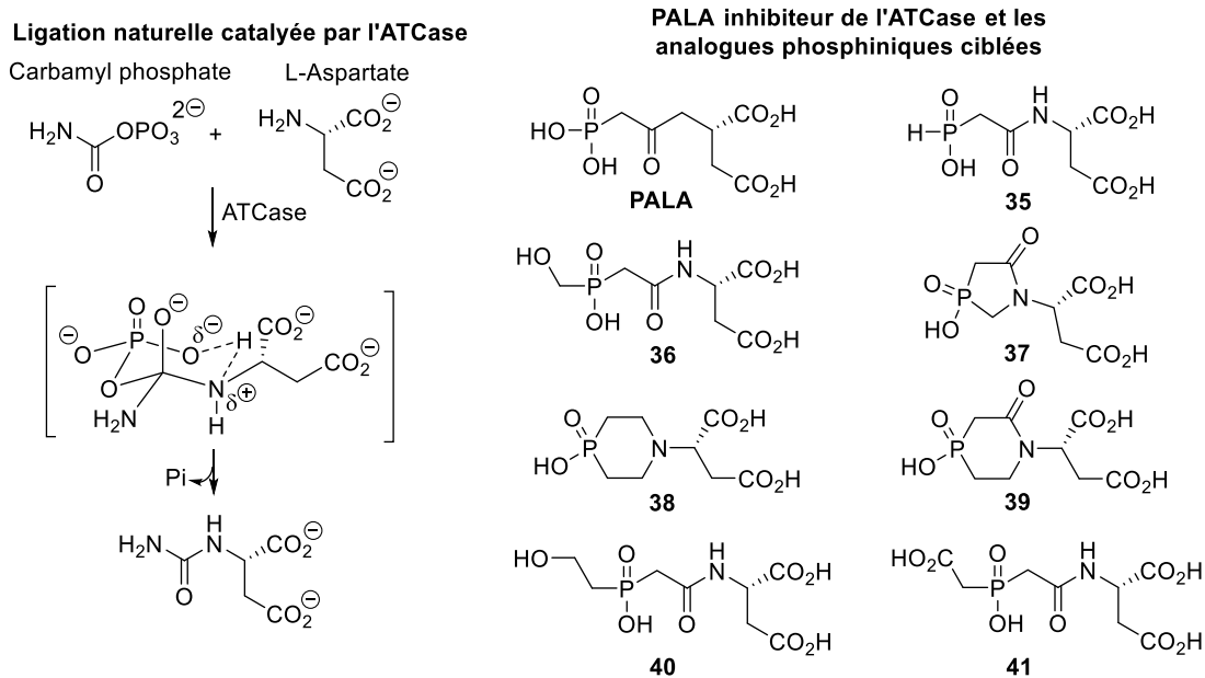
Figure 1.11 : Ligation catalysée par l'ATCase et les inhibiteurs ciblés.
