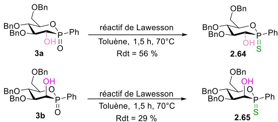
Schéma 2.37 : Synthèse des thiophostines 2.64 et 2.65 par sulfuration directe.
