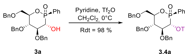
Schéma 3.8 : Synthèse de l'ester triflique à partir de l'alcool 3a .
