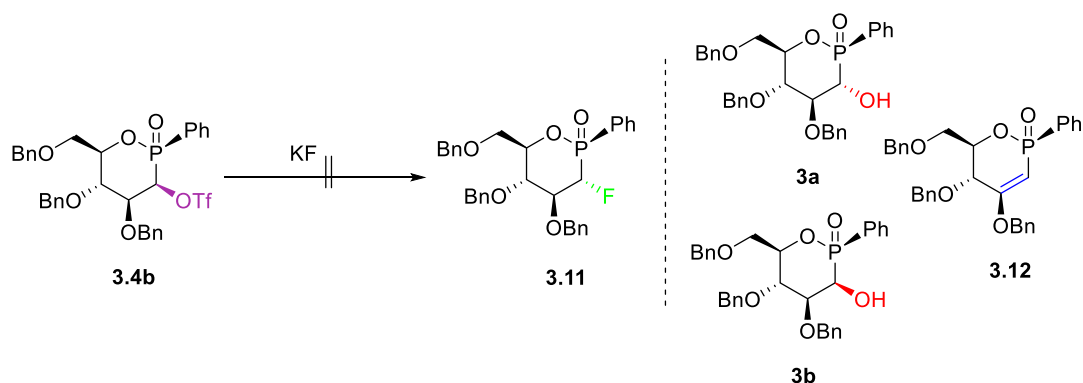
Schéma 3.12 : Fluoration de triflate 3.4b .
