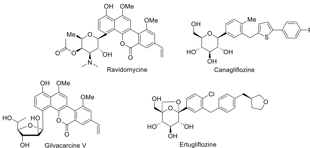
Figure 3 : Exemples de C-aryl glycosides biologiquement actifs.
