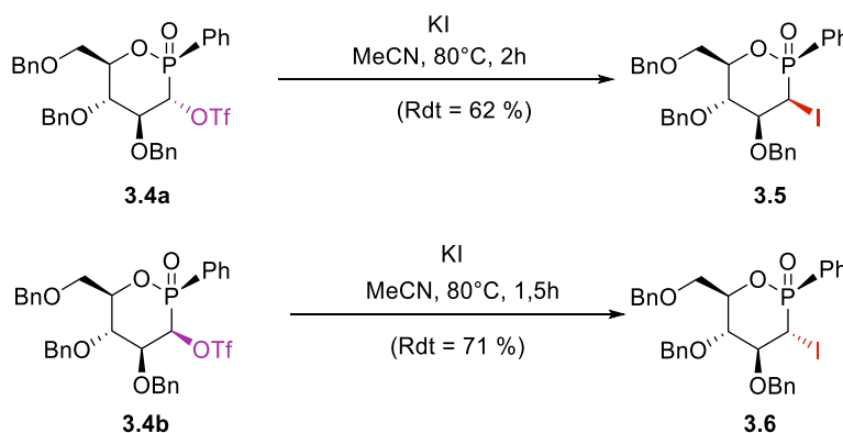
Schéma 3.9 : Synthèse des dérivés iodés 3.5 et 3.6 .
