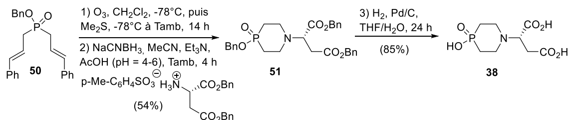
Schéma 1.6 : Synthèse de l'analogue phosphinique 38 du PALA.
