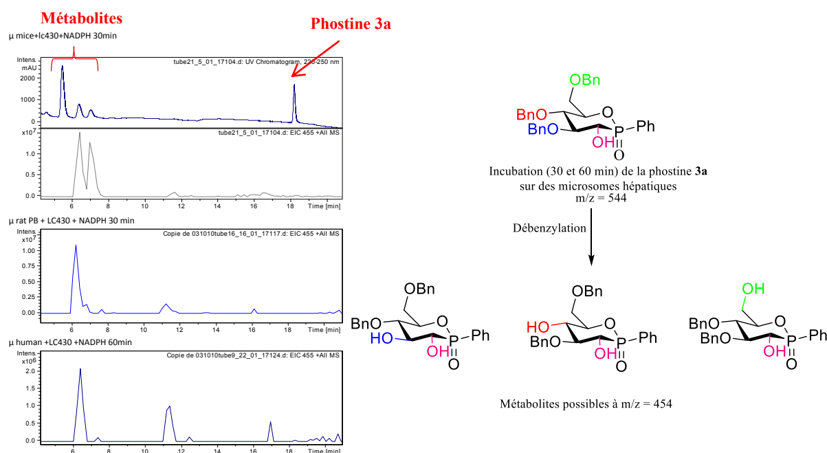
Figure 2.3 : Incubation de la phostine 3a avec les cytochromes P450 et formation d'un métabolite correspondant à une phostine débenzylée.
