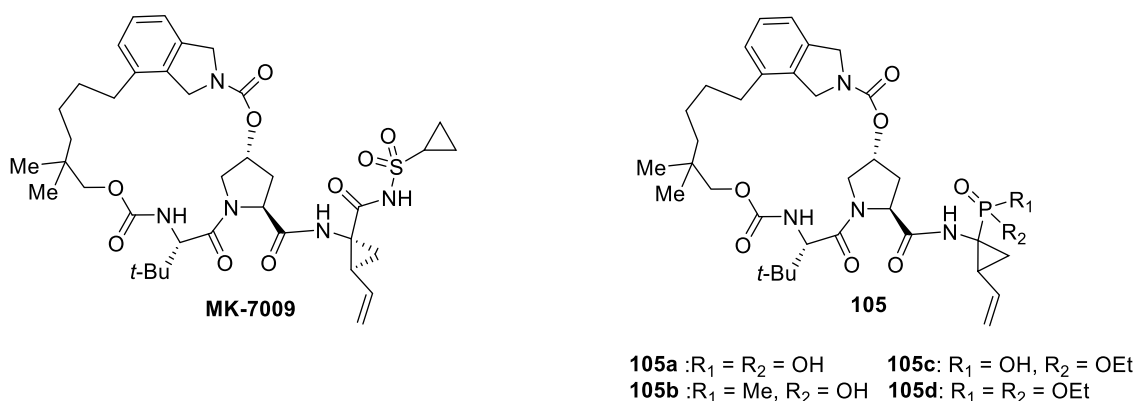
Figure 1.16 : Structure chimique du MK-7009 et de ses analogues phosphinates et phosphonates 105 .
