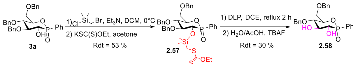
Schéma 2.33 : Synthèse du diol 2.58 par débenzylation radicalaire.
