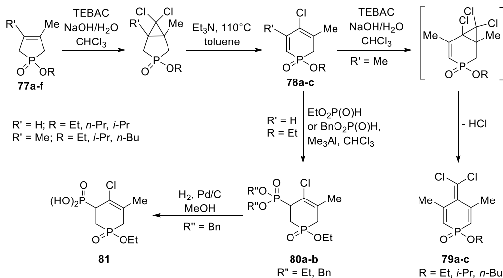
Schéma 1.10 : Synthèse de quelques dérivés phosphinates du type oxydes de 1,2 et 1,4-dihydrophosphinine et oxydes de 1,2,3,6-tétrahydrophosphinine.
