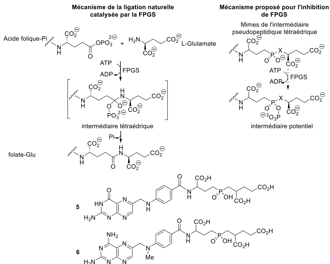
Figure 1.7 : Mécanisme de la polyglutamylation catalysée par la FPGS et de son inhibition.
