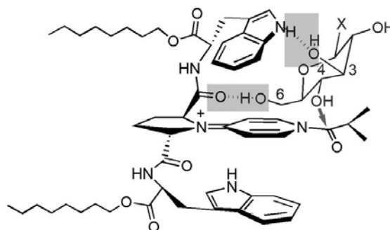
Figure 2.4 : État de transition proposé pour l'acétylation régiosélective en position 4 en présence du catalyseur 2.16 .
