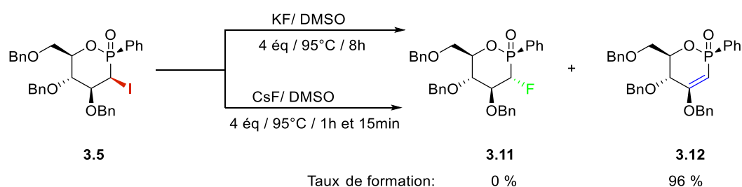
Schéma 3.13 : Fluoration versus élimination à partir de la phosphine iodée 3.5 .
