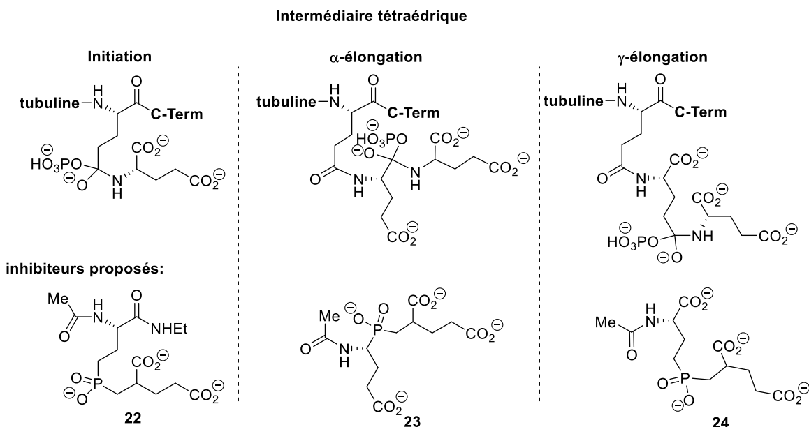
Figure 1.10 : Les structures des inhibiteurs supposés des TTLL.
