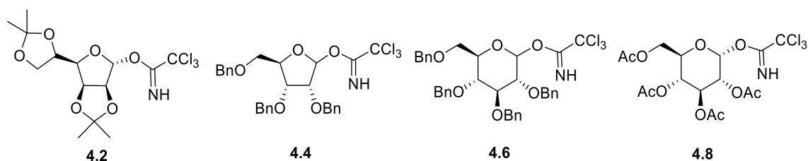
Figure 4.5 : Structures des sucres donneurs utilisées.
