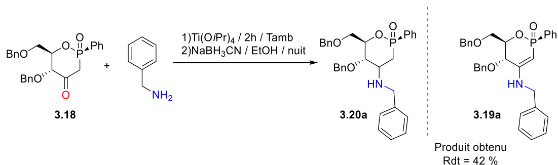
Schéma 3.29 : Essai d'amination réductrice du \beta -cétophosphinate 3.18 avec la benzylamine.
