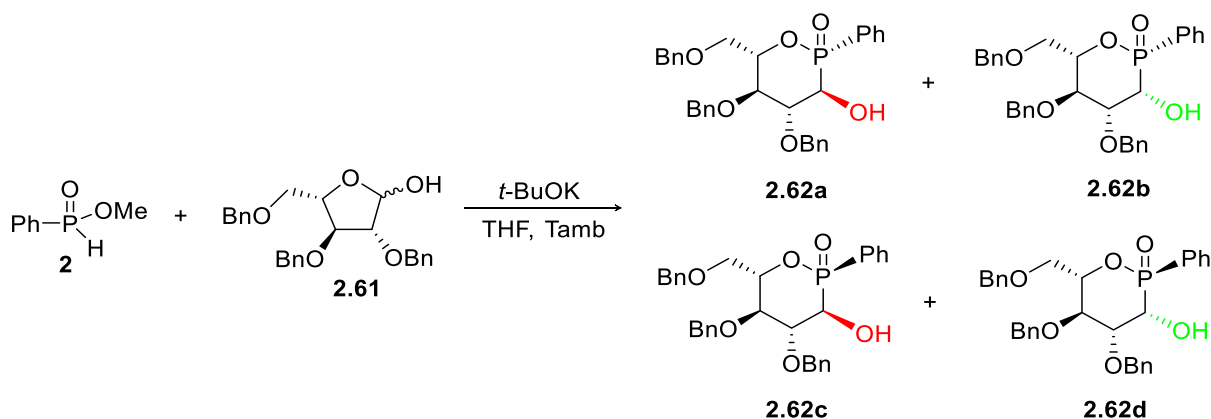
Schéma 2.35 : Synthèse des phostines via le L -arabinofuranose O -benzylé.
