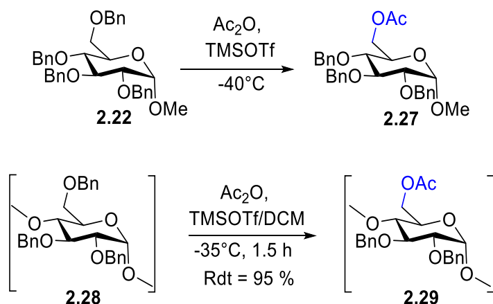
Schéma 2.18 : Débenzylation régiosélective par acétylation selon les conditions d'Engibeaud et Utile.
