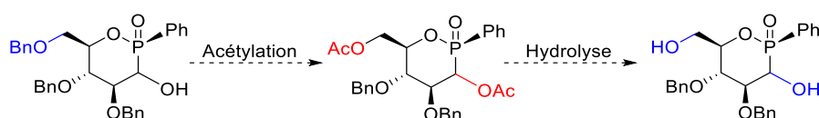
Schéma 2.29 : Méthode synthétique pour la préparation de 2,6-dihydroxy-1,2--oxaphosphinanes.
