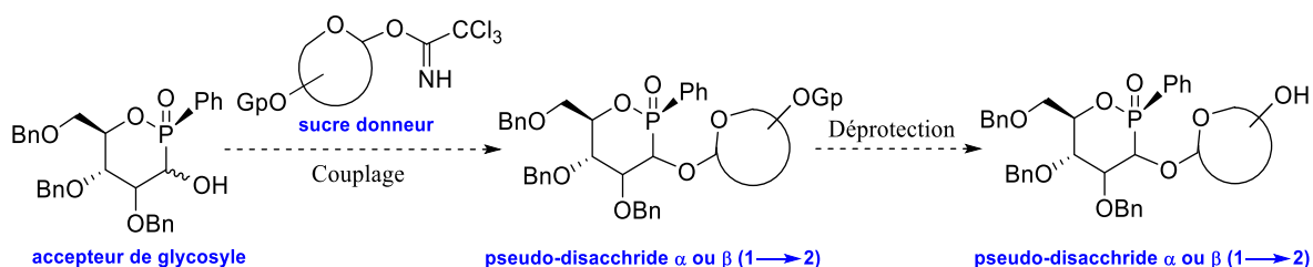
Schéma 4.4 : Méthode de synthèse pour la formation des pseudo-disaccharides (1→2).
