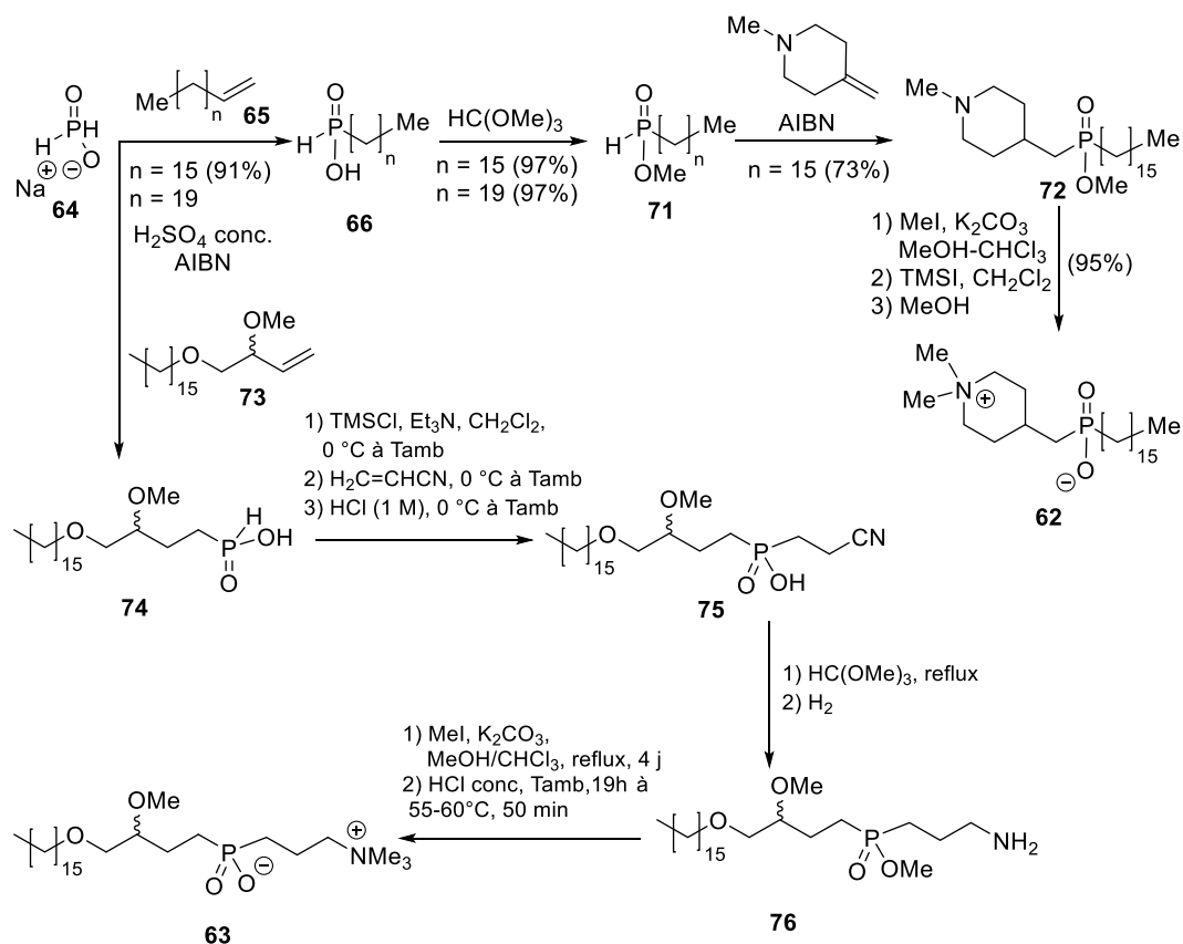
Schéma 1.9 : Synthèse d'analogues phosphinates la périfosine 62 et de l'édelfosine 63 .
