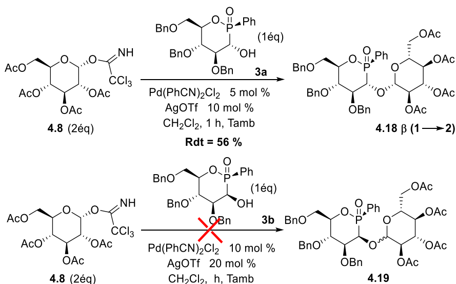
Schéma 4.16 : Synthèse de pseudo-disaccharide 4.18 β (1→2) .
