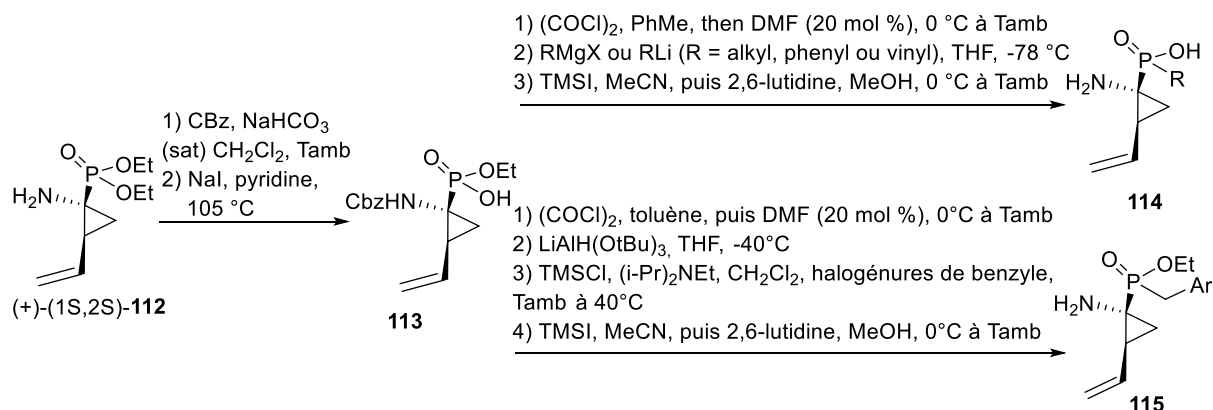
Schéma 1.14 : Préparation des précurseurs \alpha -aminophosphinates 114 et 115 .
