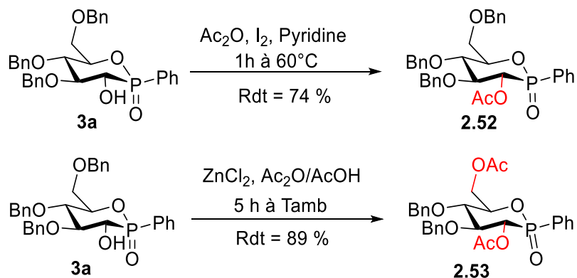
Schéma 2.30 : Acétylation de la phostine 3a .
