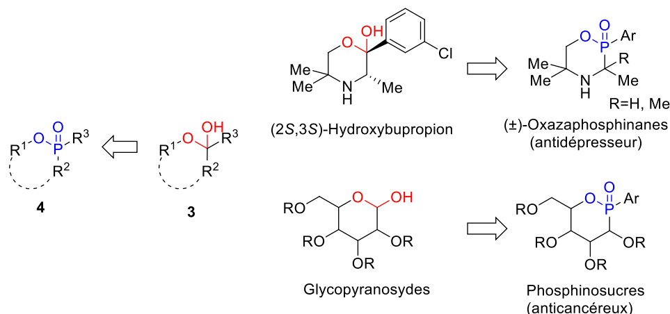
Figure 1.6 : Analogie entre la fonction lactol et la fonction phosphinolactone.
