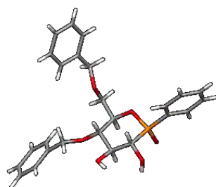
Figure 2.7 : Structure cristallographique du diol 2.58 .
