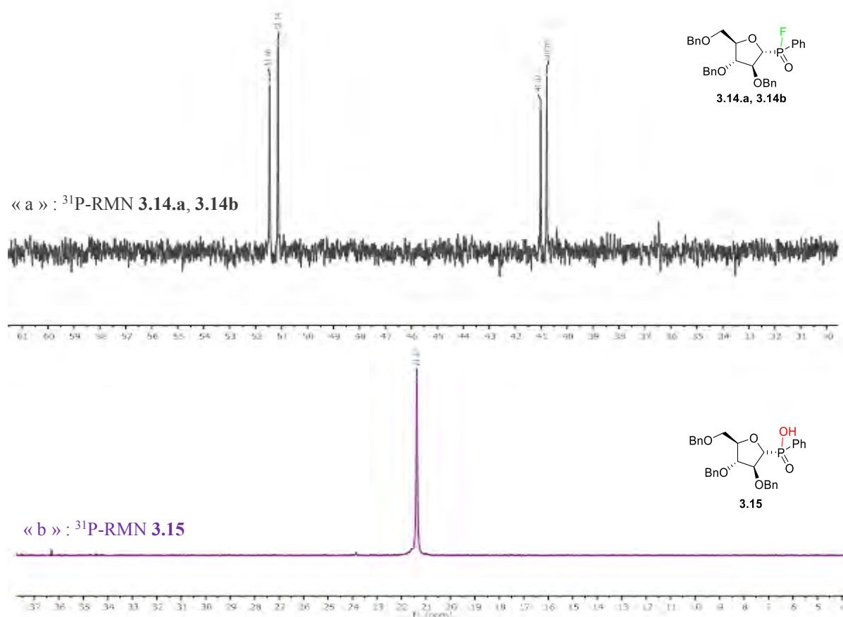
Figure 3.3 : Spectre RMN du ^{31}\text{P} du milieu réactionnel avant « a » et après l'hydrolyse « b » à partir de l'entrée 5.
