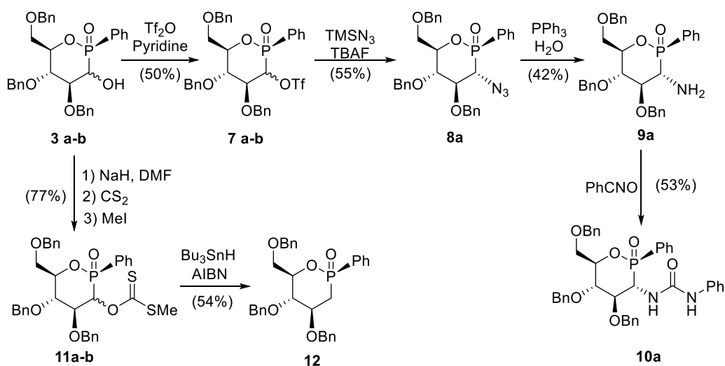
Schéma 3 : Modification structural à partir des phosphines 3a-b .
