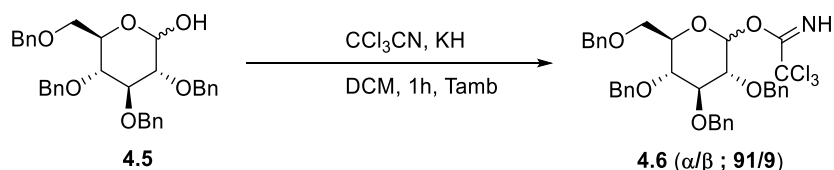
Schéma 4.7 : Préparation du sucre donneur 4.6 .
