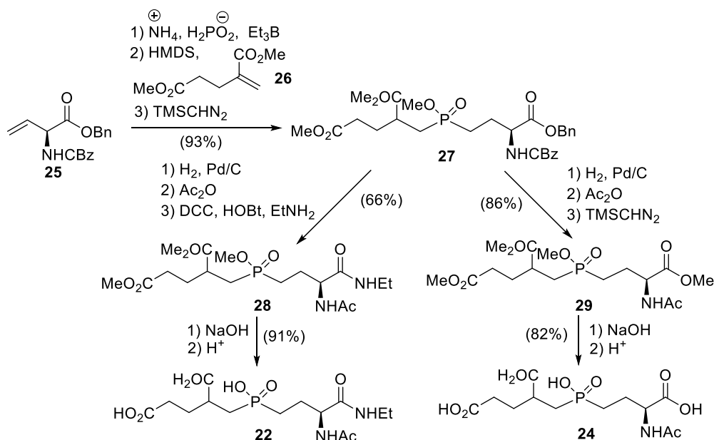
Schéma 1.2 : Synthèse des inhibiteurs 22 et 24 .
