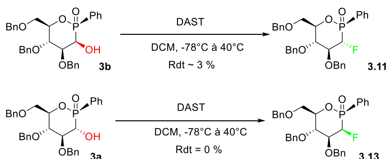
Schéma 3.18 : Synthèse de dérivés fluorés 3.11 et 3.13 .
