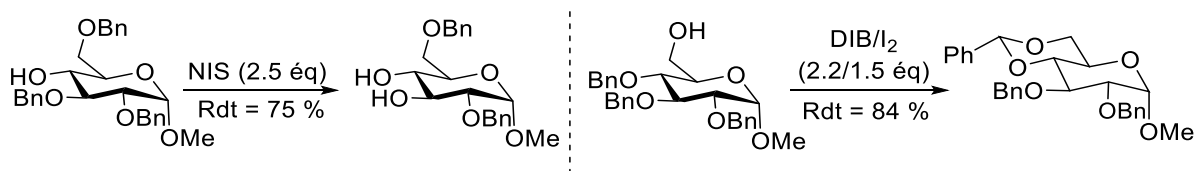
Schéma 2.24 : Débenzylation régiosélective par le NIS ou le DIB/I 2 .
