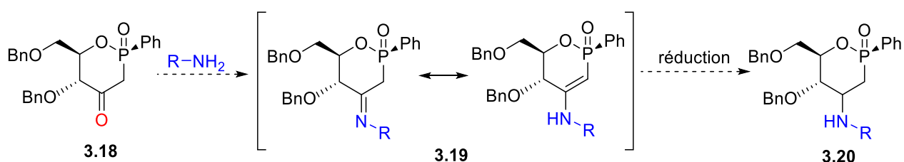
Schéma 3.28 : Méthode envisagée pour la synthèse des aminophosphinates 3.20 à partir du phosphinosucre β-cétonique 3.18 .
