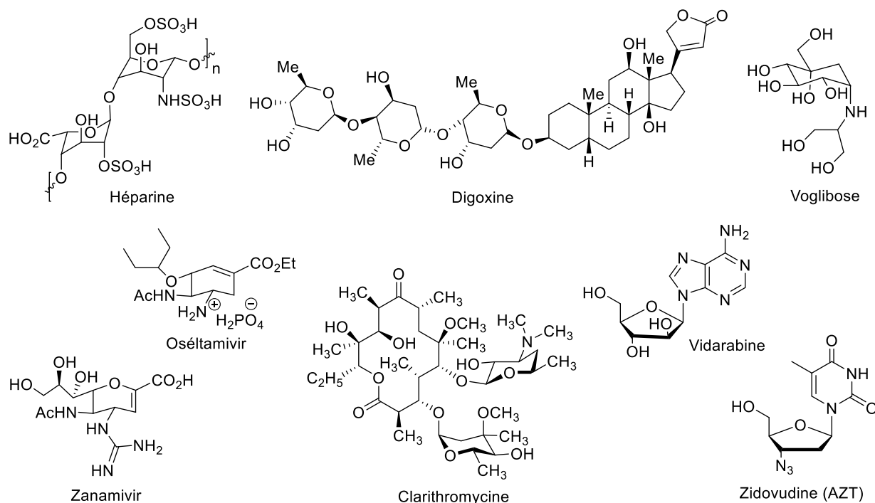
Figure 4.2 : Exemples de médicaments à base de glucide.
