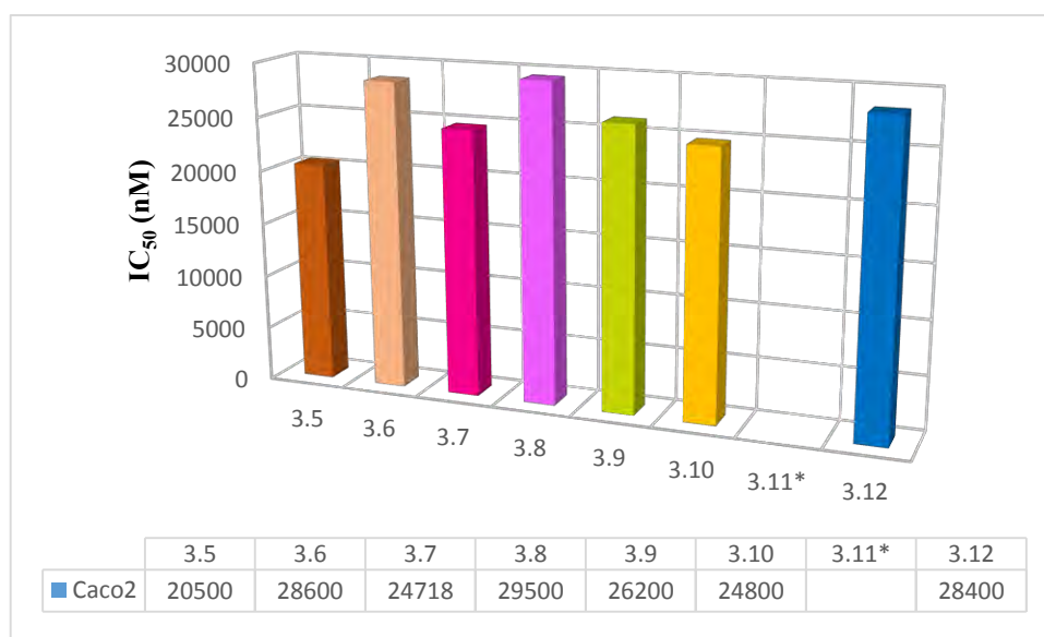
Figure 3.8 : Valeurs d'IC 50 des phostines 3.5 à 3.12 sur la lignée cellulaire Caco-2.
