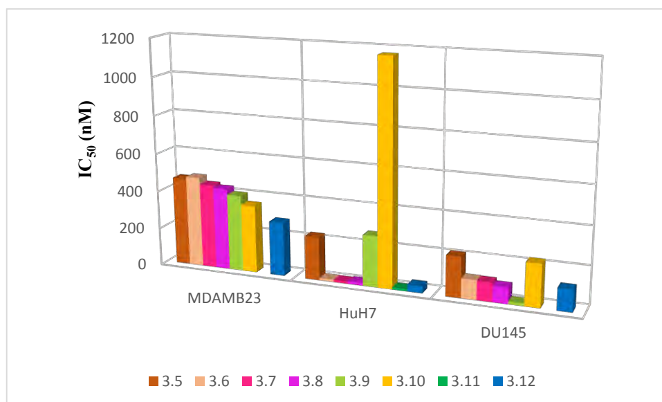
Figure 3.7 : Valeurs des IC 50 des phostines 3.5 à 3.12 envers les lignées cellulaires MDAMB23 HuH7 et DU145.
