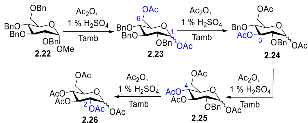
Schéma 2.17 : Ordre d'acétylolyse de 2,3,4,6-tétra- \alpha -D-glucopyranoside en présence d'acide sulfurique.
