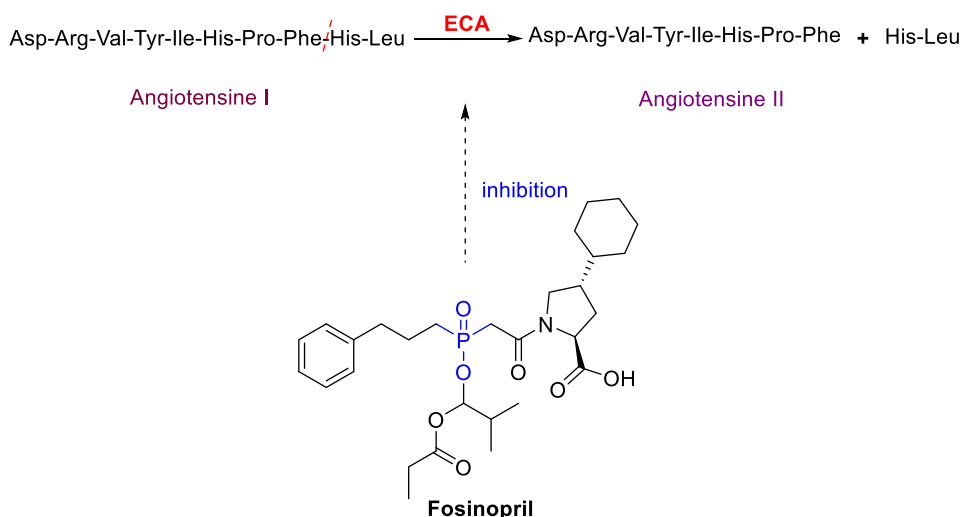
Figure 1.4 : Hydrolyse de l'angiotensine I en angiotensine II, catalysée par l'ECA et inhibition de ce processus par le Fosinopril.
