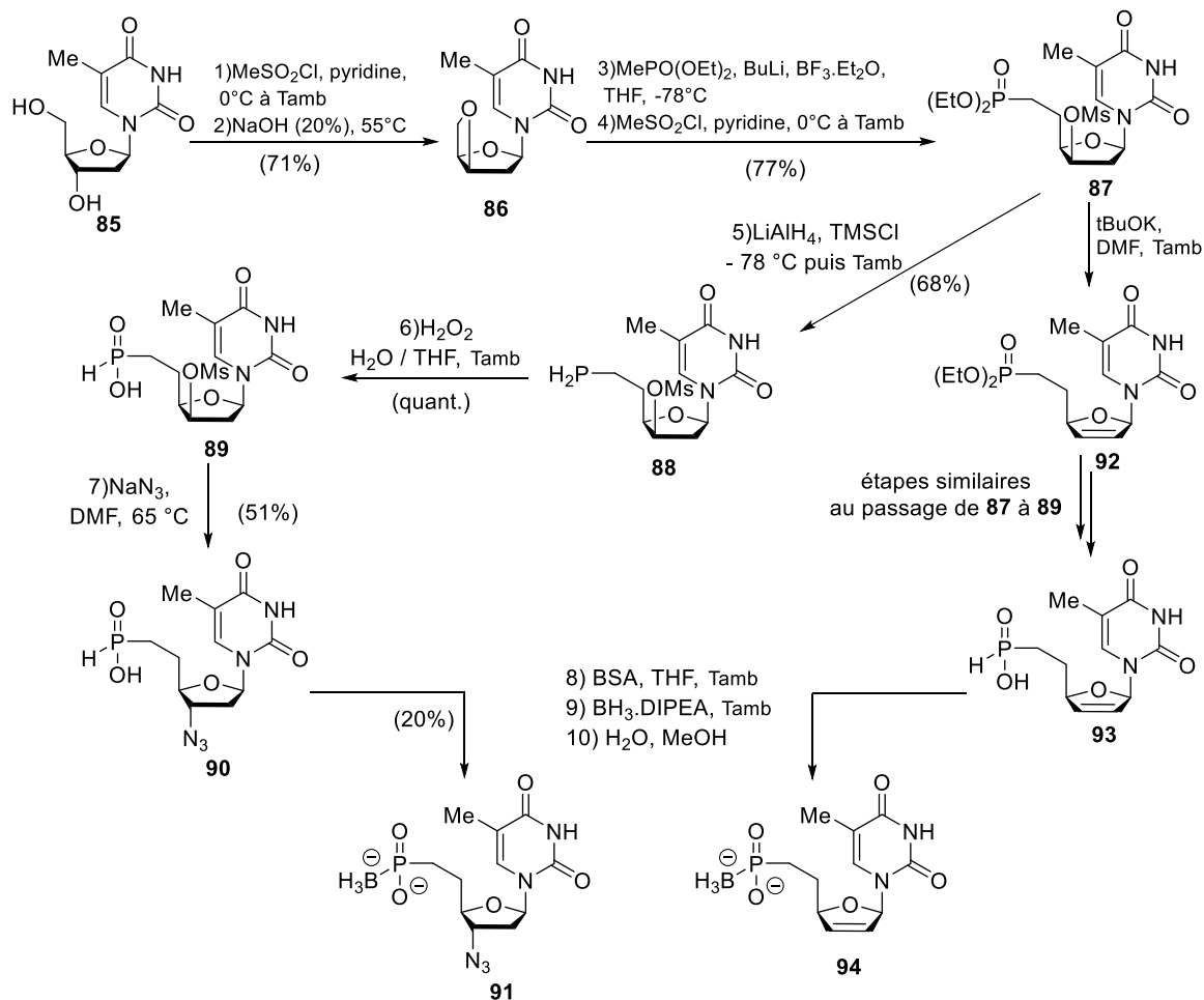
Schéma 1.11 : Synthèse d'analogues boranophosphonates dérivés de l'AZT et du d4T.
