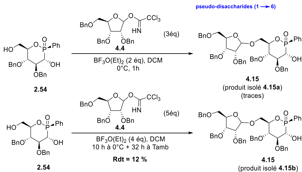
Schéma 4.12 : Couplage entre la phosphite 2.54 et le sucre donneur 4.4 catalysé par le trifluorure de bore.
