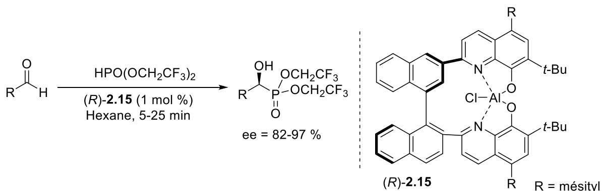
Schéma 2.15 : Hydrophosphonylation asymétrique d'aldéhydes selon les conditions de Yamamoto.
