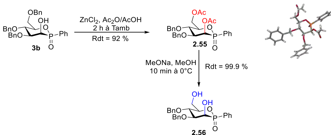
Schéma 2.32 : Synthèse du dihydroxy-2,6-oxaphosphinane 2.56 à partir de la phostine 3b .
