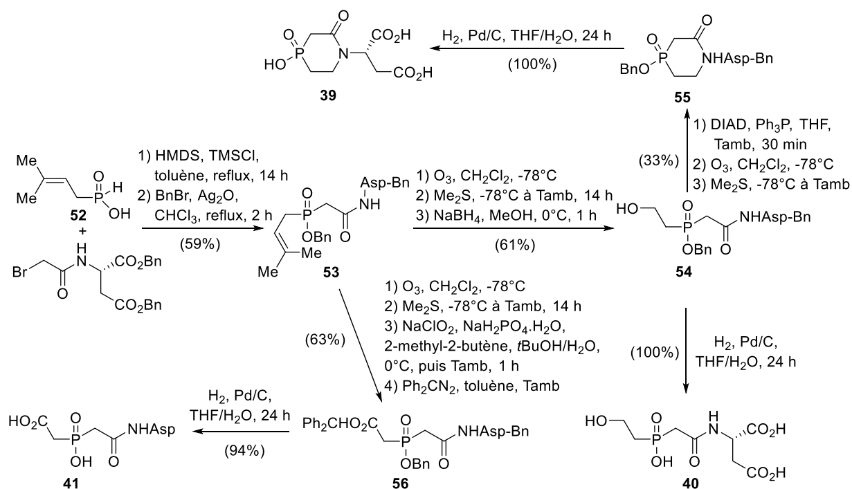
Schéma 1.7 : Synthèse des analogues phosphiniques 39 , 40 et 41 du PALA.
