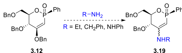
Schéma 3.27 : Formation envisagées des énaminophosphinates 3.19 à partir de l'oxaphosphinane insaturé 3.12 .
