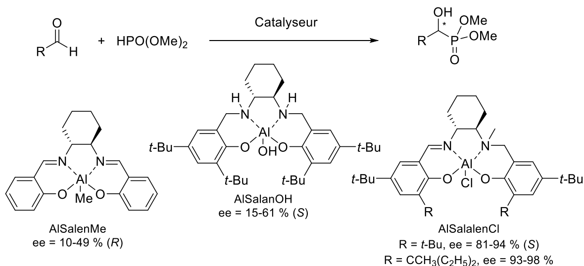
Schéma 2.13 : Utilisation des complexes d'aluminium avec ligands Salen, Salan et Salalen dans l'hydrophosphonylation asymétrique d'aldéhyde.
