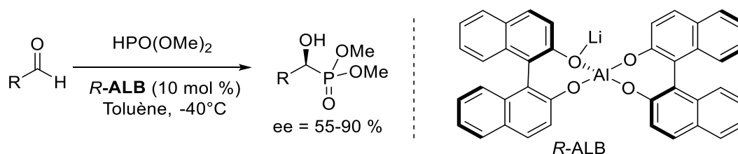
Schéma 2.11 : L'hydrophosphonylation asymétrique d'aldéhydes catalysée par le R -ALB.
