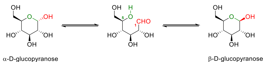
Figure 1 : Les formes anomériques du glucose.
