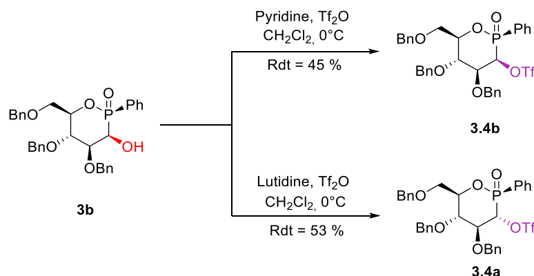
Schéma 3.6 : Synthèse de l'ester triflique à partir de l'alcool 3b .
