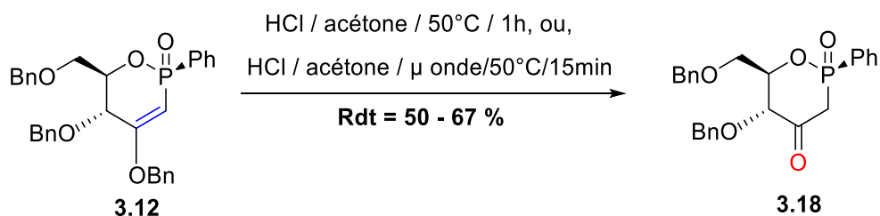
Schéma 3.26 : Conditions retenues pour la réaction d'hydrolyse de l'oxaphosphinane 3.12 .
