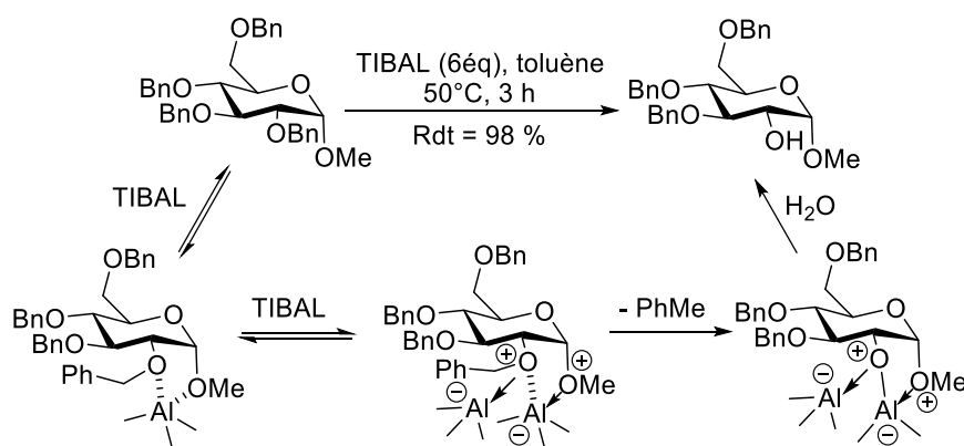
Schéma 2.25 : Débenzylation régiosélective utilisant le TIBAL.
