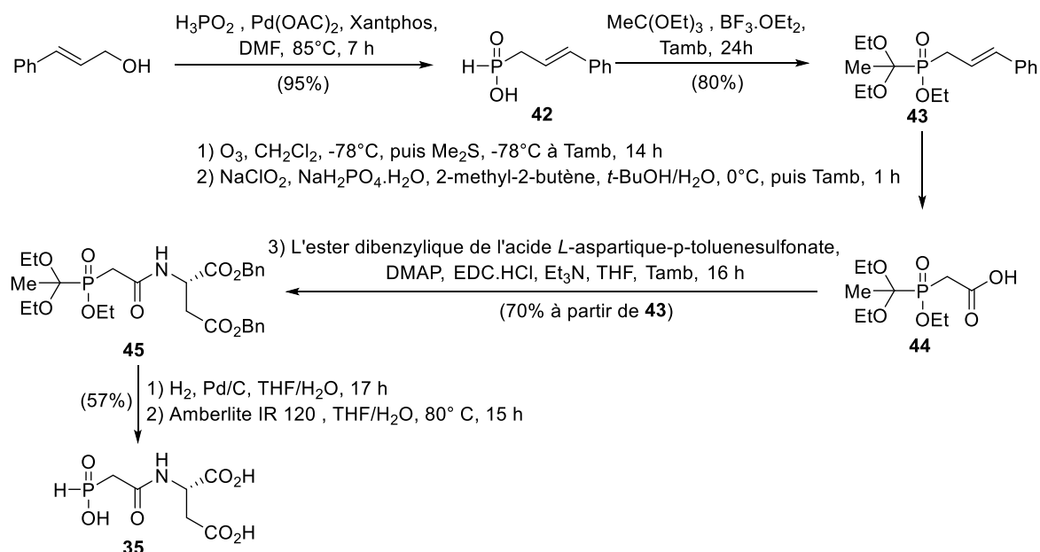
Schéma 1.4 : Synthèse de l'analogue phosphinique 35 du PALA.
