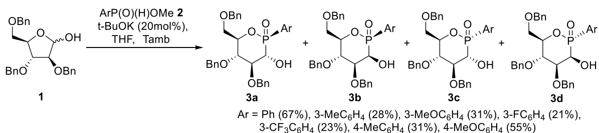
Schéma 1 : Schéma général de synthèse des phostines 3a-d .
