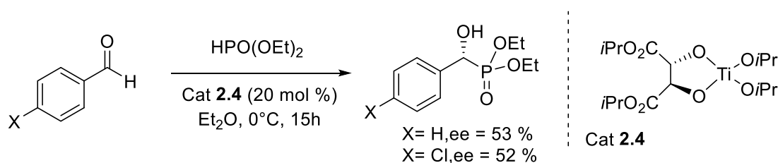
Schéma 2.6 : Hydrophosponylation asymétrique d'aldéhydes par le catalyseur de titane 2.4.
