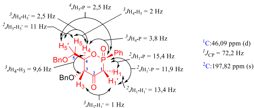
Figure 3.12 : Constante de couplage J_{\text{H-H}} et J_{\text{H-P}} avec les déplacements chimiques des carbones C 1 et C 2 du \beta -cétophosphinate 3.18 .
