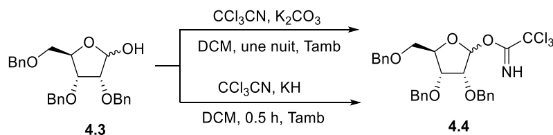
Schéma 4.6 : Préparation du sucre donneur 4.4 .
