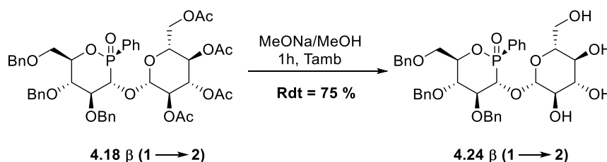
Schéma 4.21 : Déacétalysation à partir du pseudo-disaccharide 4.18 \beta (1 \rightarrow 2).
