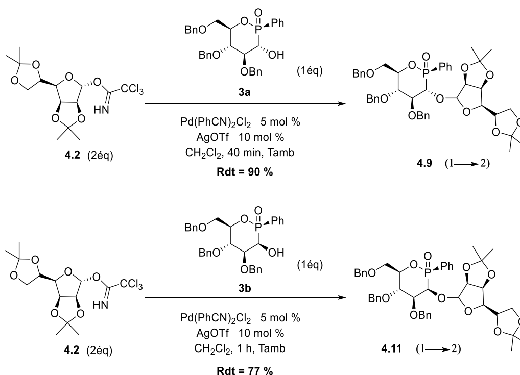
Schéma 4.14 : Synthèse des pseudo-disaccharides 4.9 ( 1 → 2 ) et 4.11 ( 1 → 2 ).
