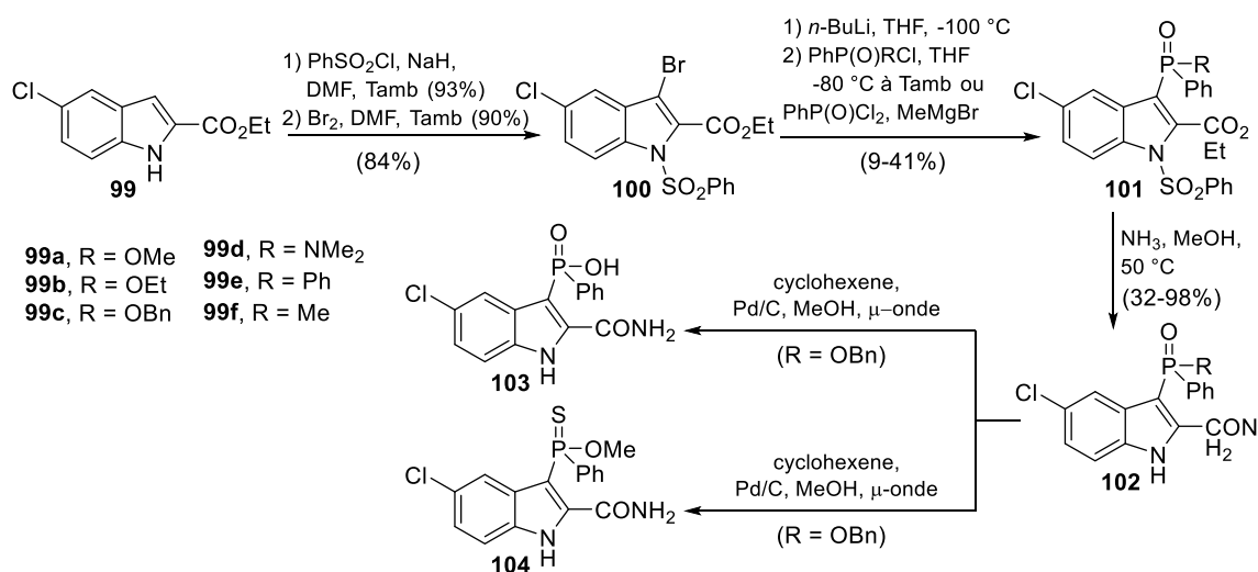
Schéma 1.12 : Synthèse de quelques phospho-indoles comme INNTI.
