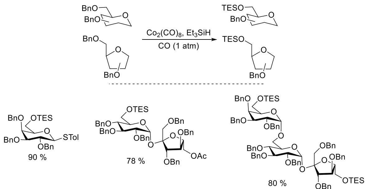
Schéma 2.23 : Débenzylation régiosélective selon la méthode de Yin.
