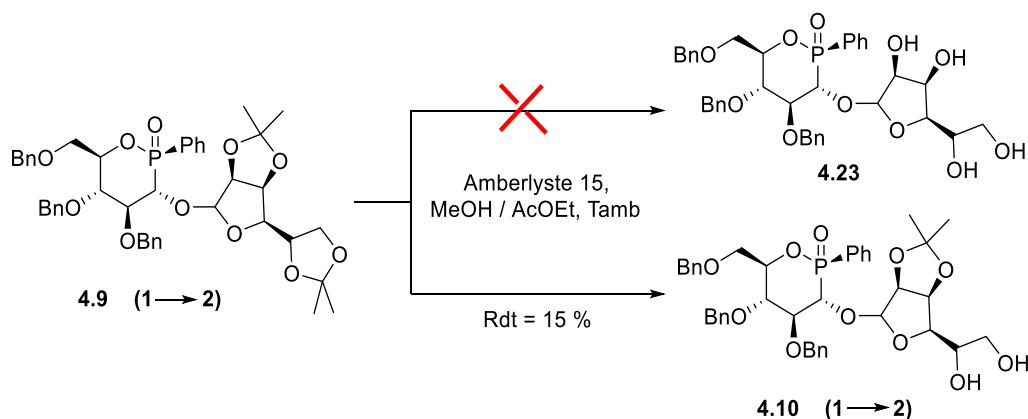
Schéma 4.20 : Hydrolyse des groupements isopropylidène du pseudo-disaccharide 4.9 (1→2).
