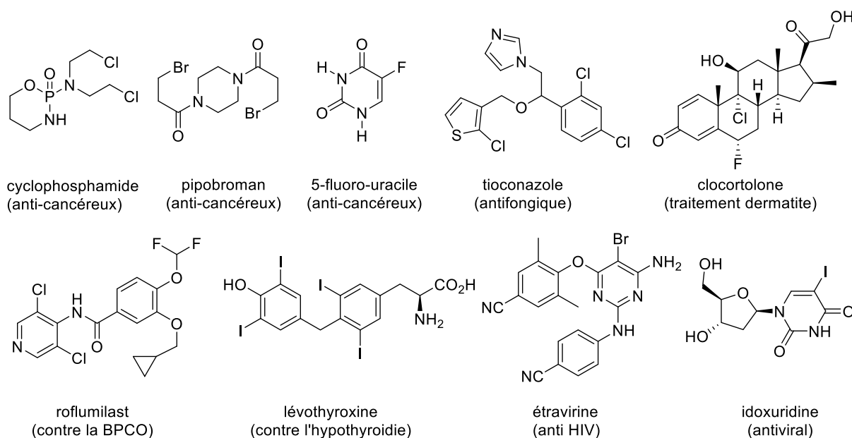
Figure 3.1 : Exemple de produits halogénés utilisés en chimie médicinale.
