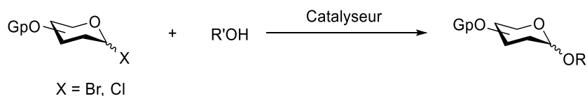
Schéma 4.1 : Glycosylation selon Koenigs et Knorr.
