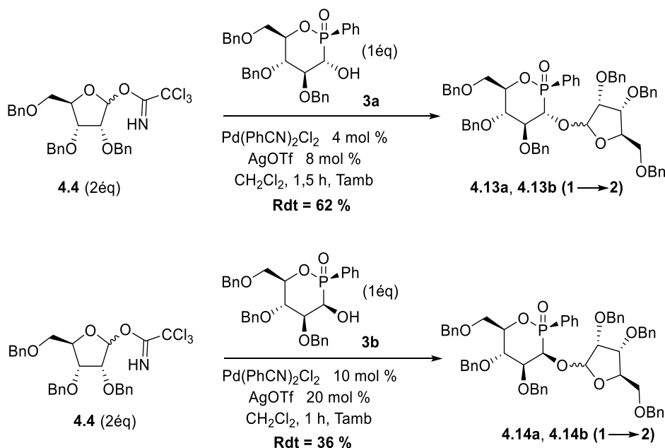
Schéma 4.13 : Synthèse des pseudo-disaccharides 4.13 (1→2) et 4.14 (1→2) .
