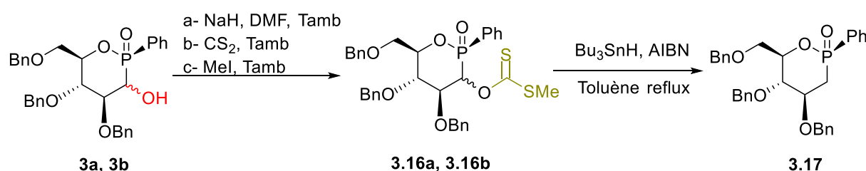
Schéma 3.20 : Synthèse de phostine \alpha -déhydroxylée.
