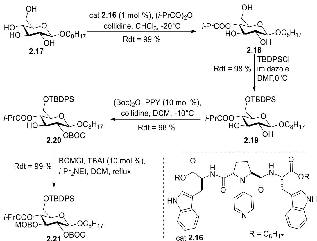
Schéma 2.16 : Exemple de protection régiosélective d'un glucopyrannose.
