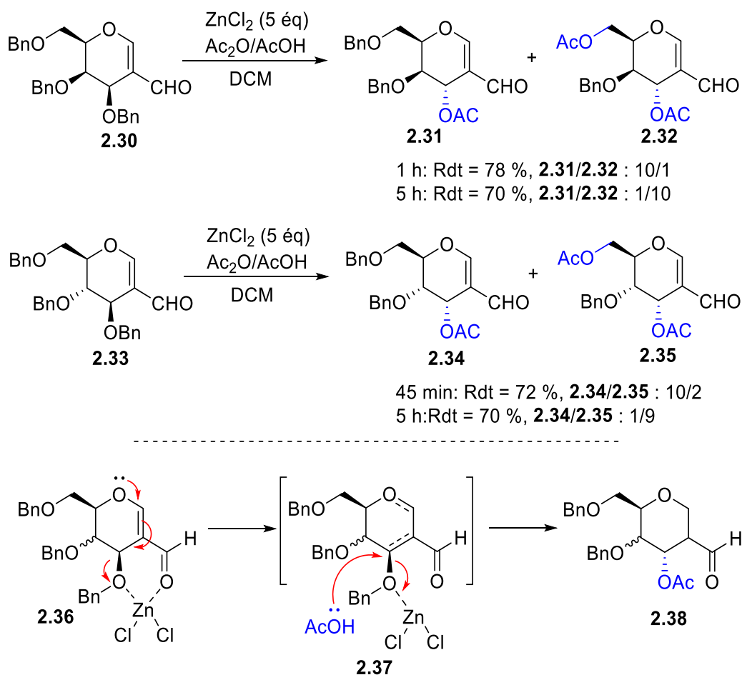
Schéma 2.20 : Débenzylation régiosélective de 2-formyl glycols catalysée par le chlorure de zinc, avec le mécanisme de déprotection.
