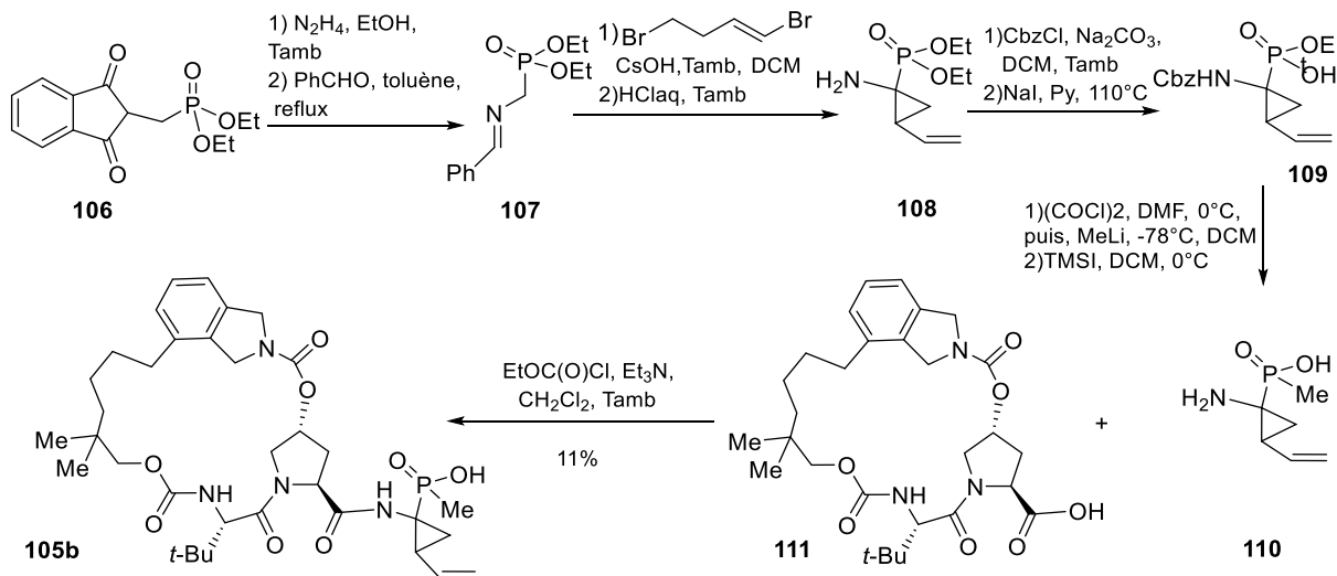
Schéma 1.13 : Synthèse de l'analogue phosphinate 105b du MK-7009.
