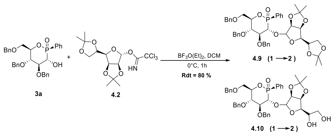
Schéma 4.9 : Couplage entre la phostine 3a et le sucre donneur 4.2 catalysé par le trifluorure de bore.
