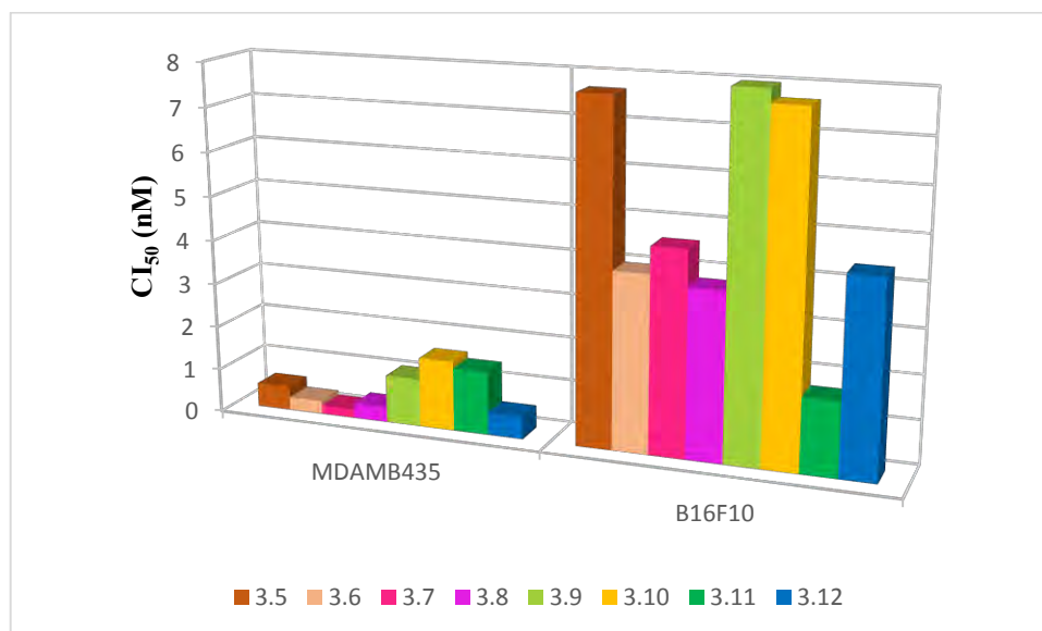
Figure 3.6 : Valeurs des IC 50 des phostines synthétisées 3.5 à 3.12 sur les lignées cellulaires MDAMB435 et B16F10.
