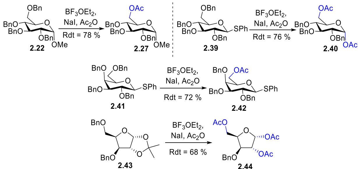
Schéma 2.21 : Débenzylation régiosélective par acétylation selon Brar et Vankar.
