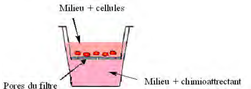
Figure 3.9 : Principe de la migration cellulaire en chambre de Boyden.
