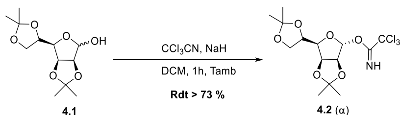
Schéma 4.5 : Préparation du sucre donneur 4.2 .
