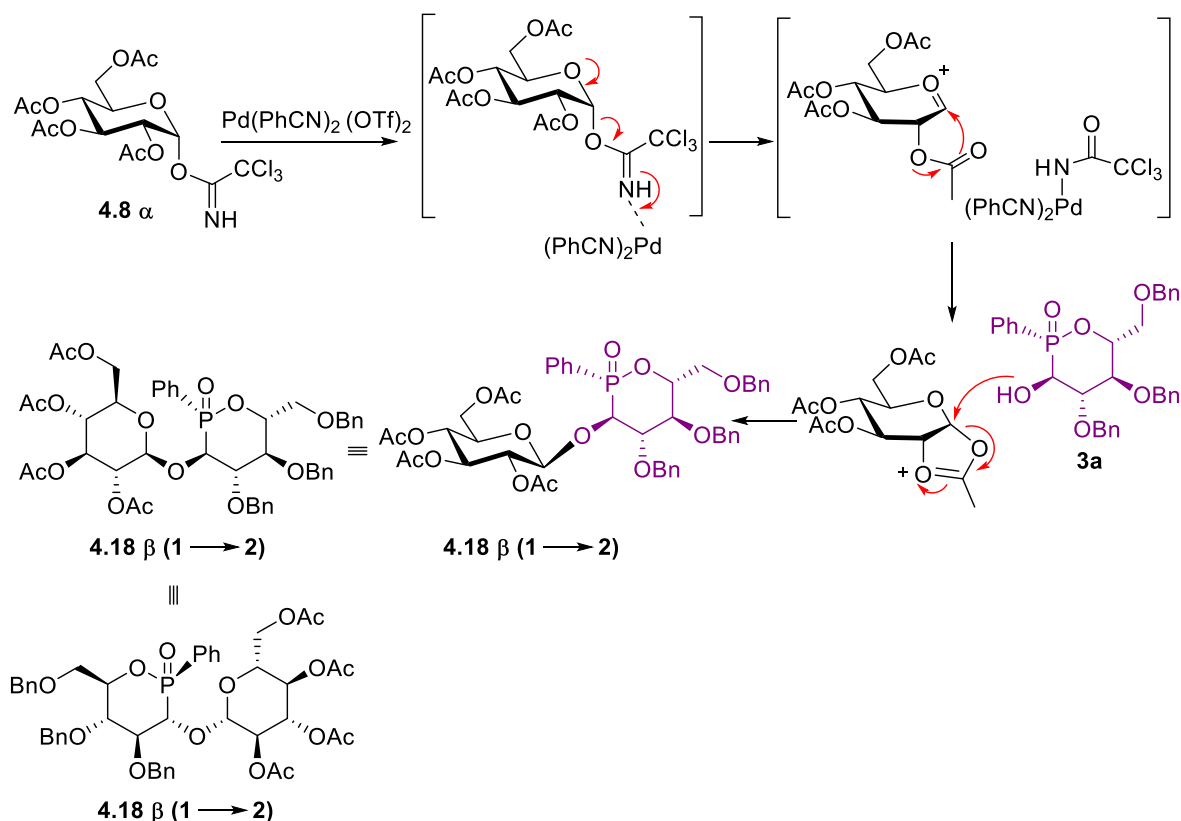
Schéma 4.17 : Mécanisme pour la formation de pseudo-disaccharide 4.18 β (1→2) .
