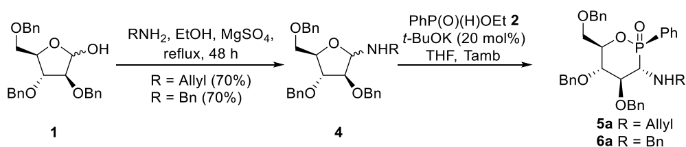
Schéma 2 : Synthèse directe des amino oxaphosphinanes 5a et 6a .
