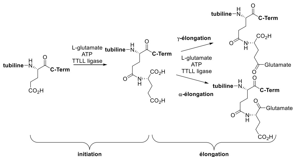
Figure 1.9 : Les étapes de la polyglutamylation catalysées par les TTLL.
