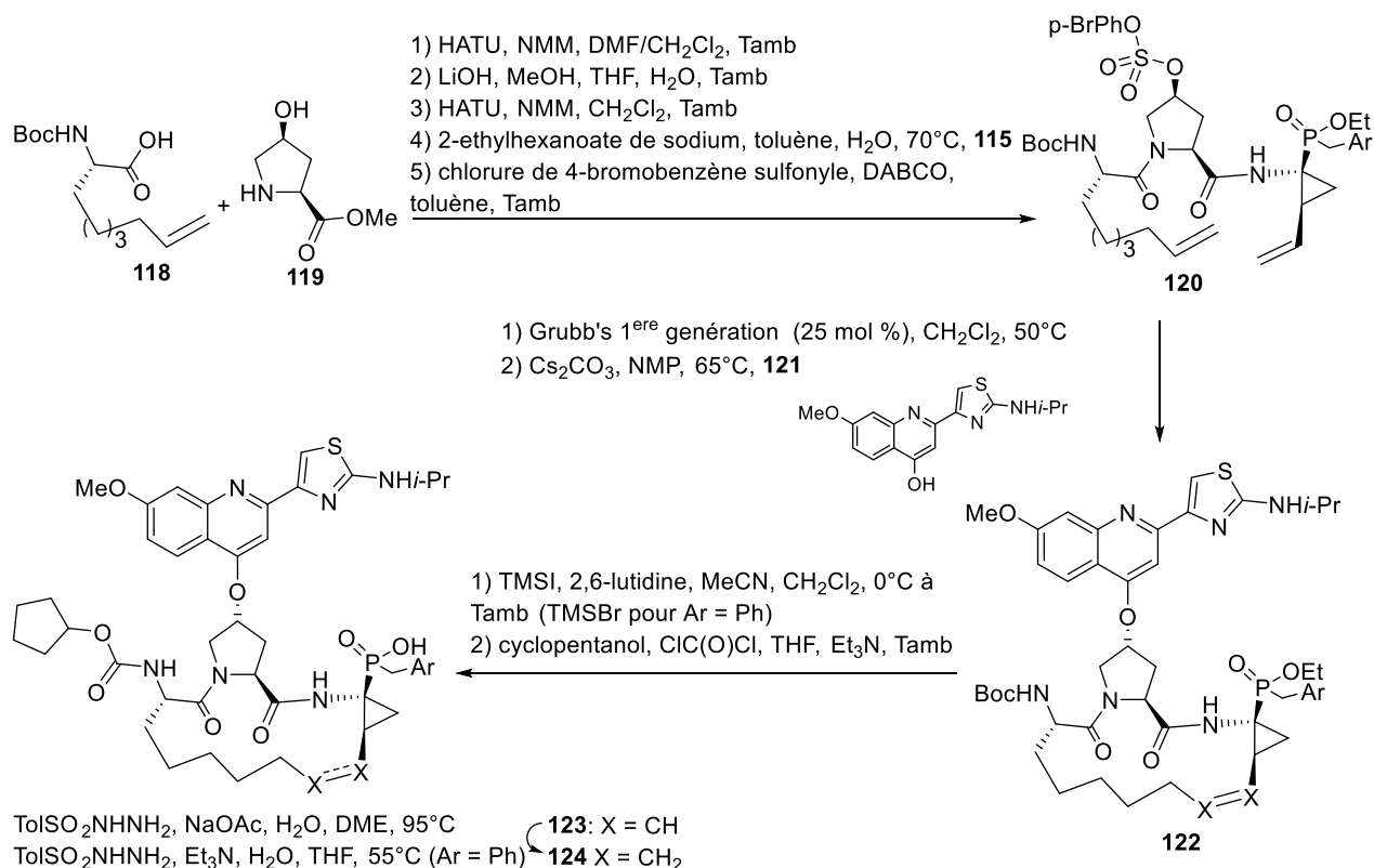
Schéma 1.16 : Préparation des analogues phosphinates macrocycliques 123 et 124 .
