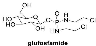
Figure 4.3 : Glufosamide, glycoconjugué à activité anticancéreuse.
