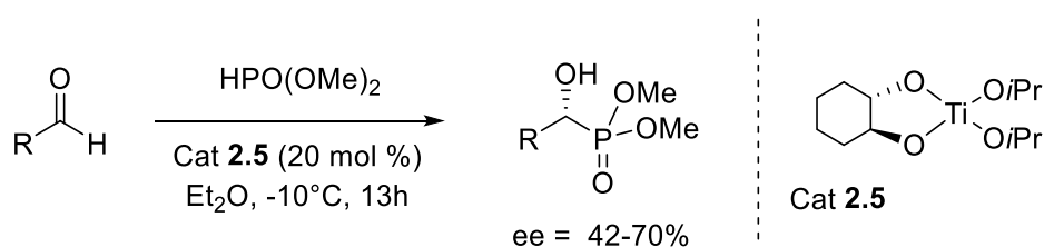
Schéma 2.7 : Hydrophosponylation asymétrique d'aldéhydes par le catalyseur 2.5.
