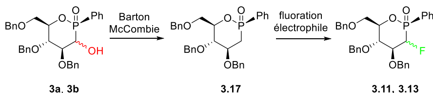
Schéma 3.19 : Fluoration à partir du phosphinosucre \alpha -déhydroxylé 170 .
