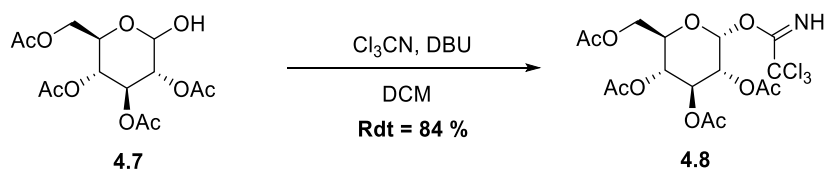
Schéma 4.8 : Préparation du sucre donneur 4.8 .
