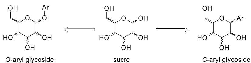
Figure 2 : Sucre, O- et C-aryl glycoside.
