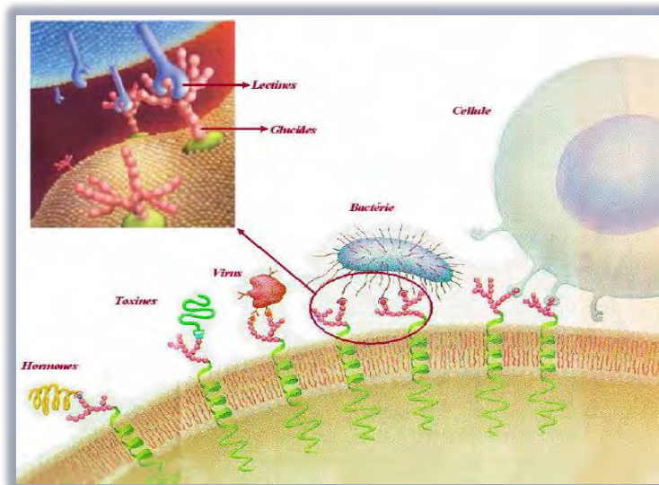
Figure 4.1 : Rôle des glycoconjugués cellulaires périphériques.
