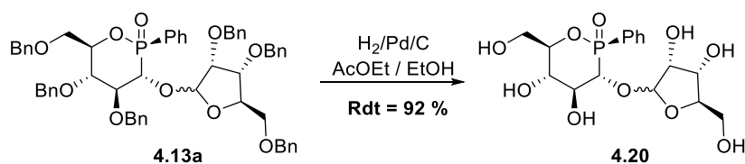
Schéma 4.18 : Déprotection à partir du pseudo-disaccharide 4.13a .
