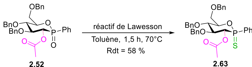
Schéma 2.36 : Synthèse de la thiophostine 2.63 .
