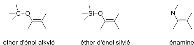
Figure 3.11 : Structures chimiques des éthers d'énol et des énamines.
