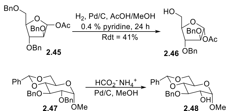
Schéma 2.22 : Débenzylation régiosélective par hydrogénolyse.
