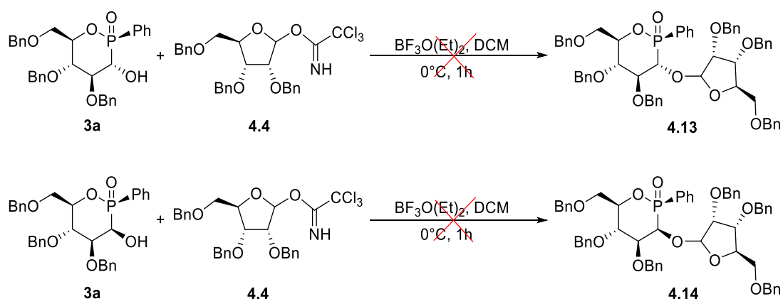
Schéma 4.11 : Tentatives de couplages entre les phostines 3a et 3b avec le sucre donneur 4.4 catalysé par le trifluorure de bore.
