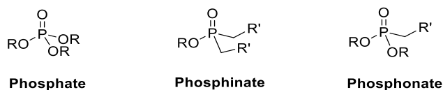
Figure 1.1 : Les phosphates et leurs formes réduites, les phosphinates et les phosphonates.
