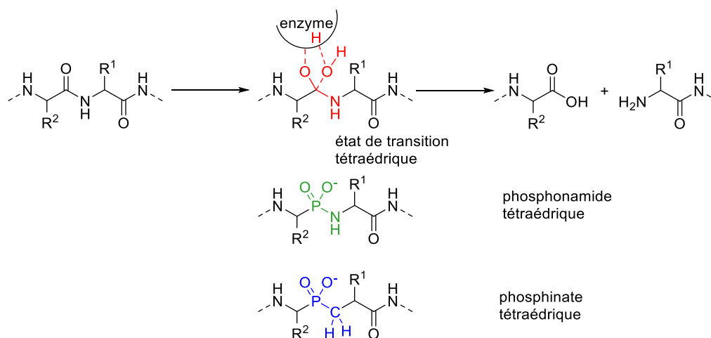
Figure 1.3 : Analogie entre une fonction phosphonamide et l'état de transition tétraédrique d'une hydrolyse de peptides catalysée par les protéases.
