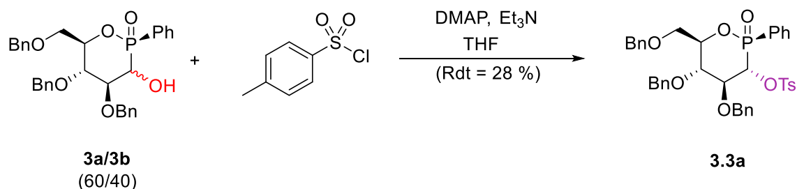
Schéma 3.4 : Synthèse du dérivé tosylate à partir du mélange d'alcools 3a/3b .
