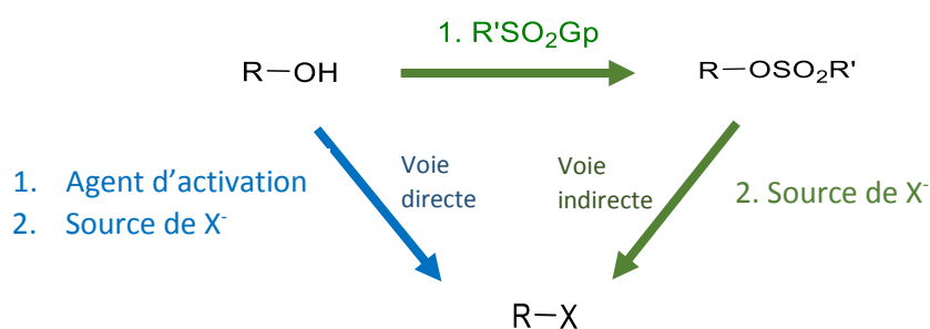
Schéma 3.1 : Voies d'halogénéation à partir d'un groupement hydroxyle.
