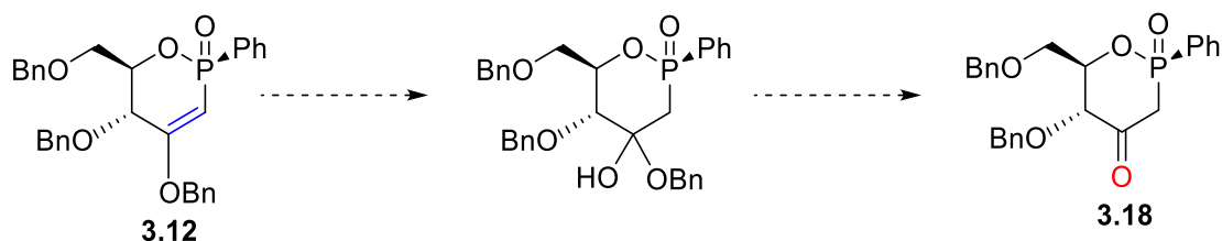
Schéma 3.25 : Réaction d'hydrolyse envisagée pour la formation de dérivé \beta -cétophosphate 3.18 .
