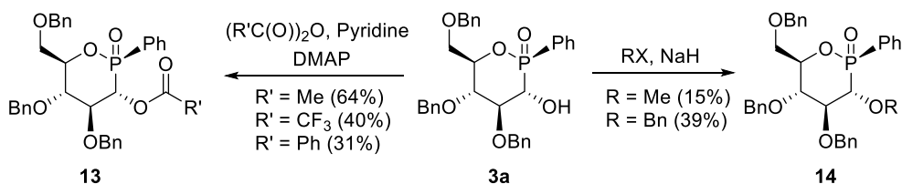
Schéma 4 : Synthèse de phosphinosucres 13 et 14 .
