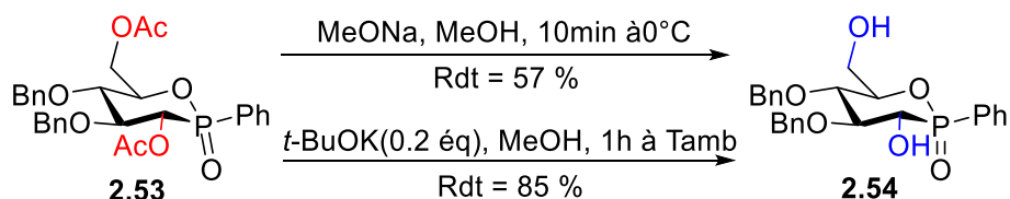
Schéma 2.31 : Désacétylation de la phostine 2.53 .
