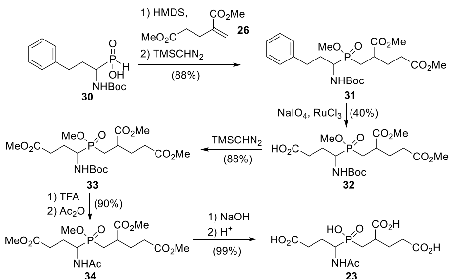
Schéma 1.3 : Synthèse de l'inhibiteur 23 .
