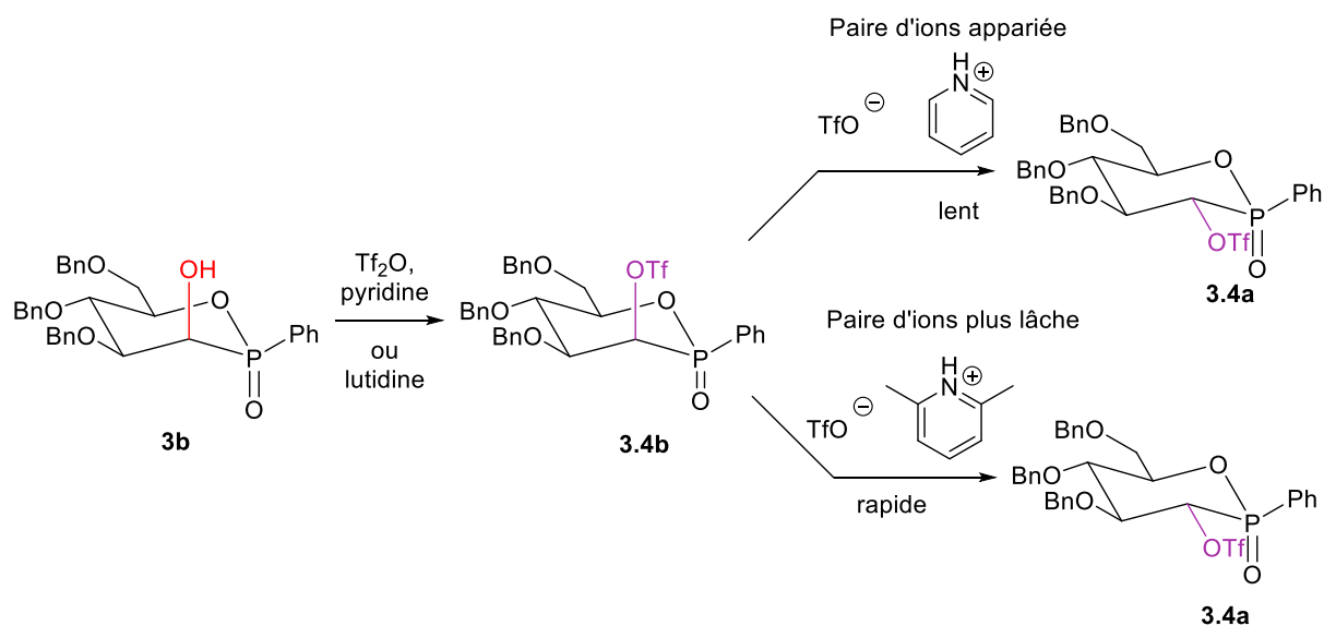
Schéma 3.7 : Explication possible de l'inversion de stéréosélectivité observée avec la lutidine.
