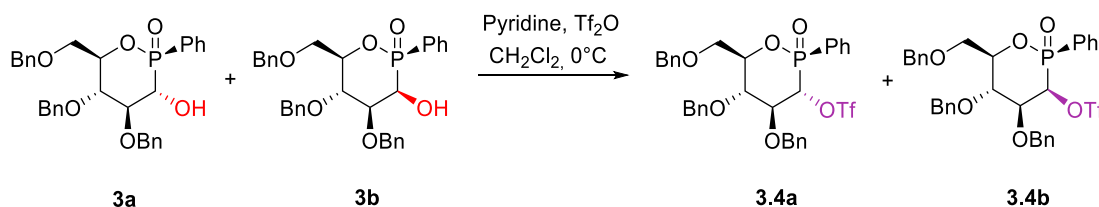
Schéma 3.5 : Synthèse de l'ester triflique à partir du mélange d'alcools 3a et 3b .
