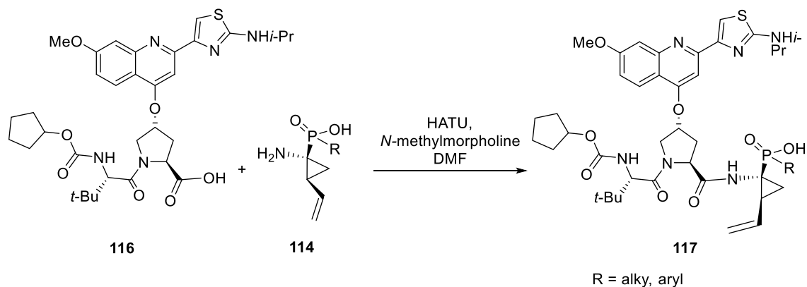
Schéma 1.15 : Préparation des analogues phosphinates acycliques 117 .
