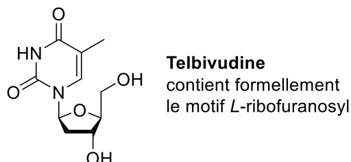
Figure 2.8 : Exemple de médicament à base de sucre lévogyre.
