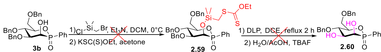
Schéma 2.34 : Essai de synthèse du diol 2.60 par débenzylation radicalaire.
