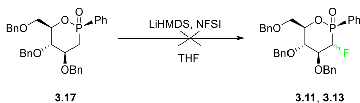
Schéma 3.21 : Essai de fluoration de la phostine \alpha -déhydroxylée.
