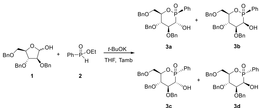
Schéma 2.1 : Synthèse des phostines via le D -arabinofuranose O -benzylé.
