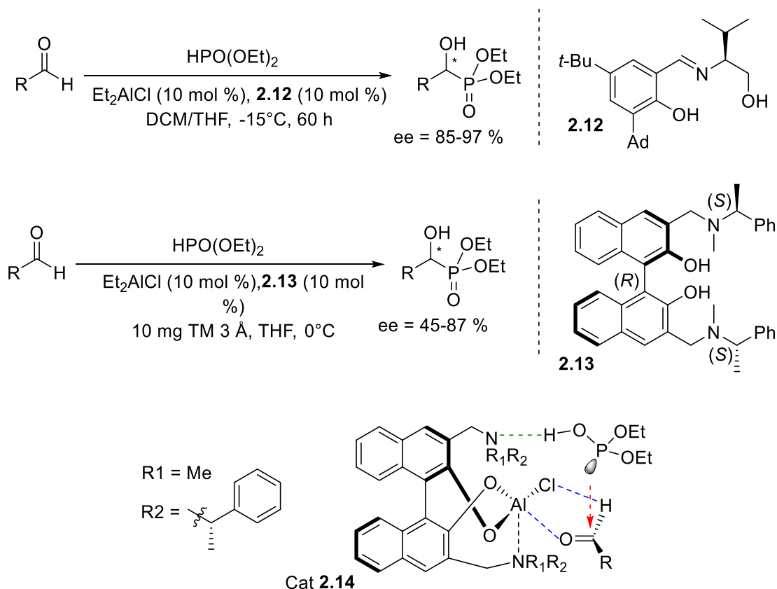
Schéma 2.14 : Hydrophosphonylation asymétrique d'aldéhyde par des complexes d'aluminium développée par Feng.
