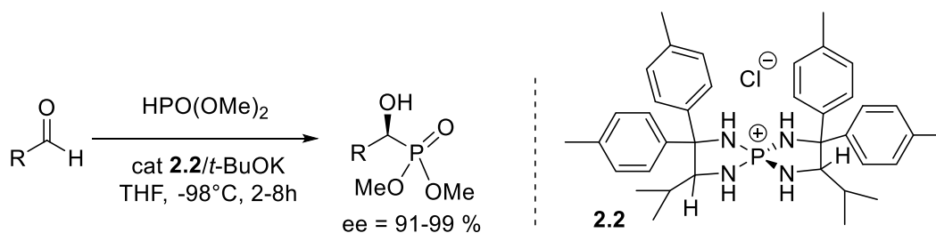
Schéma 2.4 : Hydrophosphonylation asymétrique d'aldéhydes catalysée par le sel de phosphonium 2.2 .
