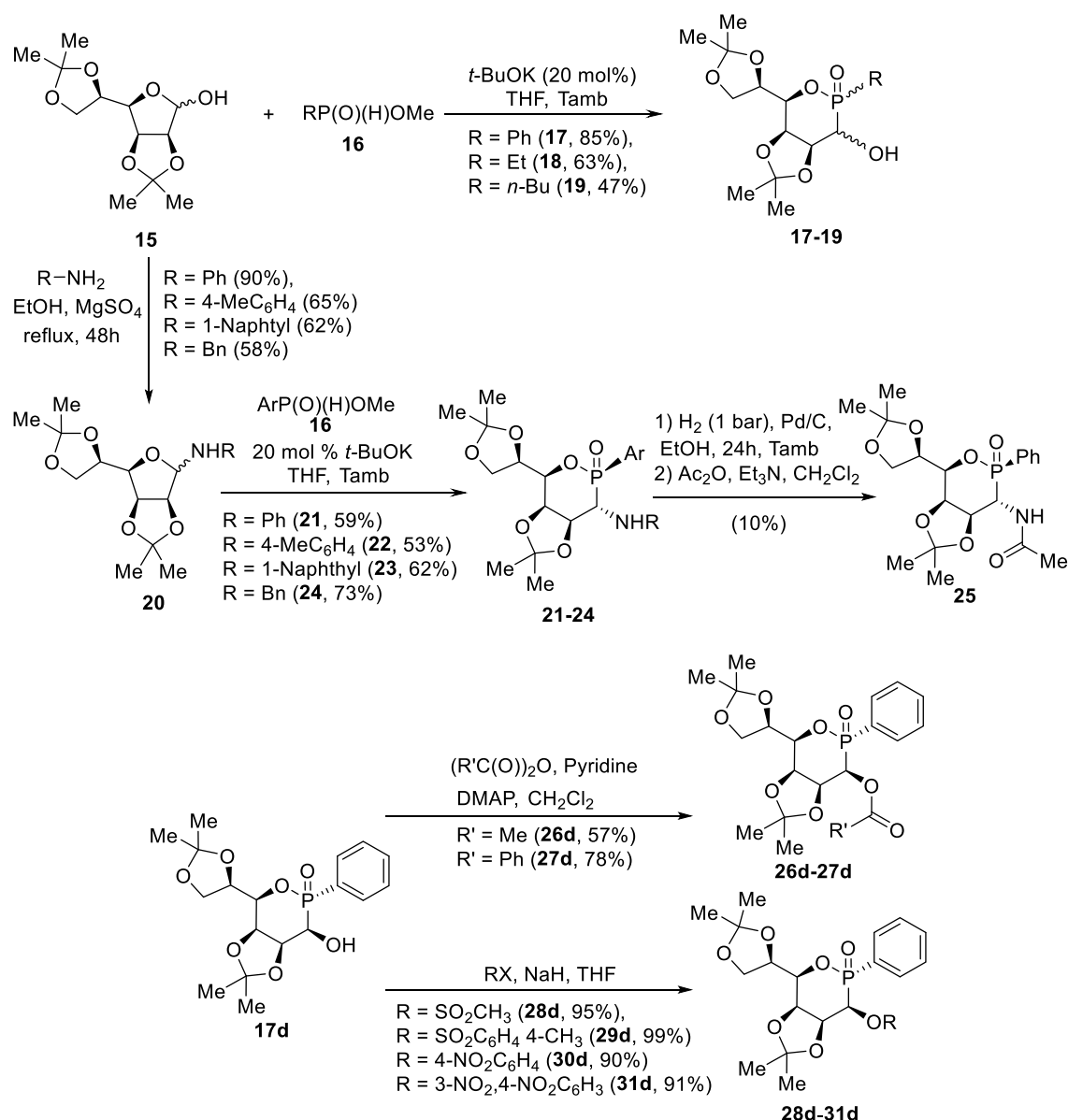
Schéma 5 : Synthèse d'analogues du D -glycero- D -talo-heptopyranose et diversification structurale.
