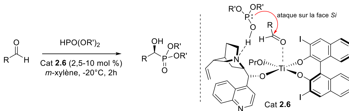
Schéma 2.8 : Hydrophosphonylation asymétrique d'aldéhydes par le catalyseur de titane 2.6 et l'état de transition proposé par You.
