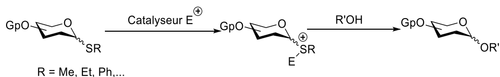
Schéma 4.3 : Méthode au thioglycoside.
