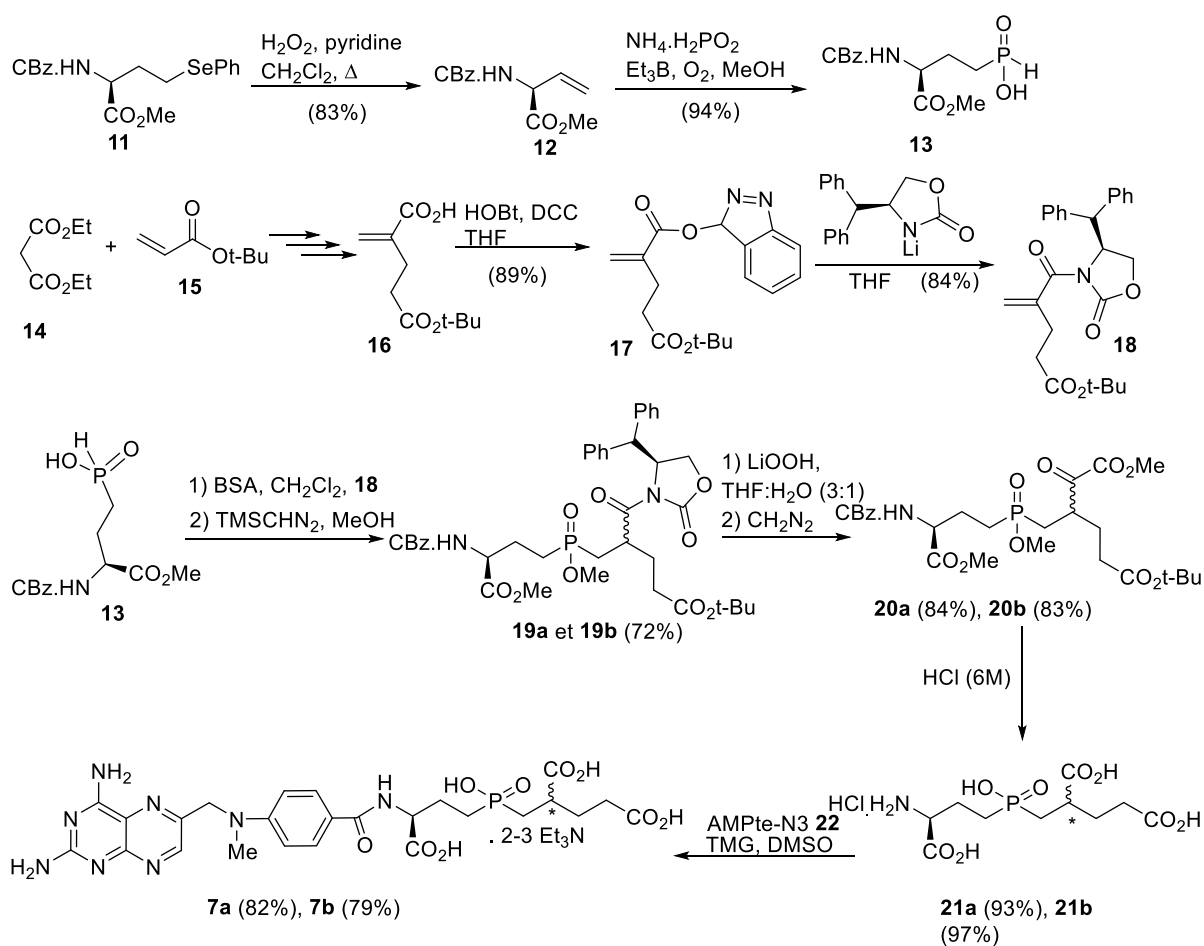
Schéma 1.1 : Synthèse des analogues phosphinates 7a , 7b .
