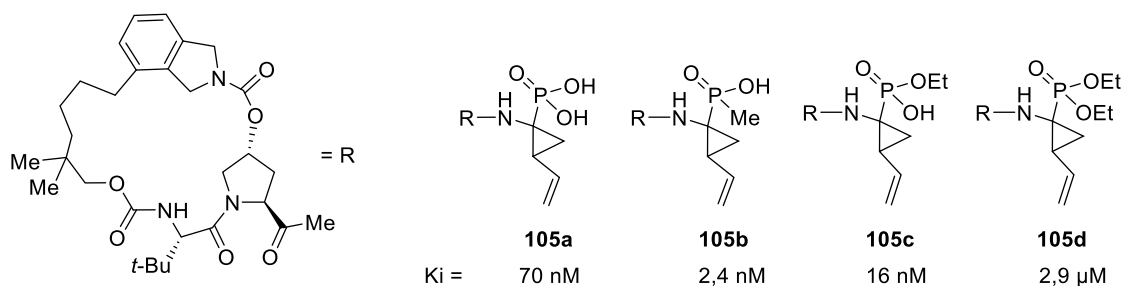
Figure 1.17 : Structures et valeurs de K_i de différents analogues du MK-7009 synthétisés.
