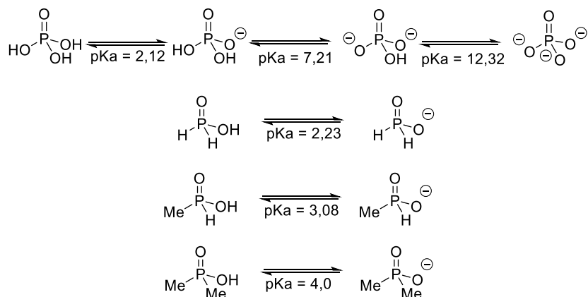
Figure 1.2 : Les pKa de l'acide phosphorique et quelques acides phosphiniques.
