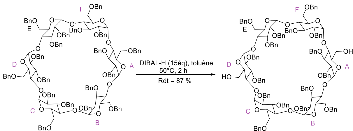
Schéma 2.26 : Utilisation du DIBAL-H dans la double débénylation sélective des cyclodextrines.
