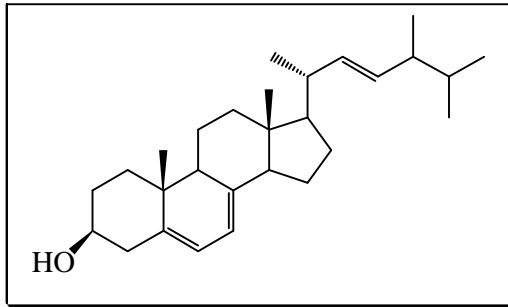
الصيغة 21 : Ergostérol
