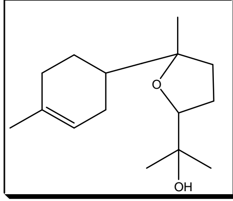
الصيغة 9.2 : Bisabolol oxide B
