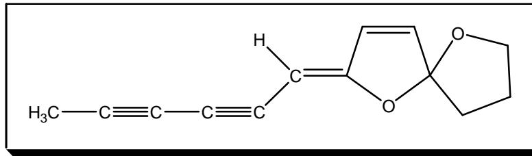
الصيغة 10.2 : cis-Spiroether
