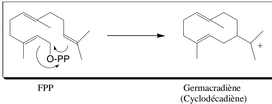
الشكل 23.1 : الاصطناع الحيوي لهيكل الجرماكرانوليد.
