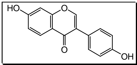
diadzène
