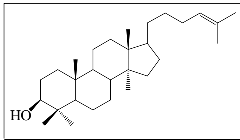
الصيغة 24 : lanostérol
