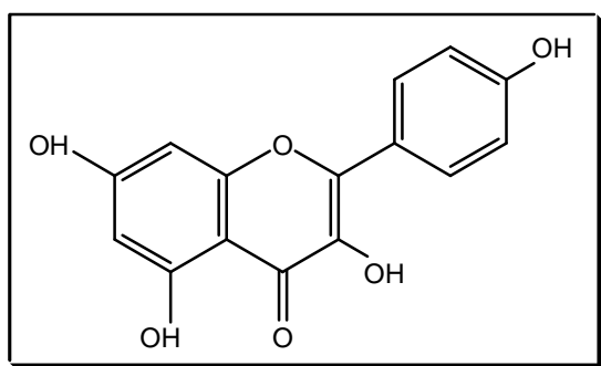
الصيغة 13.2: Kaempférol
