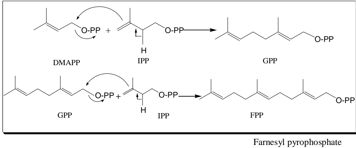
الشكل 22.1: الاصطناع الحيوي لـ FPP.
