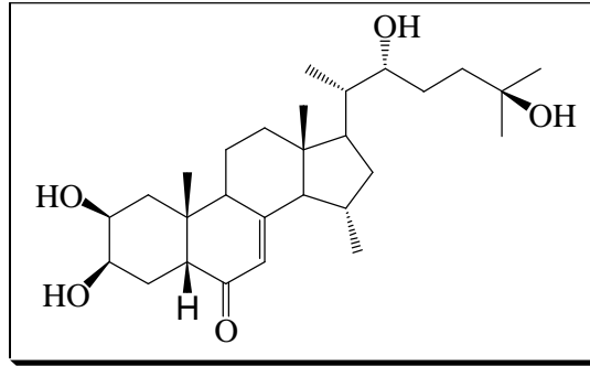
الصيغة 23 : Ecdysone
