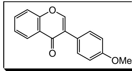
formononétine
