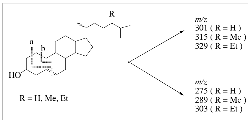
الشكل 37.1: أهم الإنشطار التي تحدث على الحلقتين A و B في المركبات 3 b - hydroxy - \Delta^5 - stérols
