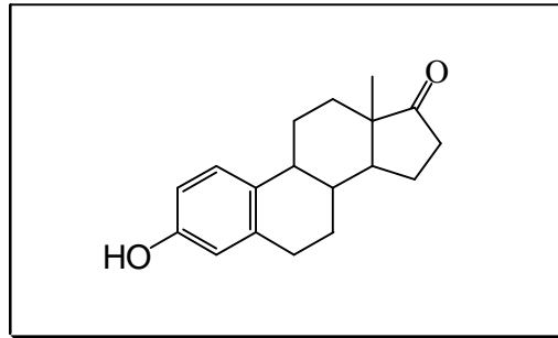
الصيغة 20 : Estrone
