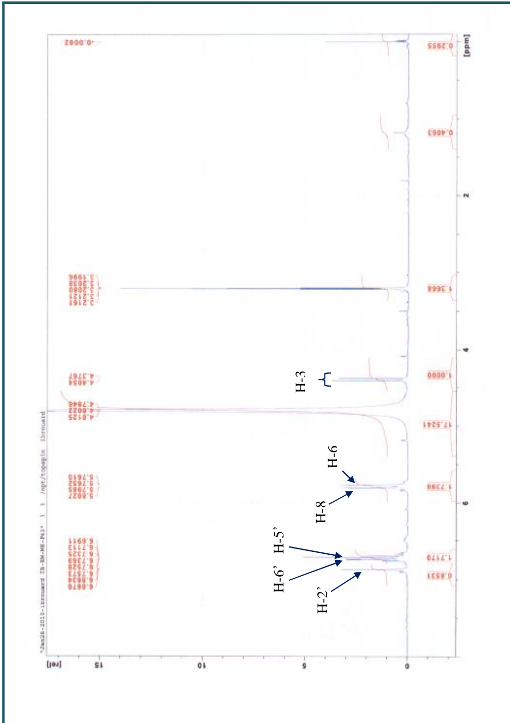
الطيف (27) : طيف ^1\text{H} RMN ( \text{CD}_3\text{OD} , 400 MHz) للمركب F 4-2
