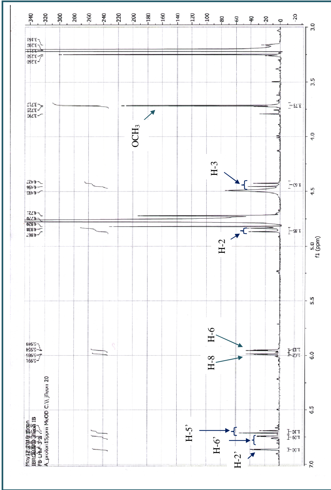
الطيف ( 24 ) : طيف 1 H RMN (CD 3 OD) للسر كـ 2-F 3
