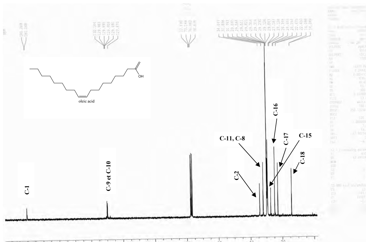
Figure-65 : Spectre RMN-C 13 (63MHz, CDCl 3 , \delta ppm) du produit F 19-24
