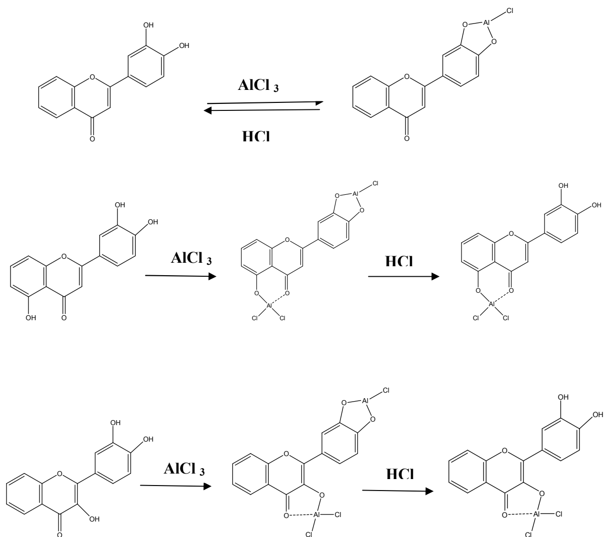
Figure-12 : Formation de complexe avec \text{AlCl}_3 et \text{HCl} .
