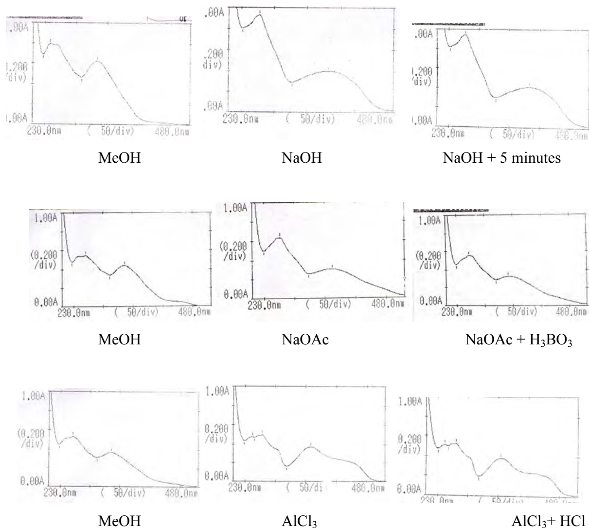
Figure-42 : Spectres d'absorption UV-visible du produit F 13 .
