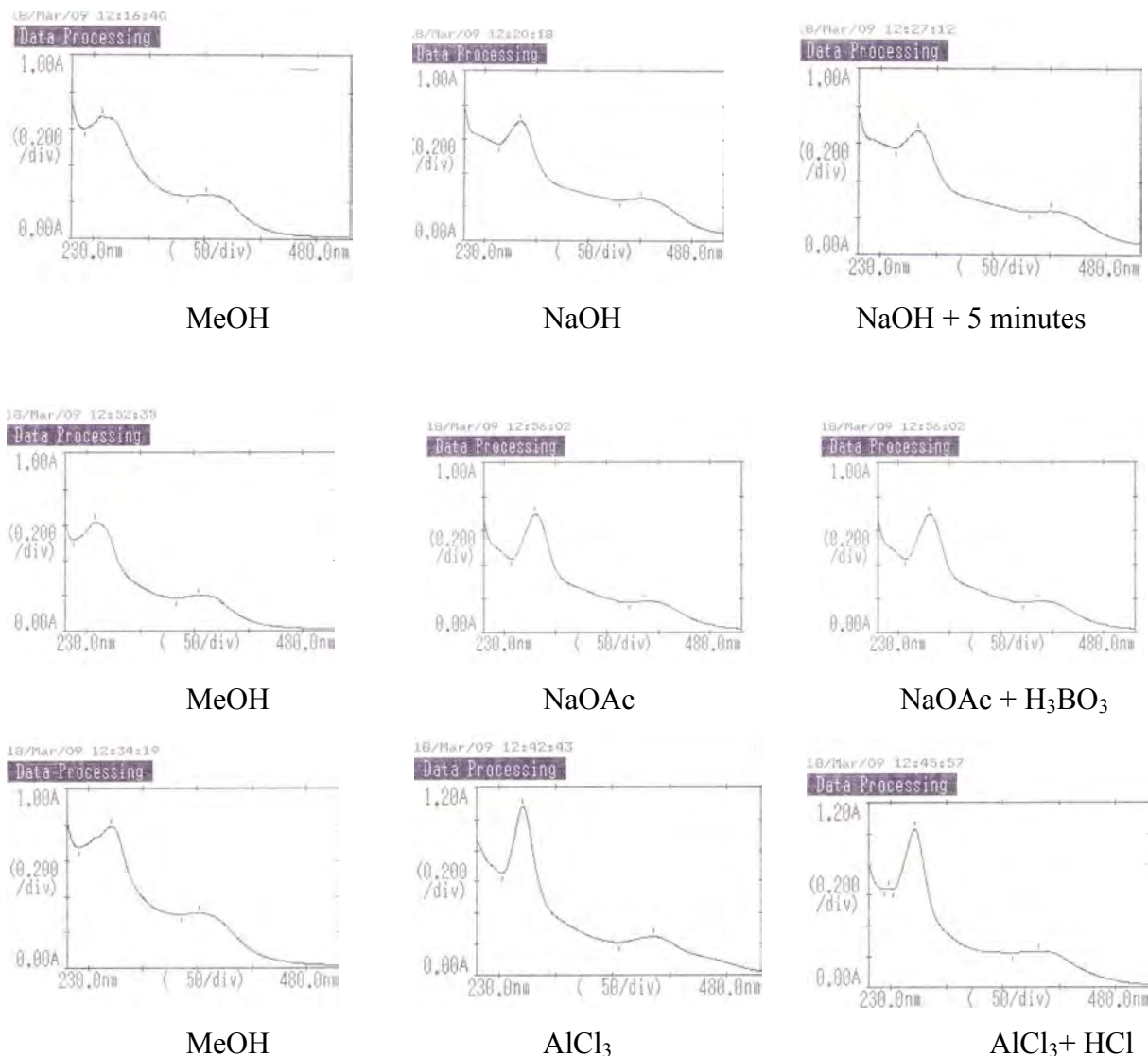
Figure-38 : Spectres d'absorption UV-visible du produit F_{e-1} .
