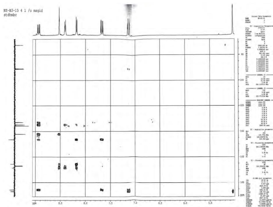
Figure-110 : Spectre HMBC (500MHz, CD 3 OD+ CF 3 COOD) du produit B 3-15.
