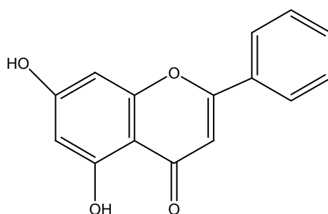
5,7-dihydroxyflavone (chrysin).
