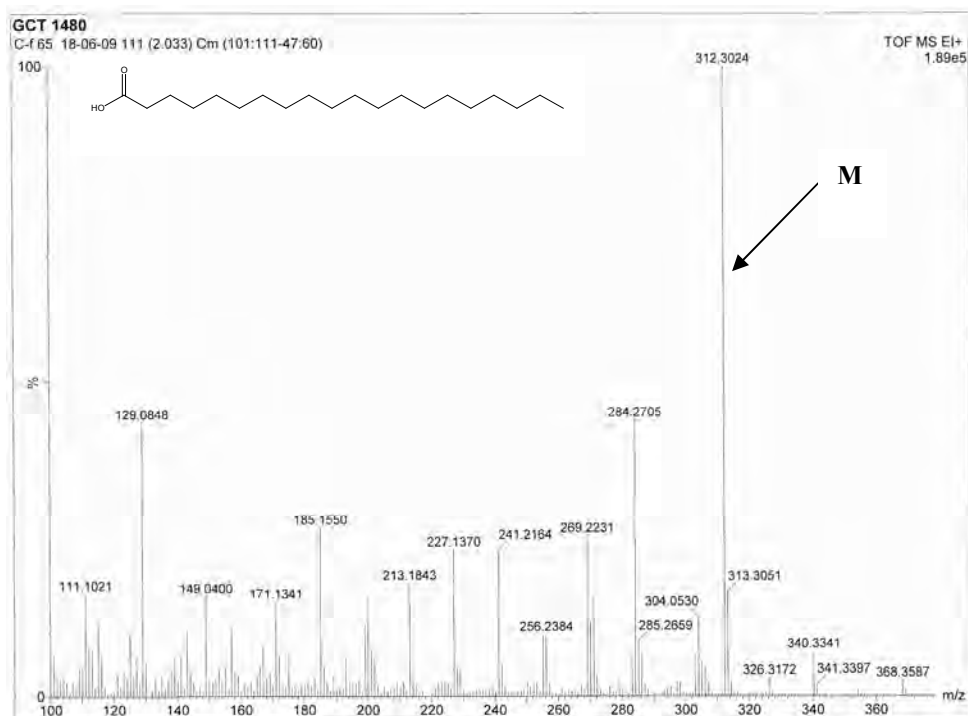
Figure-71 ; Spectre EI-MS du composé C-f65.
