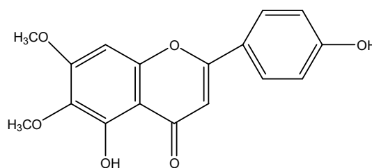
Circimaritine
