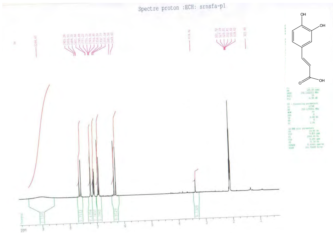
Figure-34: Spectre RMN-H 1 (250MHz, DMSO-d 6 , δ ppm) du produit F a-p1 .
