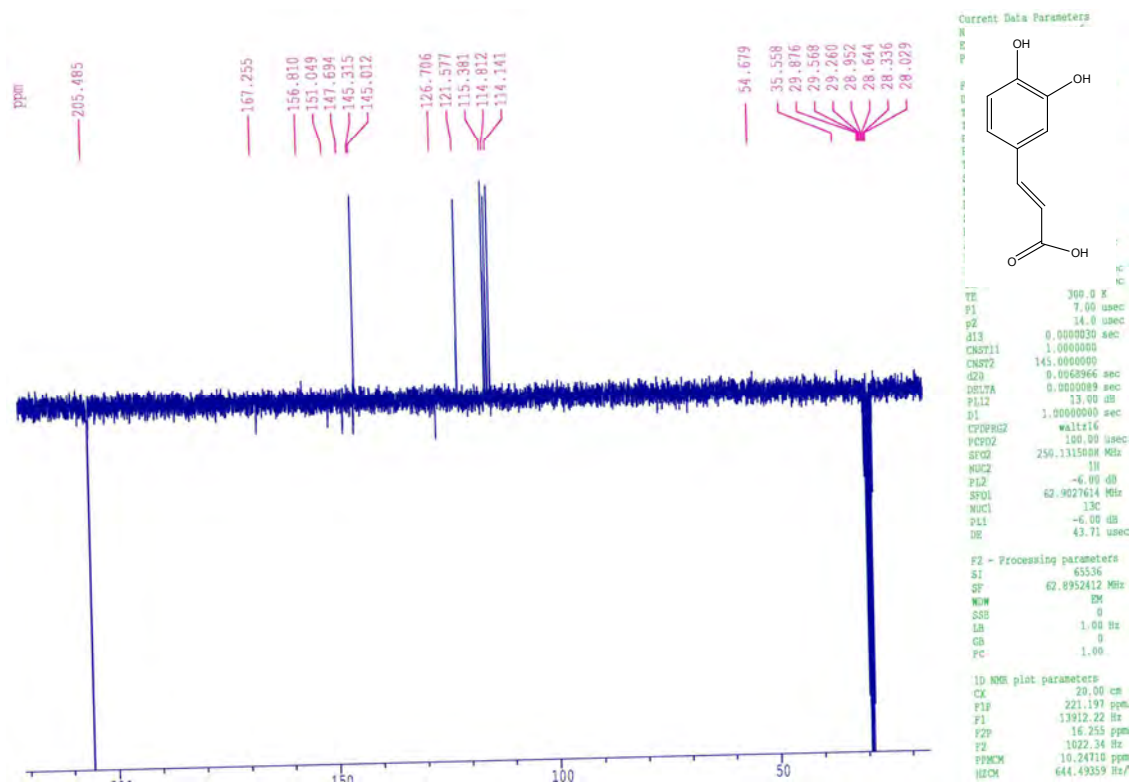
Figure-37 : Spectre J-mode (63MHz, DMSO-d 6 , δ ppm) du produit Fa-p 1 .
