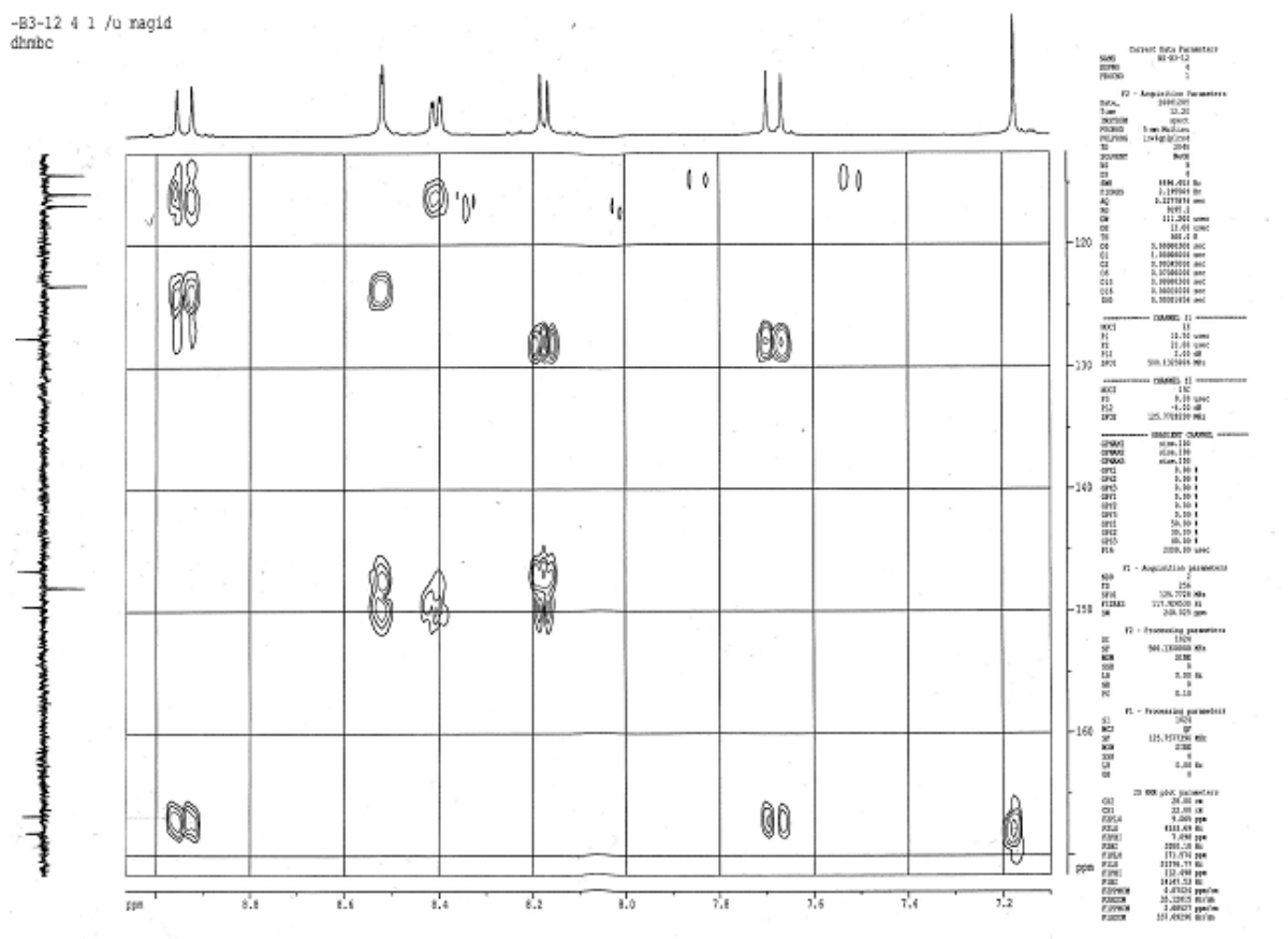
Figure-103 : Etalement du spectre HMBC (500MHz, CD 3 OD+ CF 3 COOD) du produit B 3 .
