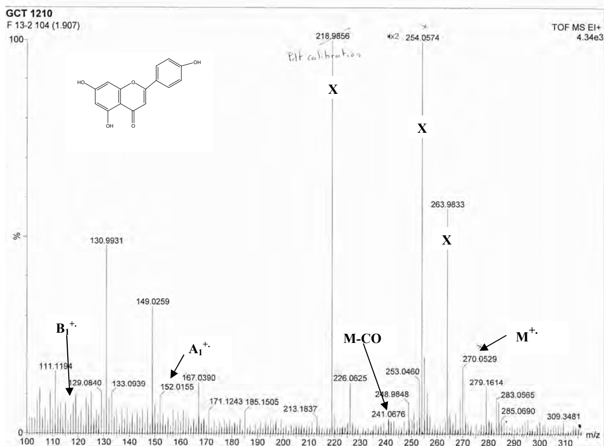
Figure-29 : Spectre de masse du produit F 13-2 .
