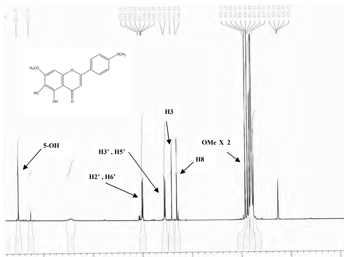
Figure-53: Spectre RMN- \text{H}^1 (250MHz, \text{DMSO-d}_6 , \delta ppm) du produit \text{F}_{14} .
