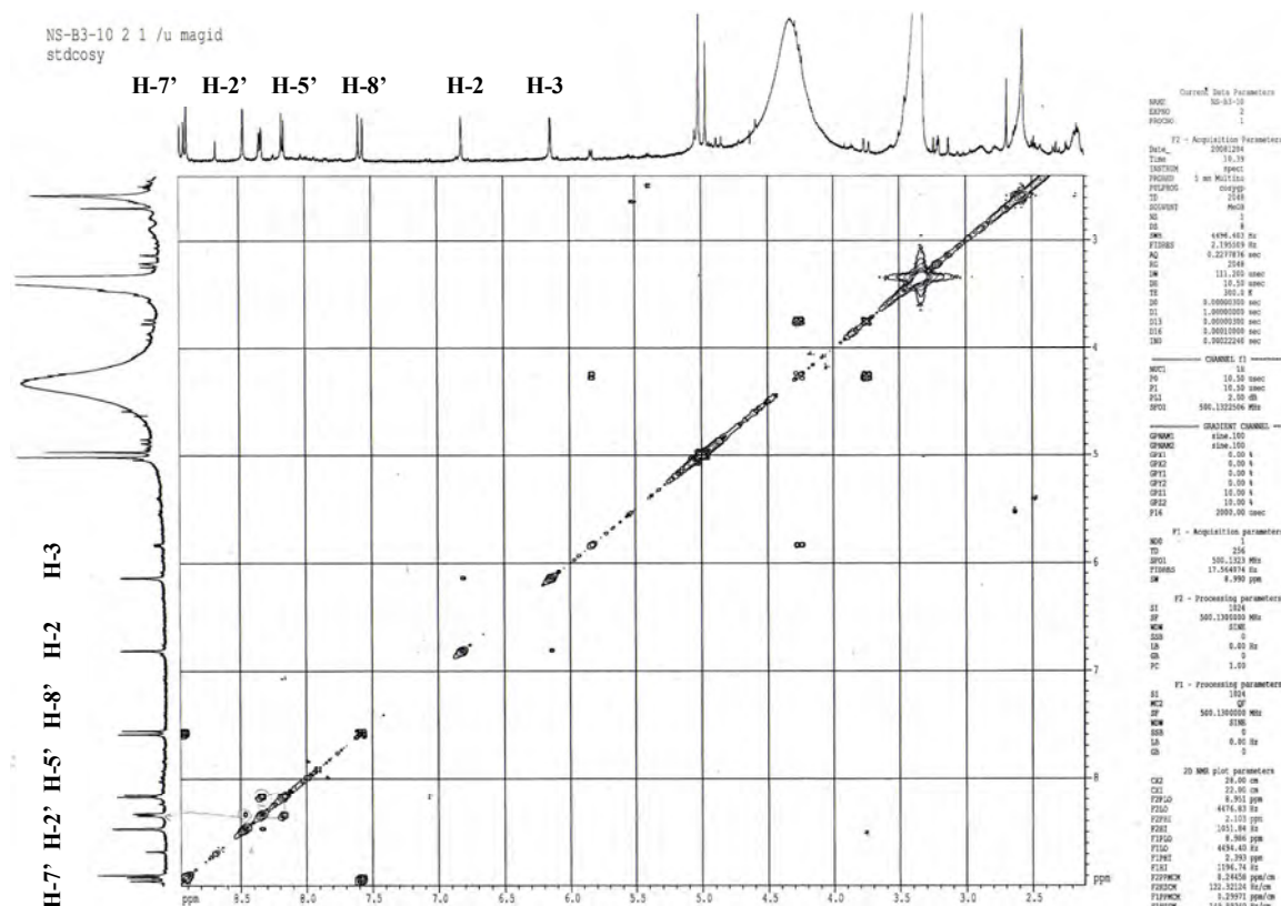
Figure-91 : Spectre COSY (500MHz, CD 3 OD) du produit B 3-10 .
