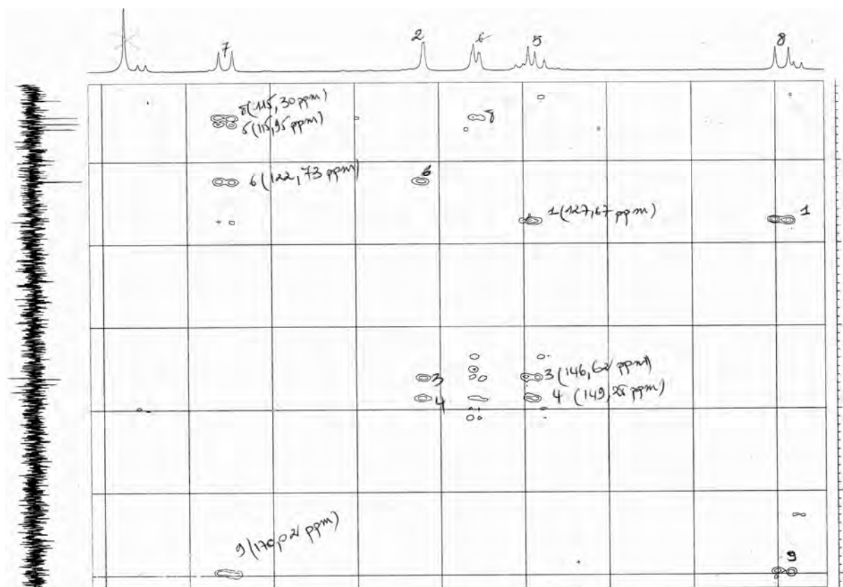
Figure-86 : étalement du spectre HMBC du produit B 3-8 .
