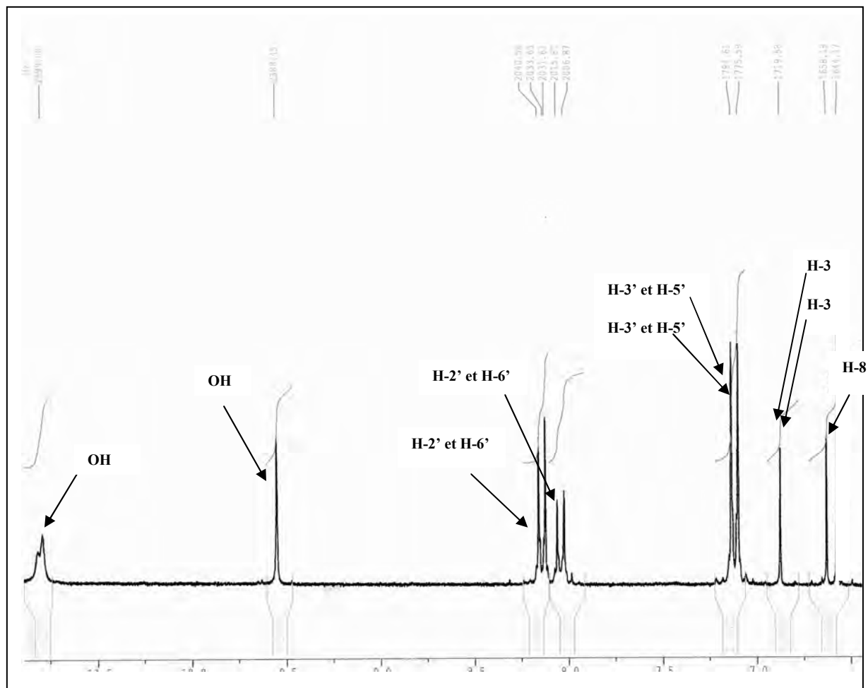
Figure-45 : Etalement du spectre RMN- H^1 du composé F_{13} .
