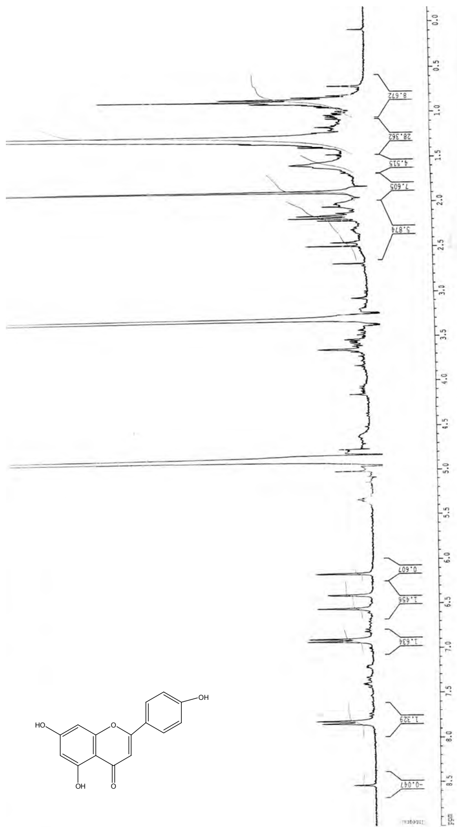
Figure-30: Spectre RMN-H 1 (250MHz, DMSO-d 6 , δ ppm) du produit F 13-2
