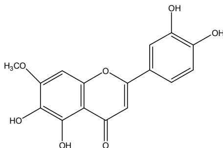
5, 6, 3', 4'-tétrahydroxy-7-méthoxyflavone
