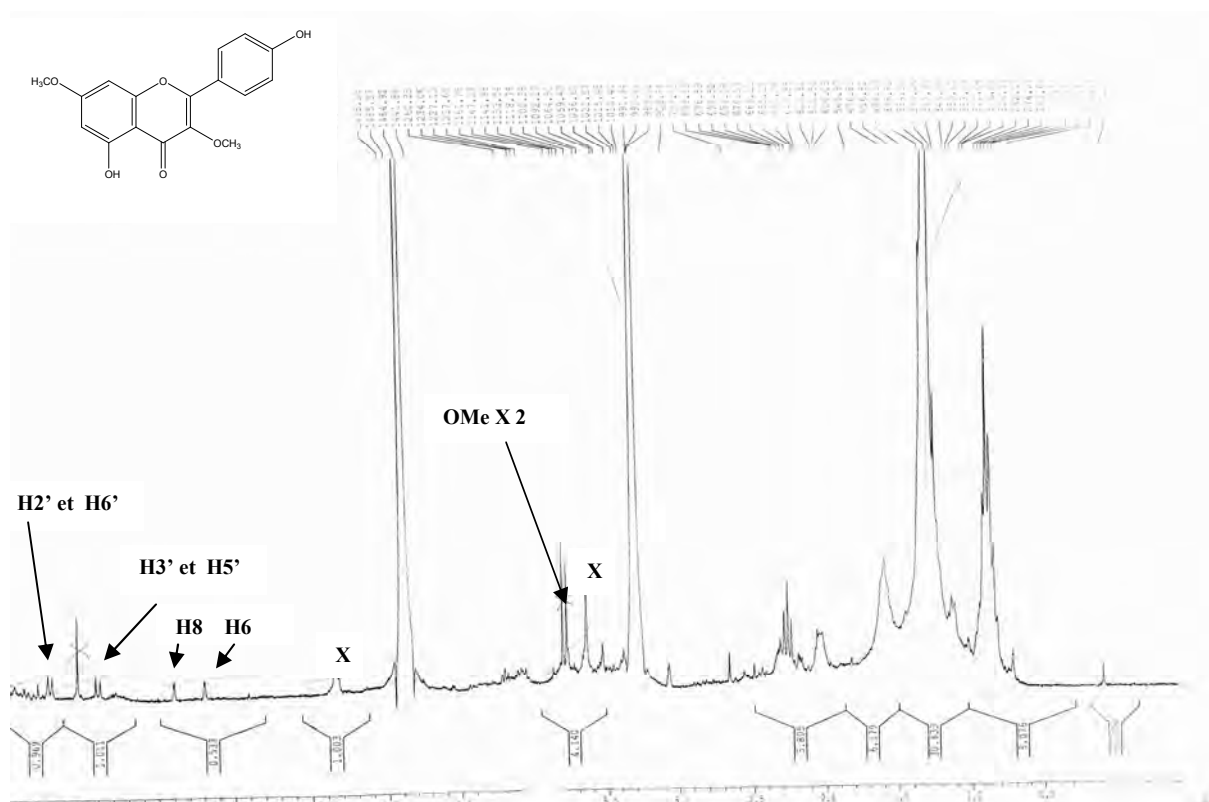
Figure-39: Spectre RMN- H^1 (300MHz, CD_3OD , \delta ppm) du produit F_{e-1} .
