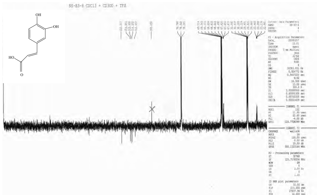
Figure-87 : spectre carbone J-modulé (125MHz, CD 3 OD, δ ppm) du composé B 3-8 .
