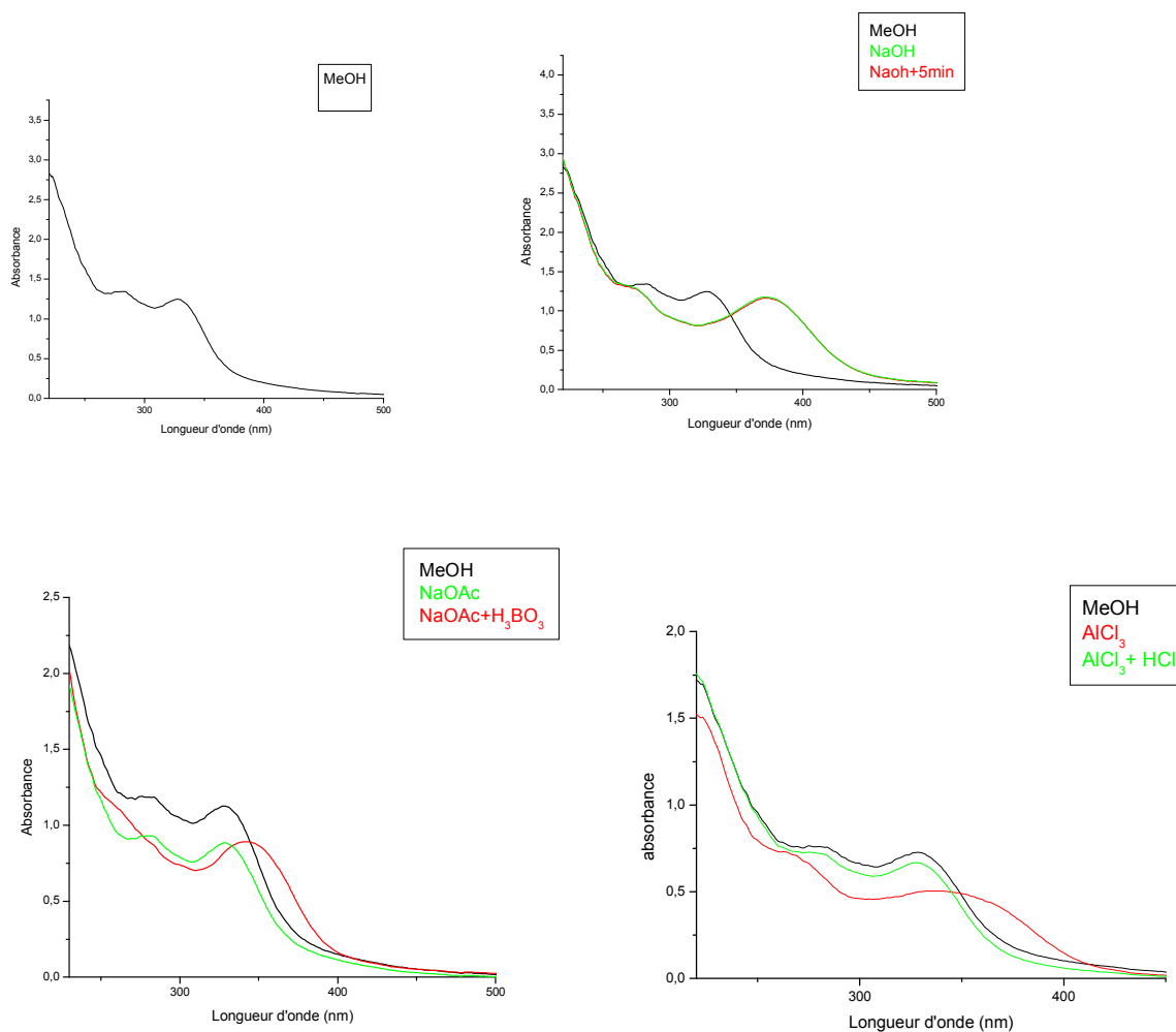
Figure-41: Spectre d'absorption UV-visible du produit SC1-F6-9.
