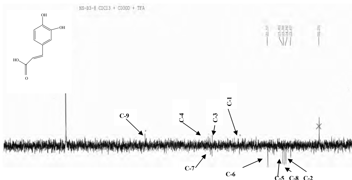
Figure-88: Etalement du spectre carbone J-modulé du composé B 3.8 .
