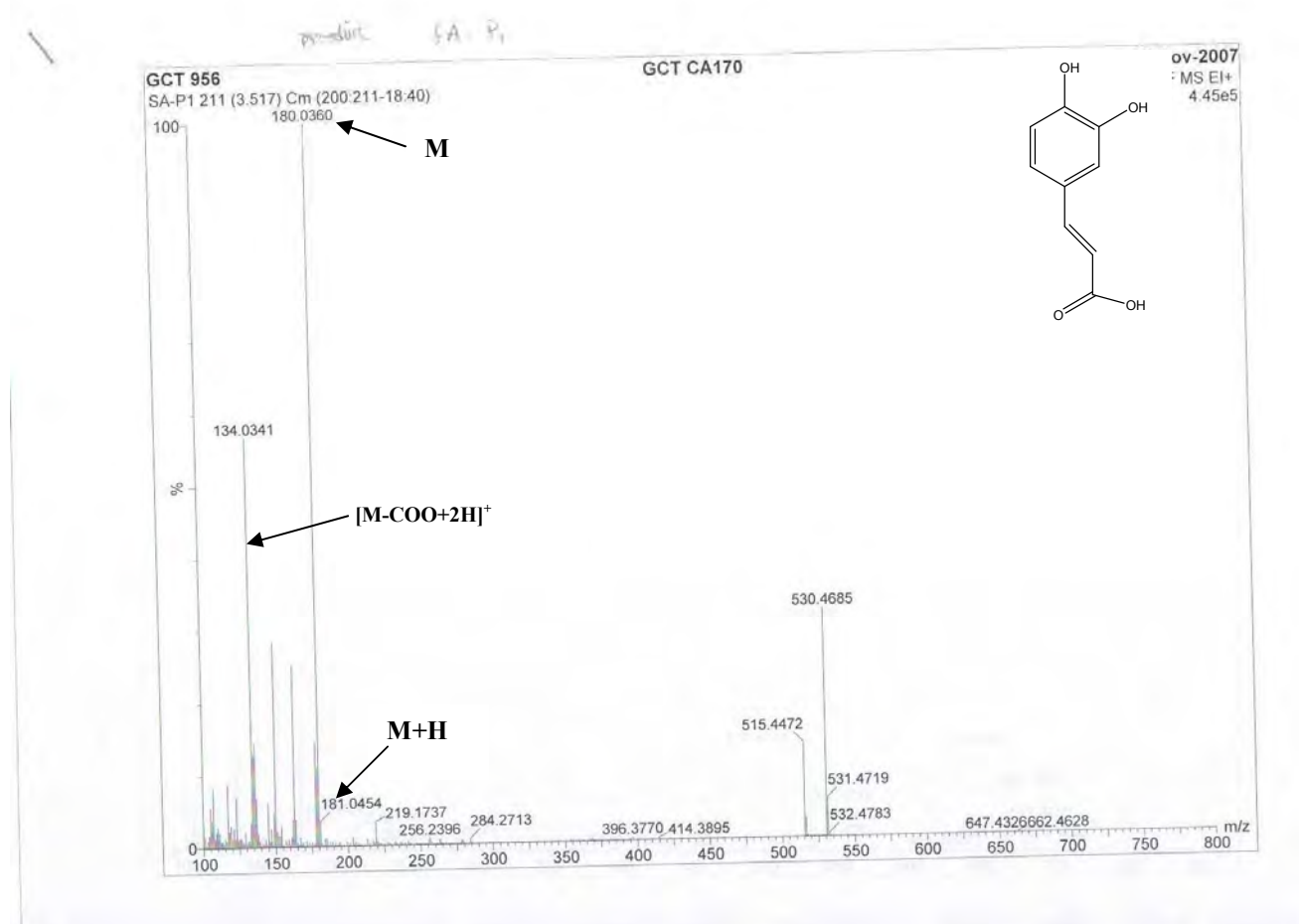
Figure-33 : Spectre EI-MS du produit Fa p1 .
