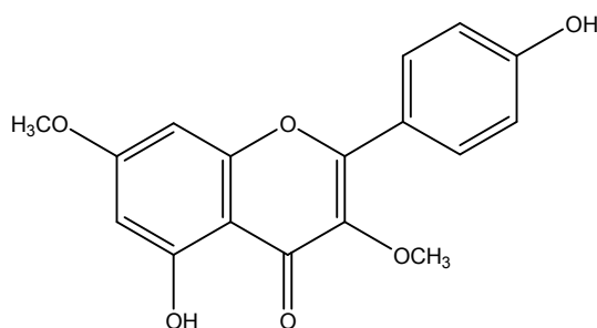
5,4'-dihydroxy-3, 7-diméthoxyflavone (Kumatakenin).
