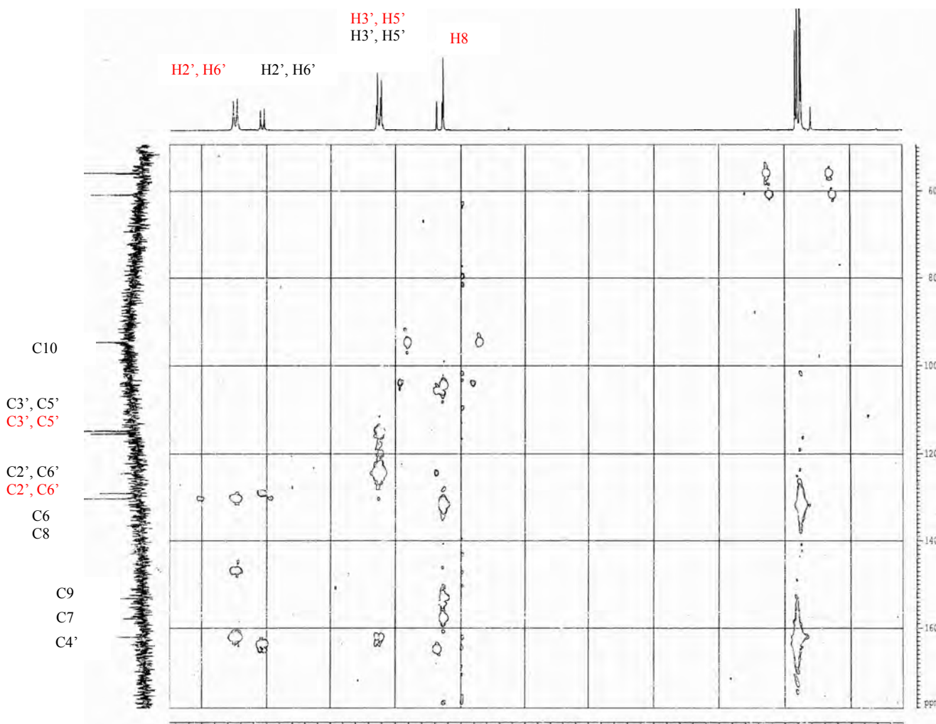
Figure-49 : Spectre HMBC (250MHz, DMSO-d6) du composé F 13 .
