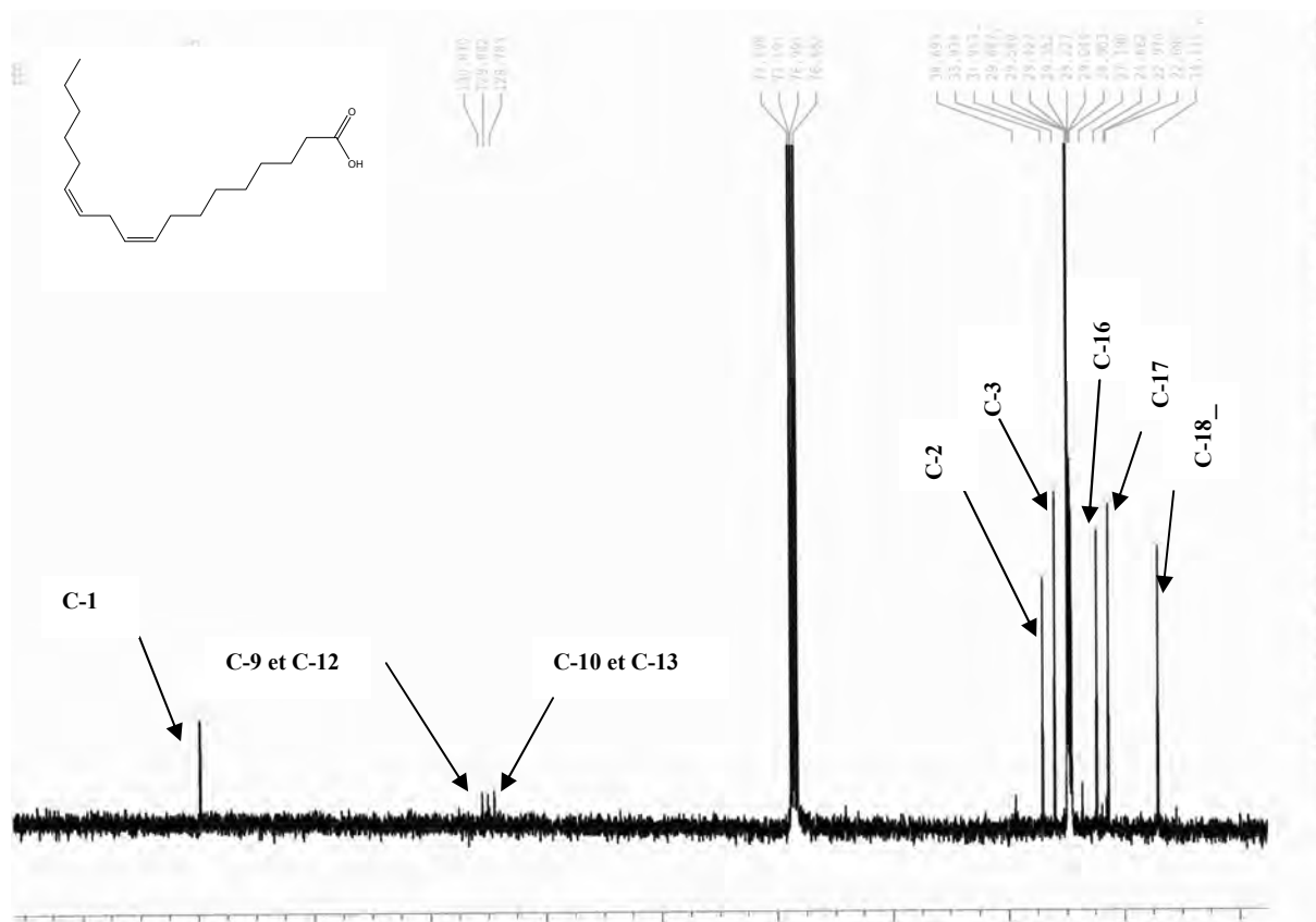
Figure-69 : Spectre RMN- C^{13} (63MHz, CDCl_3 , \delta ppm) du composé C-f55-57.
