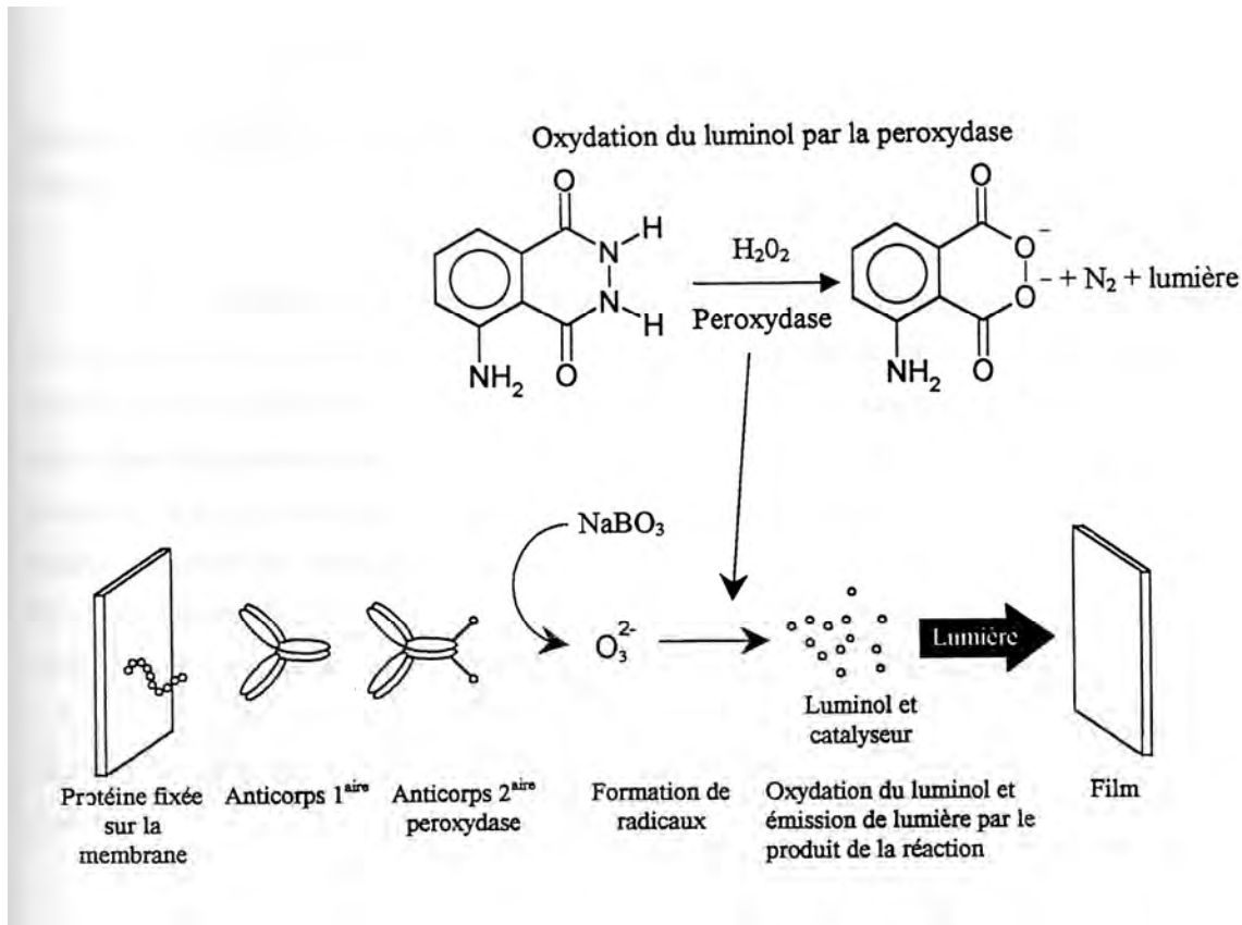
Figure-18: Schéma général de la révélation des protéines par chimiluminescence (Brassart 2000).
