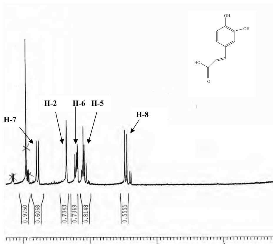
Figure-82 : Etaiement du spectre RMN-H 1 du produit B 3-8 .
