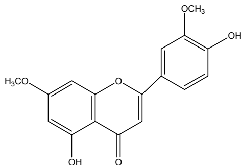
5,4'-dihydroxy-7,3'-diméthoxyflavone.
