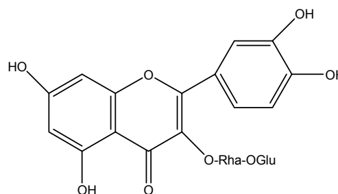
Rutine
