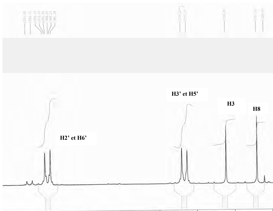
Figure-54 : Etalement du spectre RMN- \text{H}^1 du produit \text{F}_{14} .
