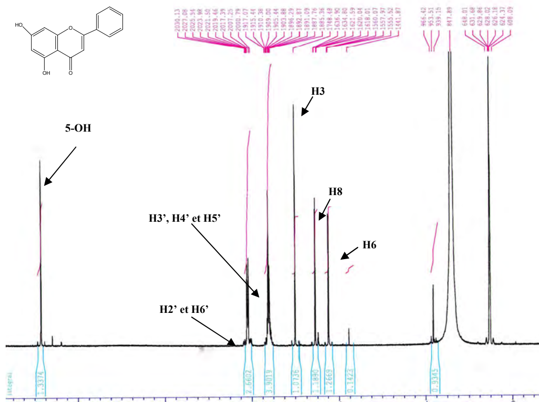
Figure-58 : Spectre RMN- \text{H}^1 (250MHz, \text{DMSO-d}_6 , \delta ppm) du produit \text{F}_{15} .
