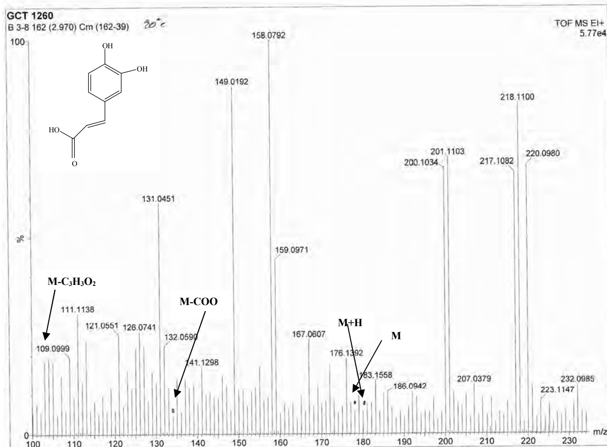
Figure-89 : Spectre EI-MS du produit B 3.8 .
