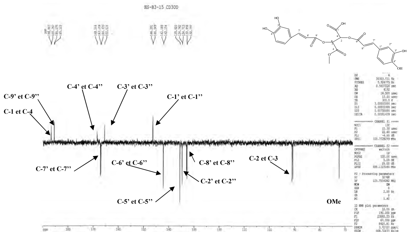
Figure-113 : Spectre J-modulé (125MHz, CD 3 OD+CF 3 COOD, δ ppm) du produit B 3-15 .
