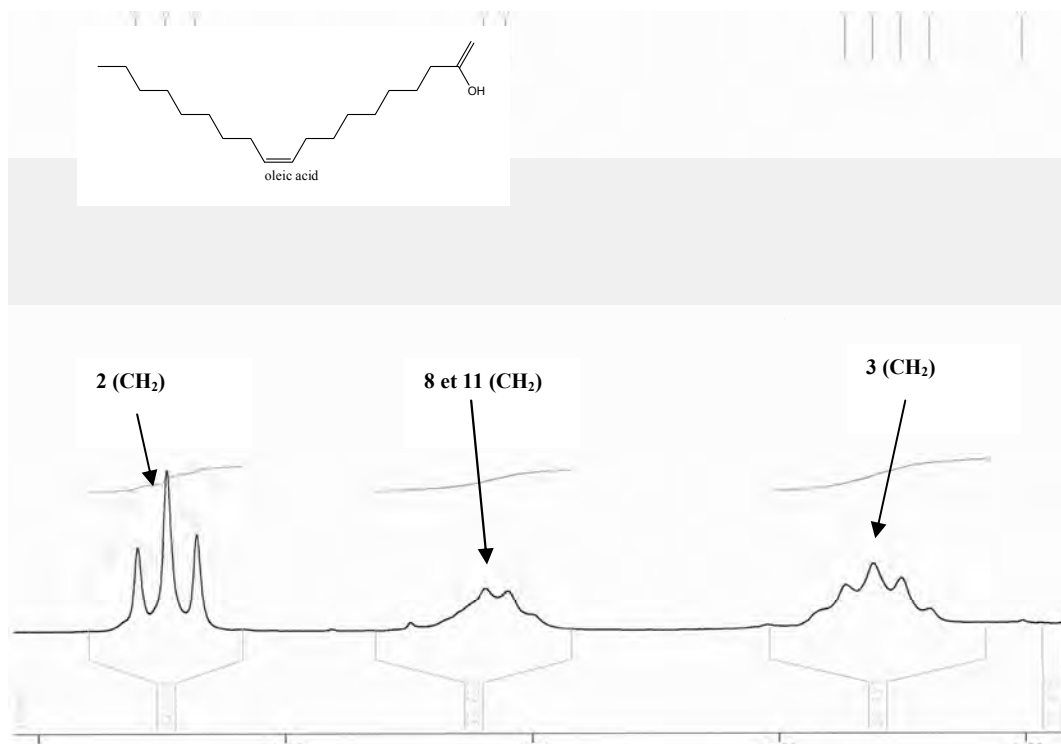
Figure-64: Etalement du spectre RMN-H 1 du produit F 19-24 .
