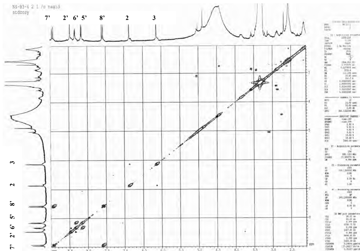
Figure-77 : Spectre COSY (500MHz, CD 3 OD) du composé B 3-4 .
