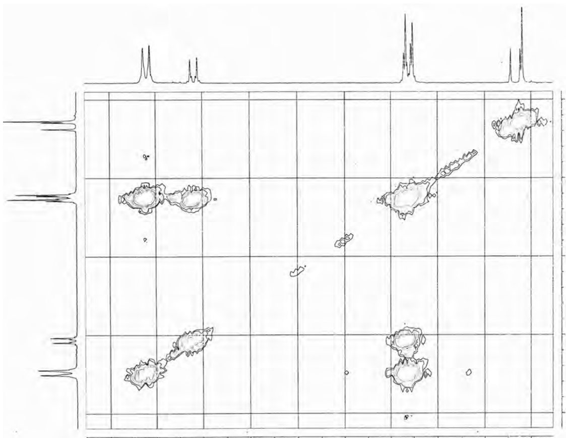
Figure-46 : Spectre COSY (250MHz, DMSO-d 6 ) du composé F 13 .
