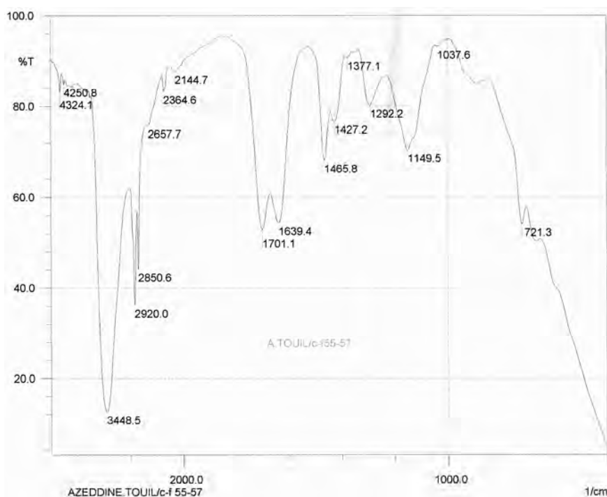
Figure-66 : Spectre infrarouge du composé C-f55-57
