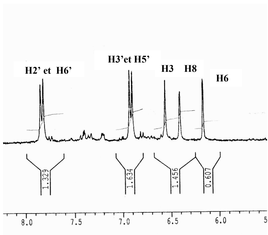
Figure-31 : Etallement du spectre RMN-H 1 du produit F 13-2
