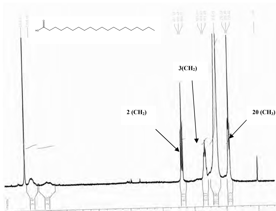
Figure-72 : Spectre RMN- H^1 (250MHz, CDCl_3 , \delta ppm) du composé C-f65.
