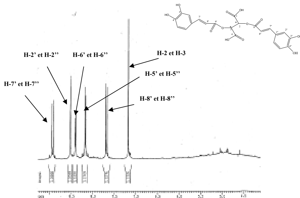
Figure-97 : Etallement du spectre RMN- H^1 du produit B 3-12 .
