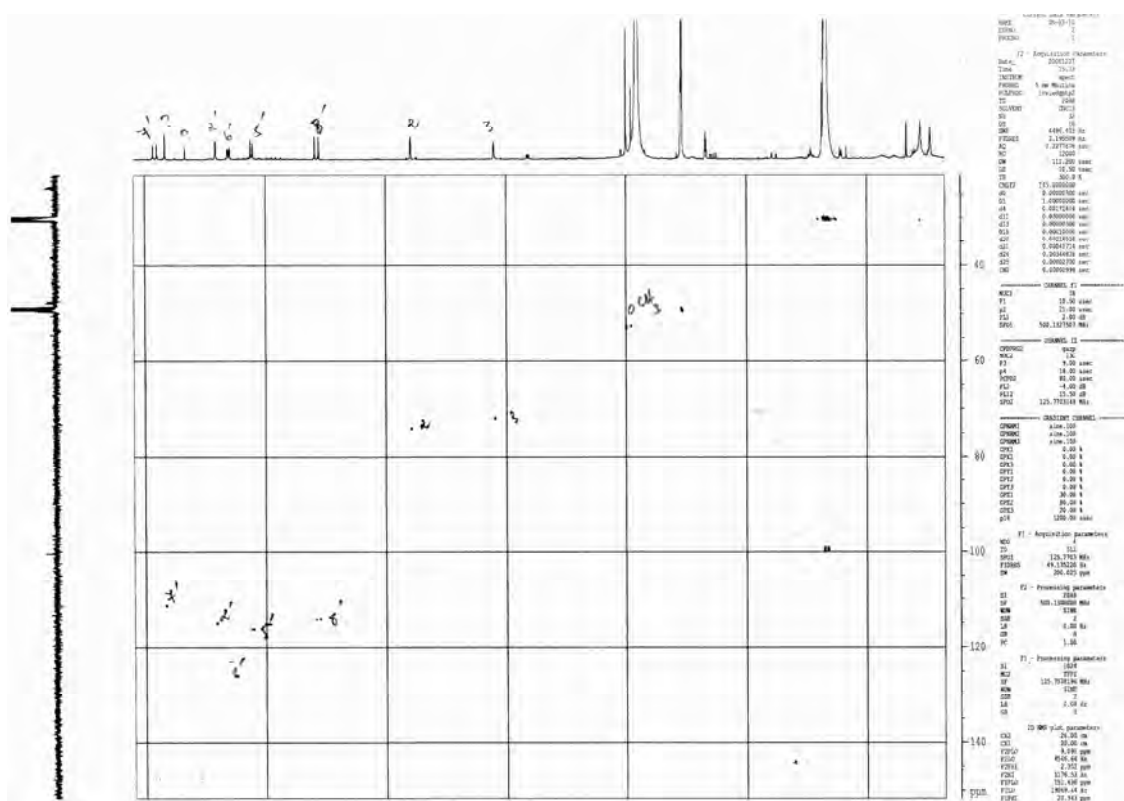
Figure-92 : Spectre HSQC (500MHz, CD 3 OD) du produit B 3 -10.
