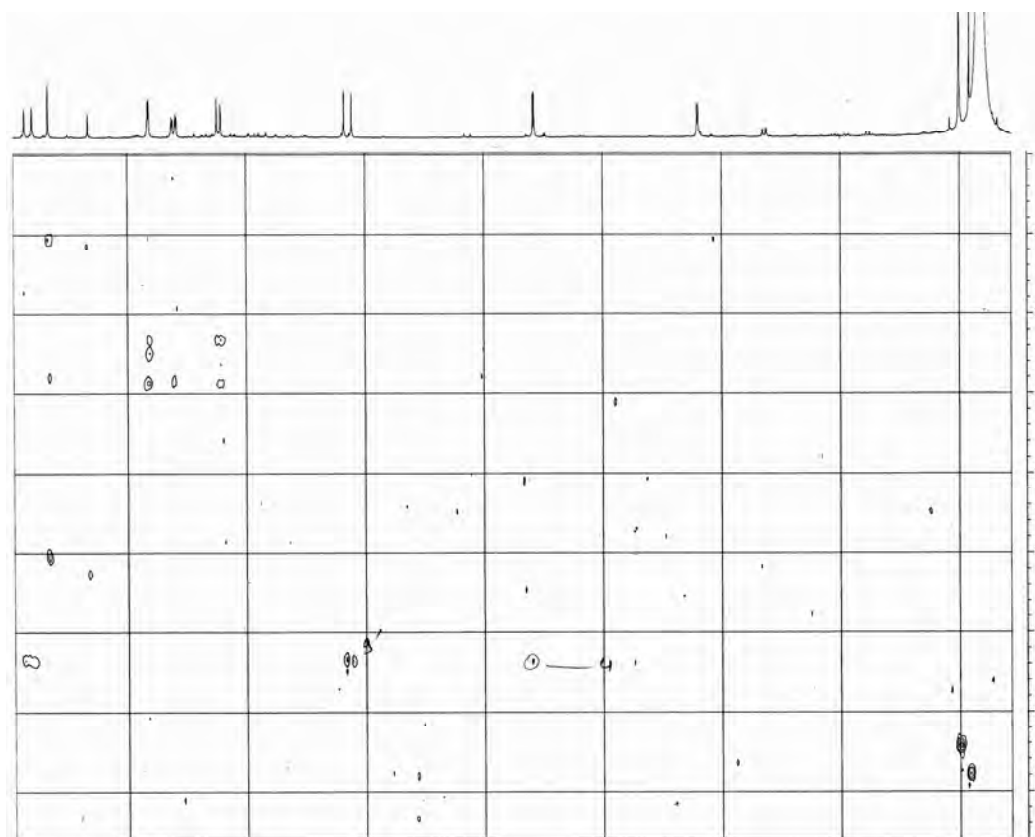
Figure-94 : spectre HMBC (500MHz, CD 3 OD) du produit B 3-10 .
