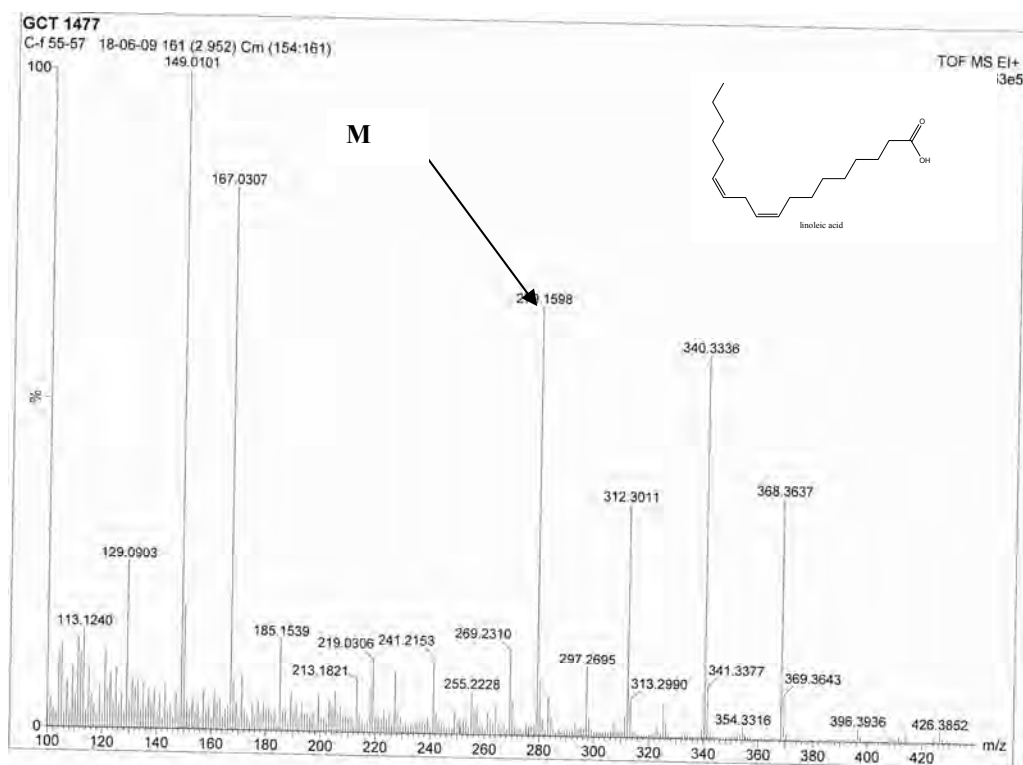
Figure-67 : Spectre de masse du composé C-f55-57
