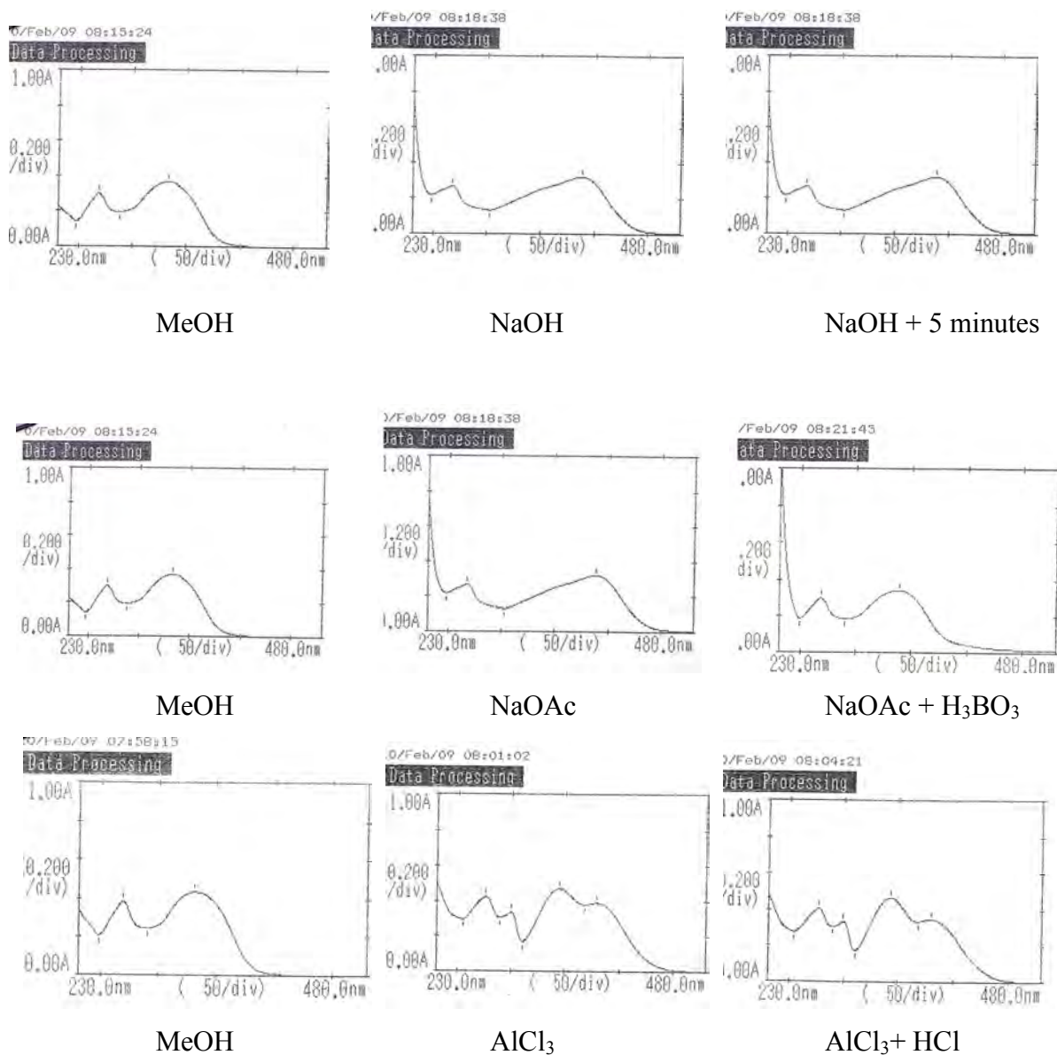
Figure-26 : Spectres d'absorption UV-visible du produit F 13-1 .
