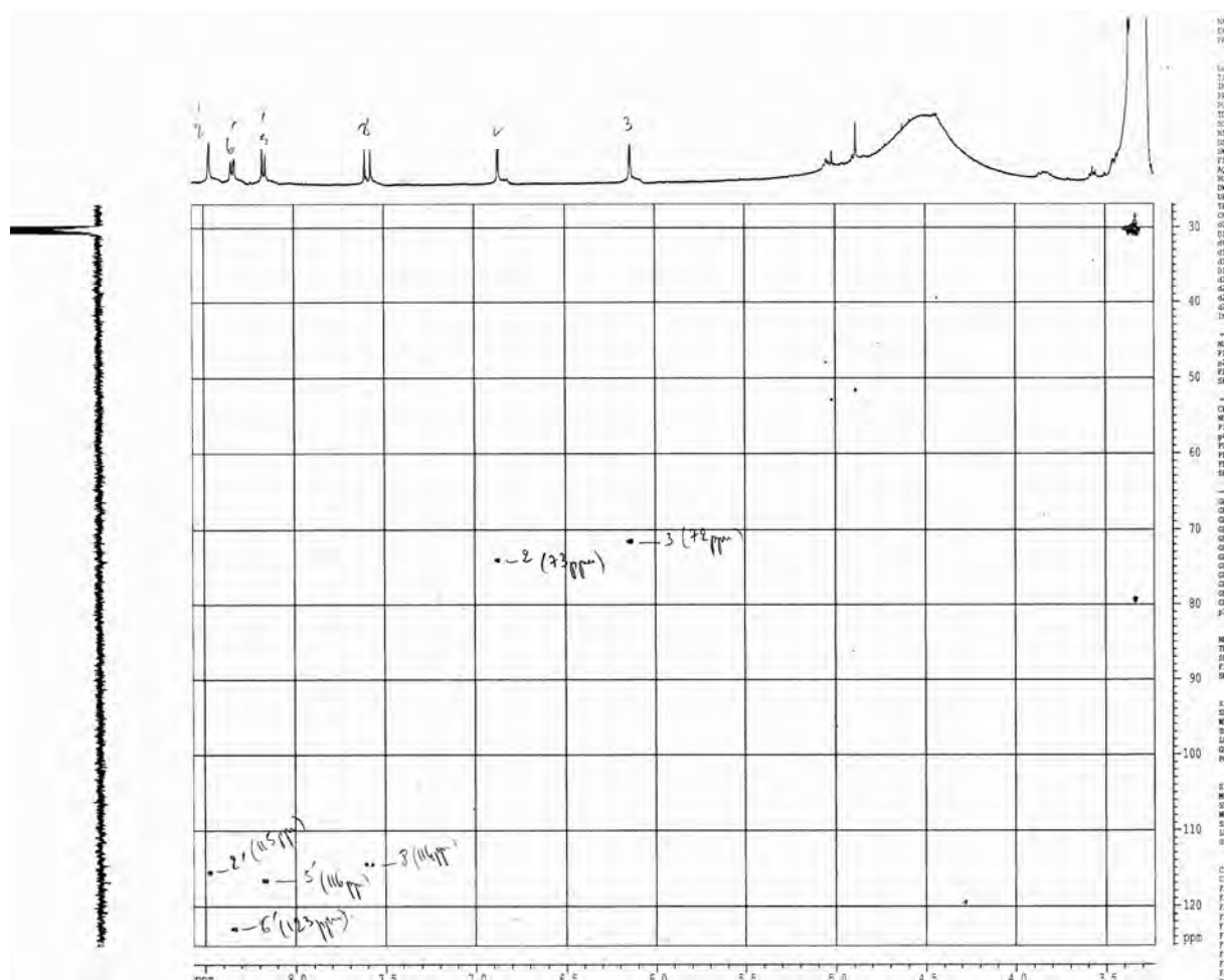
Figure-78 : Spectre HSQC (500MHz, CD 3 OD) du composé B 3-4 .
