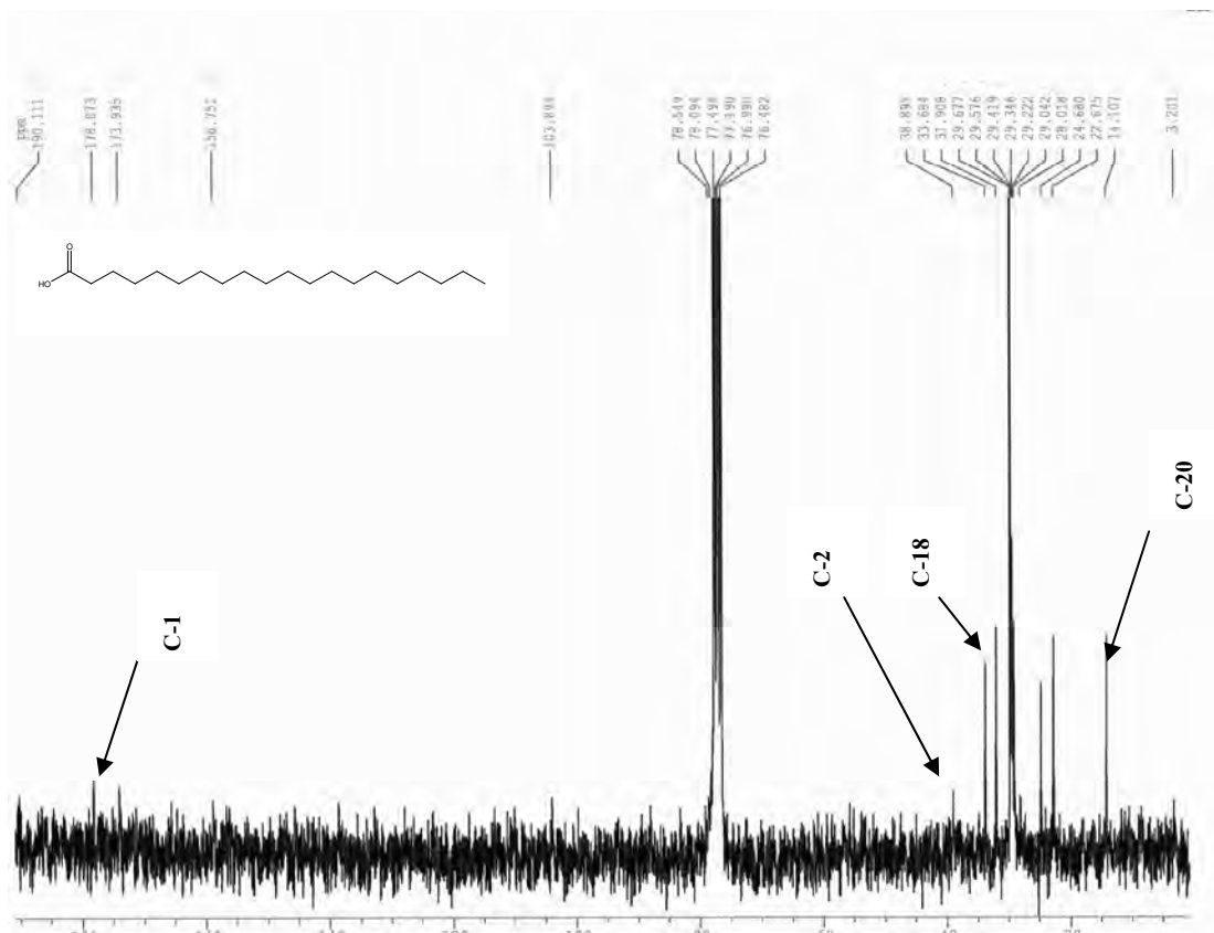
Figure-73 : Spectre RMN-C 13 (63MHz, CDCl 3 , δ ppm) du composé C-f65.
