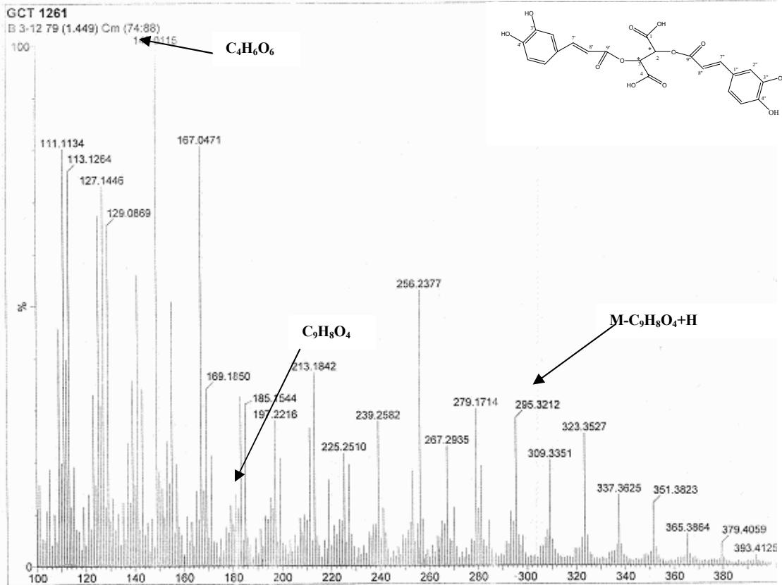
Figure-99 : Etallement du spectre EI-MS du produit B 3-12 .
