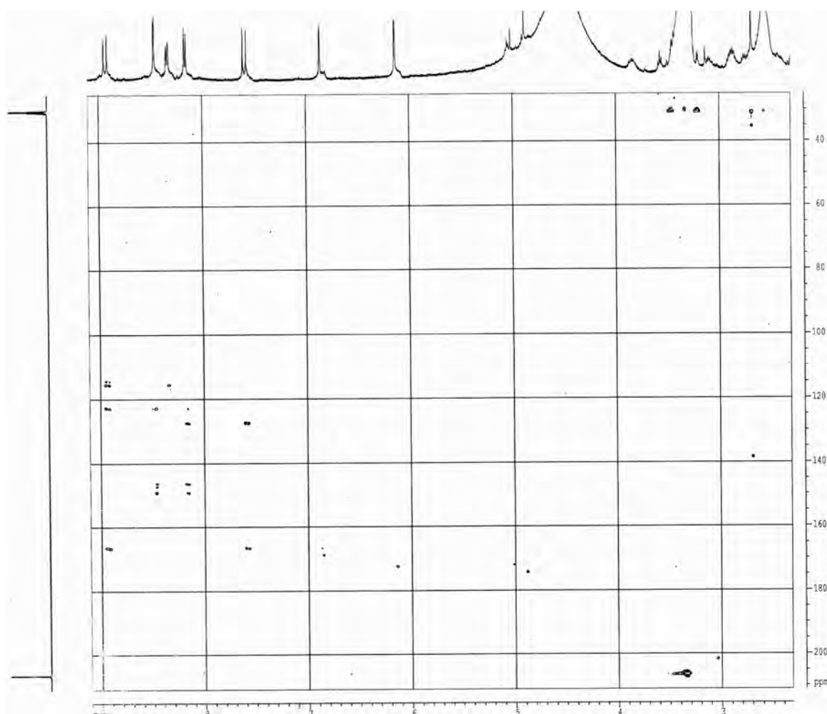
Figure-79 : Spectre HMBC (500MHz, CD 3 OD) du produit B 3-4 .
