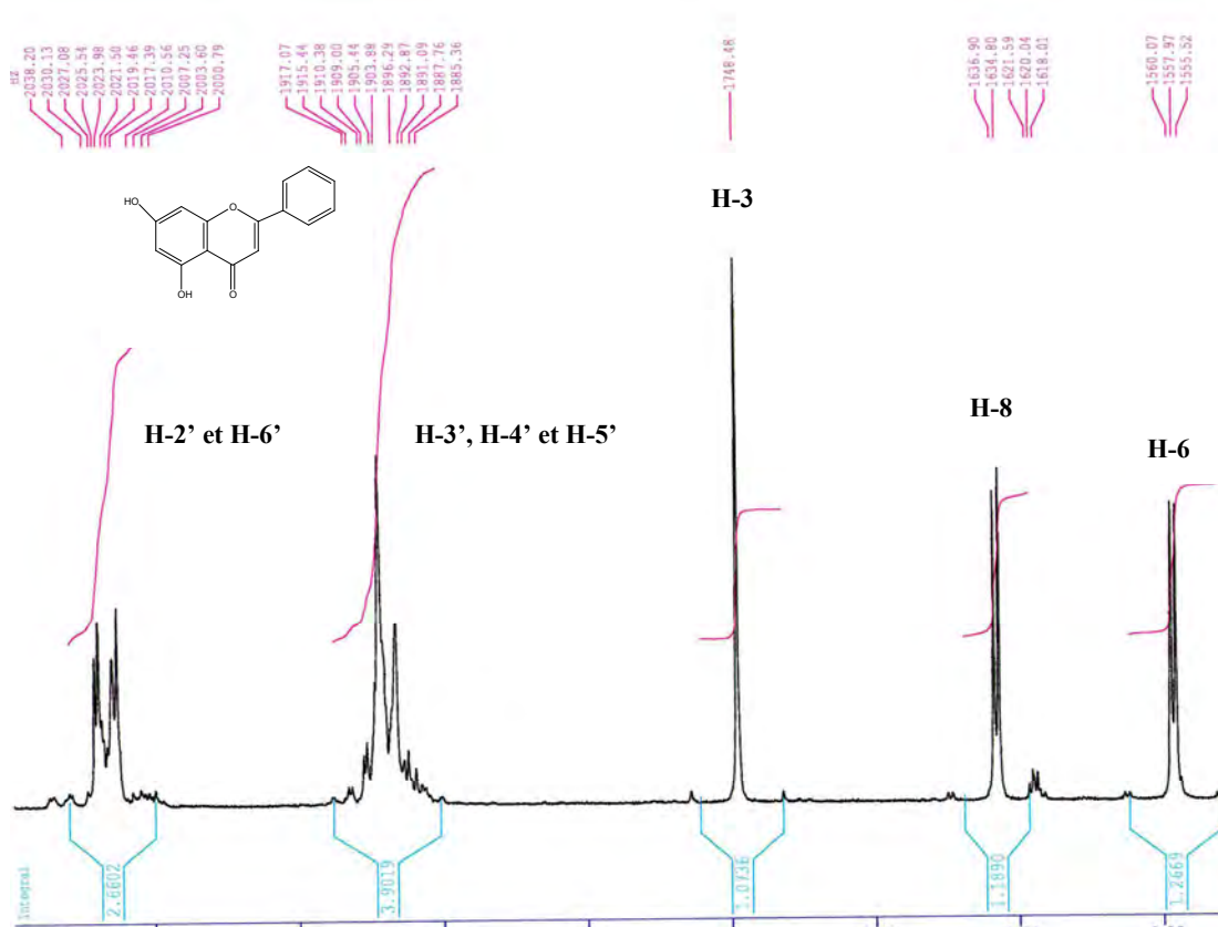
Figure-59 : Etalement du spectre RMN- \text{H}^1 du produit \text{F}_{15}
