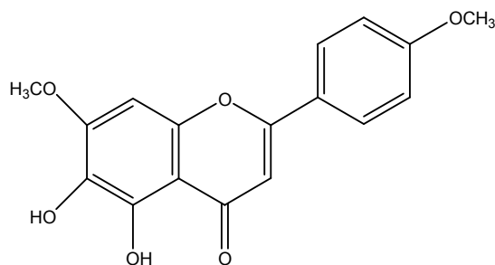
5,6-dihydroxy-7,4'-diméthoxyflavone (Ladaneine).
