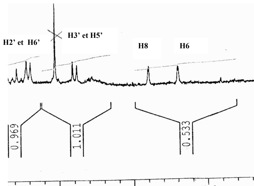
Figure-40: étalement du spectre RMN- H^1 du produit Fe-1.
