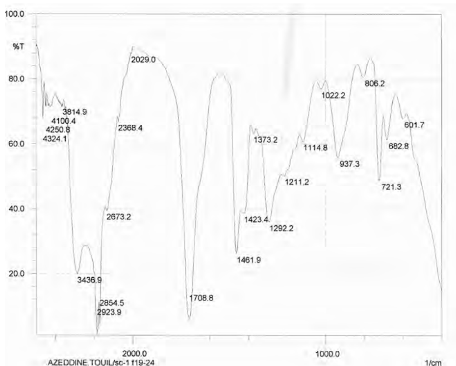
Figure-61 : Spectre infrarouge du produit F 19-24 .
