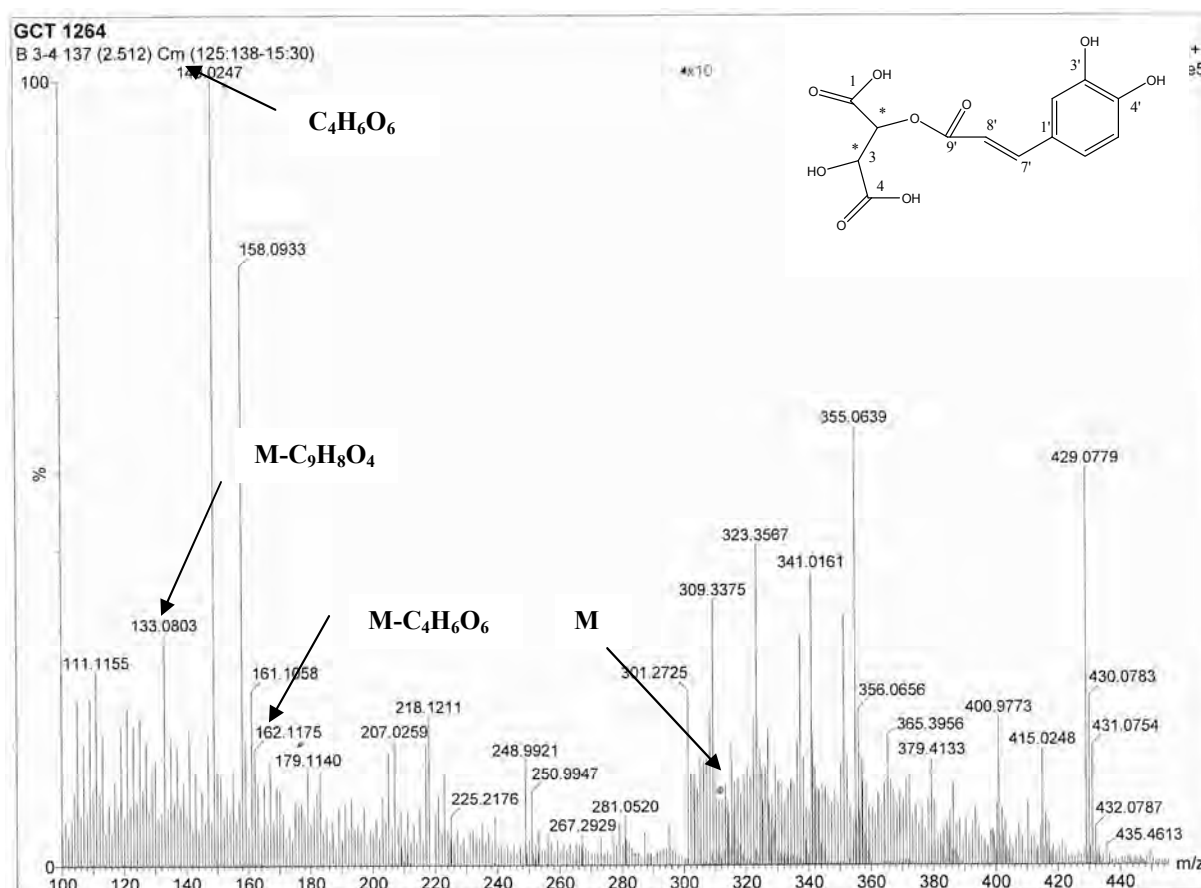
Figure-76 : Spectre EI-MS du produit B 3-4 .
