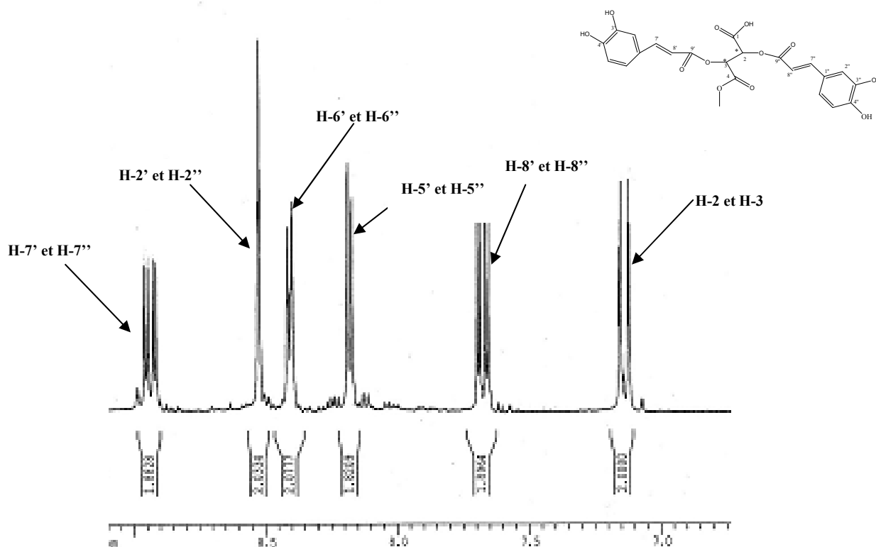
Figure-106 : Etallement du spectre RMN- H^1 (500MHz, CD_3OD + CF_3COOD , \delta ppm) du produit B_{3-15} .
