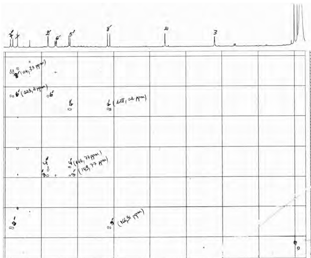
Figure-95 : Etalement du spectre HMB du produit B 3-10 .
