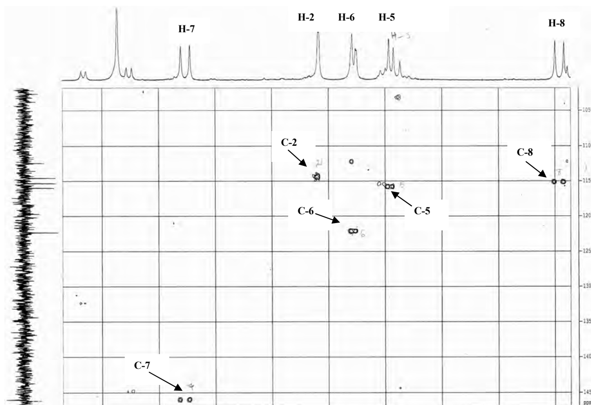
Figure-84 : Etagement du spectre HSQC du produit B 3-8 .
