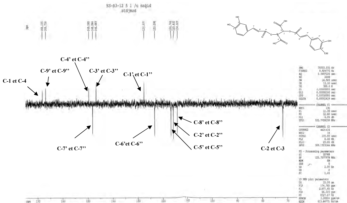
Figure-104 : Spectre J-modulé (125MHz, CD 3 OD+CF 3 COOD, δ ppm) du produit B 3-12 .
