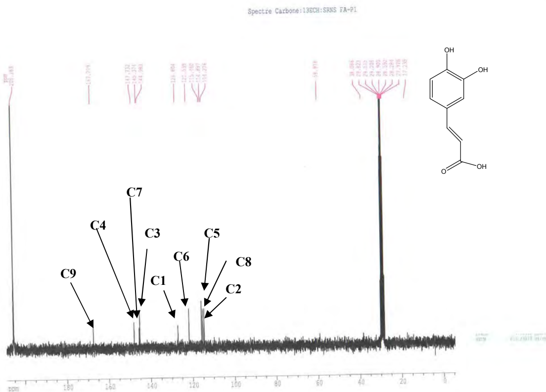
Figure-36 : Spectre RMN-C 13 (63MHz, DMSO-d 6 , δ ppm) du produit F a-p1 .
