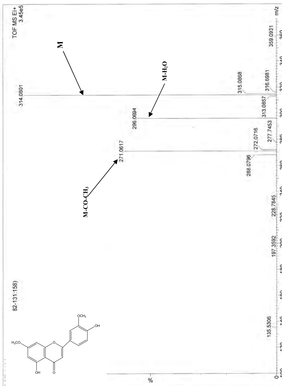
Figure-27 : Spectre de masse du produit F 13-1
