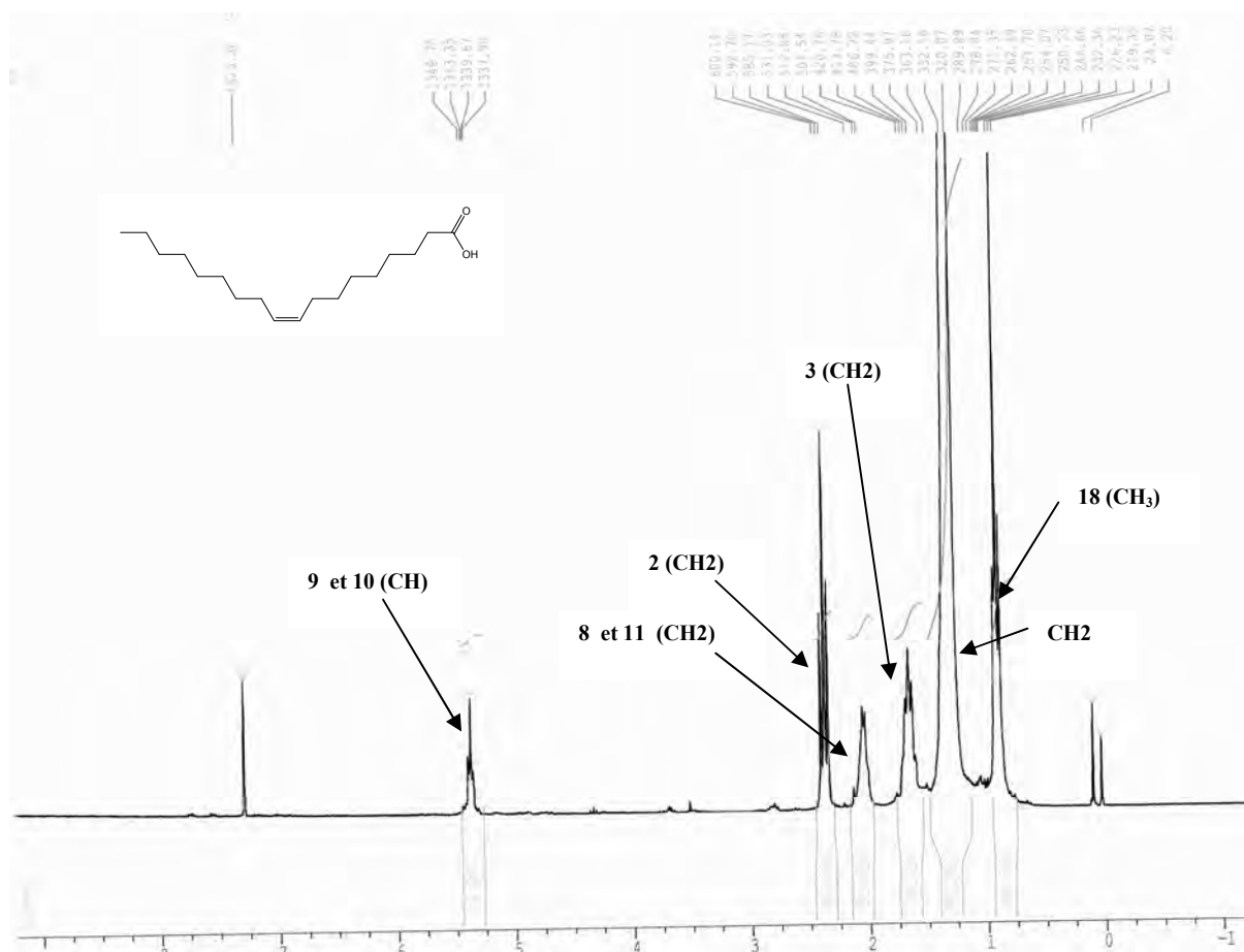
Figure-62 : Spectre RMN- H^1 (250MHz, CDCl_3 , \delta ppm) du produit F_{19-24}
