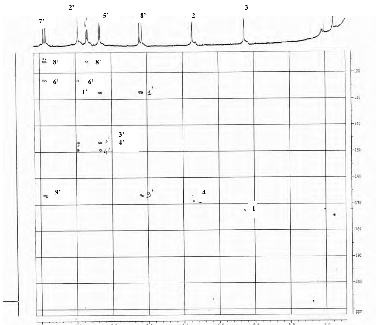
Figure-80 : Etallement du spectre HMBC du produit B 3-4 .
