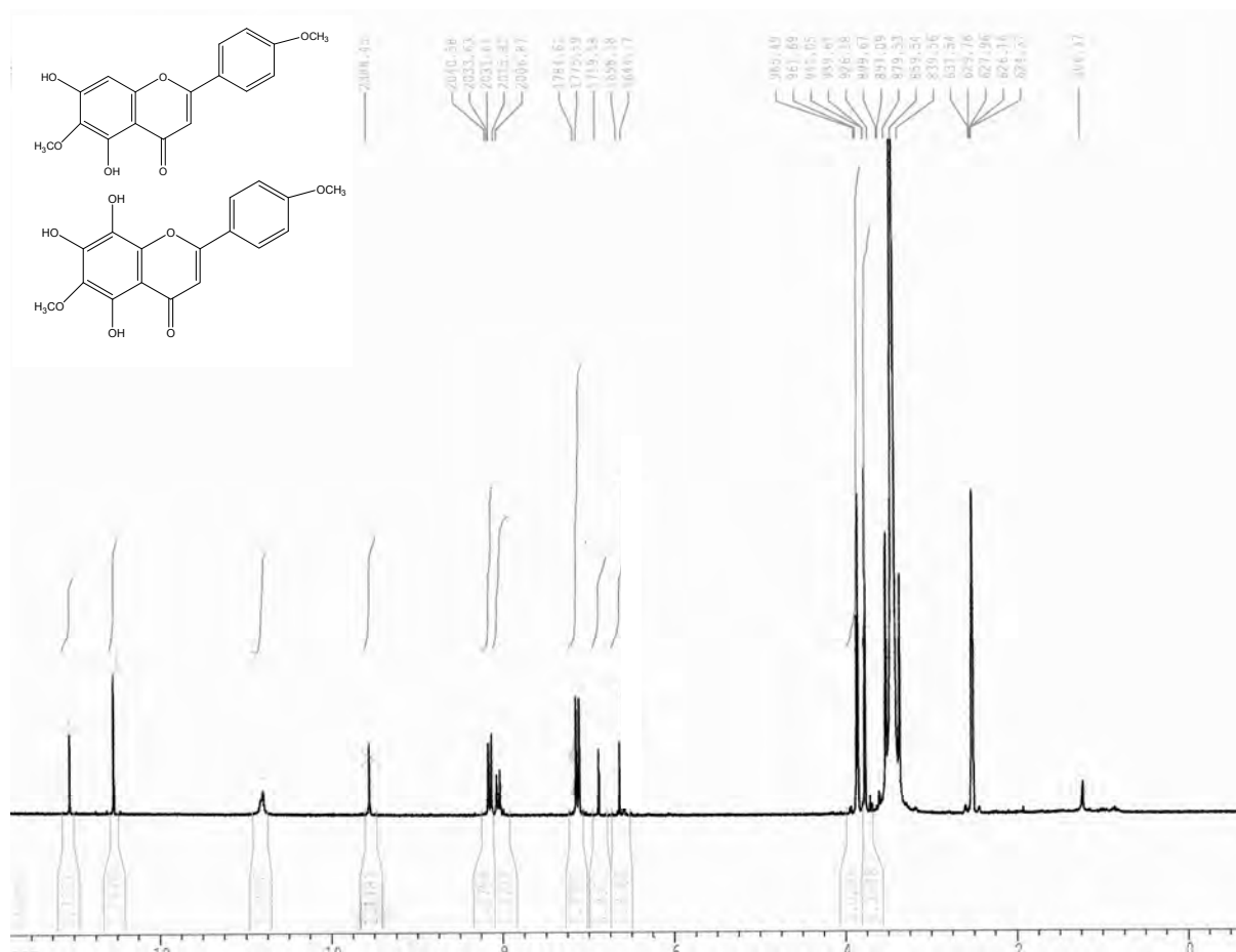
Figure-44 : Spectre RMN-H 1 (250MHz, DMSO-d 6 , δ ppm) du composé F 13
