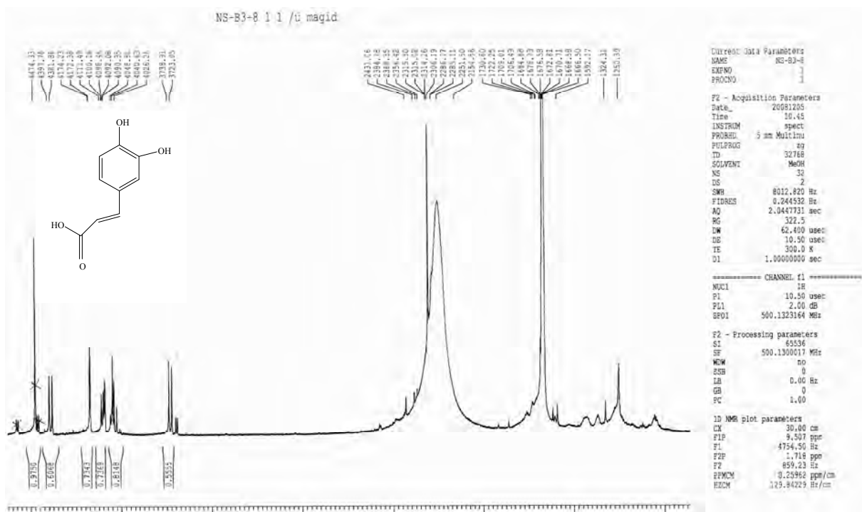
Figure-81 : Spectre RMN-H 1 (500MHz, CD 3 OD, δ ppm) du produit B 3-8 .
