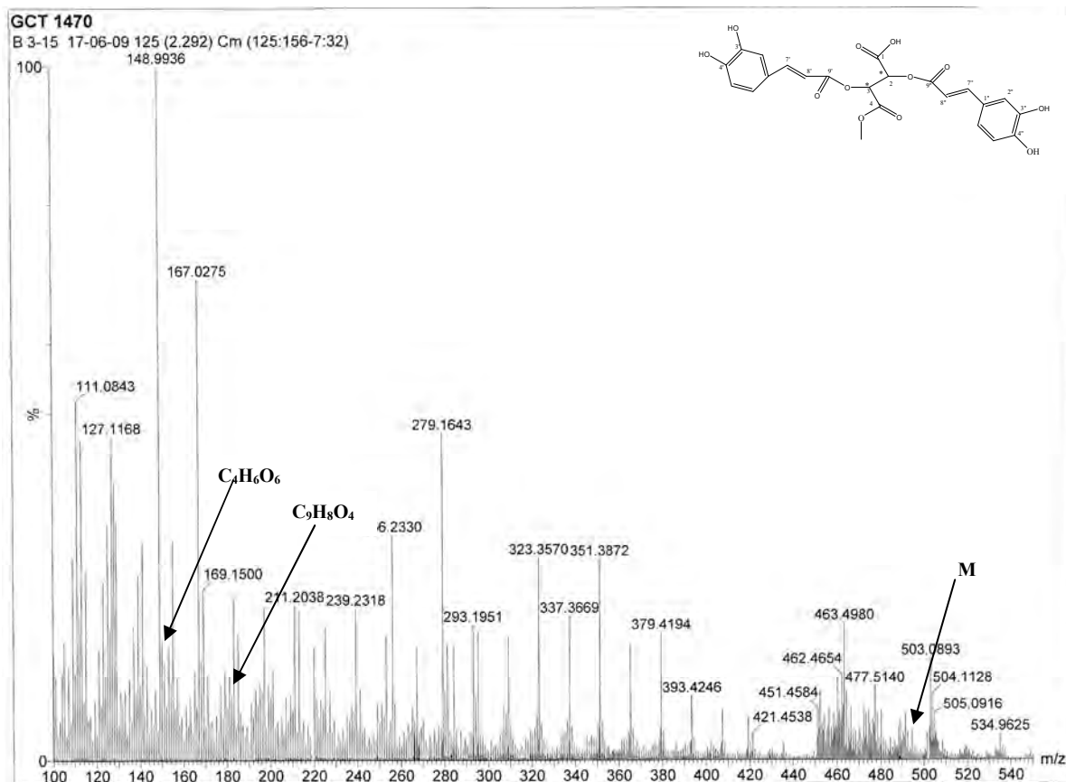
Figure-107 : Spectre EI-MS du produit B 3-15 .
