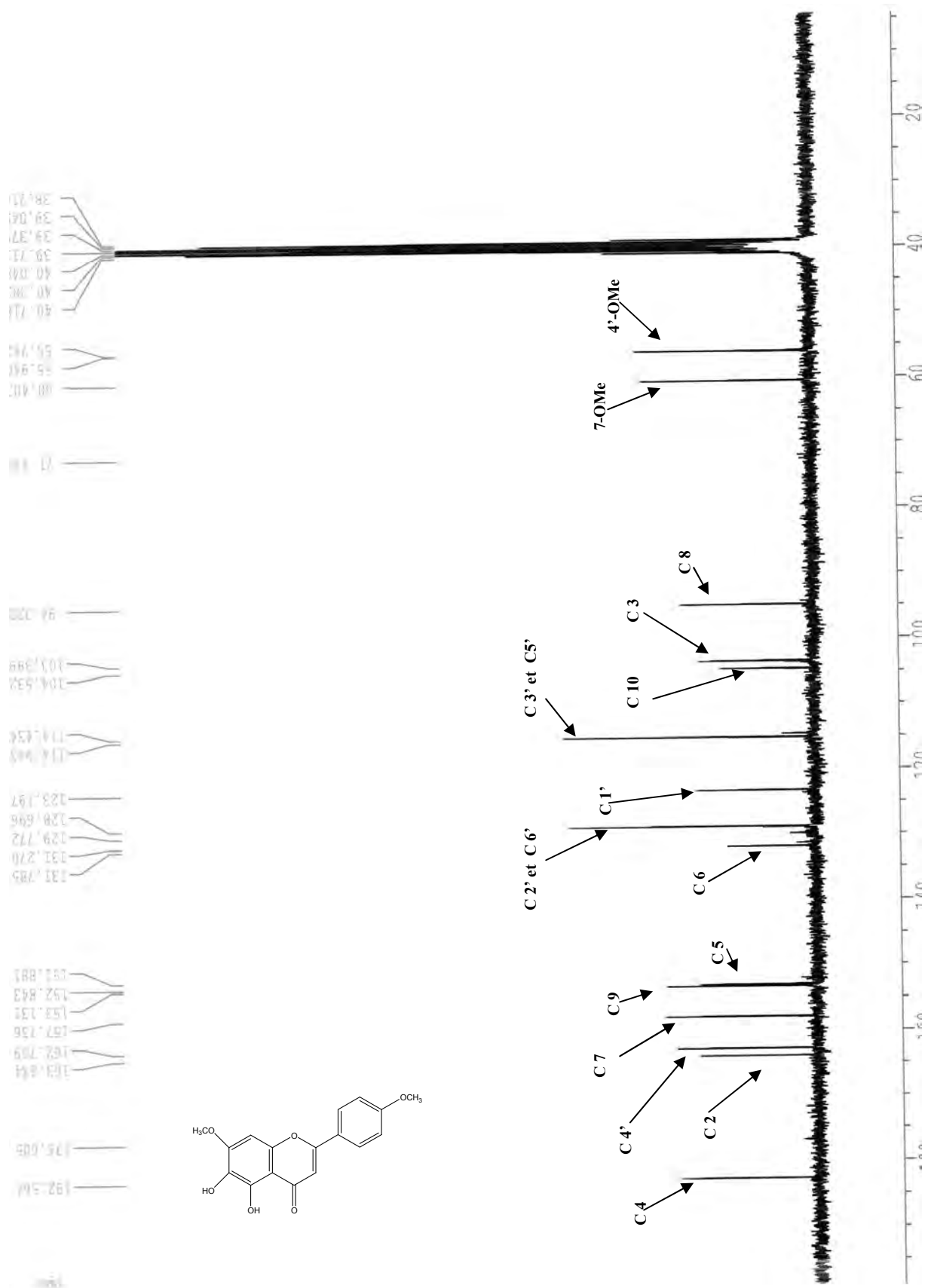
Figure-55 : Spectre RMN-C 13 (63MHz, DMSO-d 6 , δ ppm) du produit F 14
