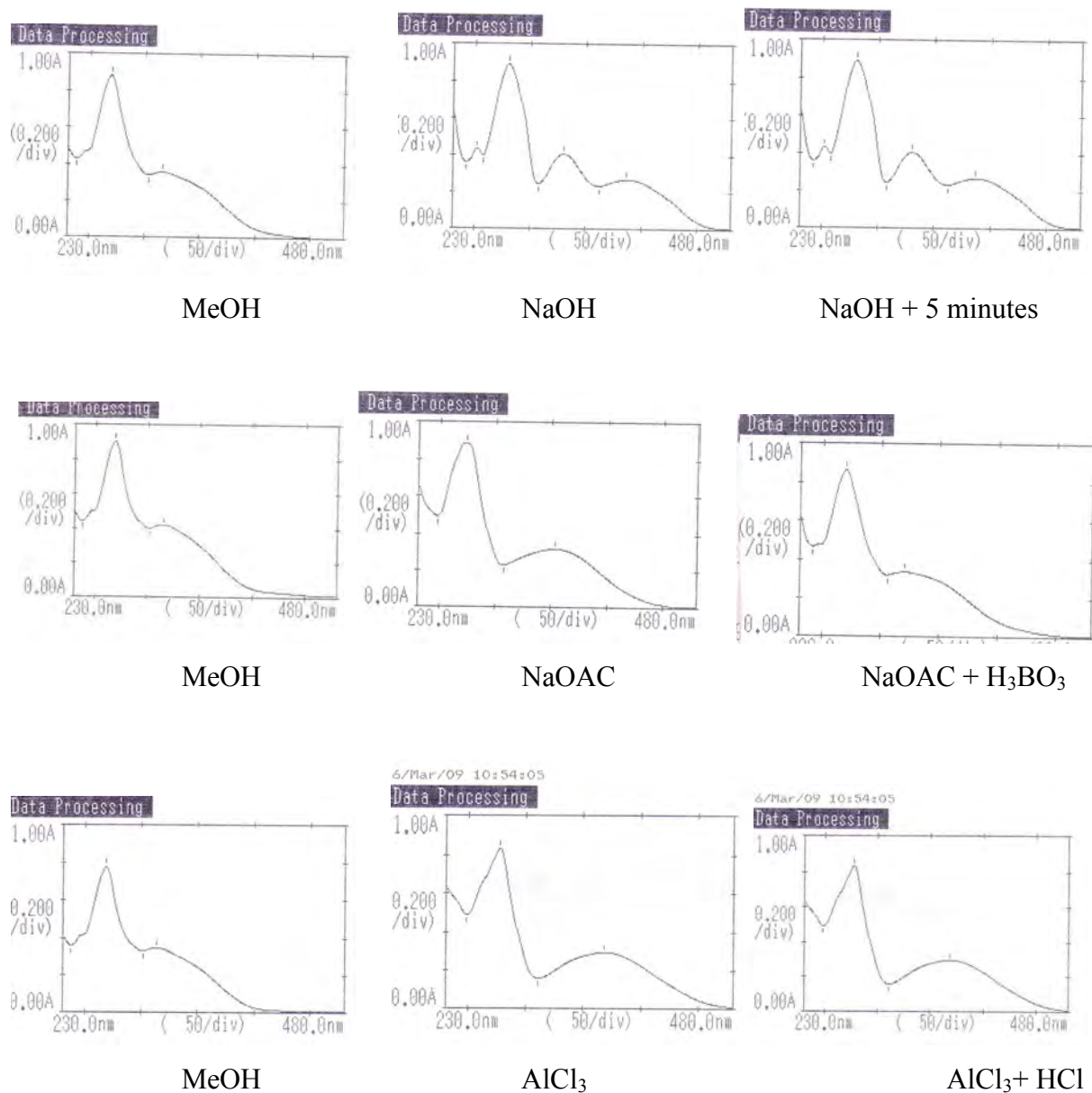
Figure-56 : Spectres d'absorption UV-visible du produit F 15 .
