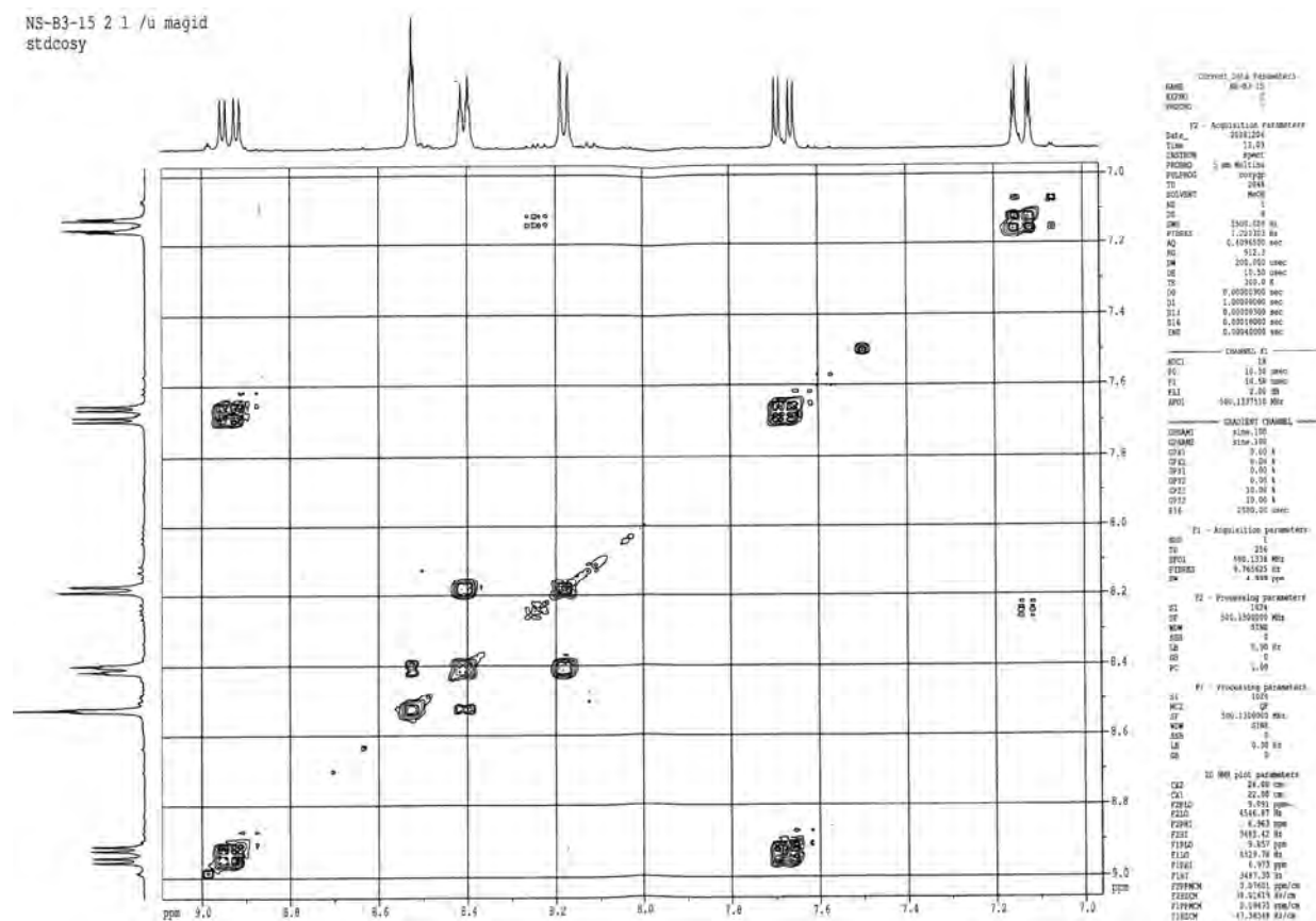
Figure-108 : Spectre COSY (500MHz, CD 3 OD+ CF 3 COOD) du produit B 3-15 .
