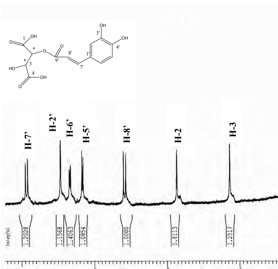
Figure-75 : Etallement du spectre RMN- H^1 du produit B_{3-4} .
