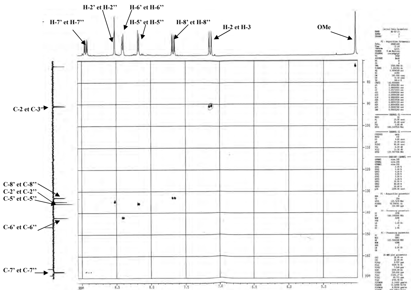
Figure-109 : Spectre HSQC (500MHz, CD 3 OD+ CF 3 COOD) du produit B 3-15 .
