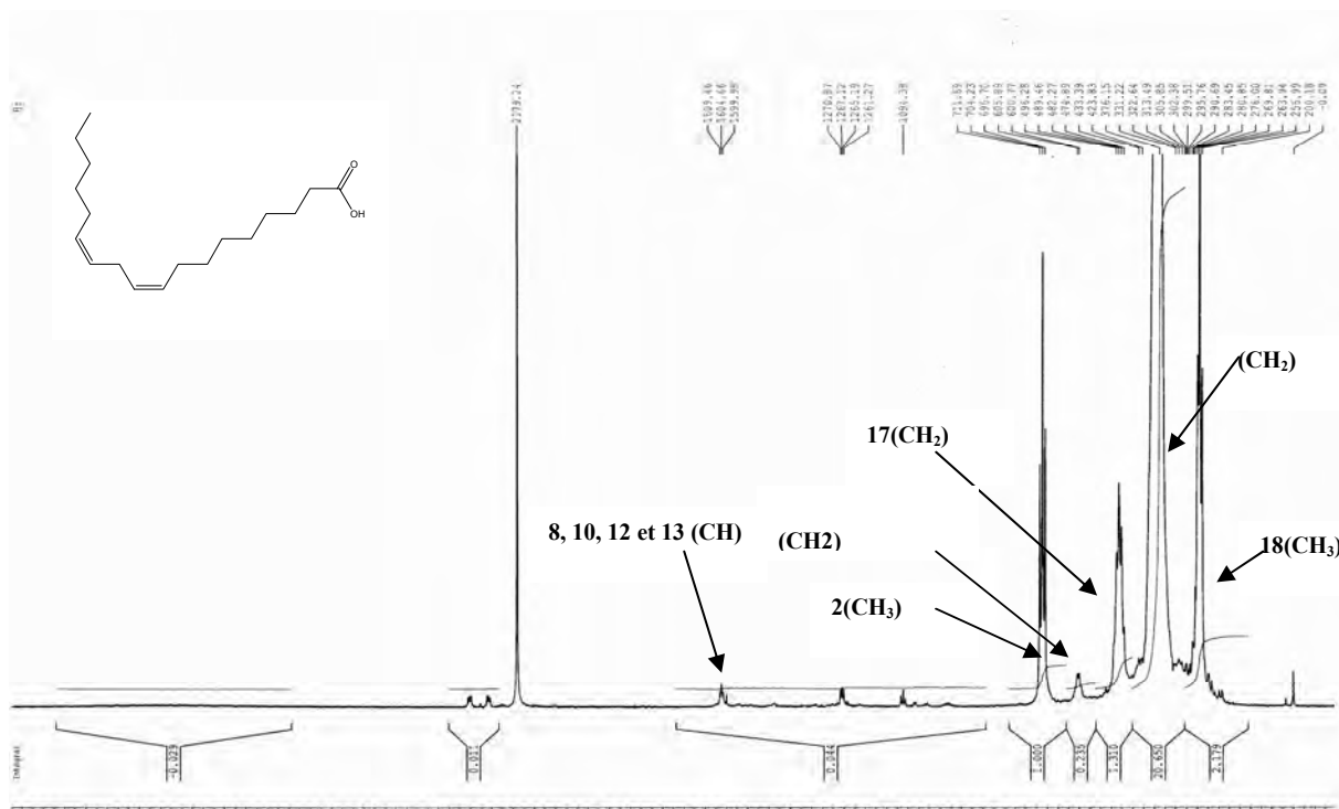
Figure-68 : Spectre RMN- H^1 (250MHz, CDCl_3 , \delta ppm) du composé C-f55-57.
