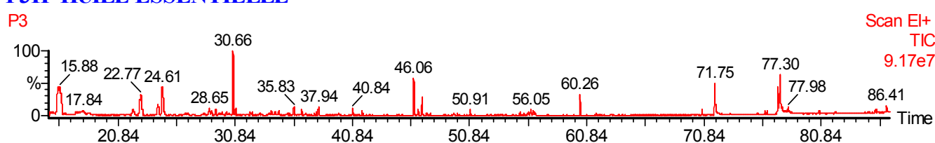
C- Chromatogramme de l'huile essentielle de P 3 (Kaous)
