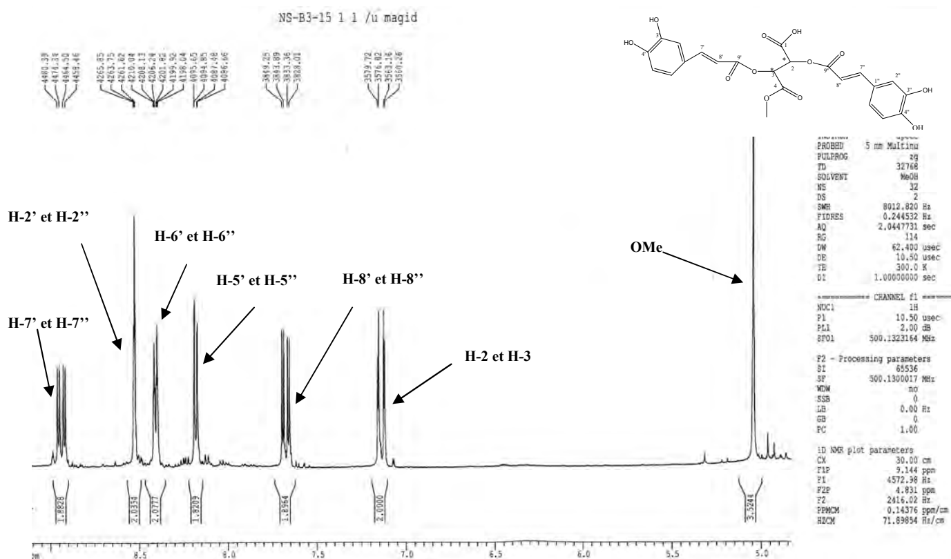
Figure-105 : Spectre RMN-H 1 (500MHz, CD 3 OD + CF 3 COOD, δ ppm) du produit B 3-15 .
