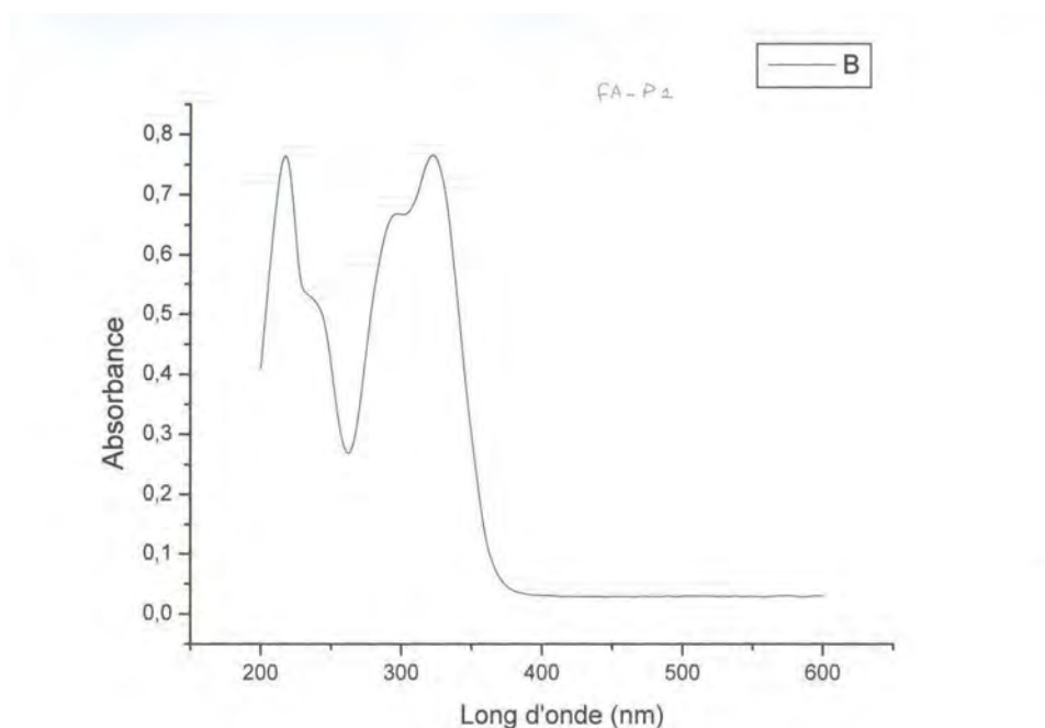
Figure-32 : Spectre d'absorption UV-visible du produit F_{a-p1} .
