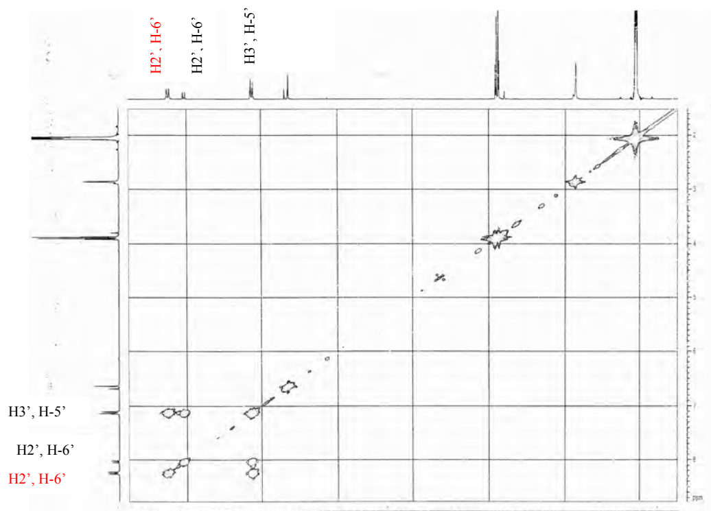
Figure-46 : Spectre COSY (250MHz, DMSO-d 6 ) du composé F 13 .
