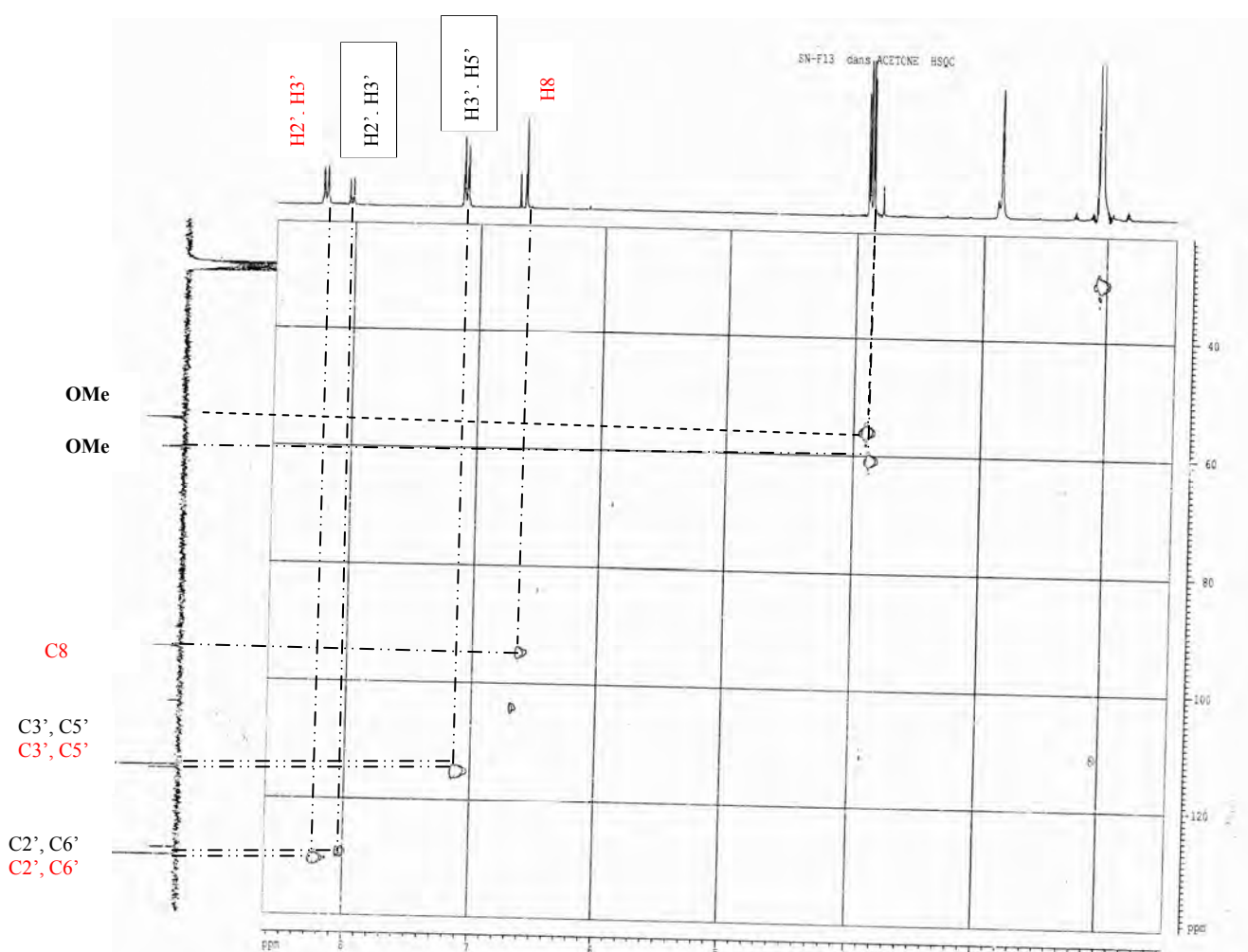
Figure-48 : Spectre HSQC (250MHz, DMSO-d6) du composé F 13 .
