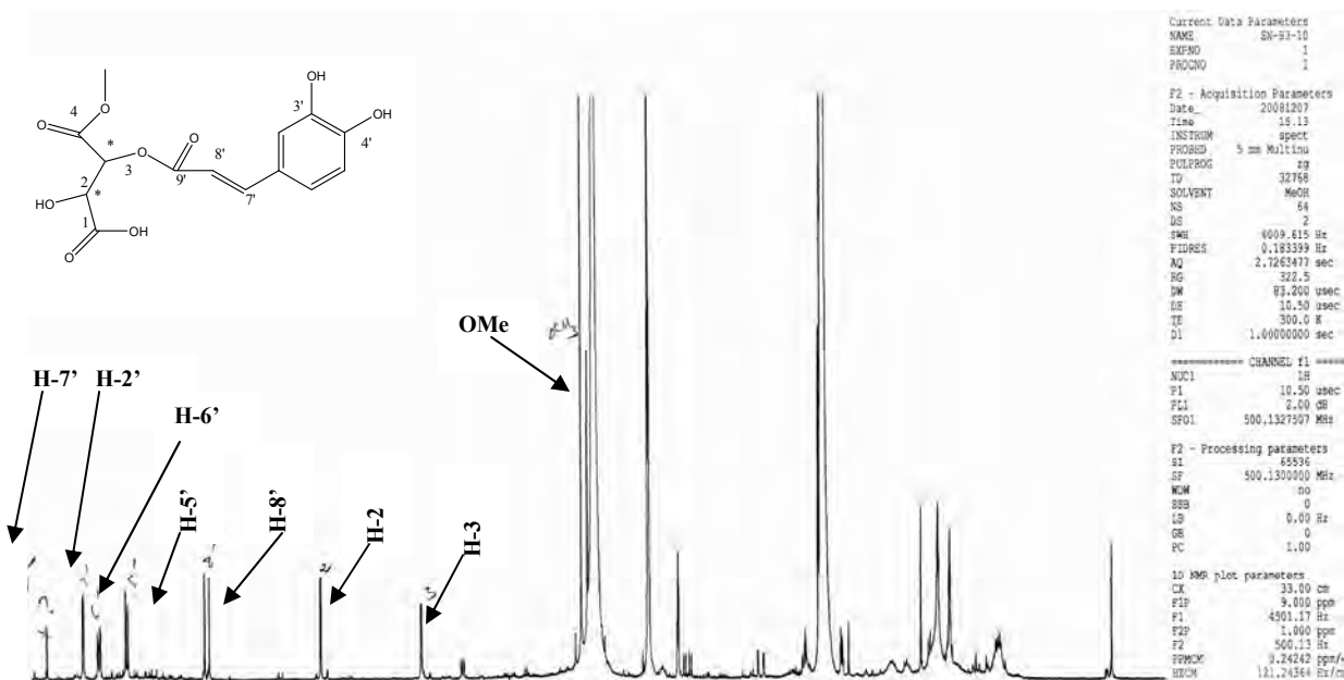
Figure-90 : Spectre RMN-H 1 (500MHz, CD 3 OD, δ ppm) du produit B 3-10 .
