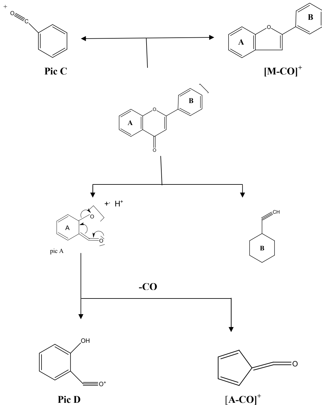
Schéma-1 : Fragmentation d'une flavone.
