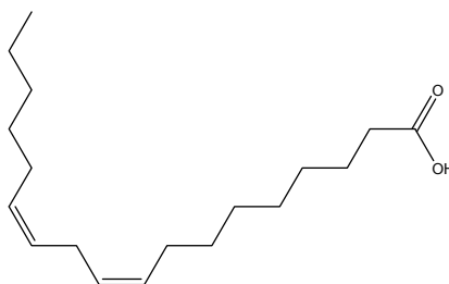
Acide cis, cis-9, 12 octadecadiénoïque (acide linoléique).
