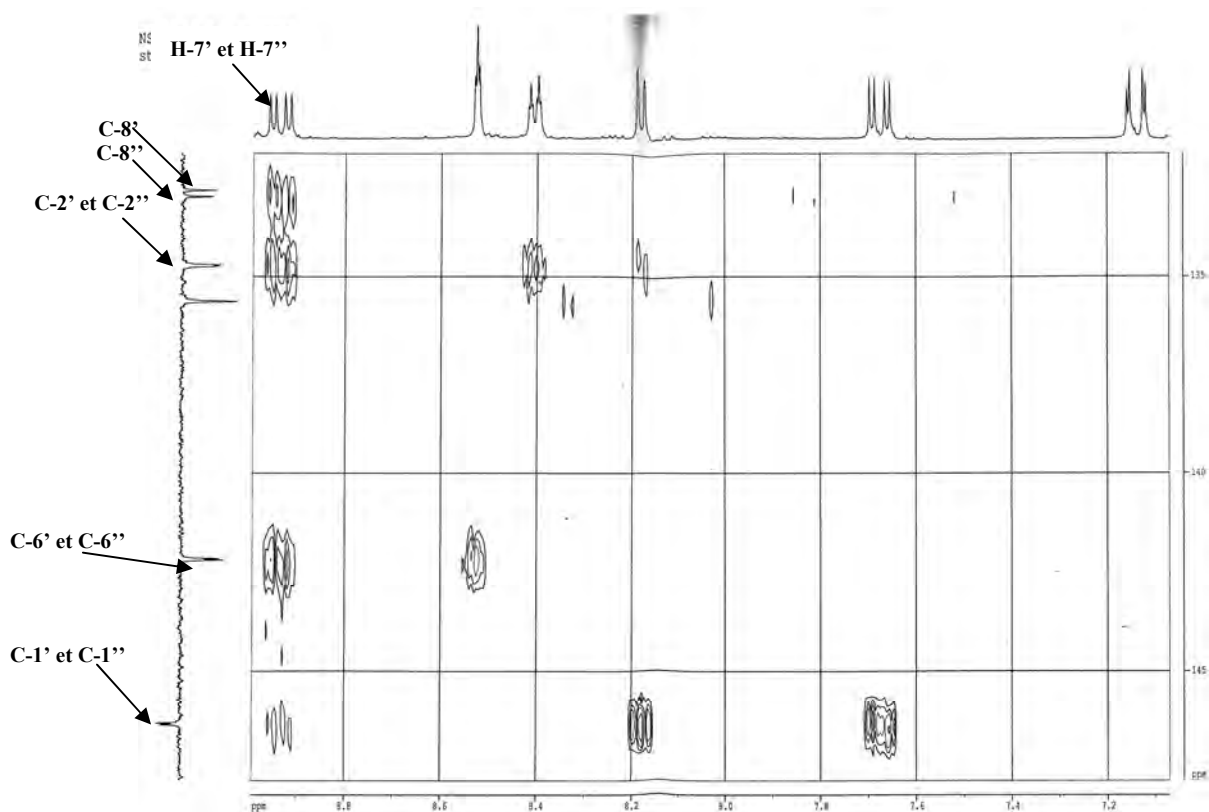
Figure-111: Etallement du spectre HMBC (500MHz, CD 3 OD+ CF 3 COOD) du produit B 3-15 .
