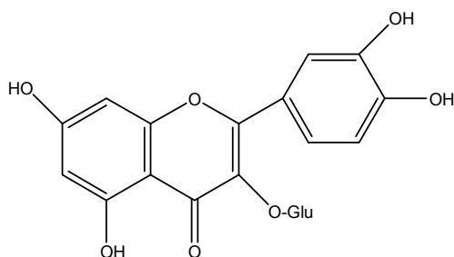
Isoquercétine
