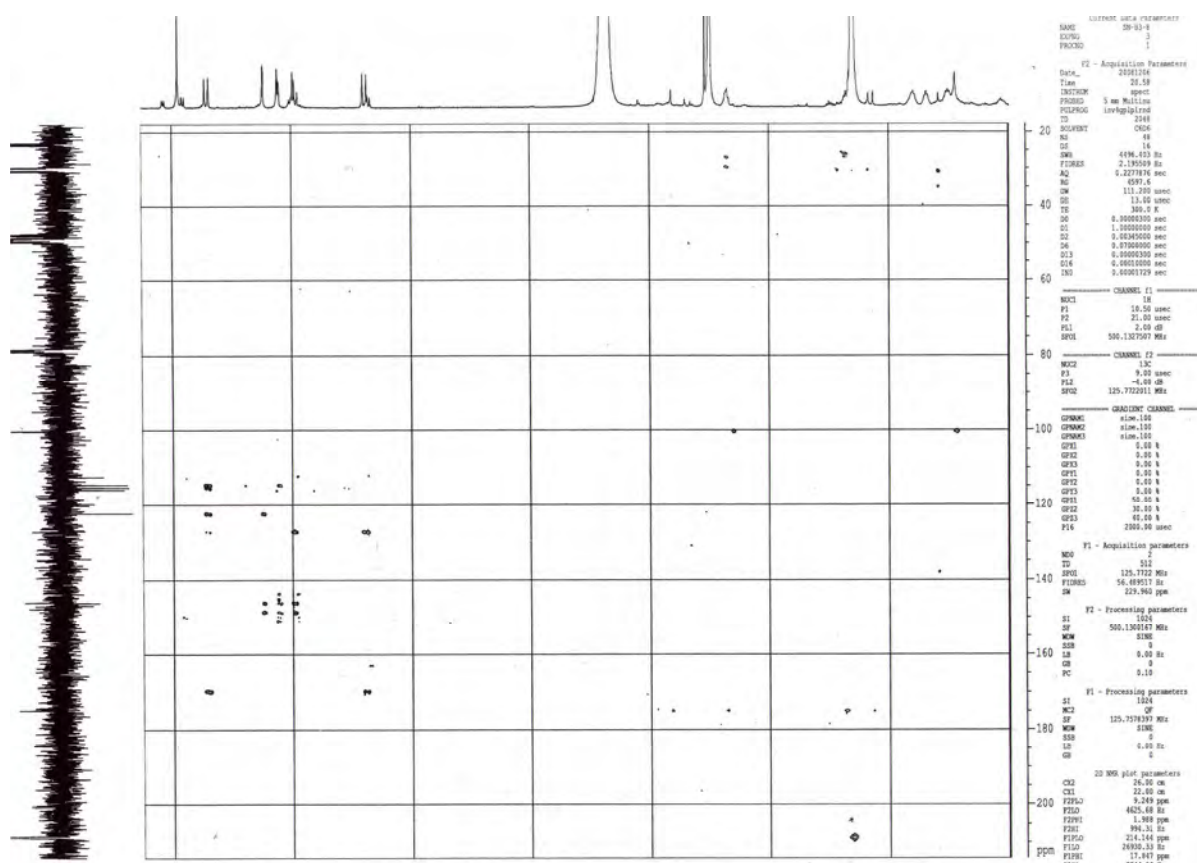
Figure-85 : Spectre HMBC (500MHz, CD 3 OD, \delta ppm) du produit B 3-8 .
