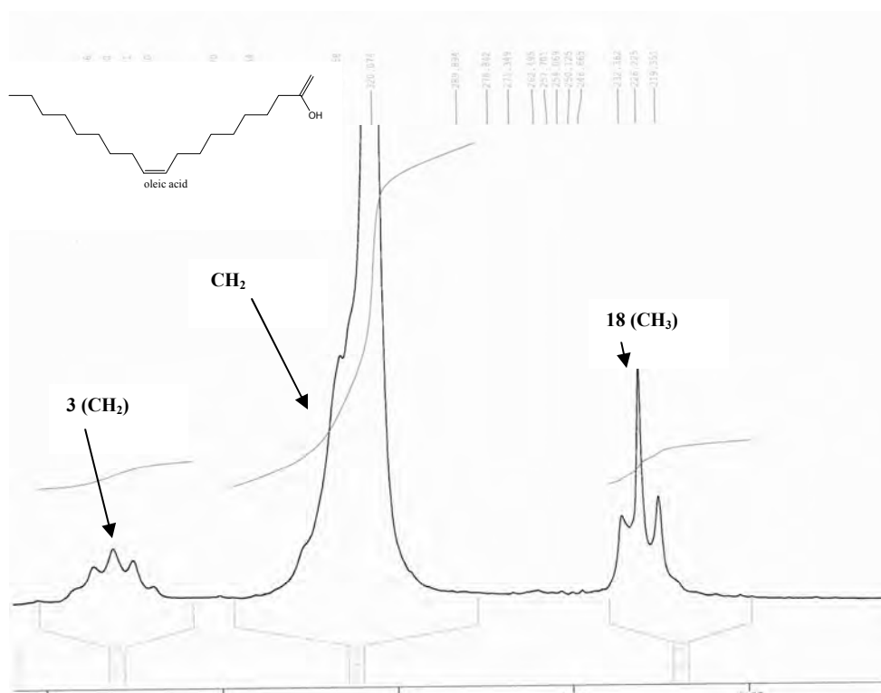
Figure-63 : Etalement du spectre RMN-H 1 du produit F 19-24
