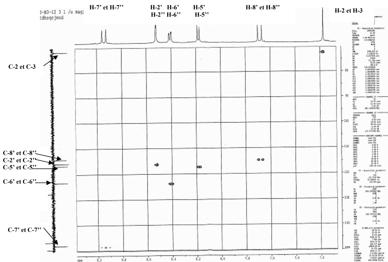
Figure-101 : Spectre HSQC (500MHz, CD 3 OD+ CF 3 COOD) du produit B 3-12 .
