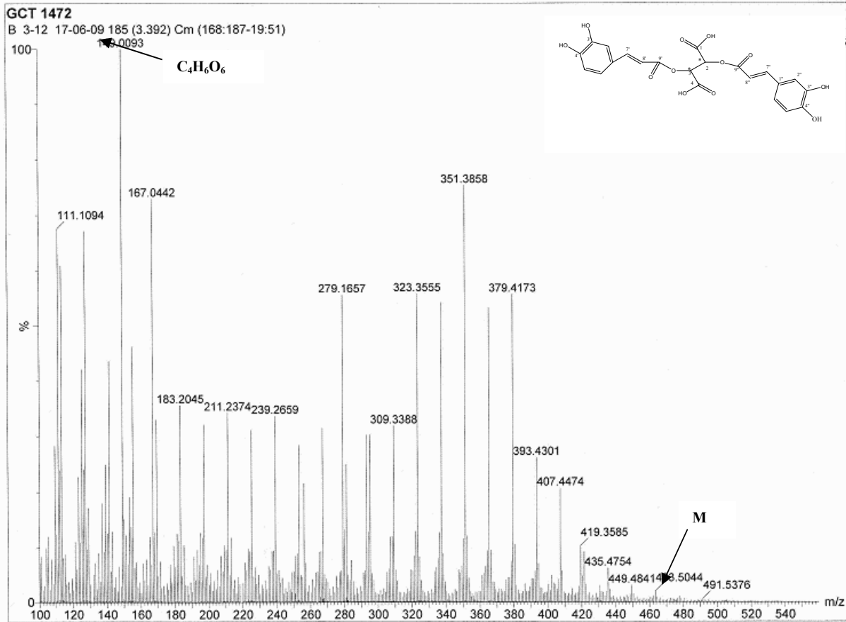
Figure-98 : Spectre EI-MS du produit B 3-12 .
