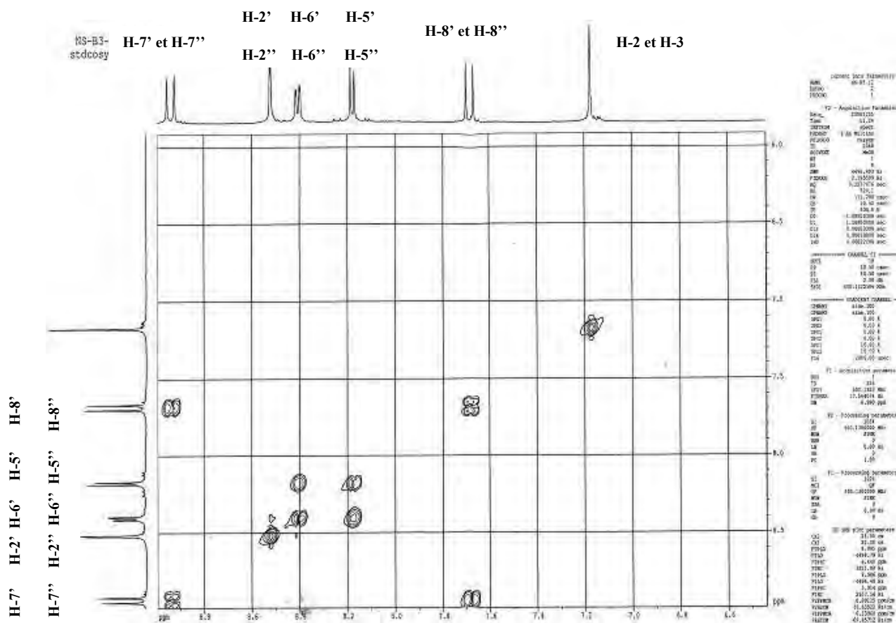
Figure-100 : Spectre COSY (500MHz, CD 3 OD+ CF 3 COOD ) du produit B 3-12 .
