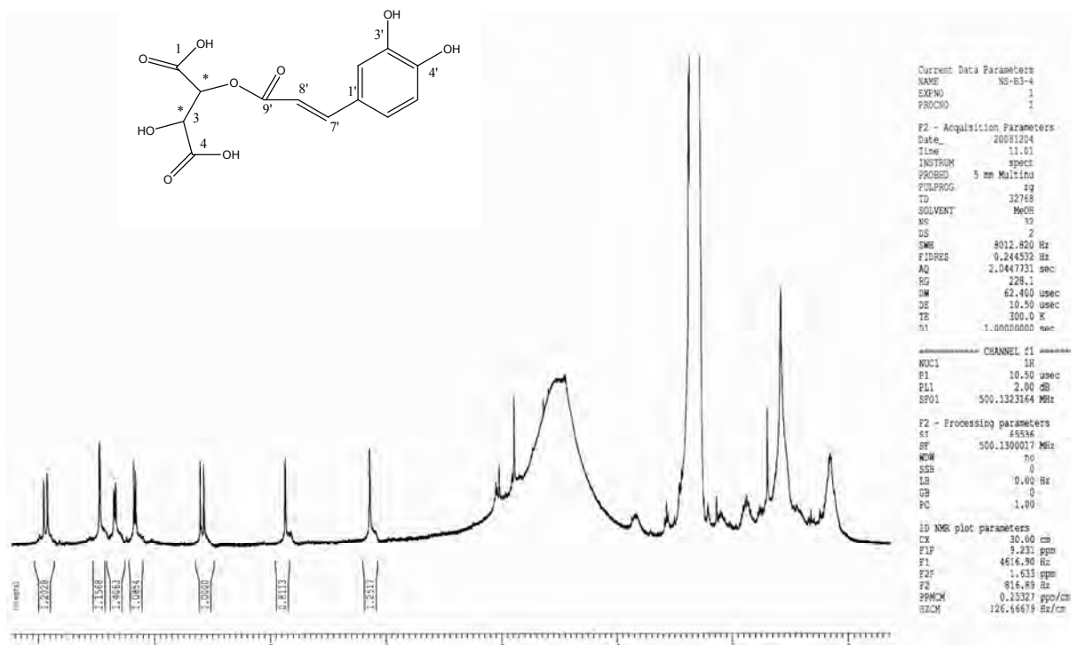
Figure-74 : Spectre RMN- H^1 (500MHz, CD_3OD , \delta ppm) du produit B_{3-4} .
