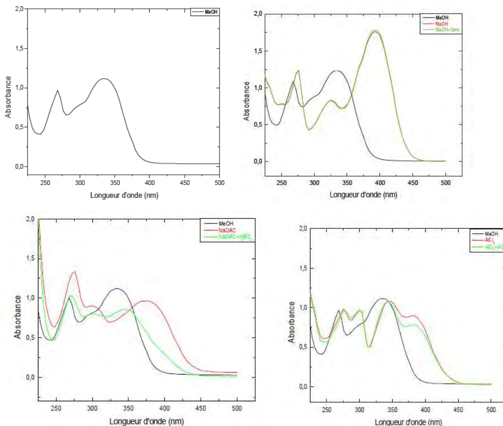
Figure-28: spectres d'absorption UV-visible du composé F 13-2 .
