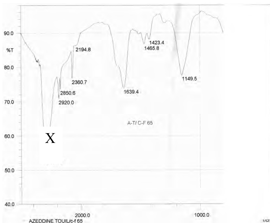
Figure-70 : Spectre infrarouge du composé C-f65.
