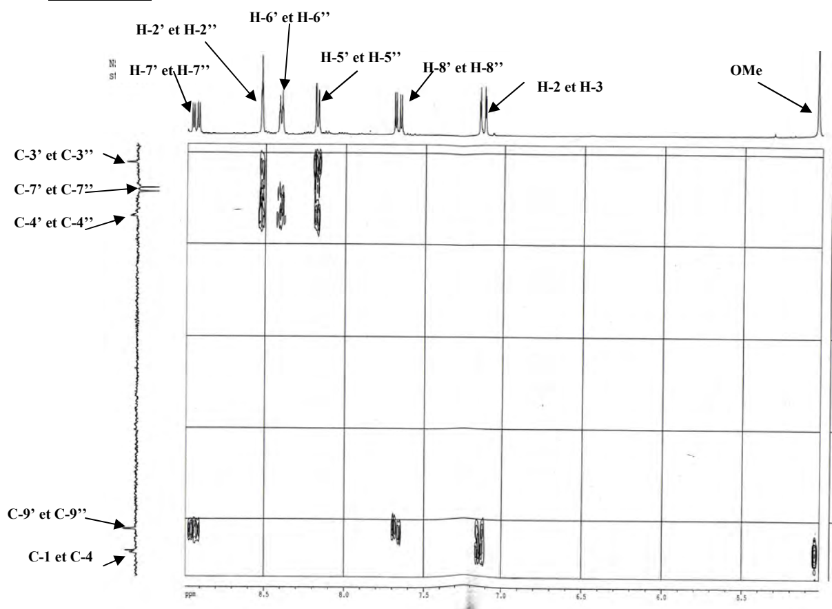
Figure-112: Etallement du spectre HMBC (500MHz, CD 3 OD+ CF 3 COOD) du produit B 3-15 .
