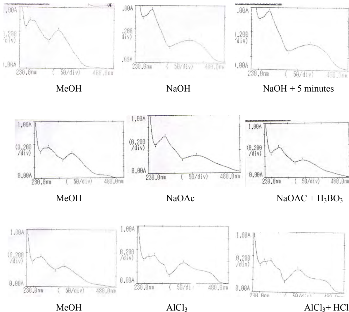
Figure-51: Spectres d'absorption UV-visible du produit F 14 .
