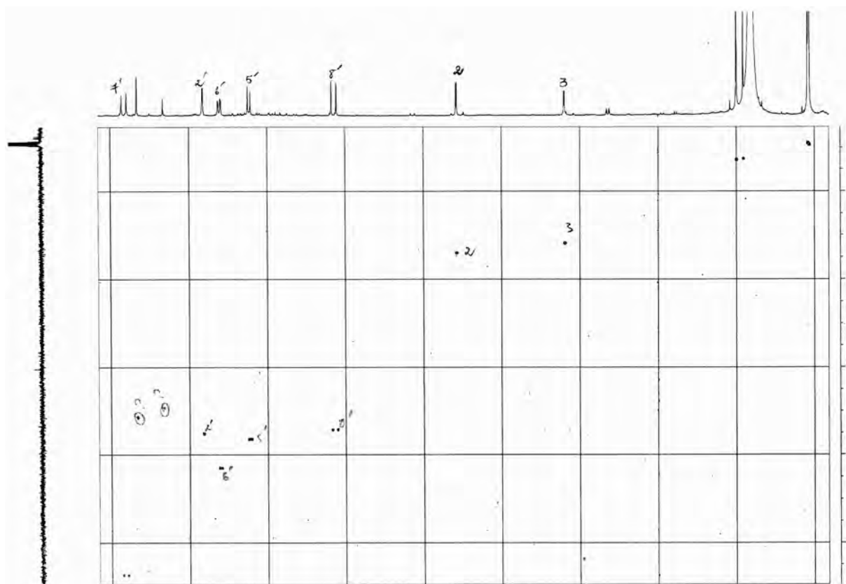
Figure-93 : Etallement du spectre HSQC du produit B 3-10 .
