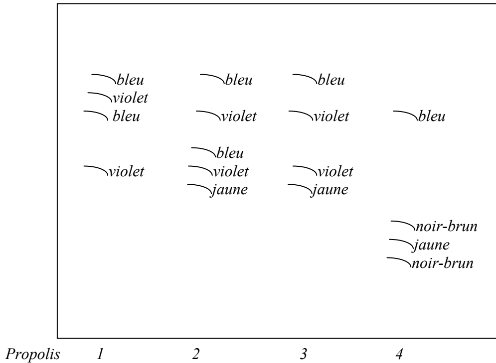
Schéma-12: Chromatographie sur couche mince.
