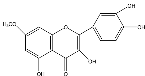
Rhamnétine
