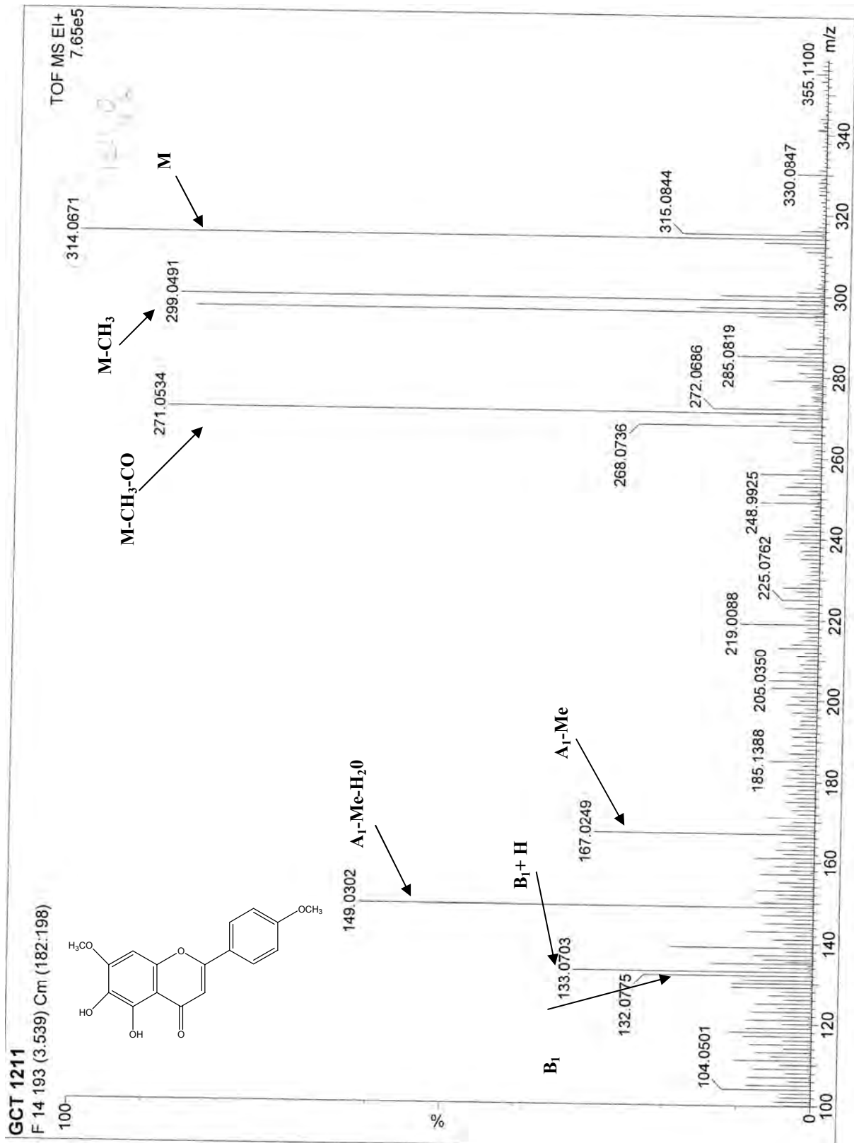
Figure-52 : Spectre EI-MS du produit F 14 .
