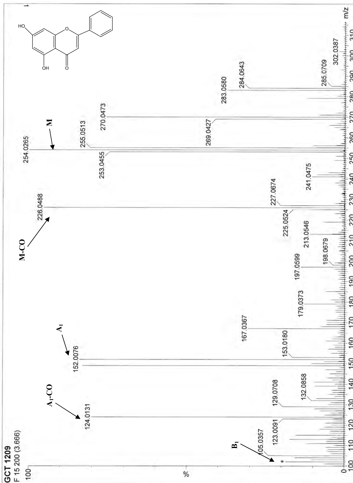
Figure-57 : Spectre EI-MS du produit F 15 .
