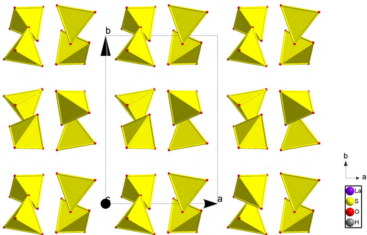
Figure 4: Projection des groupements sulfate selon le plan (a b)
