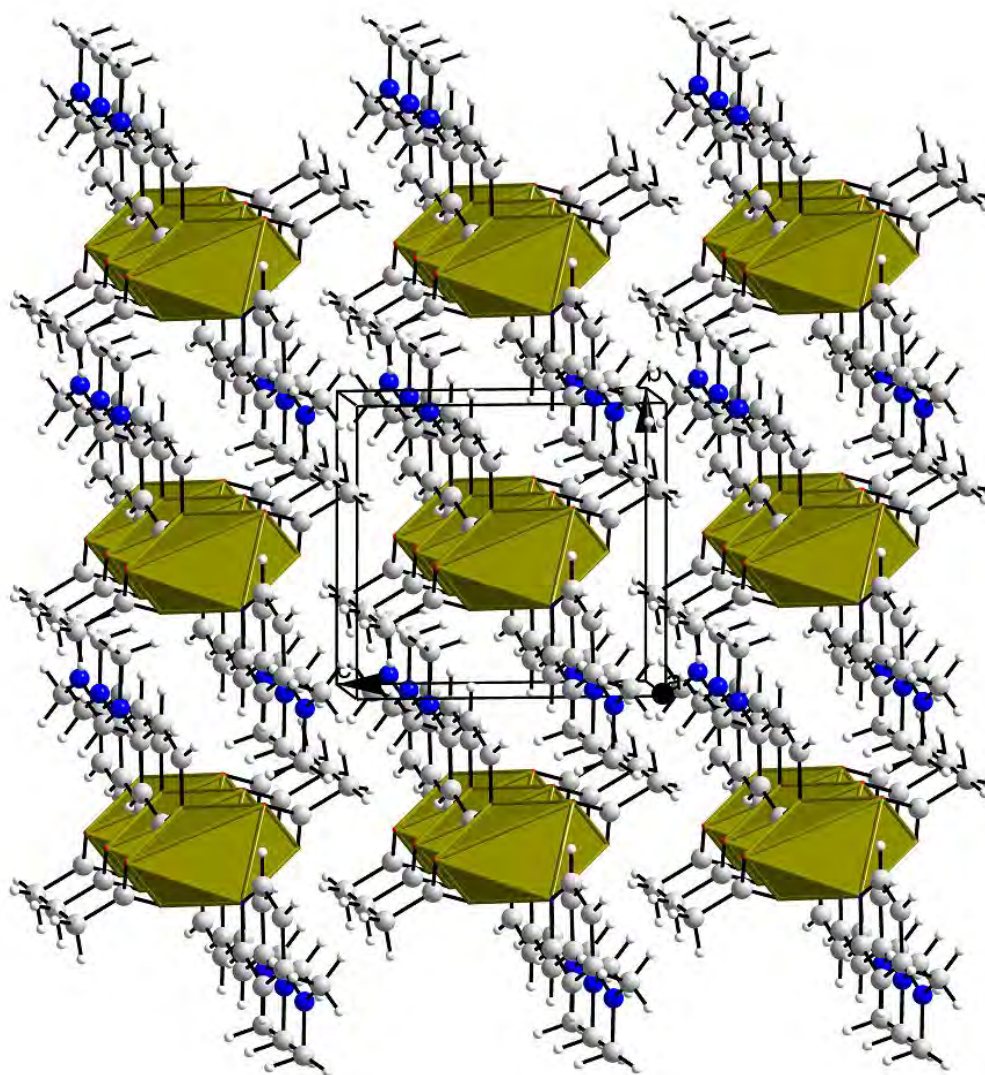
Figure 4 : Vue en perspective de la structure.
