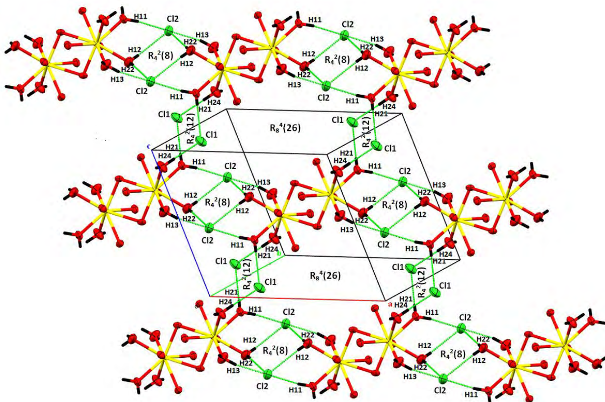
Figure7: Réseau de liaisons hydrogène O-H...Cl parallèle au plan (a c). Les atomes de carbone du cycle aromatique ont été omit par souci de simplification.
