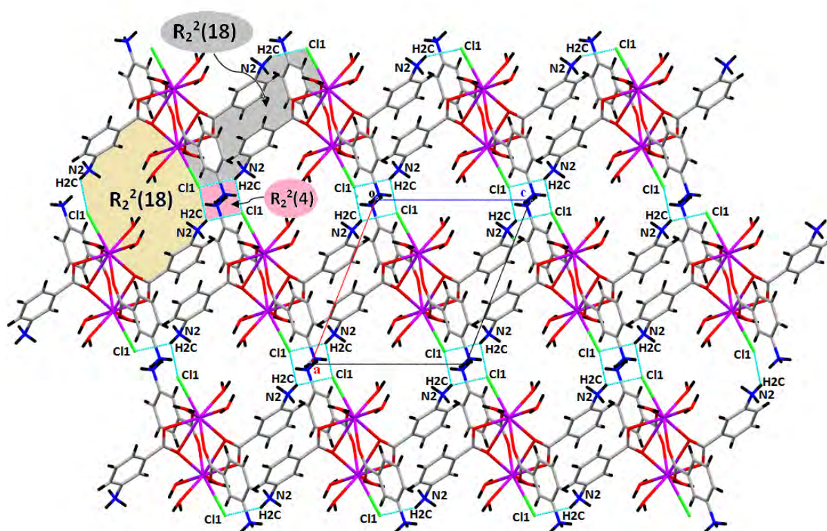
Figure 11: Liaisons hydrogène de type N2-H2C...Cl1 (ii/iv) .
