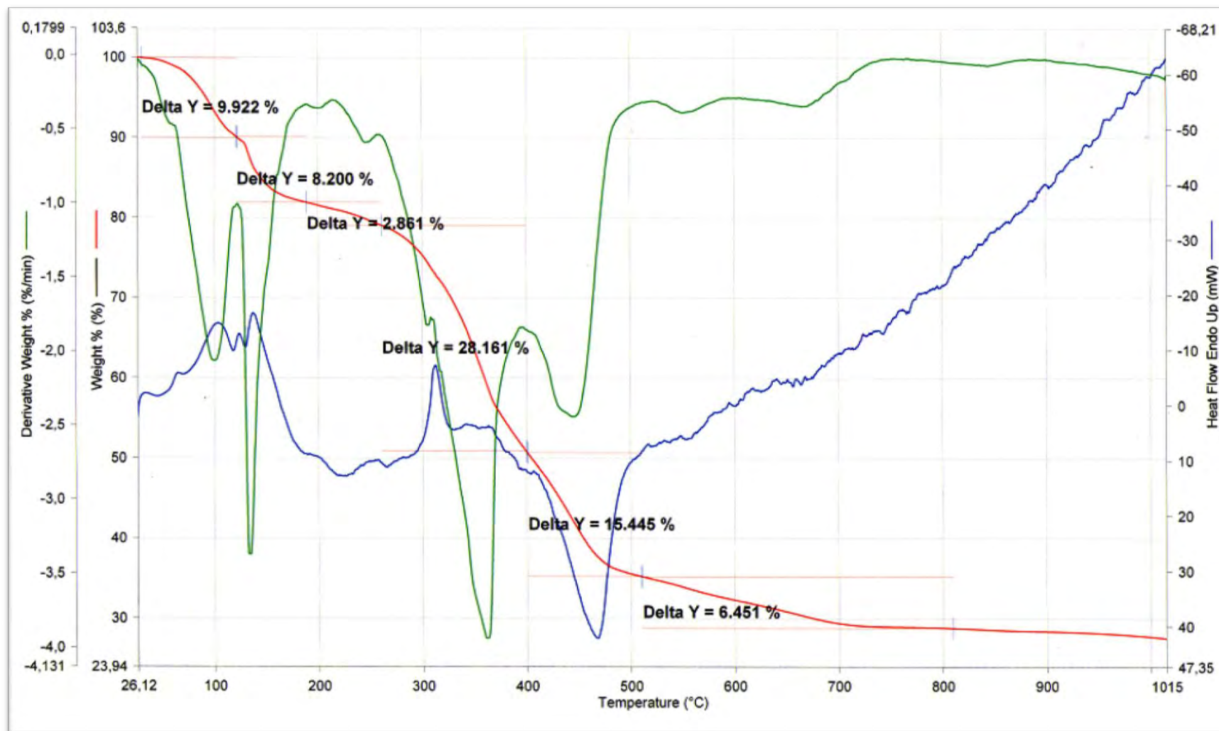
Figure 13: Analyse thermogravimétrique (ATG) et analyse thermique différentielle (ATD) du composé [\text{Nd}_2\text{Cl}_4(\text{H}_2\text{O})_{10}]^{2+}, 4(\text{C}_7\text{H}_{11}\text{N}_2)^+, 6\text{Cl}^-, 2\text{H}_2\text{O} sous \text{N}_2 avec une vitesse de chauffage de 10^\circ\text{C}\cdot\text{min}^{-1} .
