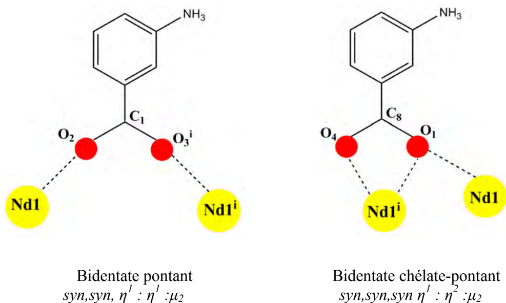
Figure 3 : Modes de coordination des fonctions carboxylates du ligand MABA.
