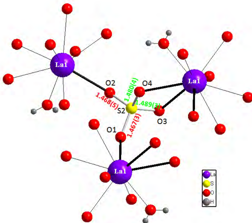
Figure 3 : Coordination tétraédrique des groupes sulfates S1, S2 dans le composé [\text{La}_2(\text{SO}_4)_3(\text{H}_2\text{O})_2] \cdot 2\text{H}_2\text{O} .
