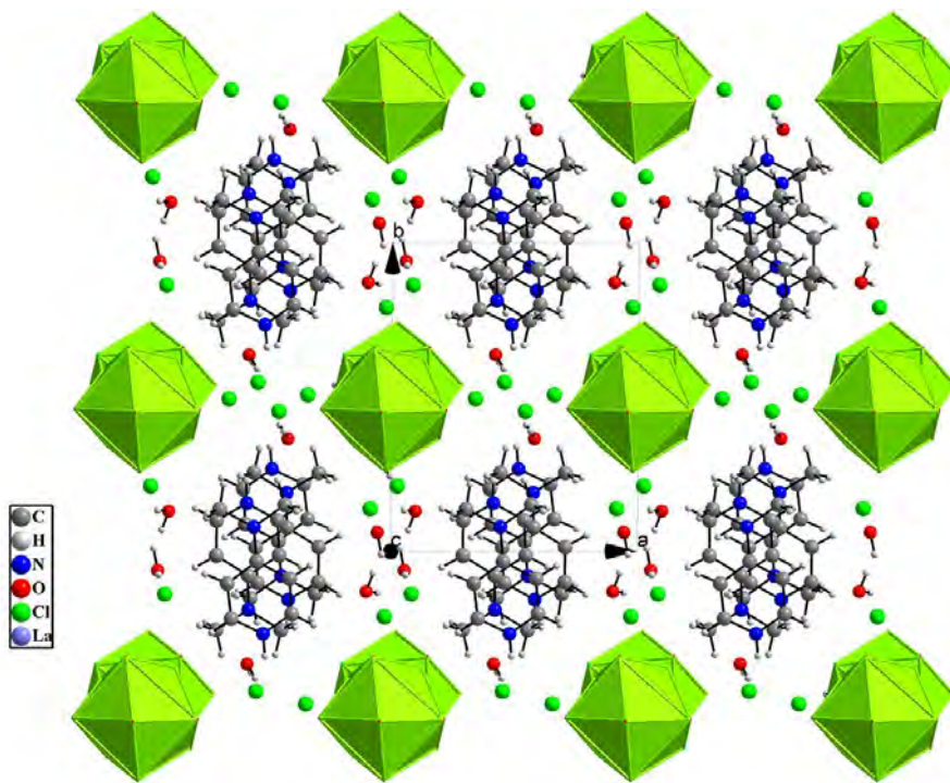
Figure 3 : Projection de la structure selon [001].
