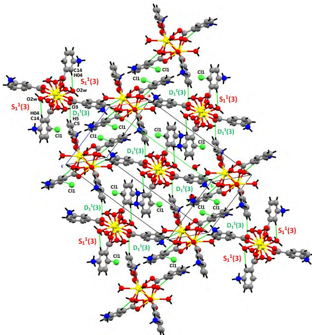
Figure 9: Liaisons hydrogène de type C-H...O et C-H...Cl.
