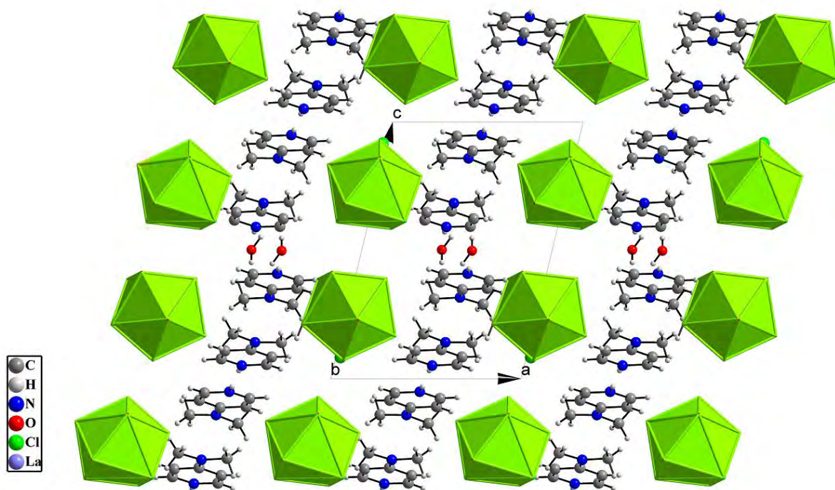
Figure 5 : Projection de la structure selon [010].
