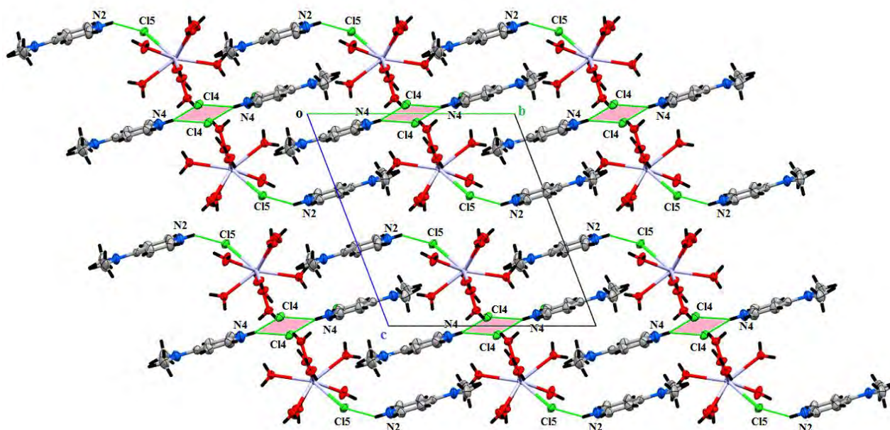
Figure 14: Liaisons hydrogène de type N-H...Cl.
