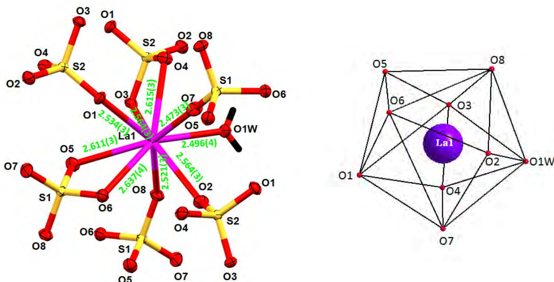
Figure 2 : Schéma représentant la coordination de l'atome de lanthane dans la composé [\text{La}_2(\text{SO}_4)_3(\text{H}_2\text{O})_2] \cdot 2\text{H}_2\text{O}
