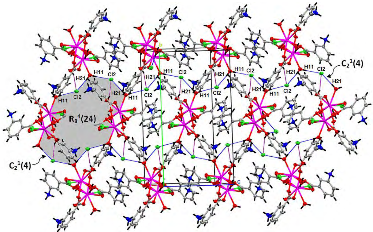
Figure 9: Enchaînement de: O1W-H11...Cl2 ii et O1W-H21...Cl2 v .
