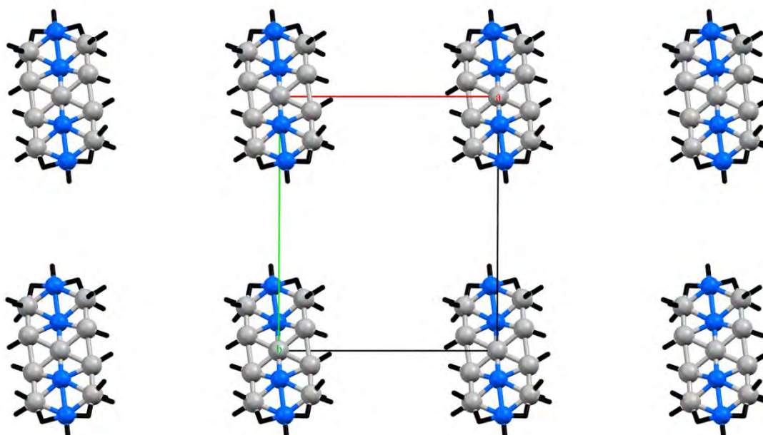
Figure 4: Enchaînement du 4-(diméthylamino)pyridinium désordonné selon le plan (a b)
