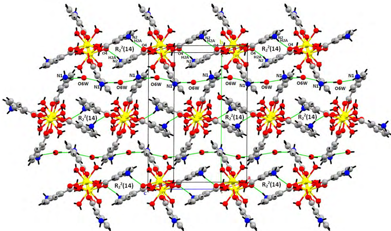
Figure 8: Liaisons hydrogène de type N-H...O.
