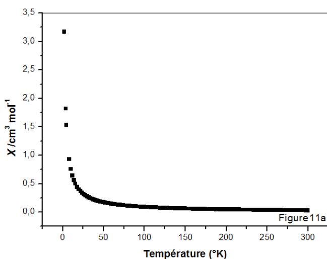
Figure 11a : Evolution de la susceptibilité magnétique en fonction de la température
