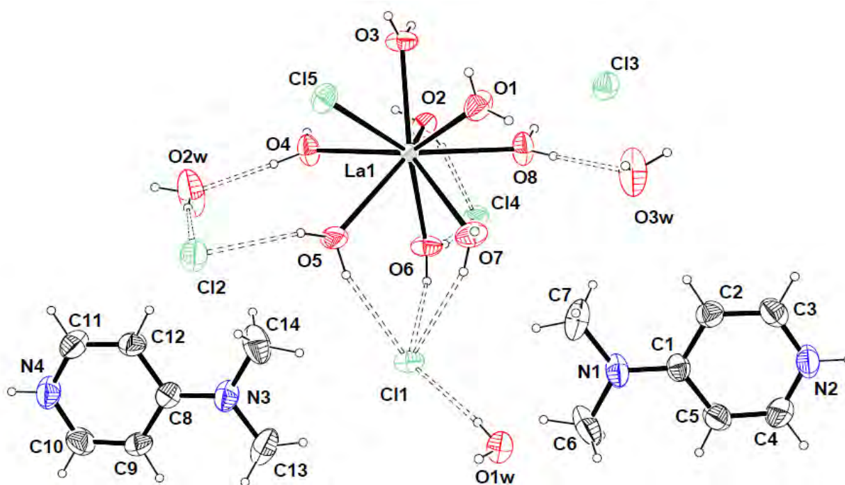
Figure 2 : L'unité asymétrique du composé [\text{LaCl}(\text{H}_2\text{O})_8]^{2+}, 2(\text{C}_7\text{H}_{11}\text{N}_2)^+, 4\text{Cl}^-, 3\text{H}_2\text{O}
