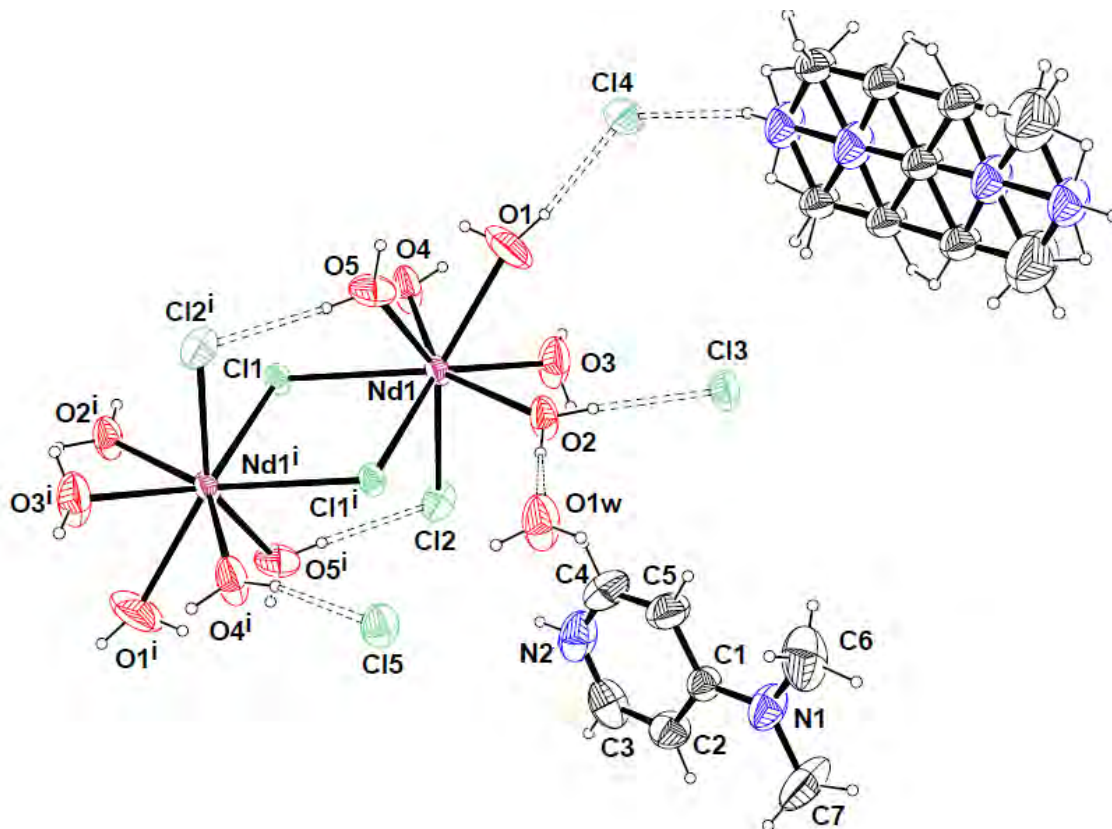
Figure 2 : La structure du composé [\text{Nd}_2\text{Cl}_4(\text{H}_2\text{O})_{10}](\text{C}_7\text{H}_{11}\text{N}_2)_2\text{Cl}_6 \cdot 2\text{H}_2\text{O} [Code de symétrie : (i) -x+1, -y+1, -z ]
