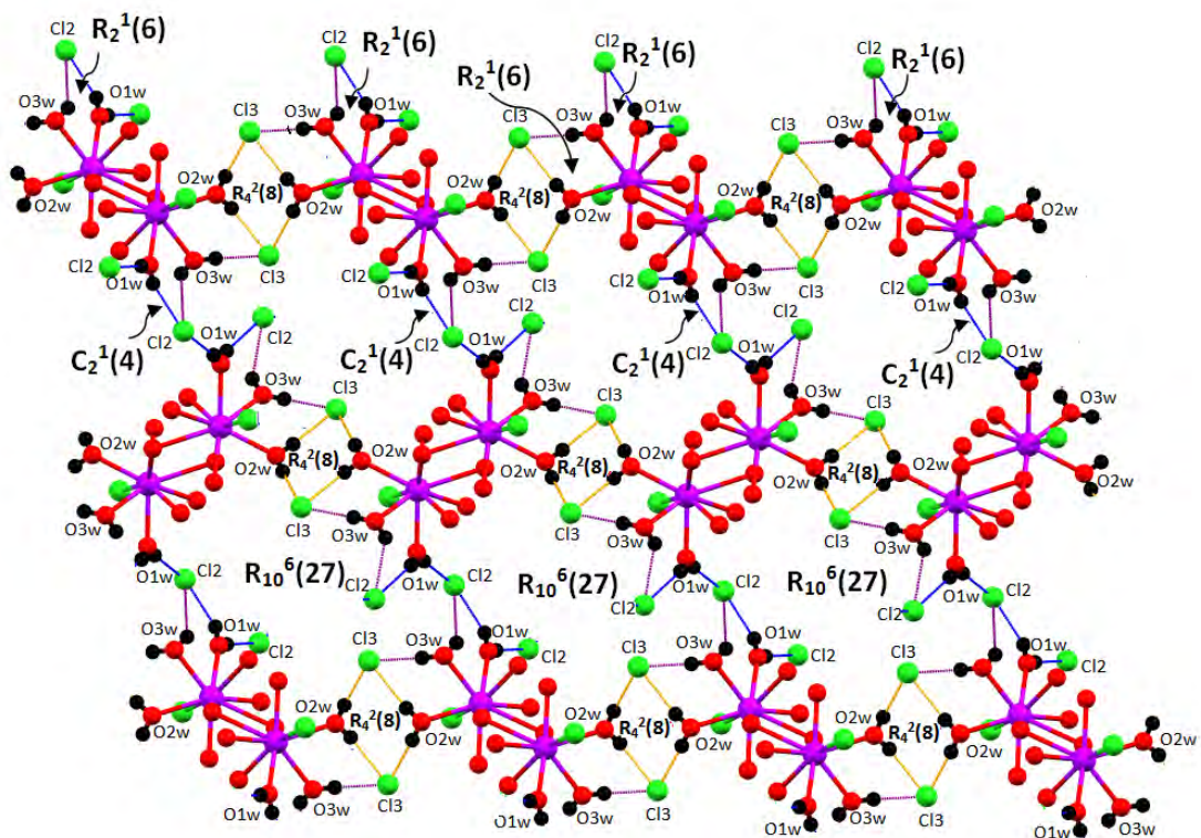
Figure 10: Réseau des liaisons hydrogène de type O-H...Cl.
