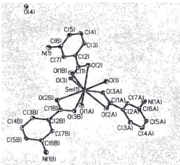
Figure 2a : La structure du composé [\text{Sm}(\text{C}_7\text{H}_6\text{NO}_2)_3(\text{H}_2\text{O})_3] \cdot \text{H}_2\text{O} [73]
