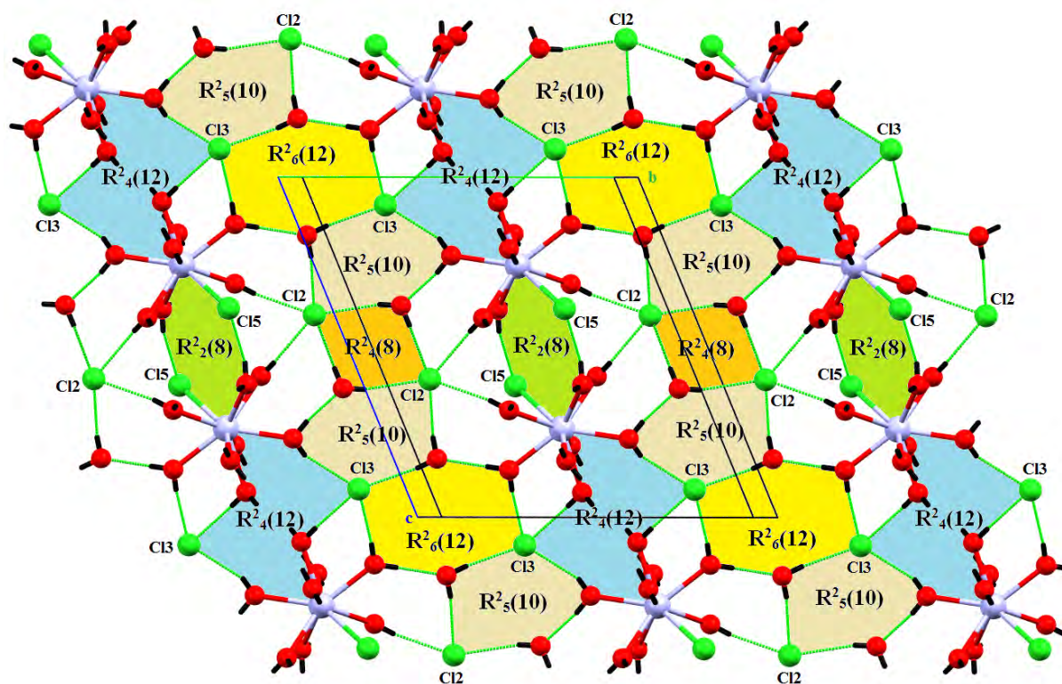
Figure 13a: Réseau des liaisons hydrogène de types O-H water ...Cl et O-H water ...O selon le plan (b c). Les atomes du cation organique ne sont pas représentés.
