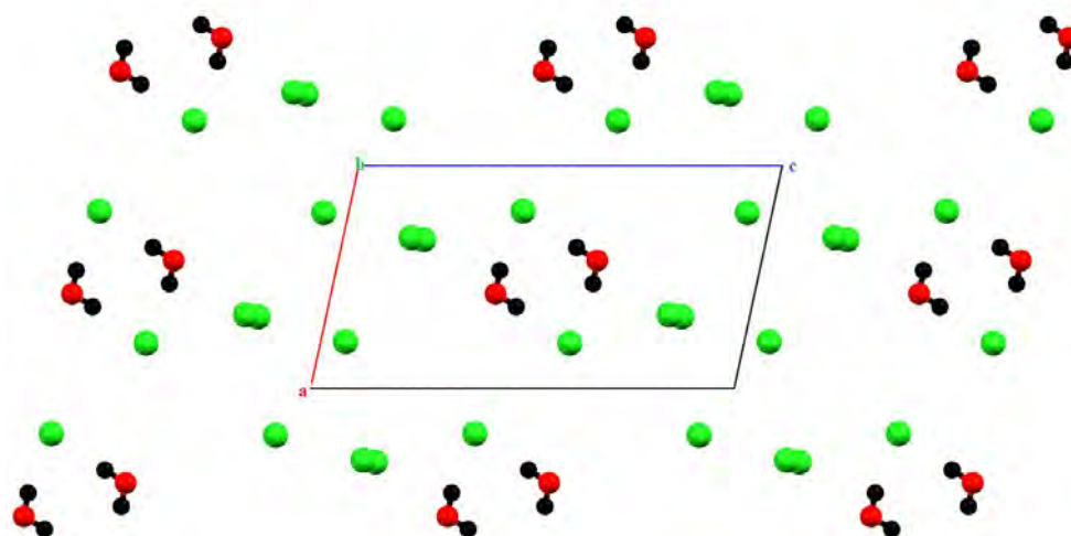
Figure 7: Enchaînement des molécules d'eau et des anions chlorure selon le plan (a c)
