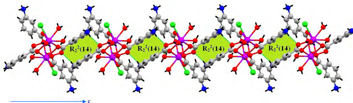
Figure 13: Liaisons hydrogène : N2-H2A...O4 ii selon [001].
