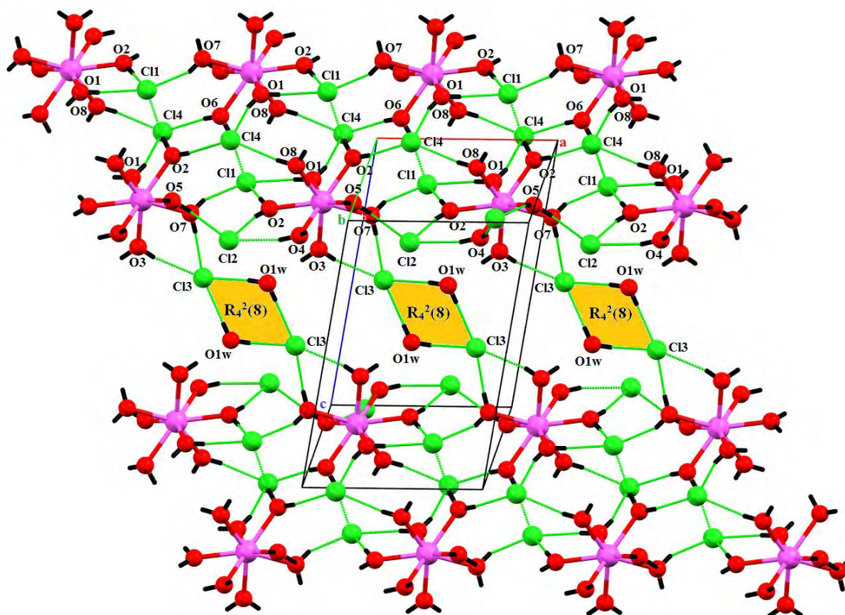
Figure 8: Liaisons hydrogène de type O-H water ...Cl
