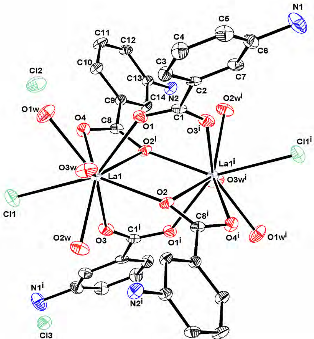
Figure 4: Le complexe [\text{La}_2(\text{C}_7\text{H}_7\text{NO}_2)_4\text{Cl}_2(\text{H}_2\text{O})_6]\text{Cl}_4 \cdot 2\text{H}_2\text{O} Les atomes d'hydrogène n'ont pas été représentés par souci de simplification. (i) : -x+1, -y+1, -z+1 .
