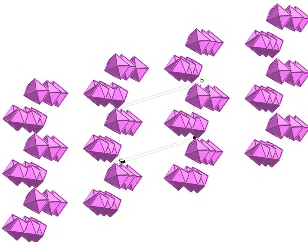
Figure 6: Enchaînement des polyèdres [\text{Er}(\text{H}_2\text{O})_8]^{3+} selon le plan (b c)
