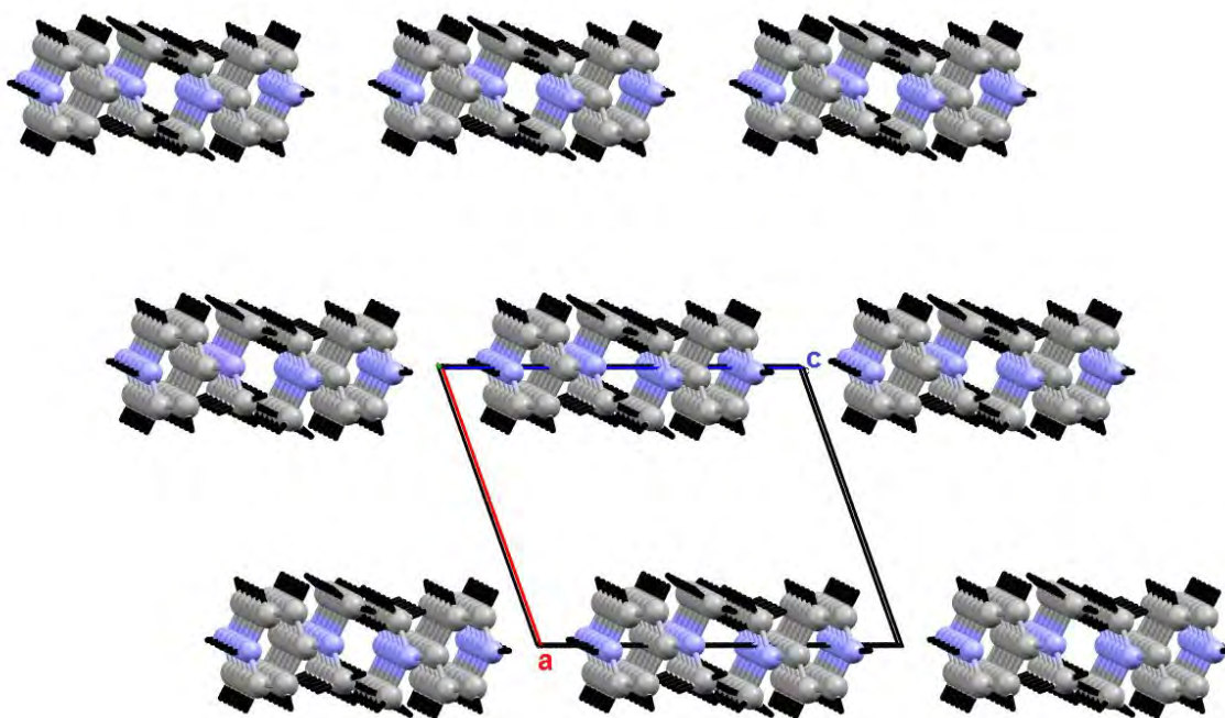
Figure 3: Enchaînement du 4-(diméthylamino)pyridinium ordonné selon le plan (a c)
