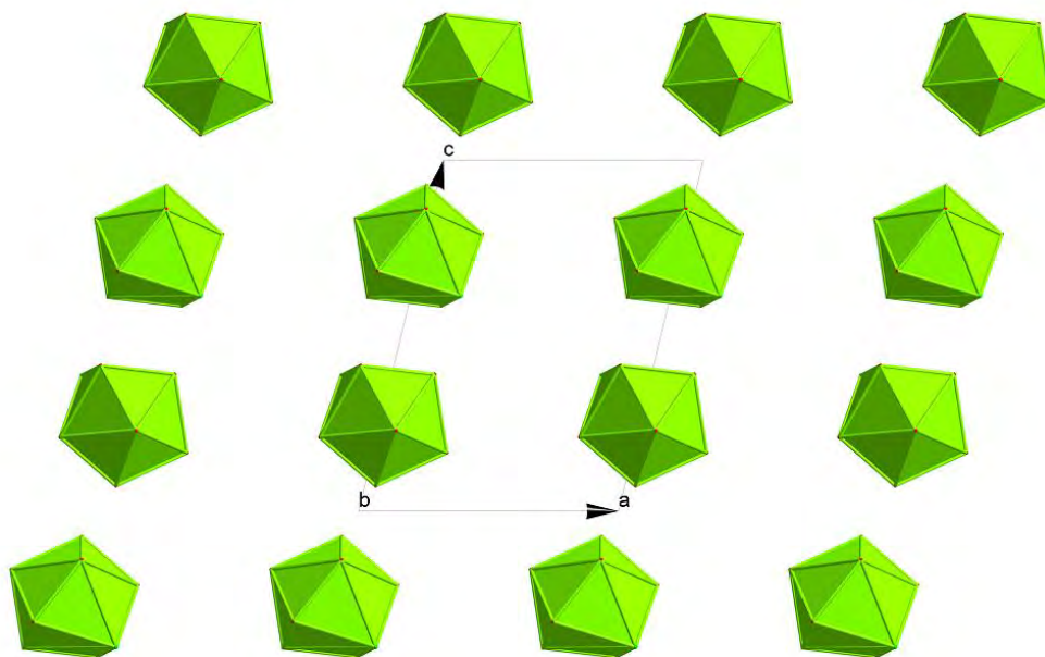
Figure 10: Enchaînement des polyèdres [\text{LaCl}(\text{H}_2\text{O})_8]^{2+} selon le plan (a c)
