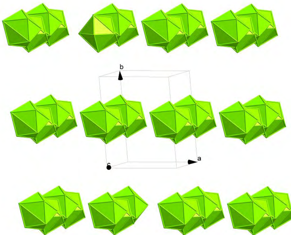
Figure 11: Vue en perspective des polyèdres
