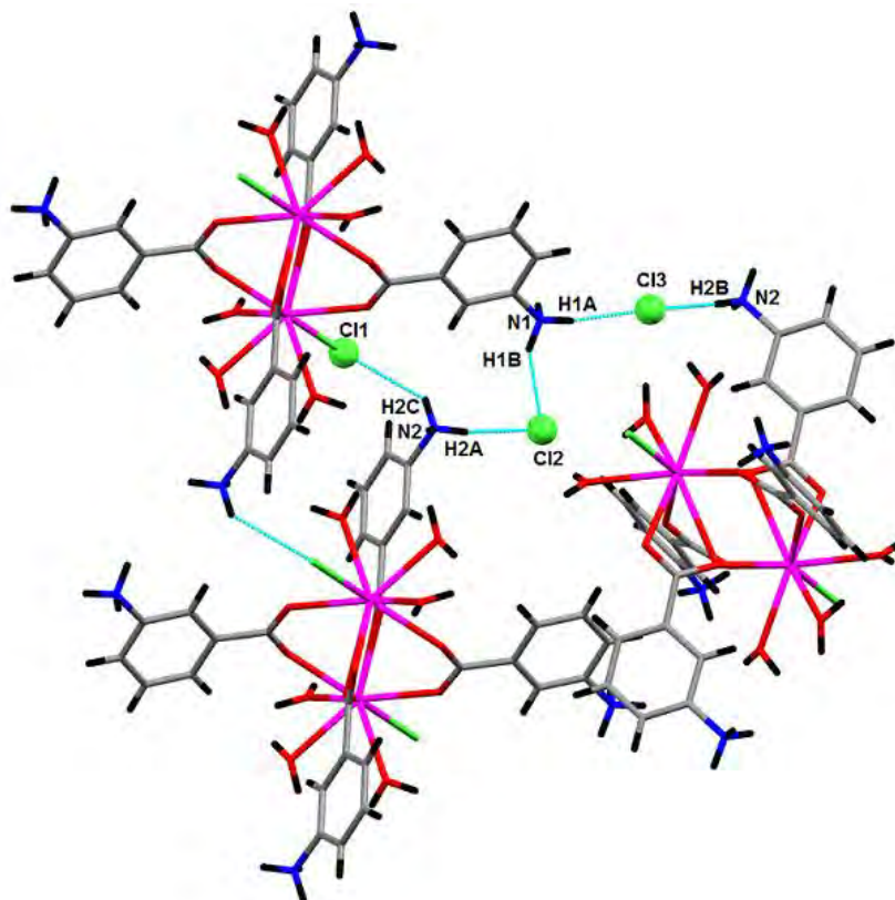
Figure 12: Liaisons dipôle-dipôle de type N-H...Cl.
