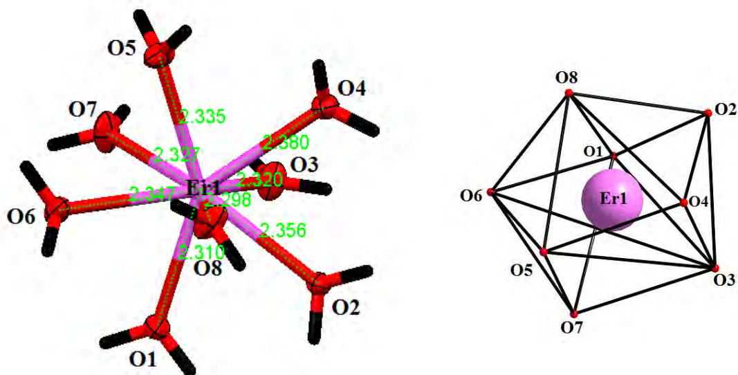
Figure 5: Schéma représentant la coordination 8 de l'atome de l'erbium
