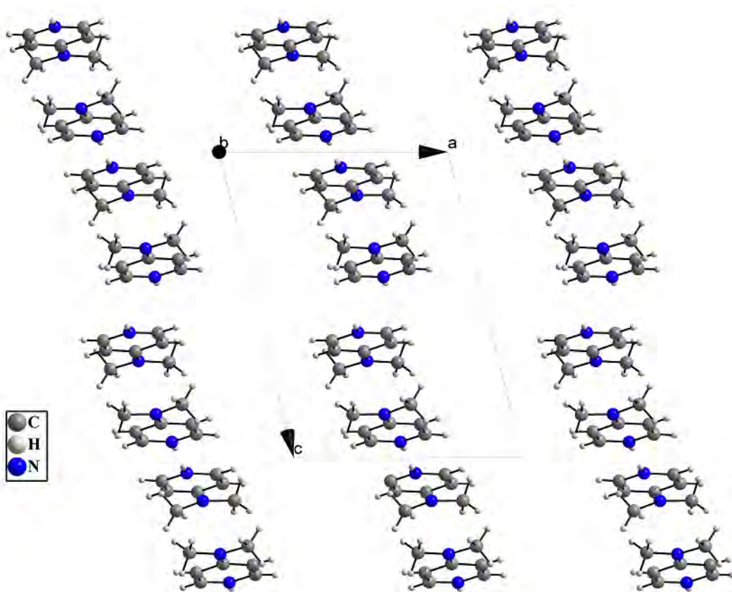
Figure 6: Enchaînement du 4-(diméthylamino)pyridinium selon [010].
