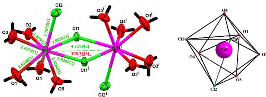
Figure 5: Schéma du dimère formé par deux atomes de néodyme [Code de symétrie (i) : -x+1, -y+1, -z ]
