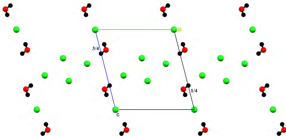
Figure 8: Enchaînement des molécules d'eau et des anions chlorures dans le plan (b c)
