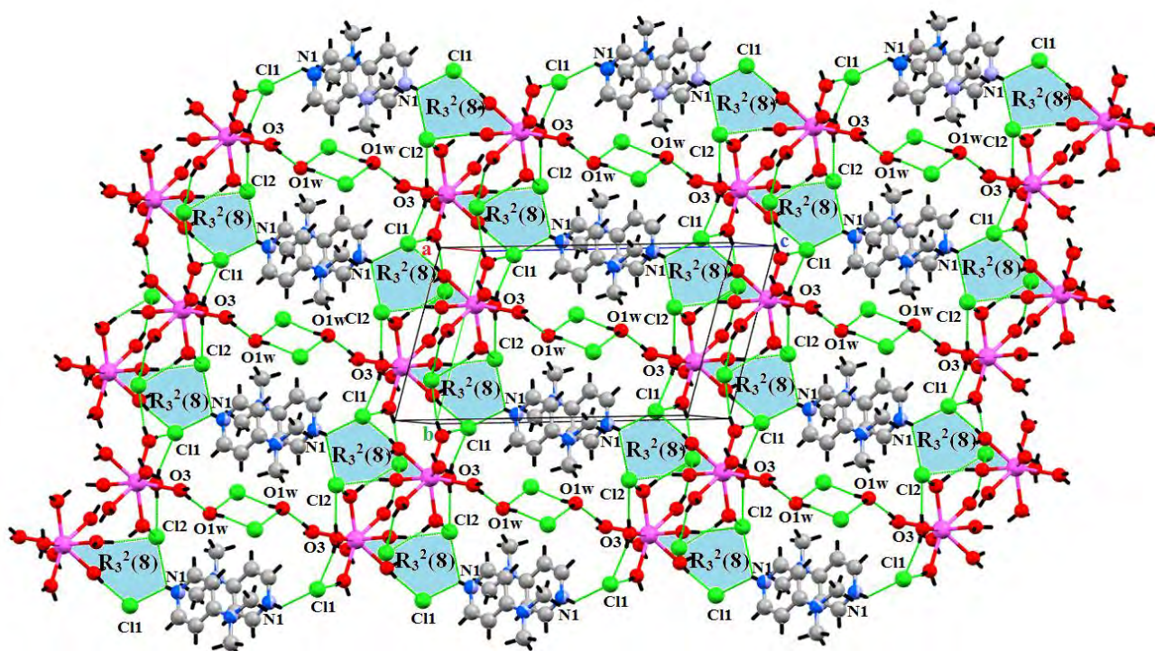
Figure 9: Liaisons hydrogène de type O-H water ...Cl, N-H...Cl et O-H...O water
