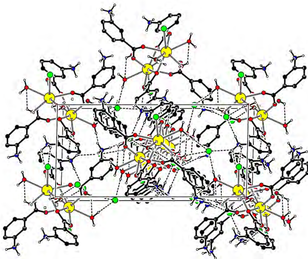
Figure 8: Liaisons hydrogène dans le composé [\text{La}_2(\text{C}_7\text{H}_7\text{NO}_2)_4\text{Cl}_2(\text{H}_2\text{O})_6]\text{Cl}_4 \cdot 2\text{H}_2\text{O} (Vue selon l'axe a )
