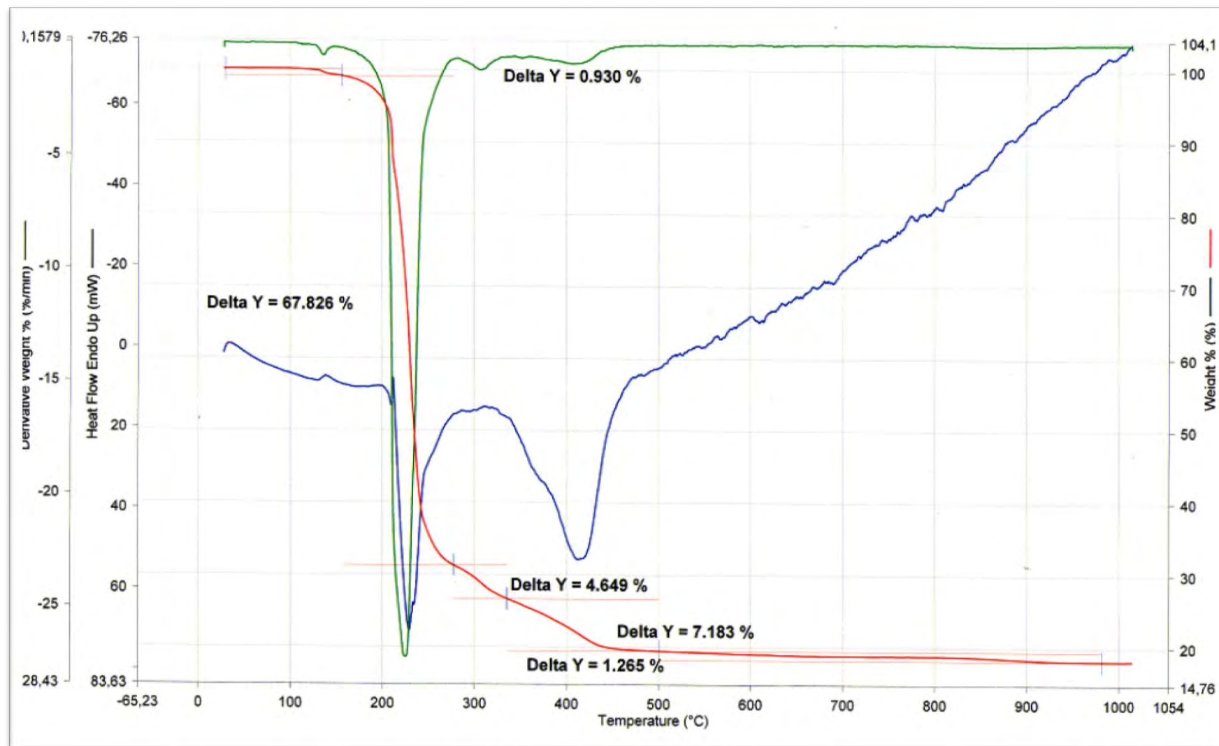
Figure 6: Analyse thermogravimétrique (ATG) et analyse thermique différentielle (ATD) du composé [\text{Cu}(\text{C}_2\text{H}_3\text{O}_2)_2(\text{C}_7\text{H}_{10}\text{N}_2)_2] sous \text{N}_2 avec une vitesse de chauffage de 10^\circ\text{C}\cdot\text{min}^{-1} .
