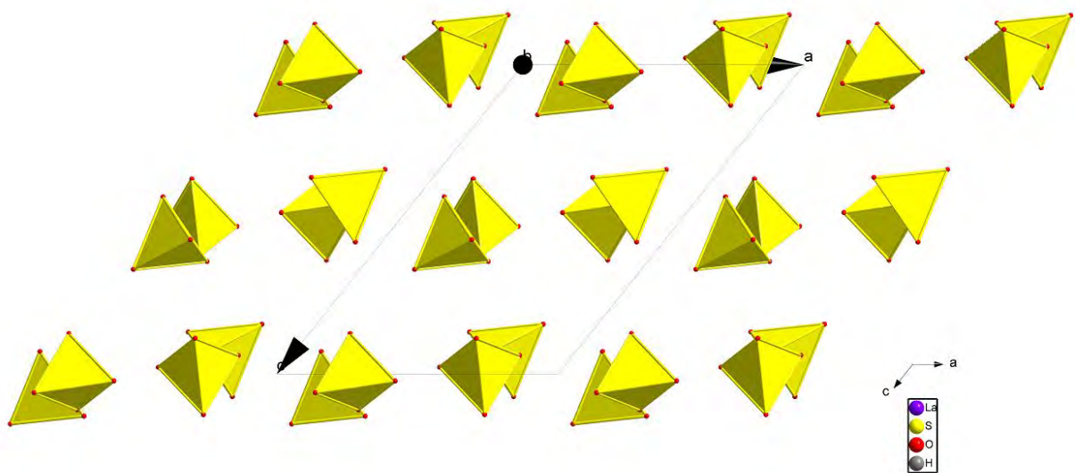
Figure 6: Projection des groupements sulfate selon le plan (a c)
