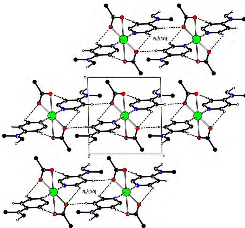
Figure 5 : Liaisons hydrogène de type C-H...O selon le plan (b c).
