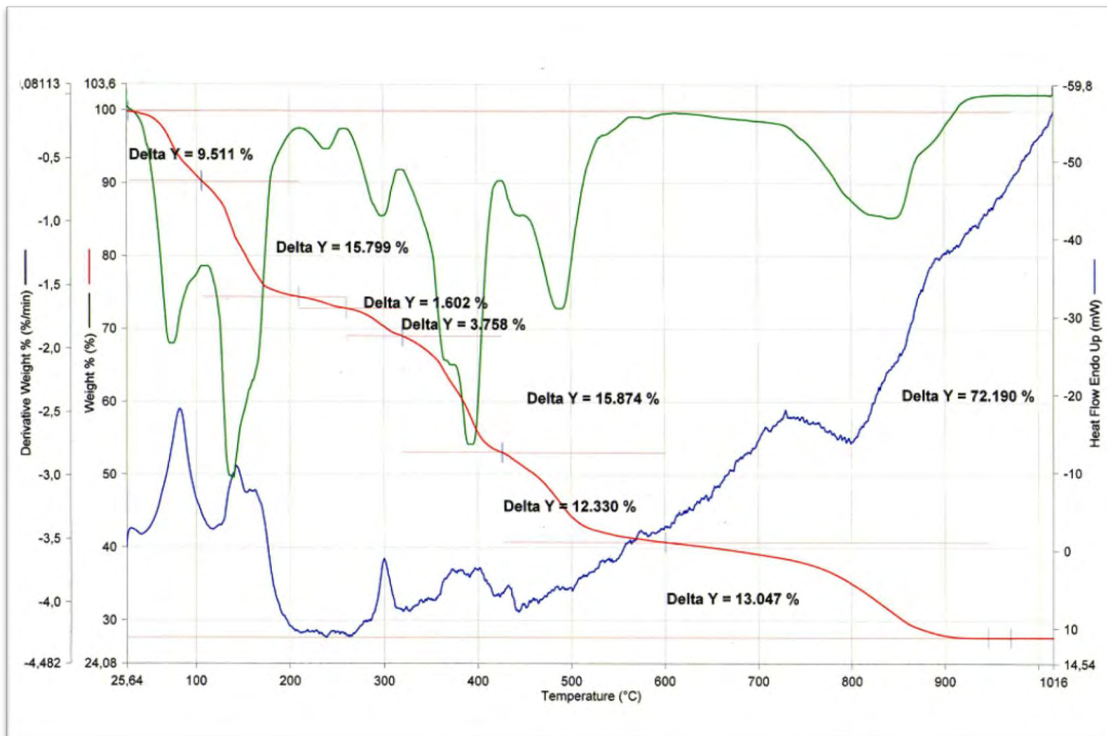
Figure 10: Analyse thermogravimétrique (ATG) et analyse thermique différentielle (ATD) du composé \text{Er}(\text{H}_2\text{O})_8]^{3+}, (\text{C}_7\text{H}_{11}\text{N}_2)^+, 4\text{Cl}^-, \text{H}_2\text{O} sous \text{N}_2 avec une vitesse de chauffage de 10^\circ\text{C}\cdot\text{min}^{-1} .
