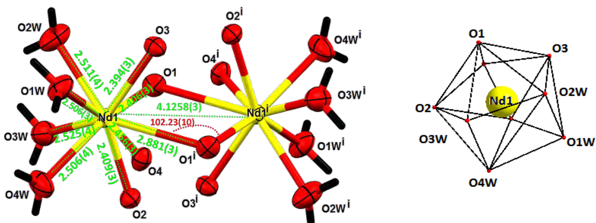
Figure 4: Environnement de l'atome de néodyme dans le dimère : distances de liaisons [Code de symétrie (i) : 1 -x, 1-y, 1-z].
