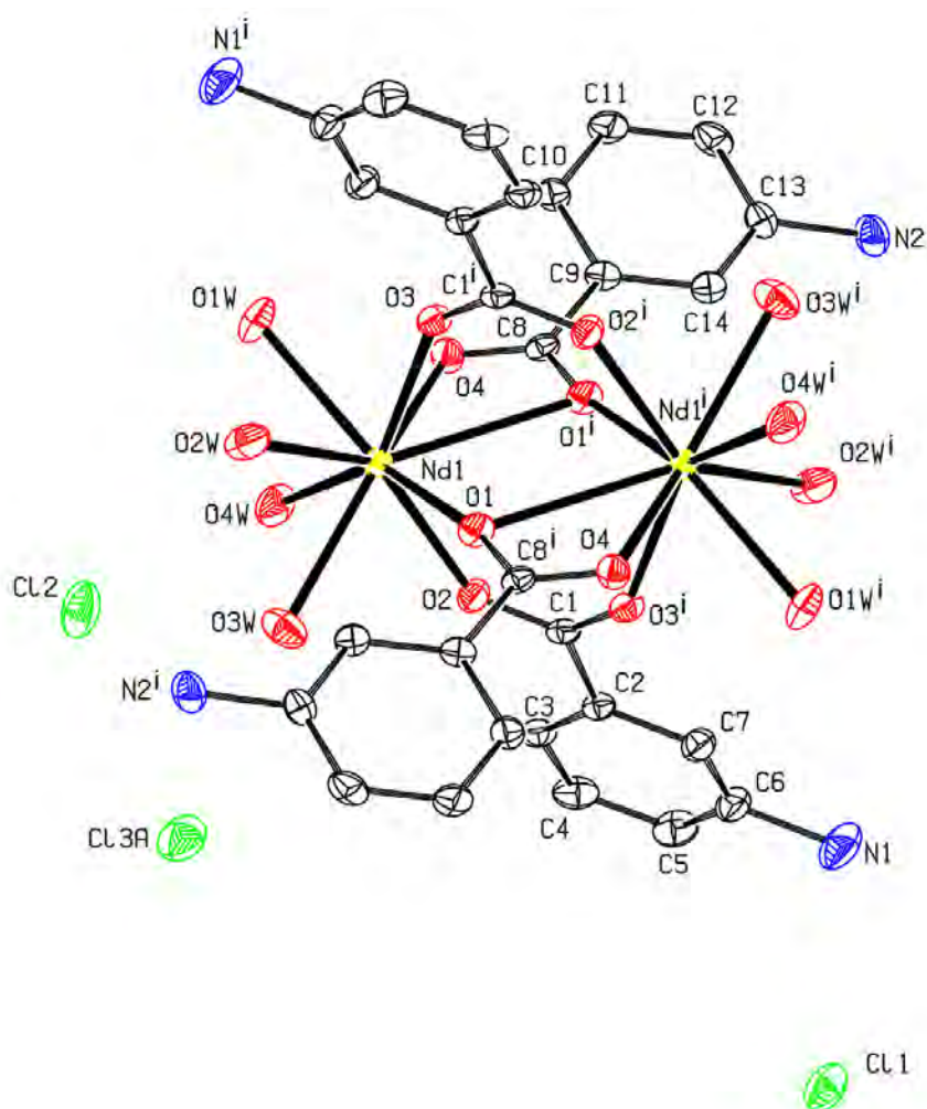
Figure 2 : La structure du composé [Nd 2 (C 7 H 7 NO 2 ) 4 (H 2 O) 8 ]Cl 6 .4H 2 O Les atomes d'hydrogène sont omis par souci de simplification. (i) : -x+1, -y+1, -z+1.
