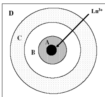
Figure 4: Zones d'hydratation d'un cation Ln 3+ . Zone A, la première sphère d'hydratation et Zone B, la seconde sphère d'hydratation, Zone C, eau désordonnée, Zone D, le solvant [14]
