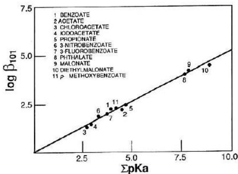
Figure 5 : Relation entre les constantes de stabilité \log \beta_{SmL} des complexes de Sm (III) et les constantes d'acidité des ligands [46]
