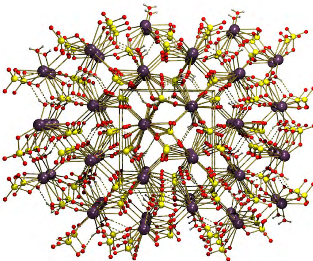
Figure 9: Vue en perspective de la structure montrant les liaisons hydrogène de type O-H...O
