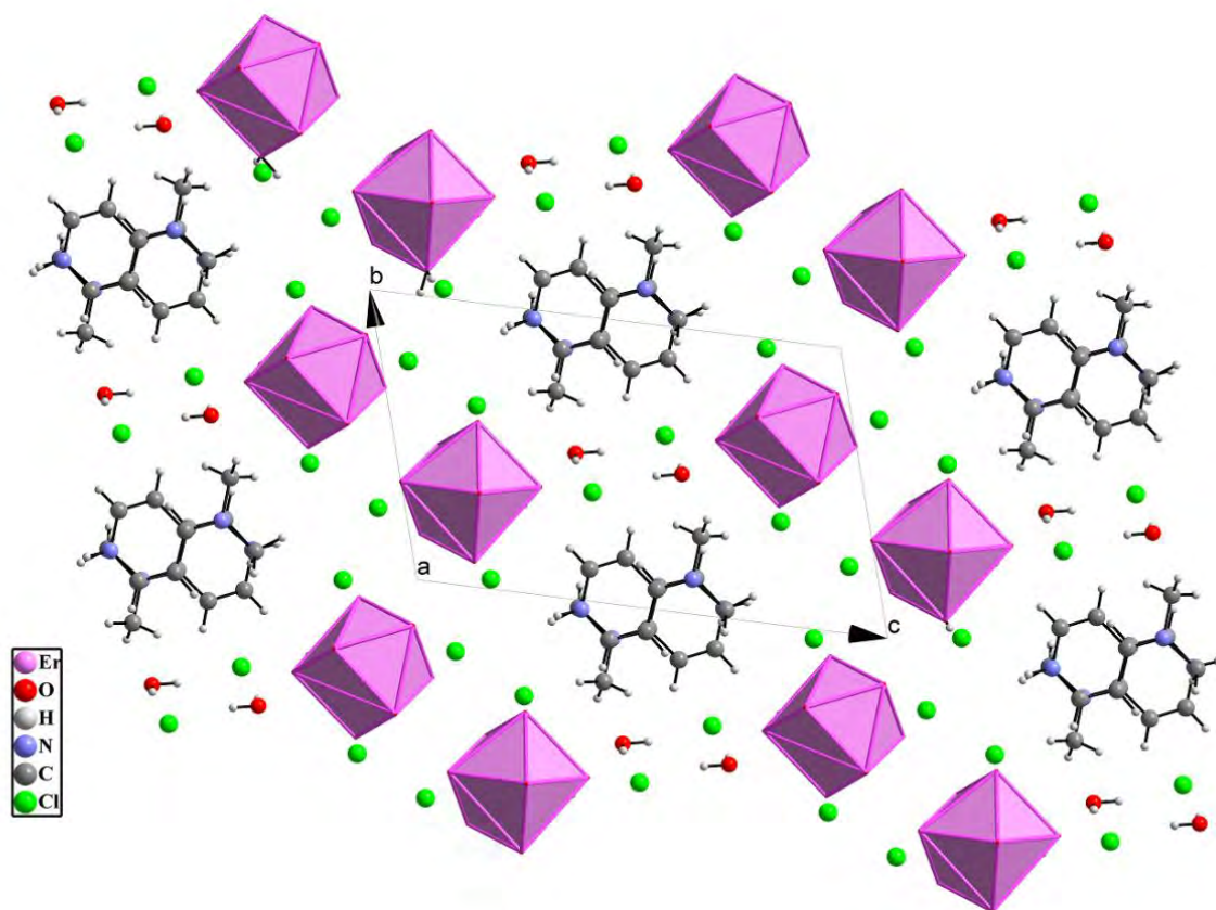
Figure 2 : Projection de la structure selon [100].
