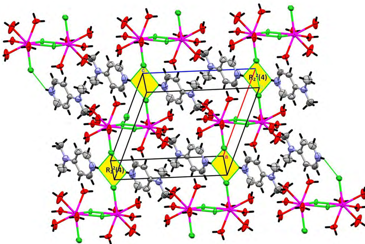
Figure 12: Liaisons hydrogène de type N-H...Cl selon le plan (a c)
