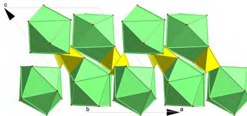
Figure 7 : Enchaînement de polyèdres \text{LaO}_9 et tétraèdres \text{SO}_4
