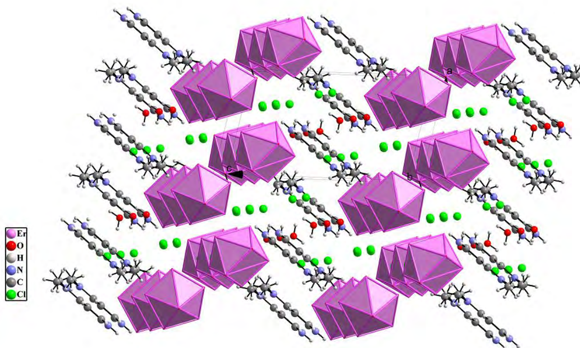
Figure 3 : Enchaînement de la structure selon le plan (a c).
