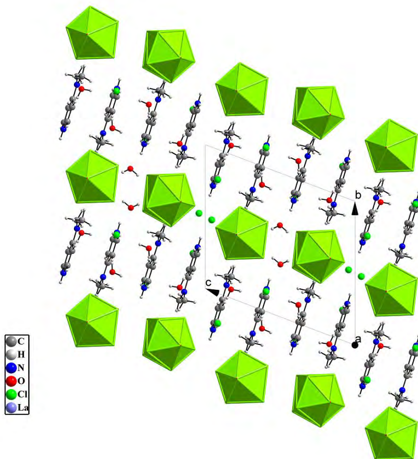
Figure 4 : Projection de la structure selon [100].
