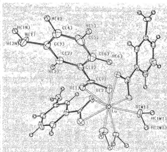
Figure 2b : La structure du composé [\text{Lu}(\text{C}_7\text{H}_6\text{NO}_2)_3(\text{H}_2\text{O})_3] \cdot 3\text{H}_2\text{O} [74]
