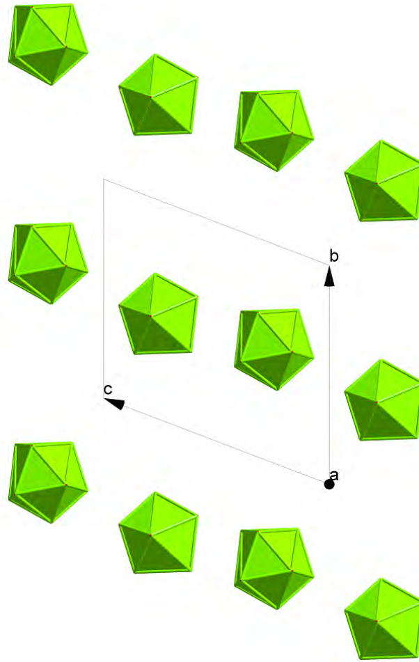
Figure 9: Enchaînement des polyèdres [\text{LaCl}(\text{H}_2\text{O})_8]^{2+} selon le plan (b c)
