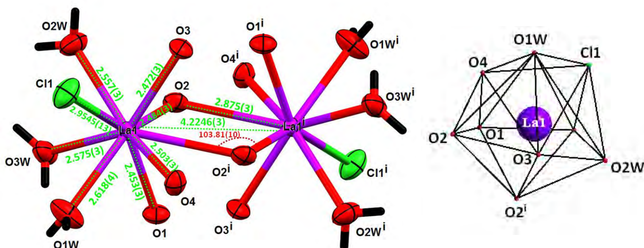
Figure 6 : Environnement de l'atome de lanthane [Code de symétrie: (i) -x+1, -y+1, -z+1 ]
