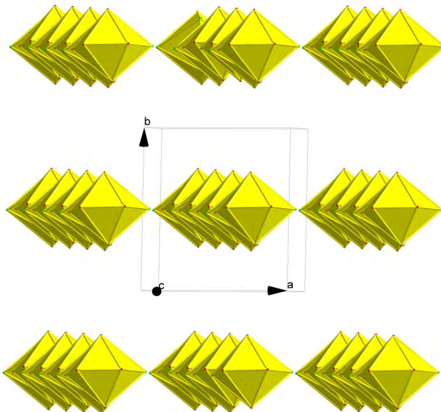
Figure 7: Enchaînement en couches du couple de polyèdres à arête commune [\text{Nd}_2\text{Cl}_4(\text{H}_2\text{O})_{10}]^{2+} selon le plan (a b)
