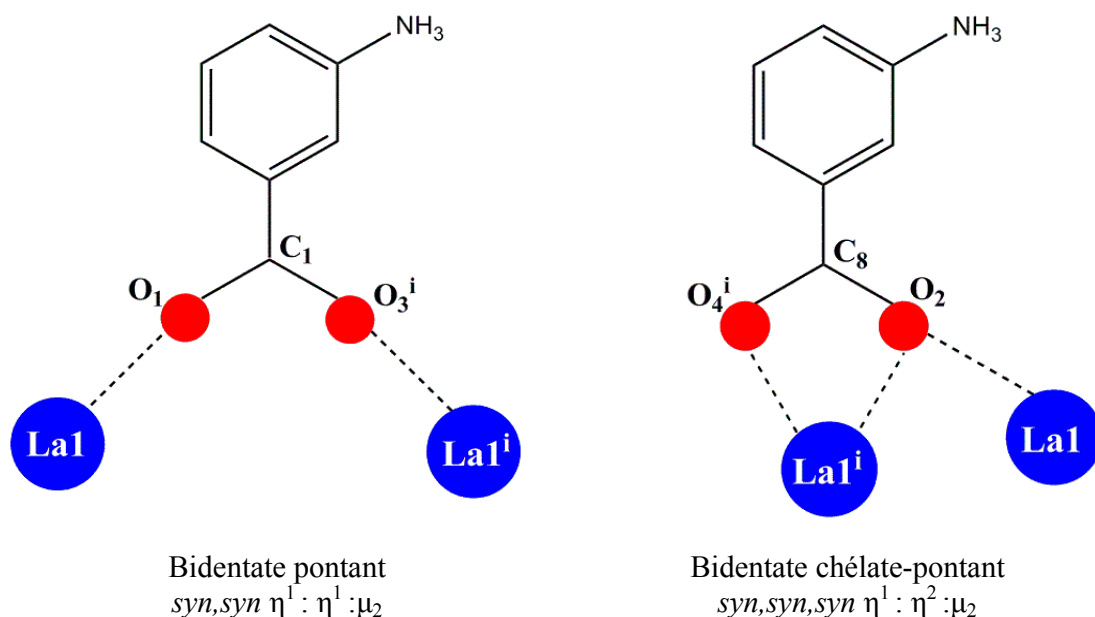
Figure 5: Modes de coordination des fonctions carboxylates du ligand MABA.
