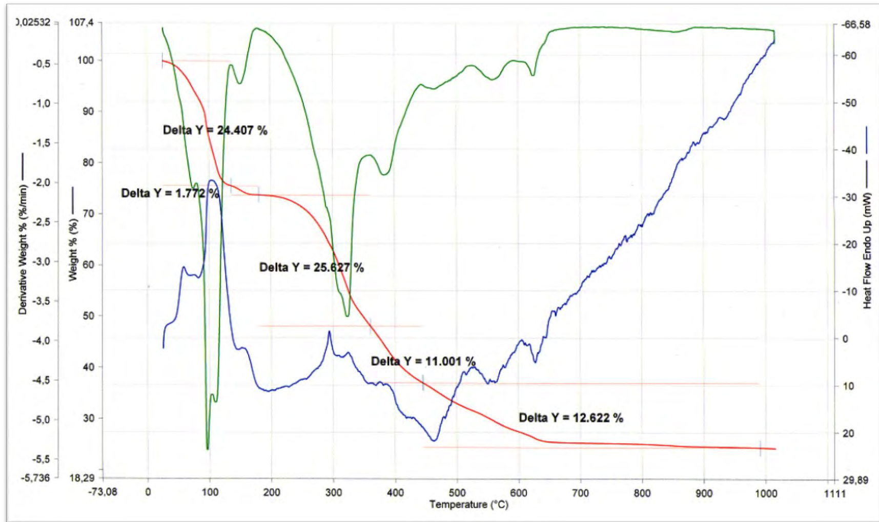
Figure 15: Analyse thermogravimétrique (ATG) et analyse thermique différentielle (ATD) du composé [\text{LaCl}(\text{H}_2\text{O})_8]^{2+}, 2(\text{C}_7\text{H}_{11}\text{N}_2)^+, 4\text{Cl}^-, 3\text{H}_2\text{O} sous \text{N}_2 avec une vitesse de chauffage de 10^\circ\text{C}\cdot\text{min}^{-1} .
