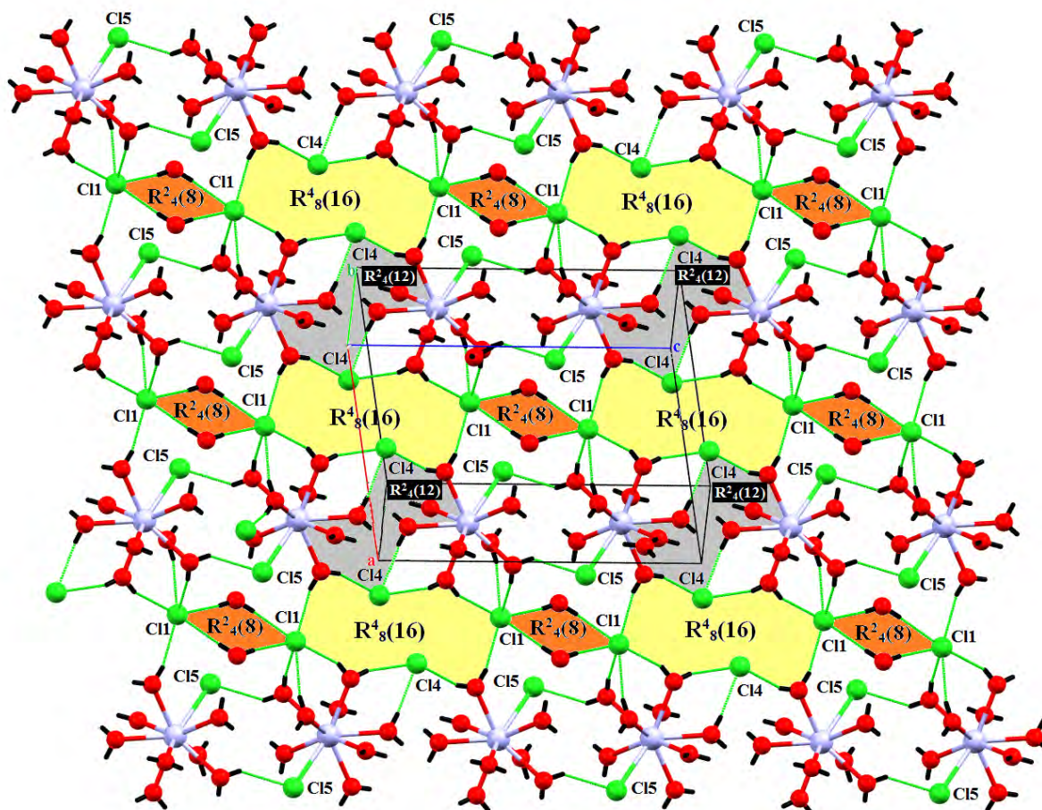
Figure 13b: Réseau des liaisons hydrogène de type O-H water ...Cl selon le plan (a c) en légère perspective. Les atomes du cation organique ne sont pas représentés.
