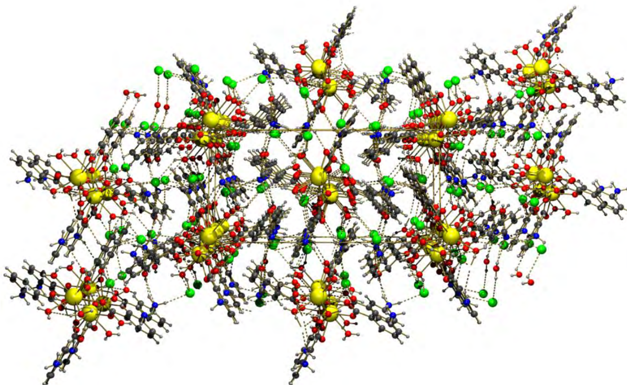
Figure 6: Liaisons hydrogène dans le composé [\text{Nd}_2(\text{C}_7\text{H}_7\text{NO}_2)_4(\text{H}_2\text{O})_8]\text{Cl}_6.4\text{H}_2\text{O}
