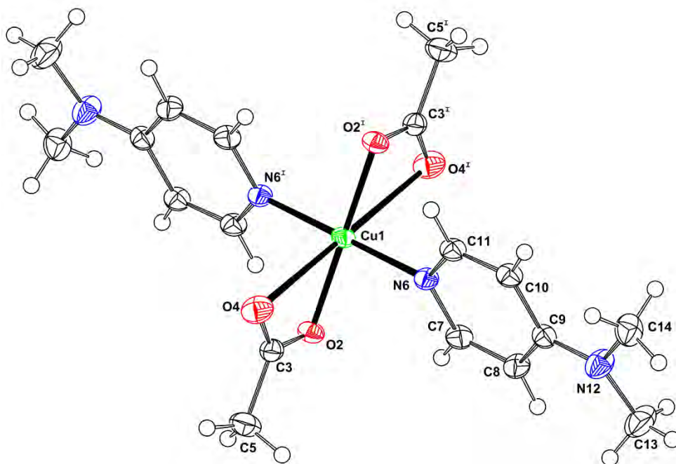
Figure 2 : La structure moléculaire du composé [\text{Cu}(\text{C}_2\text{H}_3\text{O}_2)_2(\text{C}_7\text{H}_{10}\text{N}_2)_2] (I) : -x, -y, -z .
