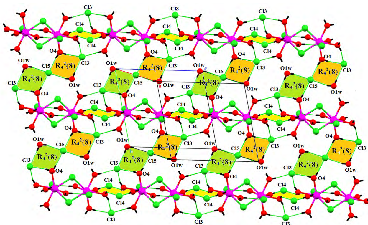
Figure 9: Liaisons hydrogène de type O-H water ...Cl
