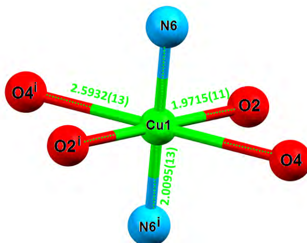
Figure 3 : Coordination octaédrique de l'atome de Cuivre [Code de symétrie (I): -x, -y, -z ]
