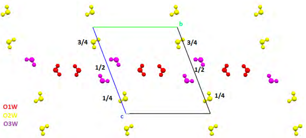
Figure 12: Enchaînement des molécules d'eau selon le plan (b c)
