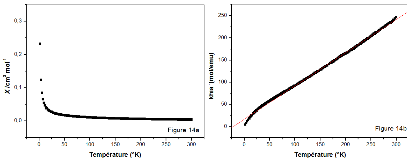
Figure 14a : Evolution de la susceptibilité magnétique en fonction de la température
