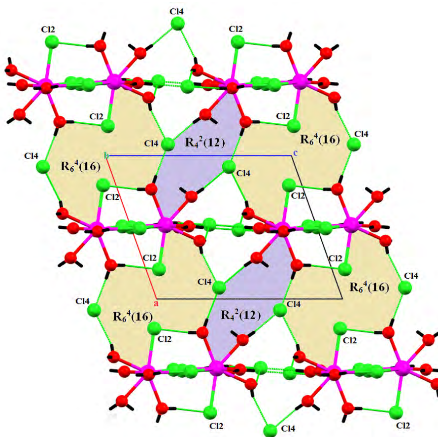
Figure 10: Liaisons hydrogène de type O-H water ...Cl selon le plan (a c)
