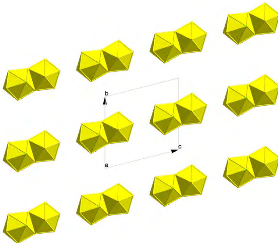
Figure 6: Enchaînement du [\text{Nd}_2\text{Cl}_4(\text{H}_2\text{O})_{10}]^{2+} selon le plan (b c)
