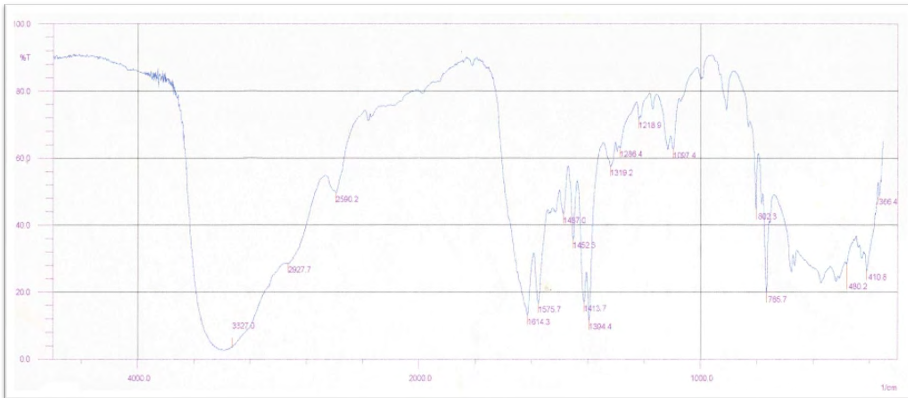
Figure 3 : Le spectre infra rouge du composé [\text{La}_2(\text{C}_7\text{H}_7\text{NO}_2)_4\text{Cl}_2(\text{H}_2\text{O})_6]\text{Cl}_4 \cdot 2\text{H}_2\text{O}
