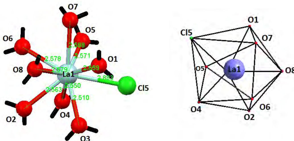
Figure 8: Schéma représentant l'environnement 9 de l'atome de lanthane
