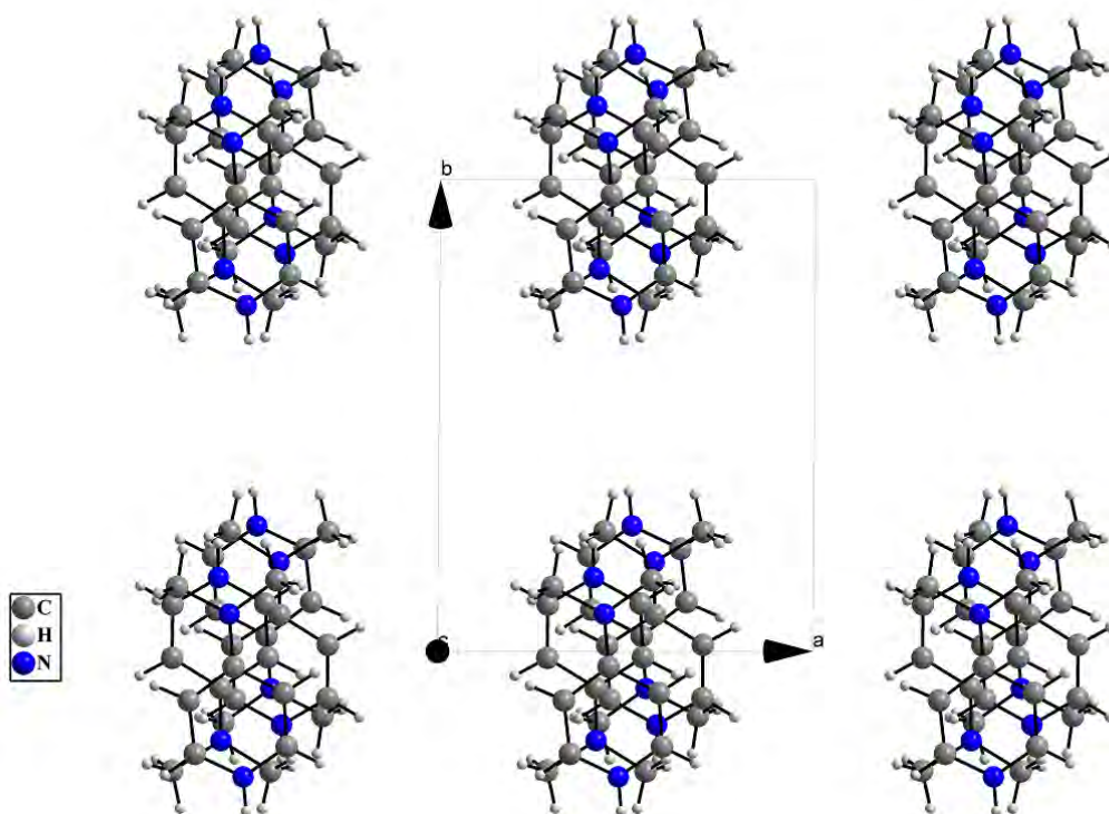
Figure 7: Enchaînement du 4-(diméthylamino)pyridinium selon [001].
