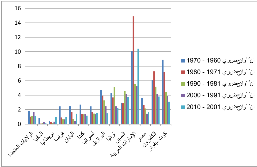
شكل 24: المنحنى البياني للنمو الحضري في العالم للفترة 1960 - 2010
