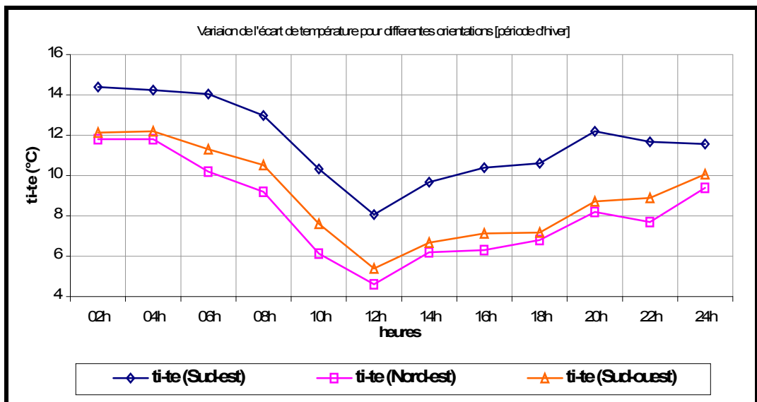
Figure 6-34 : Comparaison Des Ecart Entre Température Intérieure Et Extérieure [Période d’hiver] Constantine, 2004.
