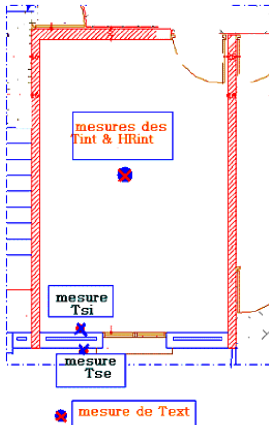
Figure 6-6 : Position des appareils de mesures au niveau du séjour
