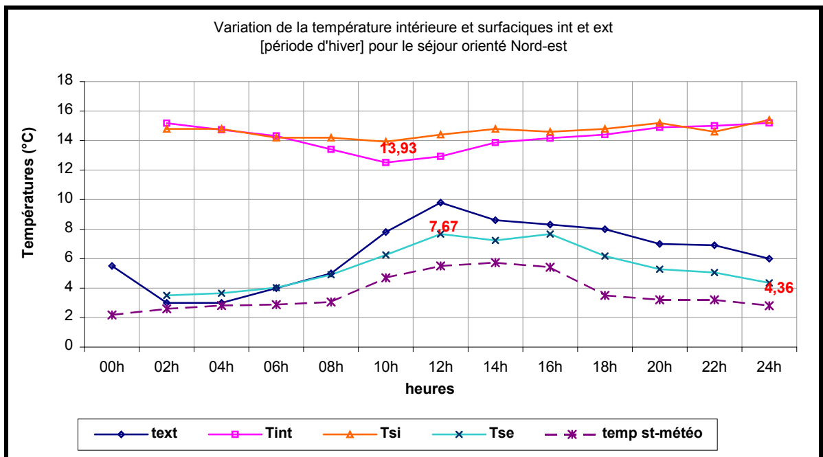
Figure 6-25 : Variation de la température intérieure et surfacique intérieure et extérieure pour le séjour orienté Nord-est. [Période d'hiver] Constantine, 2004.
