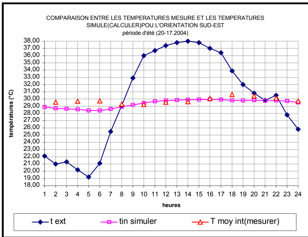
Figure 7- 3 : Comparaison des températures intérieures mesurée et simulée pour l'orientation Sud-est [période d'été] journée du 20-07-2004.
