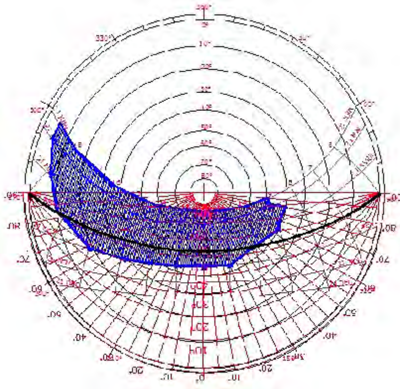
Figure 4-39 : Masque d'ombre de la protection solaire de la fenêtre sud. Source : Auteur.
