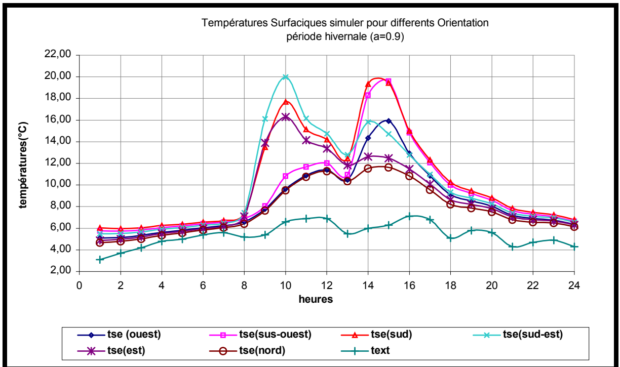
Figure 7-29 : Températures surfaciques des différentes orientations pour une couleur sombre (période d’hiver)
