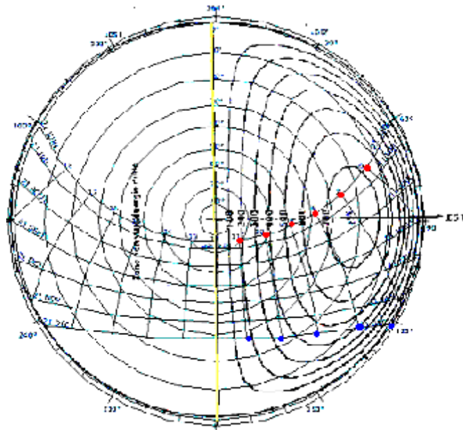
Figure 3-26 : Irradiation solaire sur une paroi verticale orienter Est' (azimut mur = -90°)
