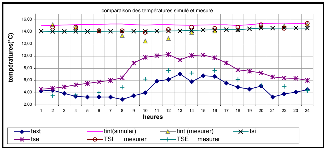
Figure 7-12 : Comparaison des températures surfaciques mesurées et simulées pour l'orientation Nord-est. [Période d'hiver] journée du 07-01-2005.
