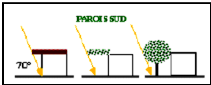
Figure 4-35 : Une paroi verticale SUD est facile à protéger: la moindre saillie d'un plan horizontal placé au-dessus de la paroi est suffisante. L'effet d'auvent est donc le plus adéquat pour ombrer une paroi SUD. Source : Groupe ABC, 1999.
