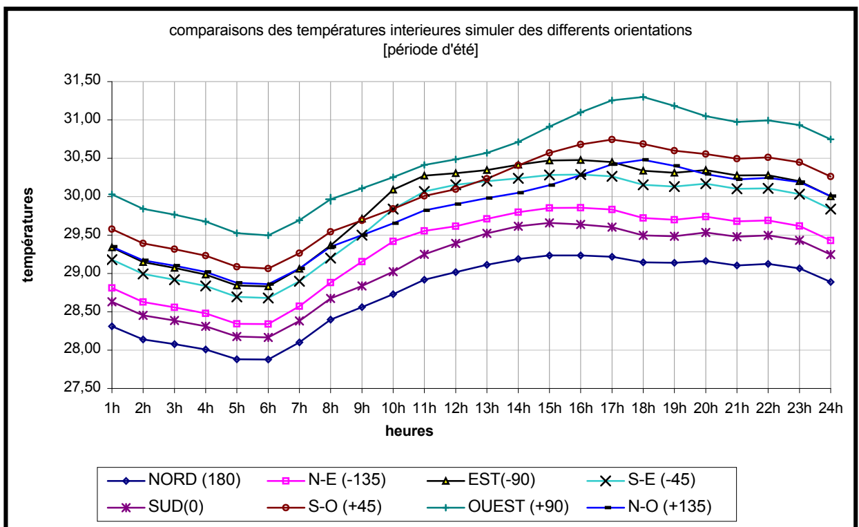
Figure 7-17 : Effet de l'orientation sur la température intérieure [période d'été]
