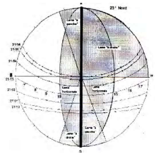
Figure 5-40 : La façade OUEST protégée par des éléments verticaux formant un angle 45^\circ avec le plan de la façade (ou il y a deux hauteurs pour les ouvertures) et le contrôle de la façade OUEST est total pour les mois les plus chauds. Palais de l'association des filateurs à Ahmedabad, par LE CORBUSIER. SOURCE : IZARD.J.L, 1993
