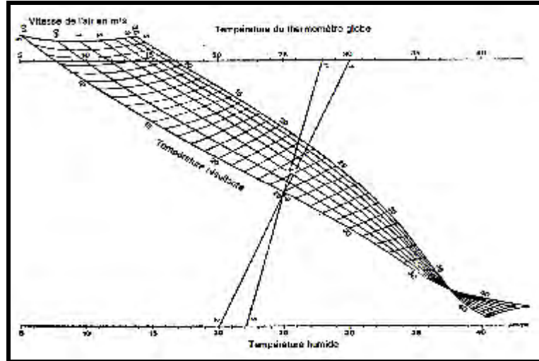
Figure 2-13 : Abaque pour la détermination de la température résultante (d’après le Ashve Guide). Source : GIVONI. B, 1978
