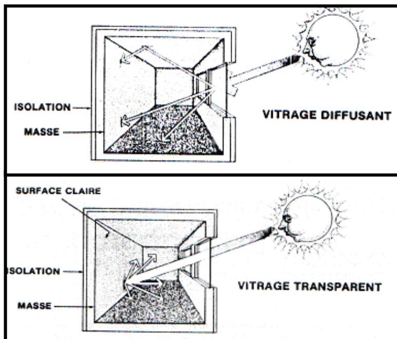
Figure 4- 3 : Apport solaire suivant la nature du vitrage, et stockage dans l'inertie des murs intérieurs. Source : MAZRIA. Ed,
