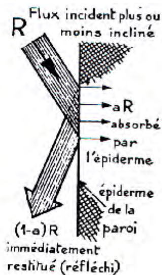
Figure 4- 4: Flux énergétique incident sur une paroi opaque.
