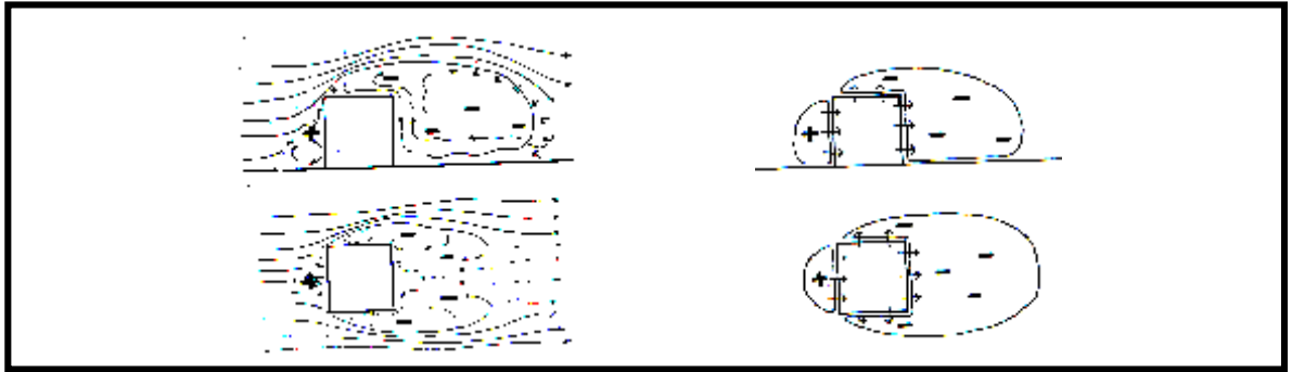
Figure 4-46: Effet du vent sur les éléments du bâtiment. Source. MARTIN EVANS, 1980.
