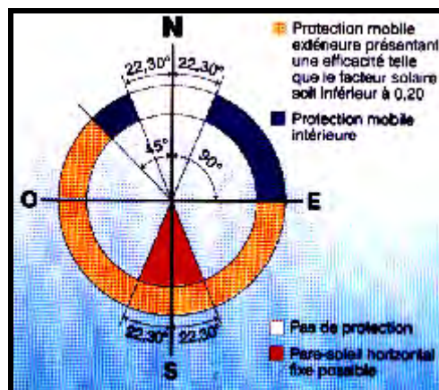
Figure 4-45 : Protections solaires fixes ou mobiles.
