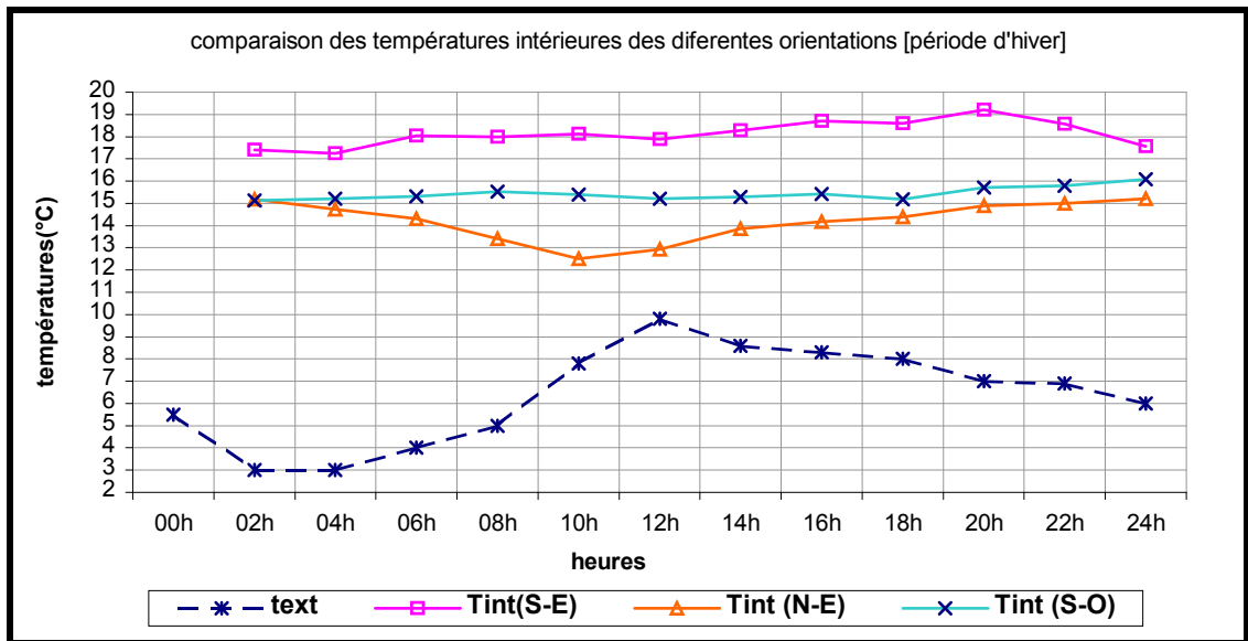
Figure 6-32 : Comparaison des températures intérieures des trois séjours [période d'hiver] Constantine, 2004.
