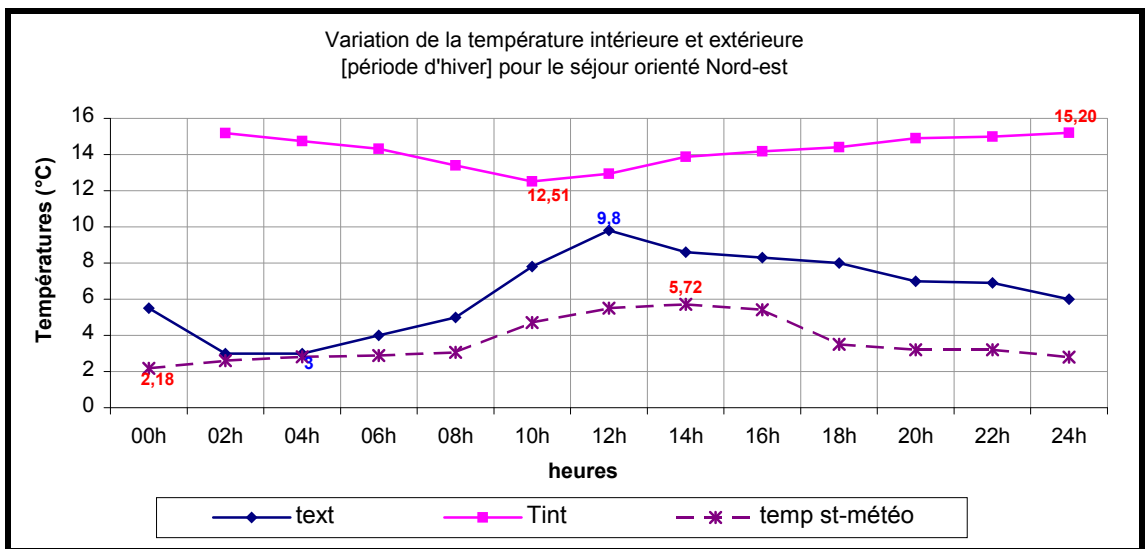
Figure 6-23 : Variation de la température intérieure et extérieure pour le séjour orienté Nord-est. [Période d'hiver] Constantine, 2004.
