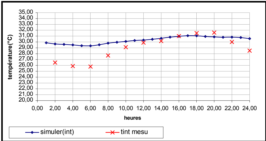
Figure 7-7: Comparaison des températures intérieures mesurée et simulée pour l'orientation Sud-ouest. [Période d'été] journée du 20-07-2004.
