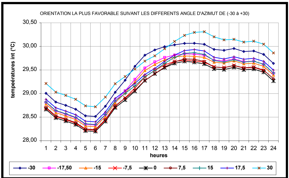
Figure 7-19 : Effet du changement de l'angle d'azimut (pour les orientations proche au Sud) sur la température intérieure
