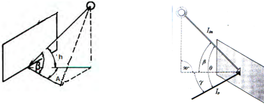
Figure 3-22 : Angle d'incidence pour une surface verticale. Source : S.V.SZOCLAY, 1978
