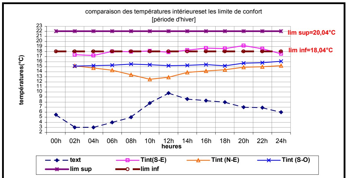
Figure 6-36 : Comparaison des températures intérieures des trois séjours et les limites sup. et inf. de confort. [Période d'hiver] Constantine 2004.
