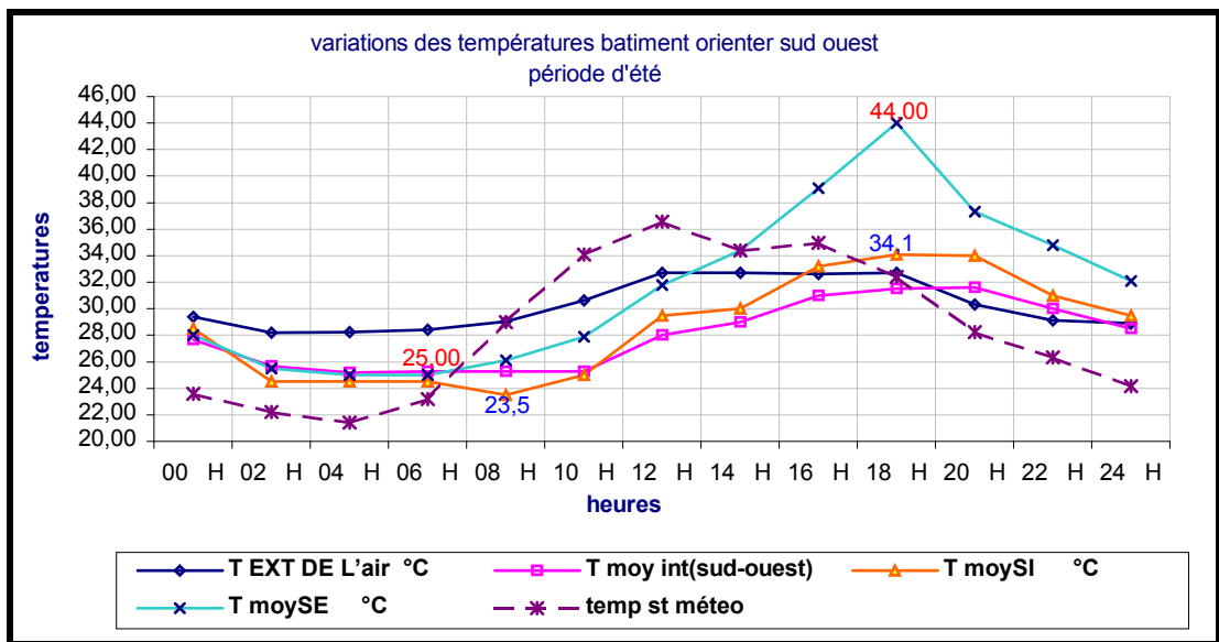
Figure 6-18 : Variation de la température surfacique interne et externe pou l'orientation Sud-ouest. Constantine, 2004 [période d'été].
