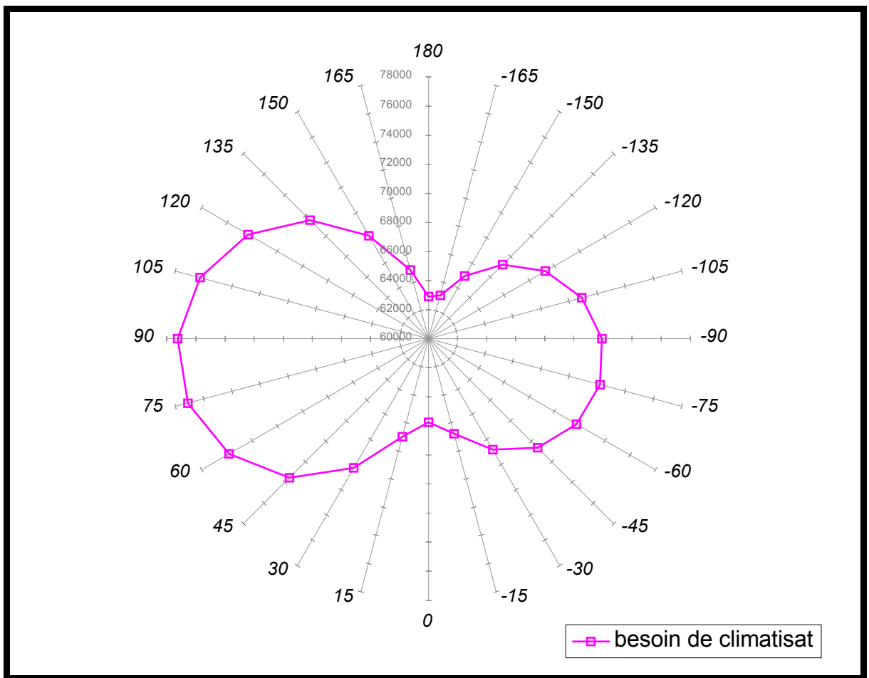
Figure 7-24 : Le besoin de climatisation suivant l'orientation (en kJ).
