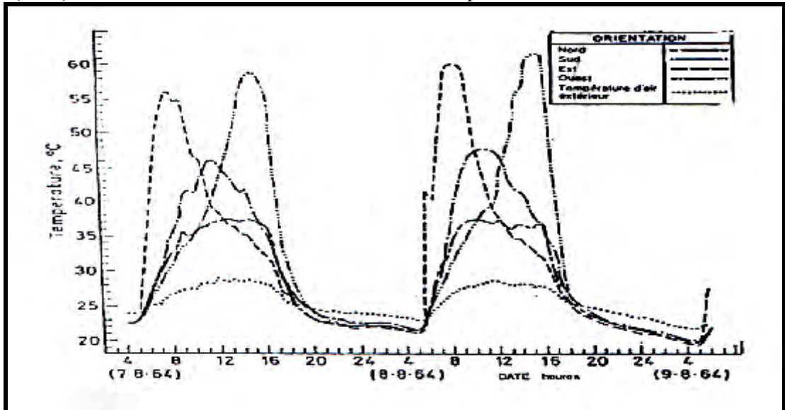
Figure 5-13 : Températures de surfaces externes de murs gris de différentes orientations.
