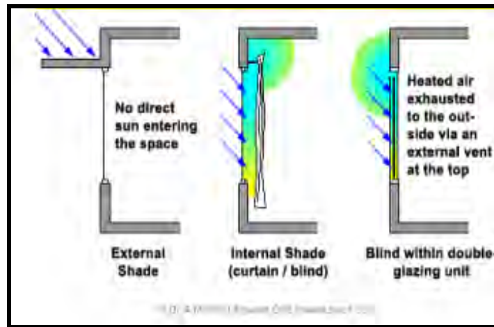
Figure 4- 23: L’impact de la position d’un brise-soleil Par rapport au vitrage sur le flux de chaleur interne. Source : MARSH. A ( www.squ1.com )
