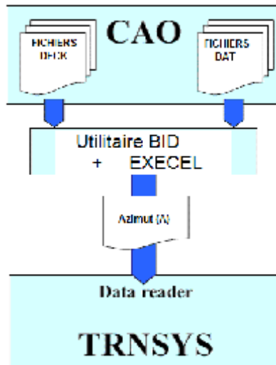
Figure 7-2: Schéma de déroulement de la simulation.
