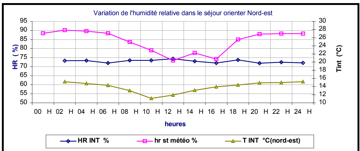
Figure 6-24 : Variation de l'humidité relative dans le séjour Nord-est. [Période d'hiver] Constantine, 2004.
