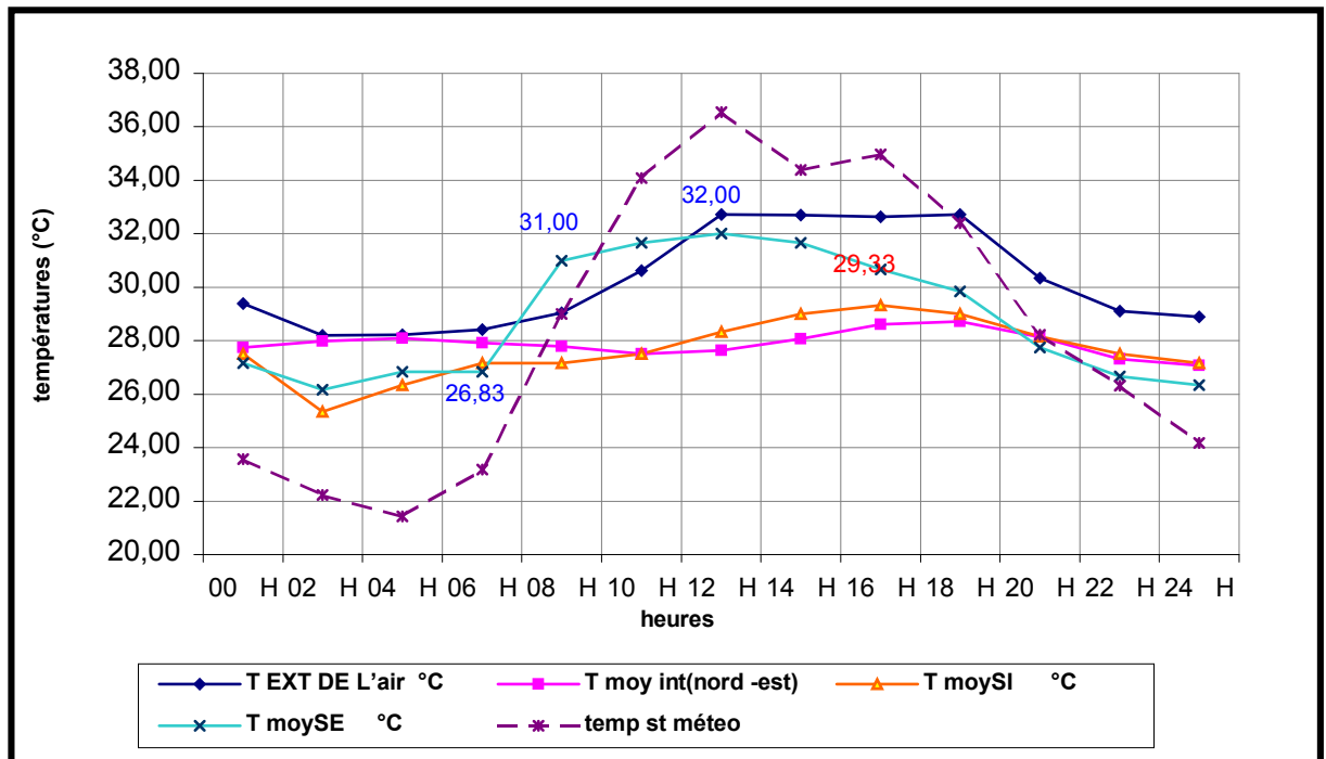
Figure 6-13 : Variation des températures surfaciques internes et externes, pour l'orientation Sud-est. Constantine, période d'été.
