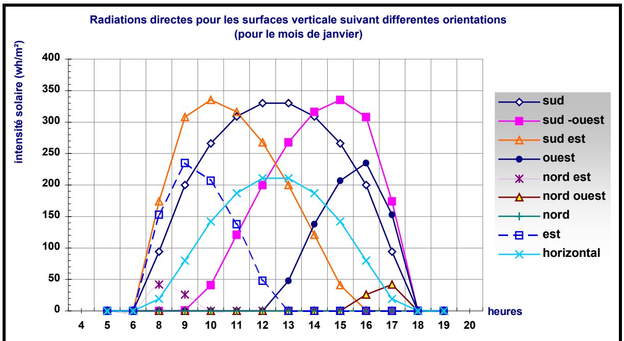
Figure 3-33 : radiations directes pour une surface verticale pour différentes orientations durant un mois froid de l'année -JANVIER- pour la ville de constantine. Source : CAPDEROU.1988.
