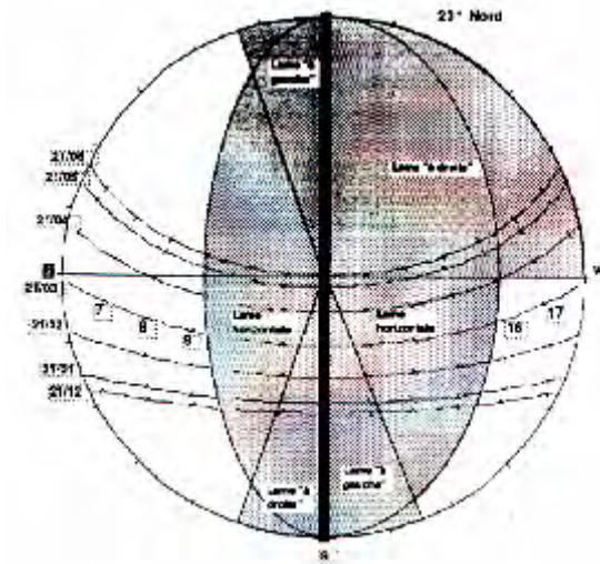
Figure 5-39 : Le contrôle solaire par des brises solaires en façade EST(a gauche) et OUEST(a droite), SOURCE : IZARD.J.L, 1993.
