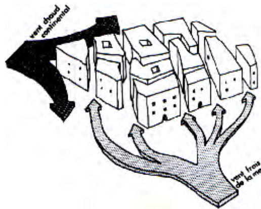
Figure 5-27: Organisation et Orientations des rues pour canaliser l'air frais.
