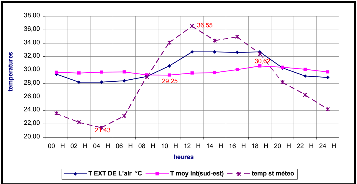
Figure 6-14 : Variation de la température intérieure et extérieure, orientation Sud-est. Constantine période d'été.
