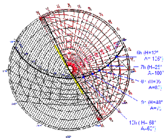
Figure 5-24 : Masque d'ombre de la protection solaire de la fenêtre du séjour NORD-EST.
