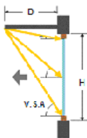
Figure 4-25 : Protection horizontale pour une orientation sud.
