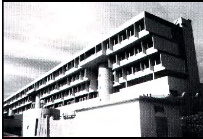
Figure 5-41 : Exemple d'effet d'auvent ; les étages en encorbellement de la cité des étudiants de l'université de Constantine, par KENZO TANGE
