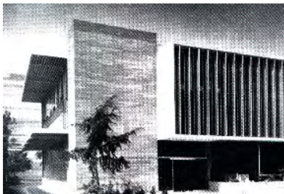
Figure 5-37 : Le traitement de la façade SUD à gauche et de la façade EST de face illustrent la maîtrise du contrôle de l'ensoleillement dans un climat chaud et ensoleillé en été, exemple de l'immeuble de la société mutuelle d'assurance incendie du Nord-ouest de Los Angeles, Californie, par RICHARD NEUTRA. Source : IZARD.J.L, 1993
