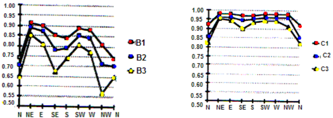
Figure 4-32 : Variation de Ft avec l'orientation pour un flanc. Source : IZARD.J.L 1993 P.37
