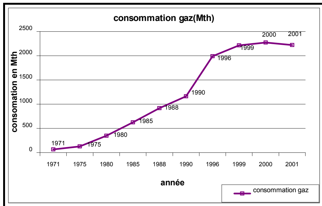
Figure 1-6 : Consommation gazière de la ville de Constantine (en Mth).
