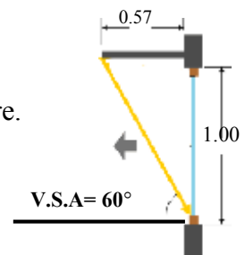
Figure 4-40 : Profondeur requise de l'auvent pour l'orientation sud.
