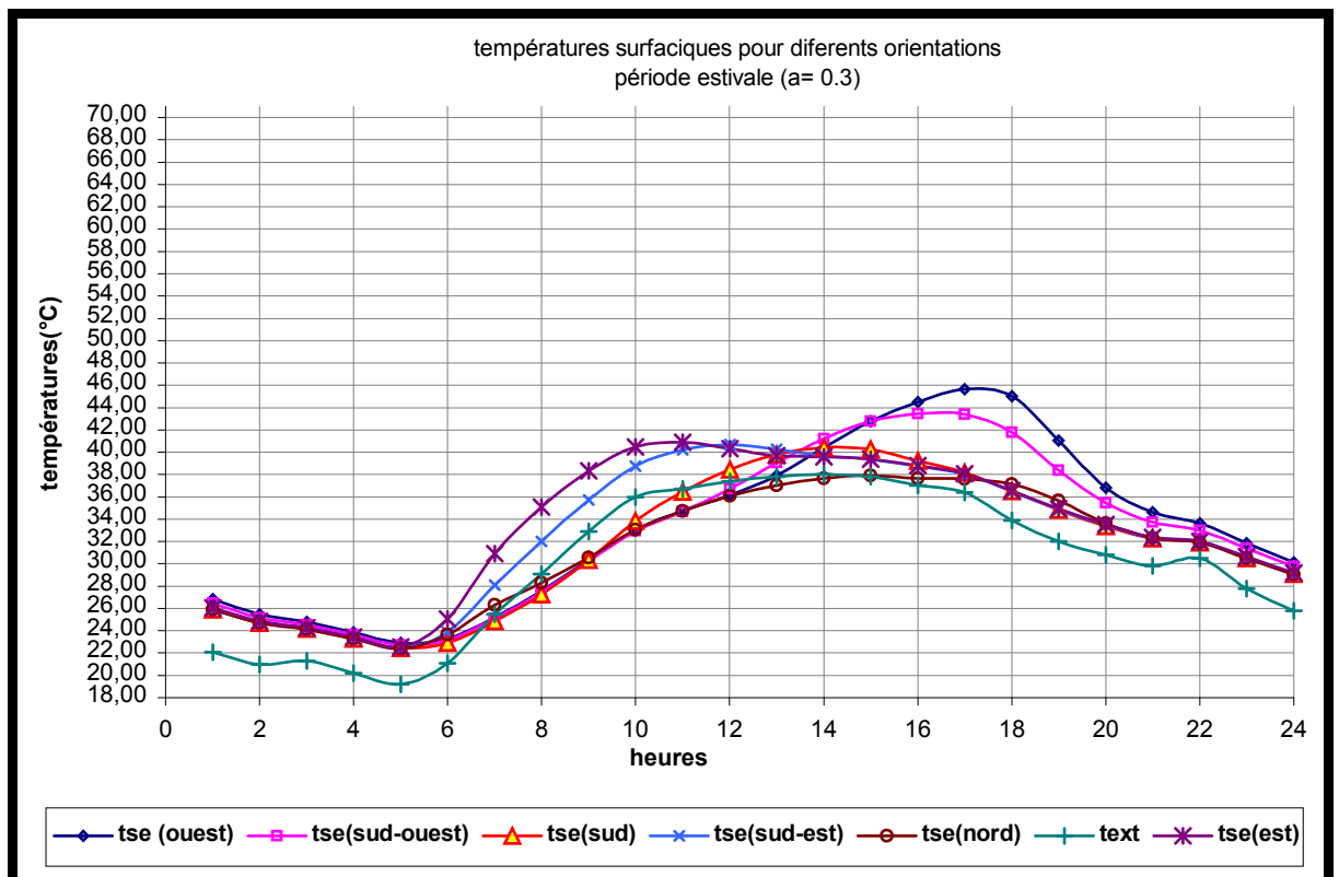
Figure 7-27 : Températures surfaciques des différentes orientations pour une couleur claires(période d'été)
