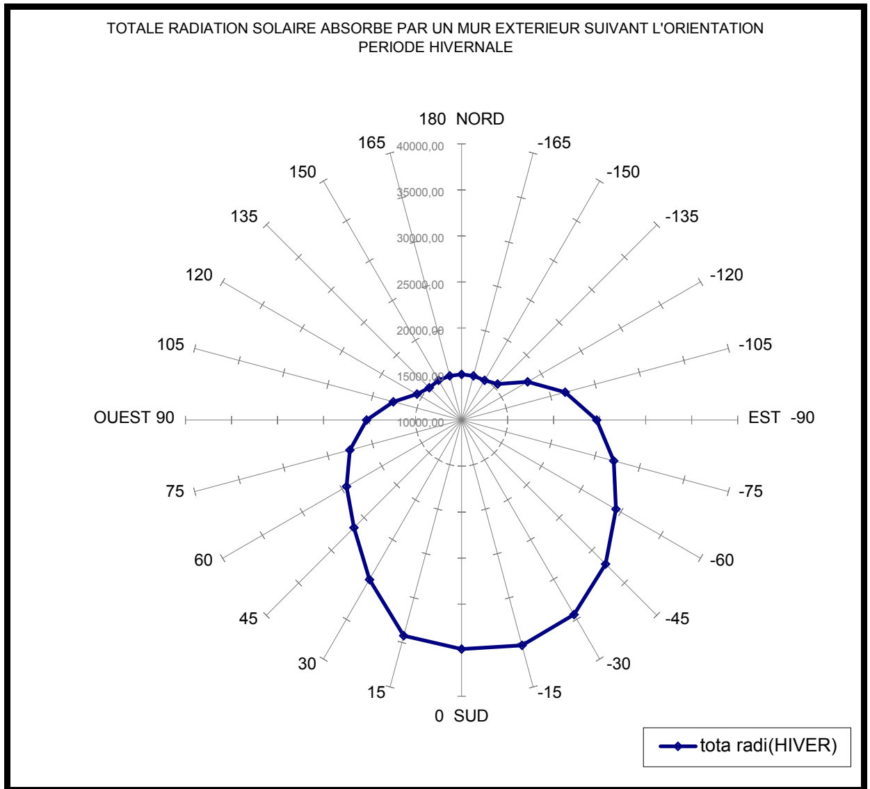
Figure 7-22 : Totale de radiation solaires absorbé par la paroi extérieure en (kJ/m 2 .h) suivant l'orientation. Période hivernale.
