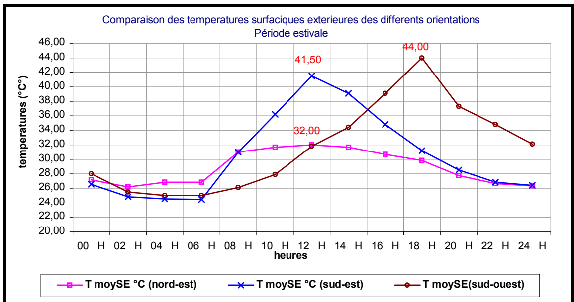
Figure 6-20 : Comparaison des températures surfaciques extérieures des trois orientations [période estivale].
