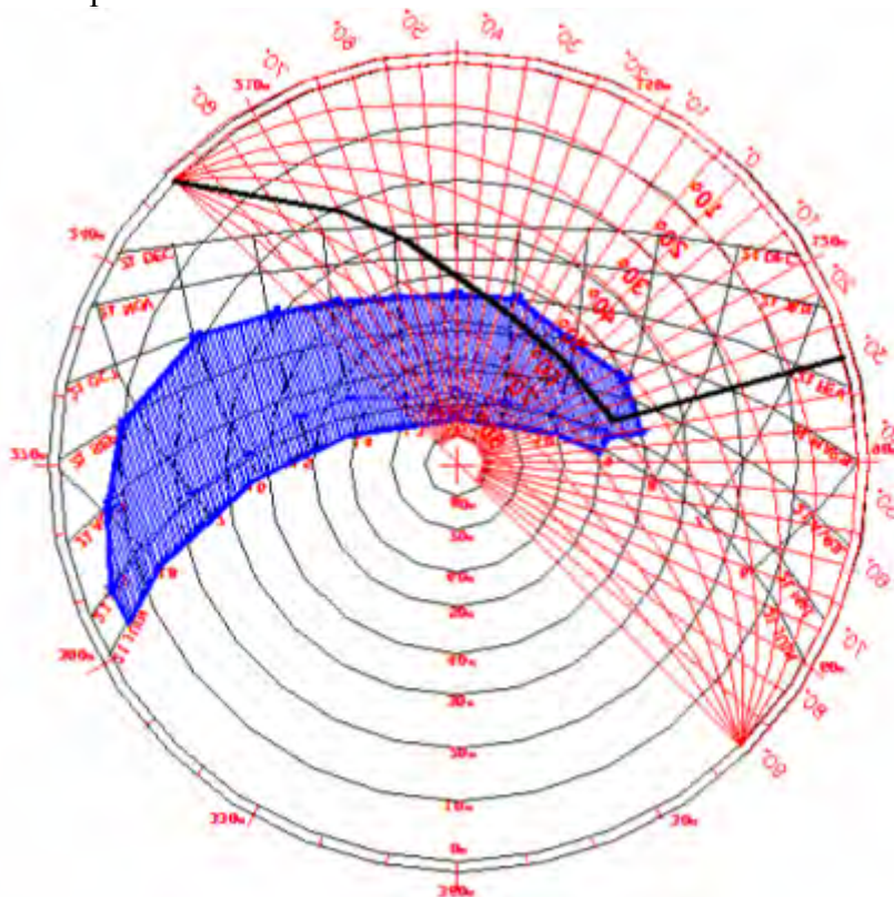
Figure 4-41 : Masque d'ombre de la protection solaire de la fenêtre Sud-est. Source : Auteur.
