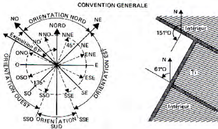
Figure 5- 3 : Convention générale d'orientation. Source : CSTB, 1986
