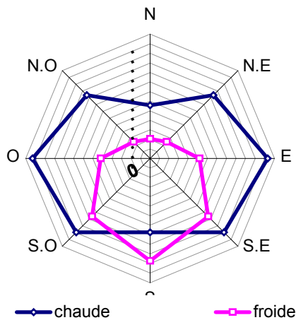
Figure 5-11 : Radiations solaires à la latitude 36°17 (pour une période de surchauffe et une deuxième de sous chauffe). Sources : CAPDEROU. M, 1988
