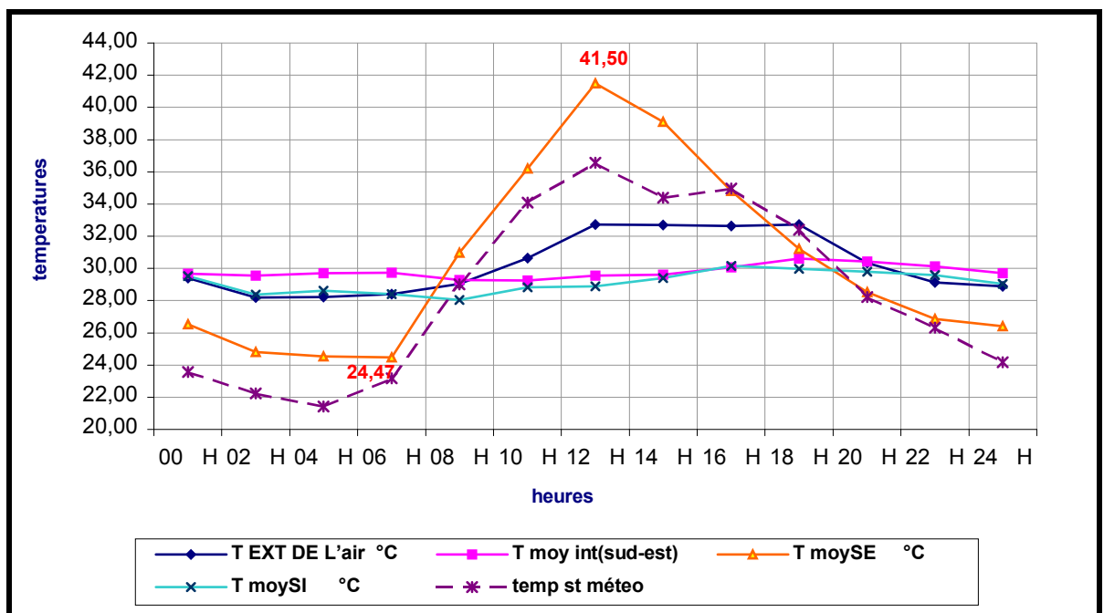
Figure 6-16 : Variation de la température intérieure et des températures surfaciques interne et externe pour le séjour orienté Sud-est. Constantine, 2004 [période estivale]
