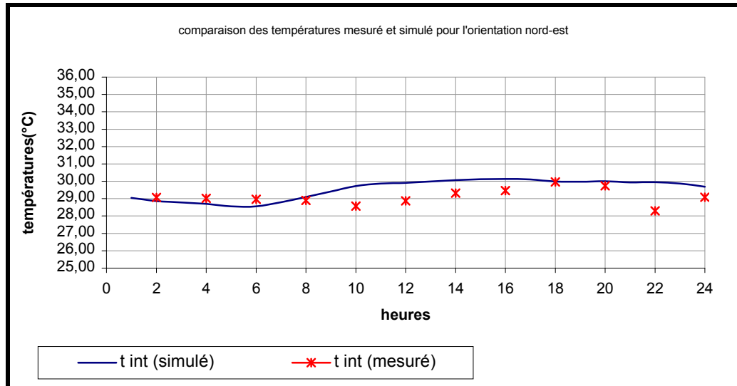
Figure 7-5 : Comparaison des températures intérieures mesurée et simulée pour l'orientation Nord-est. [période d'été] journée du 20-07-2004
