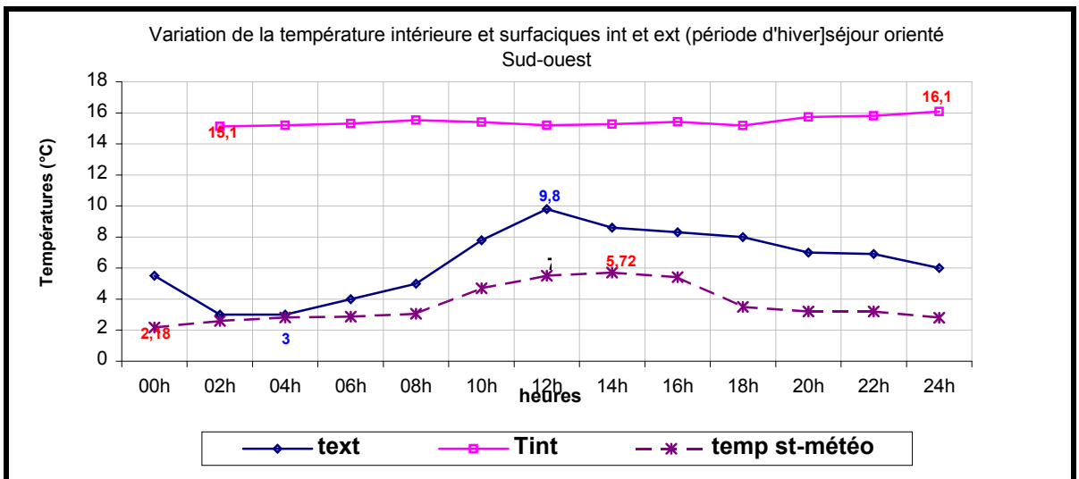
Figure 6-29 : Variation de la température intérieure et surfaciques intérieure et extérieure pour le séjour orienté Sud-ouest. [Période d’hiver] Constantine, 2004.
