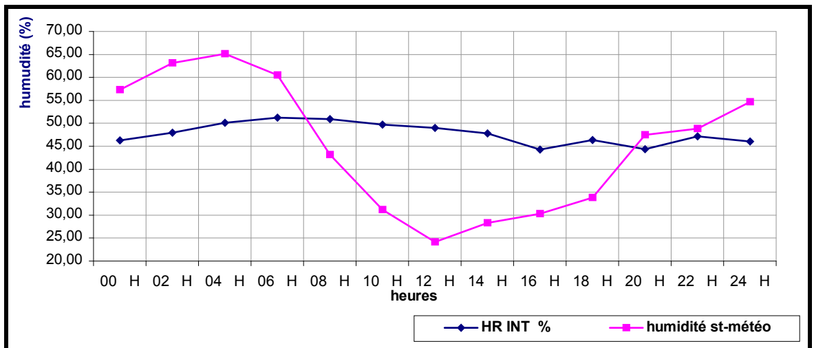
Figure 6-11 : Variation de l'humidité relative dans le séjour orienté Nord-est. Constantine période d'été.
