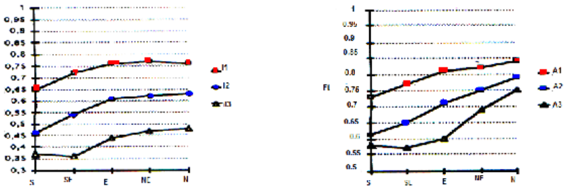
Figure 4-28 : Variation de facteur de transmission avec l’orientation pour un auvent. Source : IZARD.J.L (1993) p.33
