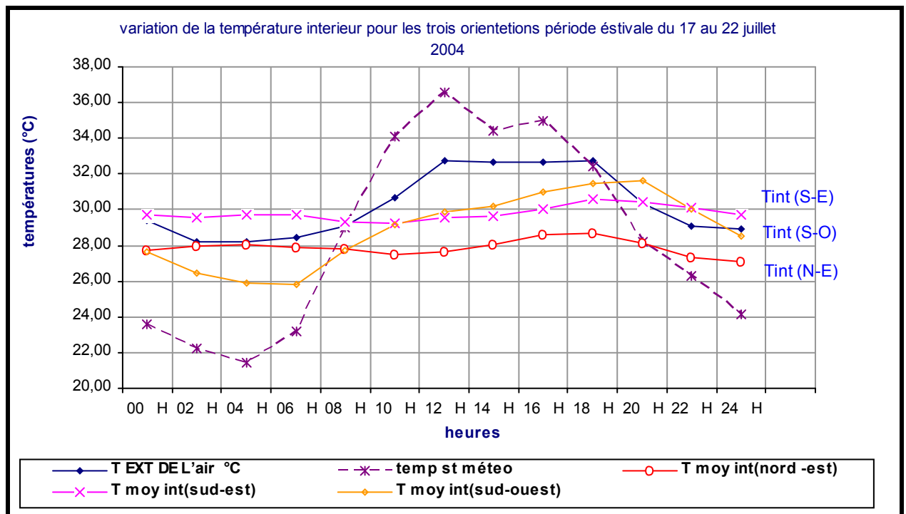
Figure 6-19 : Comparaison de la variation de la température intérieure pour les trois orientations [période estivale]. Constantine, 2004.
