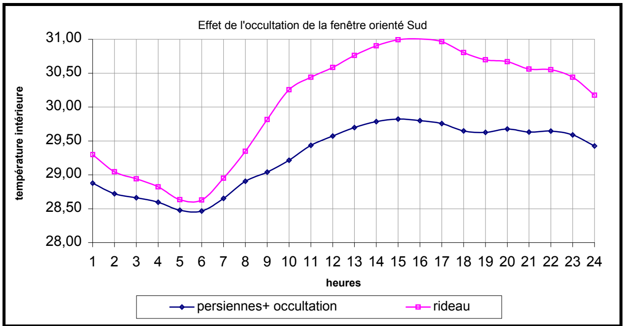
Figure 7-33 : Effet de la protection de l'ouverture.
