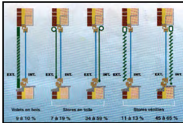
Figure 4-24 : Facteurs solaires de différentes protections solaires pour un vitrage simple. Source : ALAIN LIEBARD & ANDRE DE HERDE, 2003.
