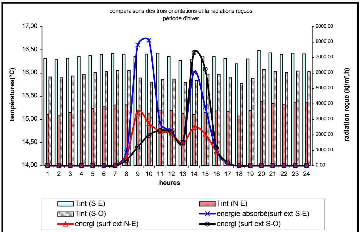
Figure 7-16 : Comparaisons des températures intérieures des trois orientations et la radiation reçue par la face externe ce la paroi (période d'hiver)
