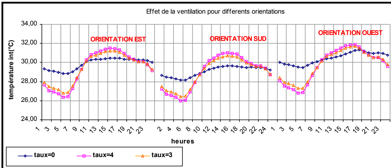
Figure 7-37 : Effet de la ventilation sur l'abaissement de la température intérieure pour les trois orientations cardinales (période d'été)
