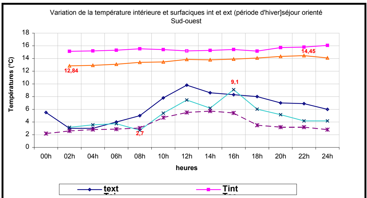
Figure 6-31 : Variation de la température intérieure et de surfaces int. et ext. pour le séjour orienté Sud-ouest. [Période d'hiver] Constantine, 2004.
