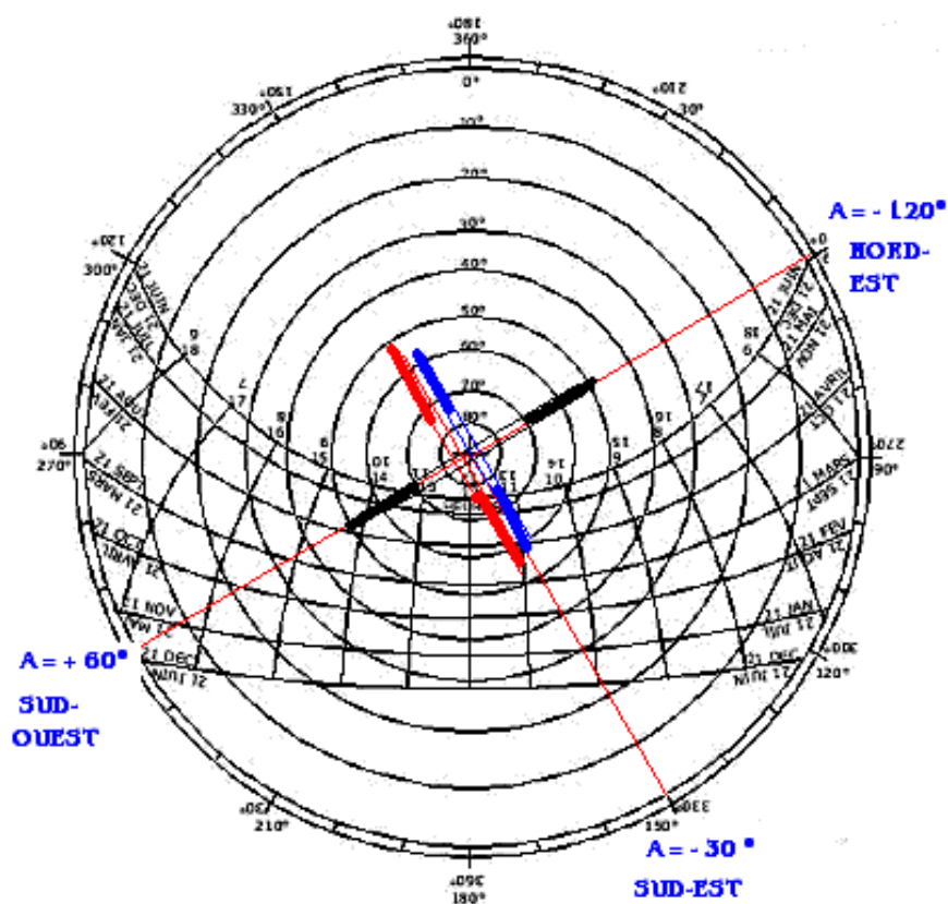
Figure 6-2 : Orientations des trois parois extérieures des séjours dans lesquelles se déroulent les mesures.
