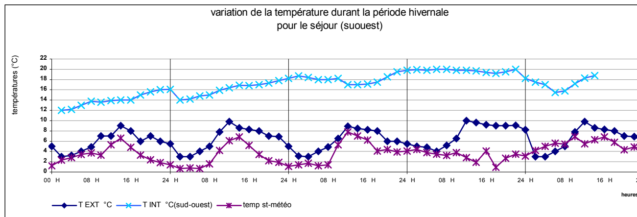
Figure A-11 : variation de la température intérieure durant la période (17/07 à 22/07/2004) séjour orienté à 60 azimuth ouest.(périod
