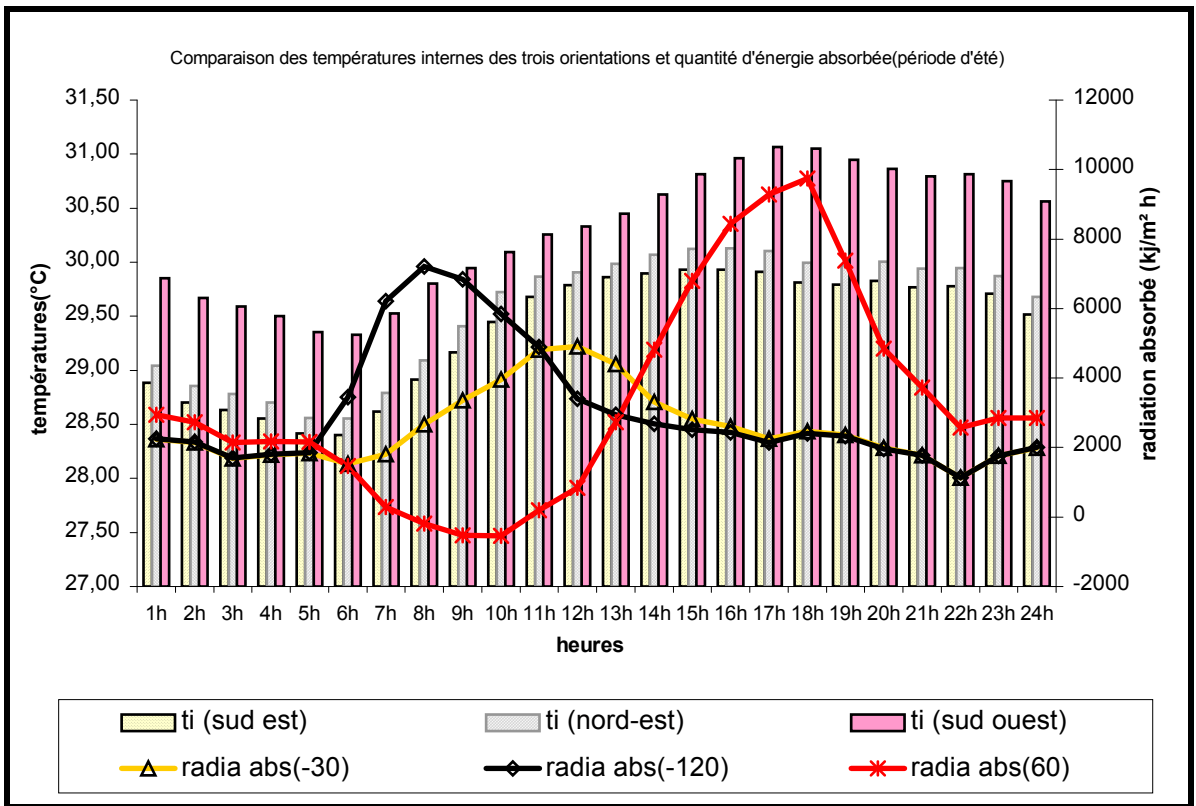
Figure 7-15 : Comparaisons des températures intérieures des trois orientations et quantité d'énergie absorbée par la paroi externe [période d'été].
