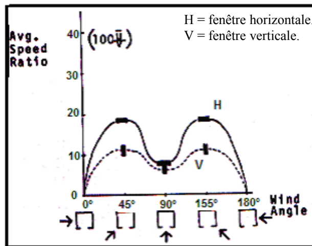
Figure 6-18 : Effet de la direction du vent sur la distribution de l'air à l'intérieur des chambres. Source : HARRIS J. SOBIN, 1981
