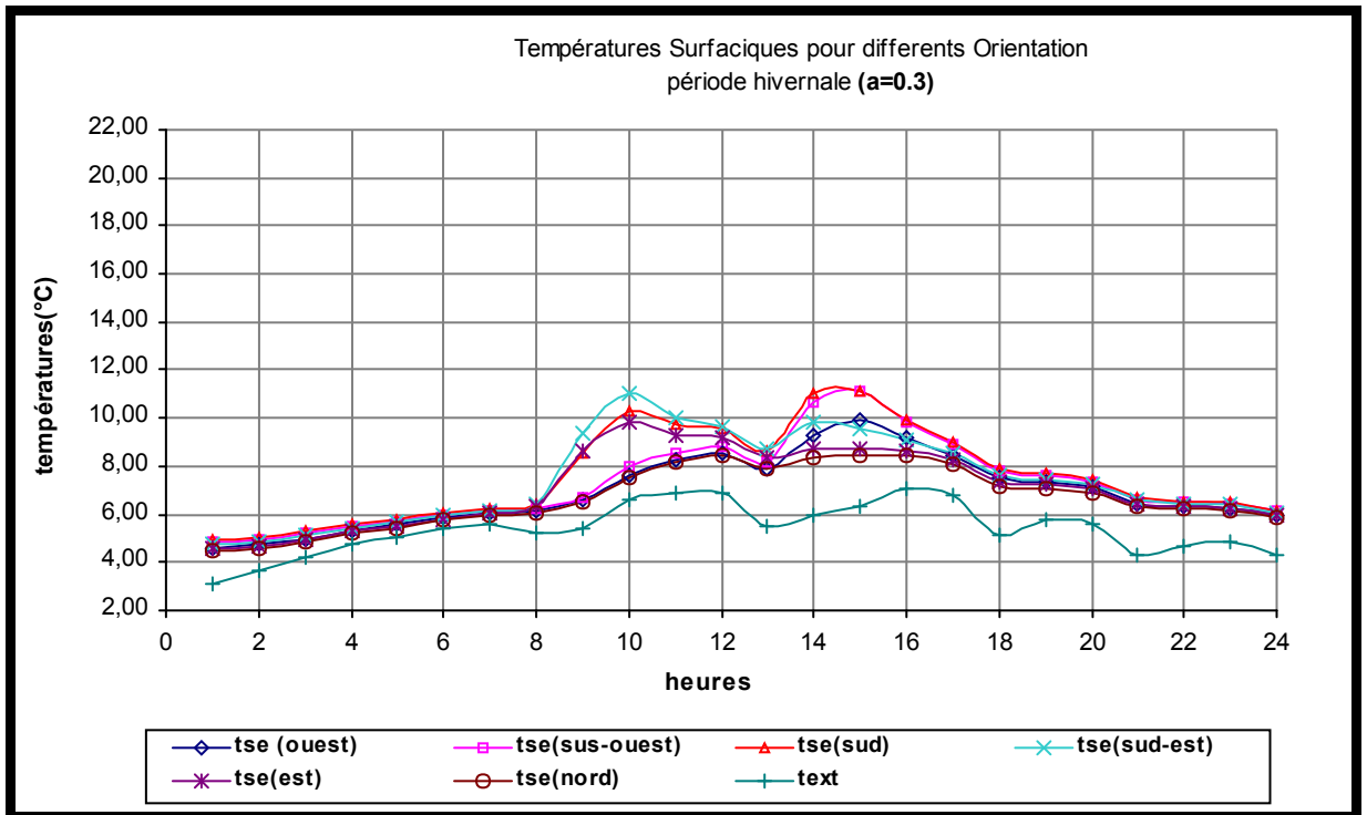
Figure 7-30 : Températures superficielles des différentes orientations pour une couleur claire (période d'hiver)
