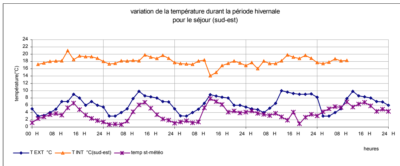
Figure A-10 : variation de la température intérieure durant la période (17/07 à 22/07/2004) séjour orienté à 30 azimuth est.(période d'hiver)
