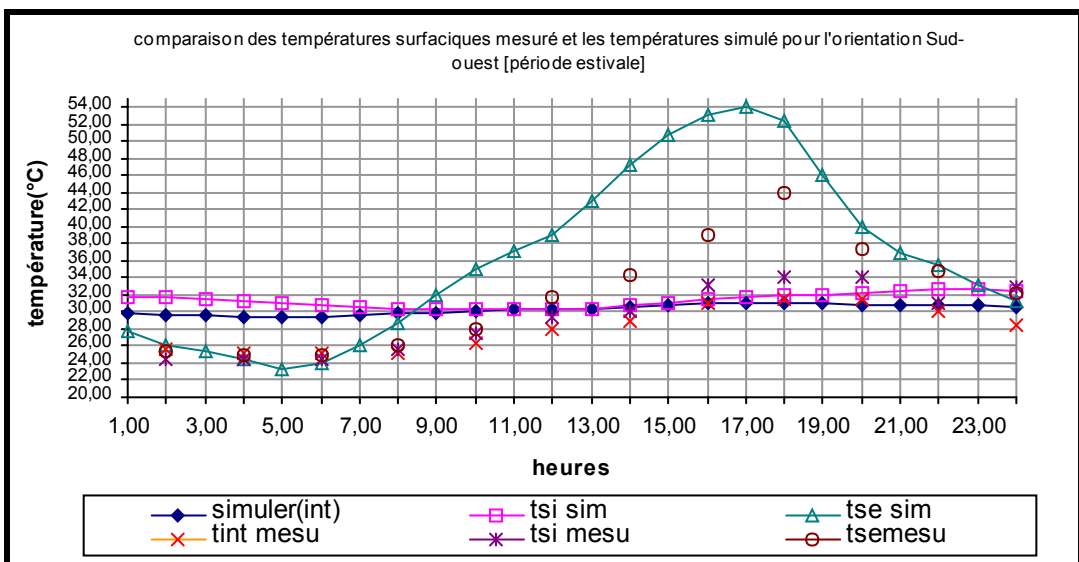
Figure 7-8 : Comparaison des températures surfaciques mesurée et simulée pour l'orientation Sud-ouest. [Période d'été] journée du 20-07-2004.
