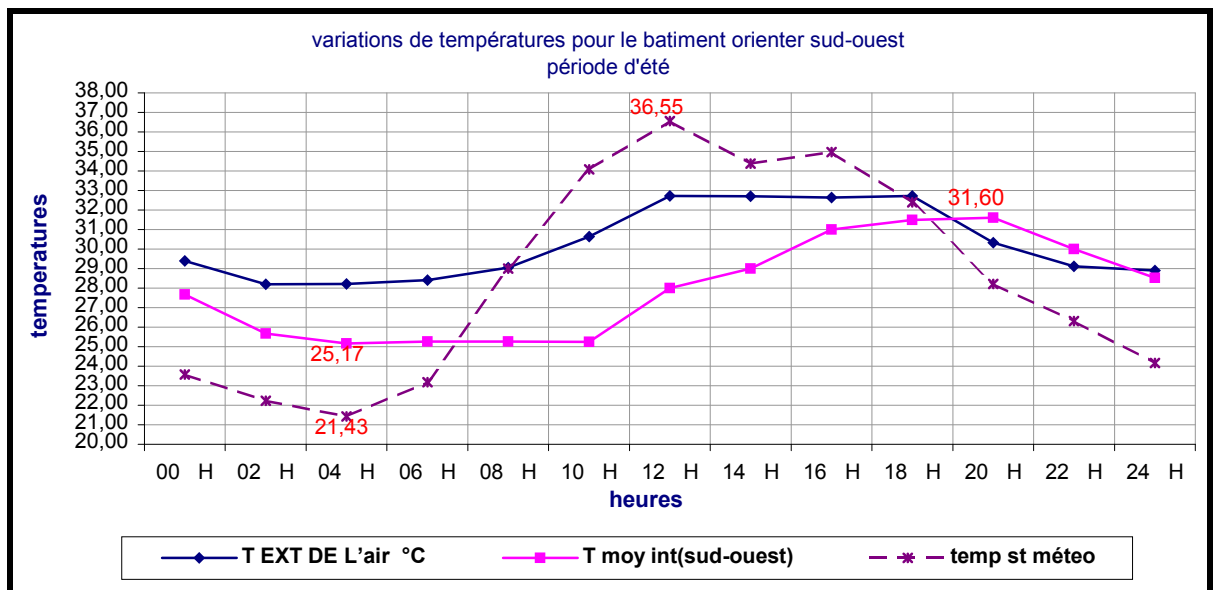
Figure 6-17 : Variation de la température intérieure et extérieure pour le séjour orienté Sud-ouest. Constantine, 2004 [période d'été].
