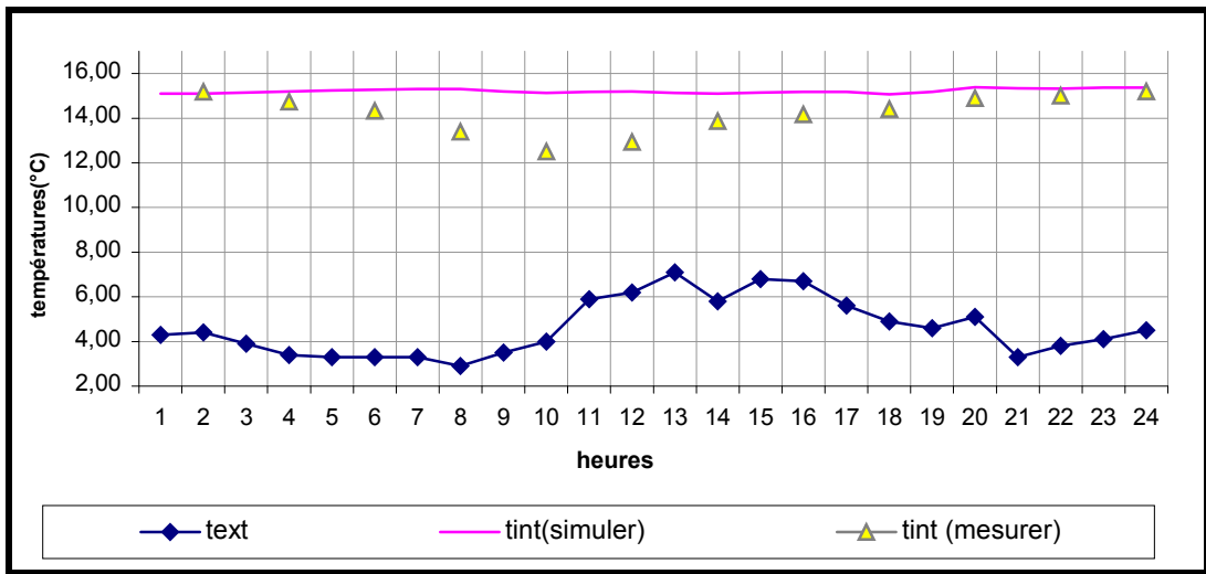
Figure 7-11 : Comparaison des températures intérieures mesurées et simulées pour l'orientation Nord-est. [Période d'hiver] journée du 07-01-2005.
