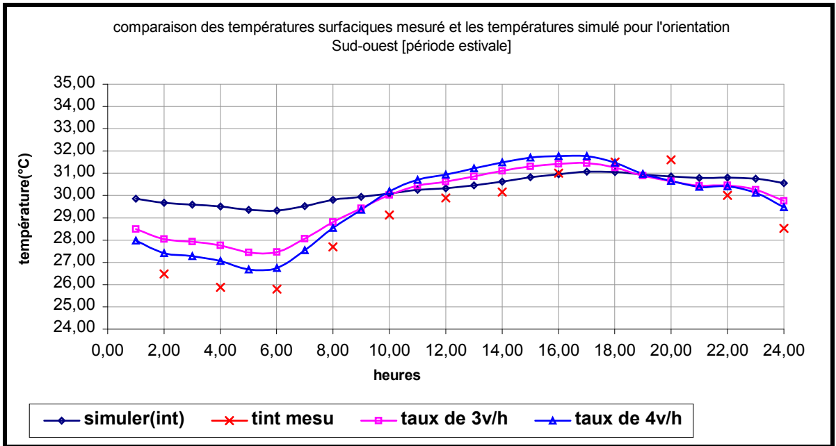
Figure 7-36: Effet de la ventilation sur la température intérieure (orientation sud ouest)
