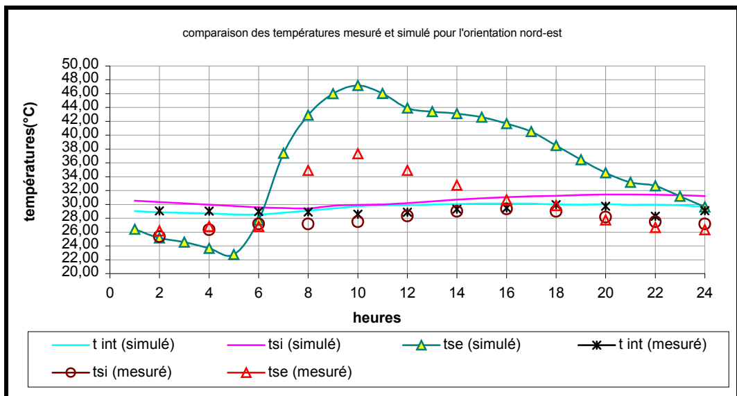
Figure 7-6 : Comparaison des températures surfaciques mesurée et simulée pour l'orientation Nord-est. [Période d'été] journée du 20-07-2004.
