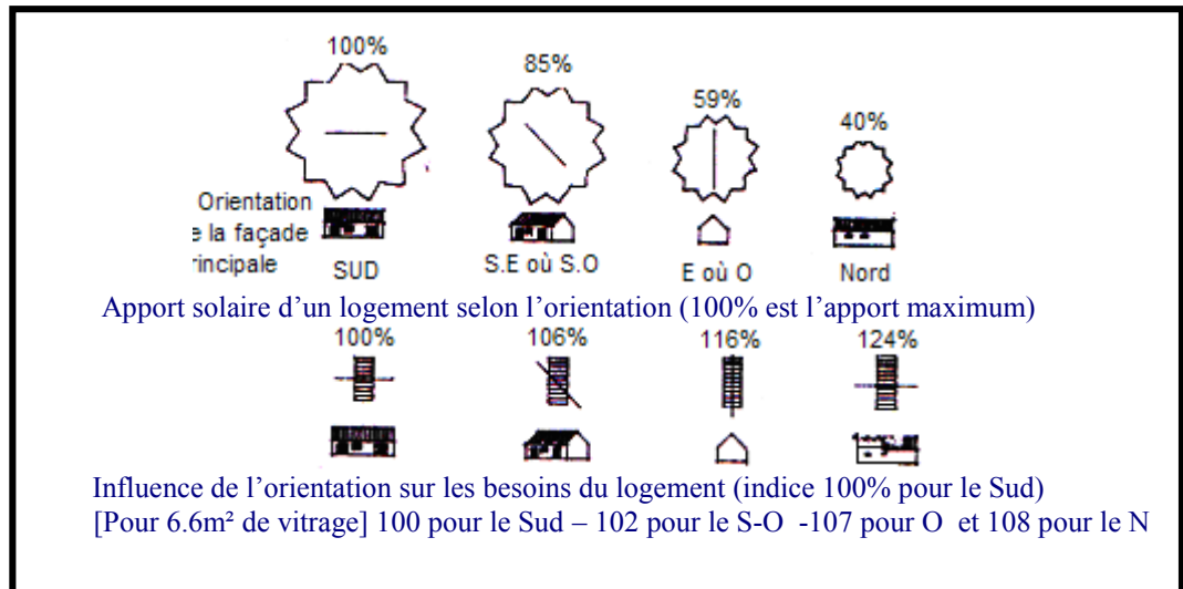
Figure 5-9 : Influence de l'orientation sur les besoins du logement. Source : G.R.P.A.C.A, 1988.
