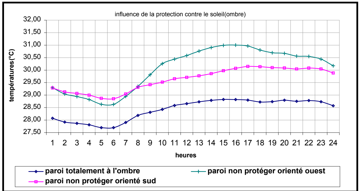
Figure 7-35 : Effet de la protection de la façade des rayons solaires.
