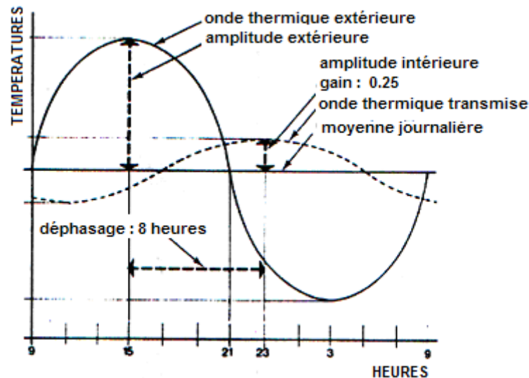
Figure 4- 2 : Définition du déphasage et de l'amplitude de l'onde incidente par une paroi homogène. Source : IZARD. J.L ET GUYOT.A, 1979.
