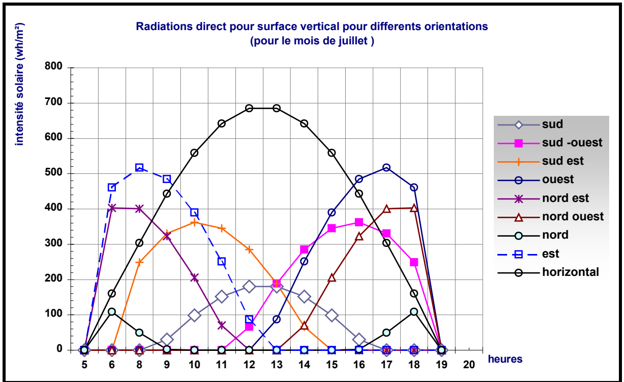
Figure 3- 32 : Radiations directes pour une surface verticale pour différentes orientations durant un mois chaud de l'année – JUILLET- pour la ville de constantine. Source : CAPDEROU.1988.
