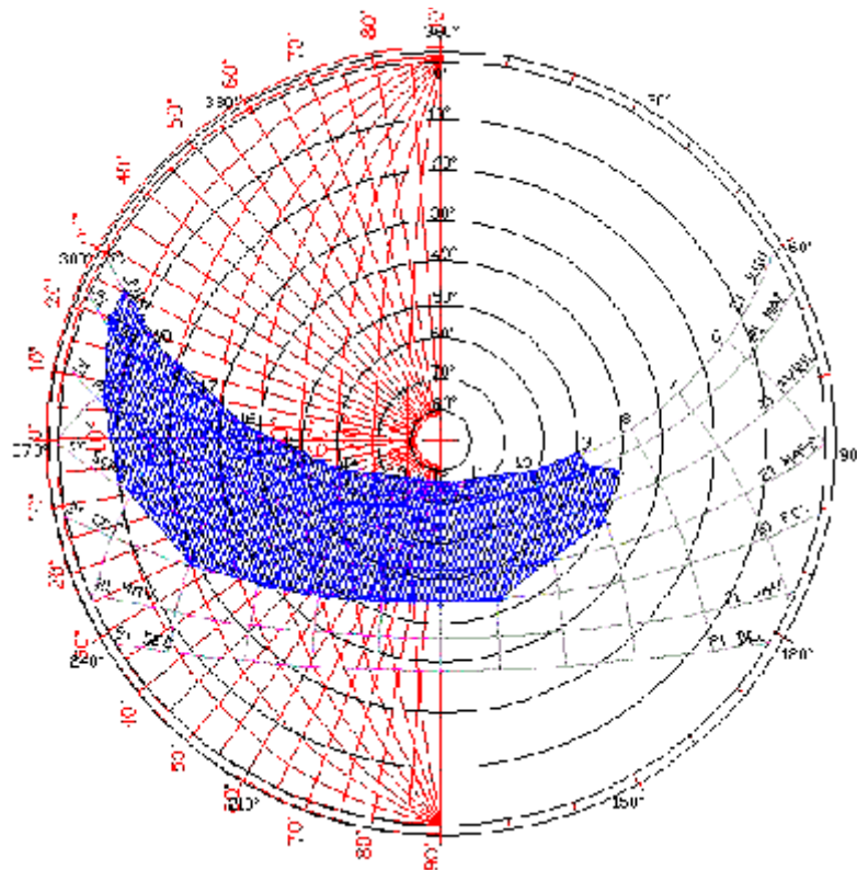
Figure 4-44 : Masque d'ombre de la protection solaire de la fenêtre Ouest. Source : Auteur.
