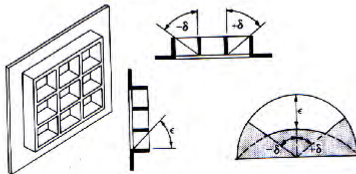
Figure 4-33 : Type de protection combinée. Source: S V SZOKOLAY, 1979.
