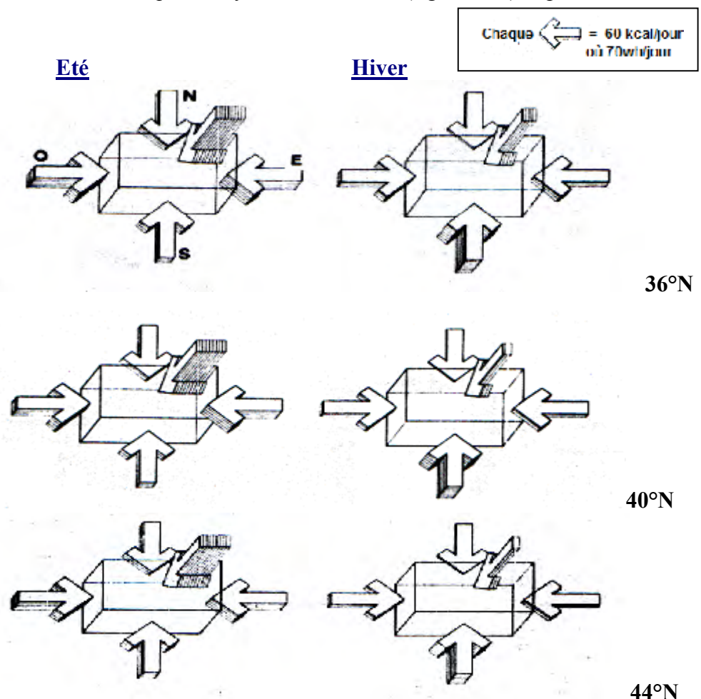
Figure 5-7: Intensité Du Rayonnement Solaire Sous Différentes Latitudes. Source : MAZRIA. ed, 1981.
