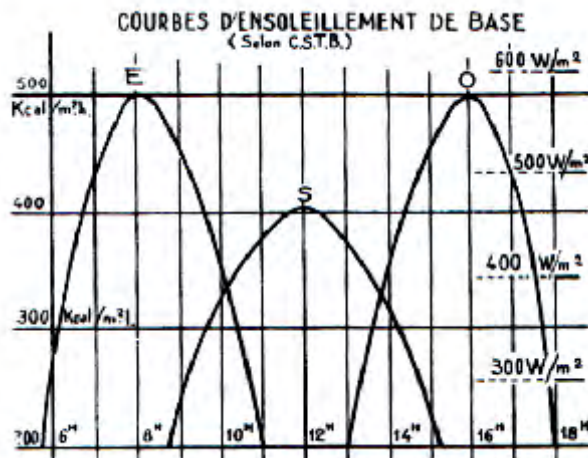
Figure 3-17 : Courbes d'ensoleillement de base selon C.S.T.B.
