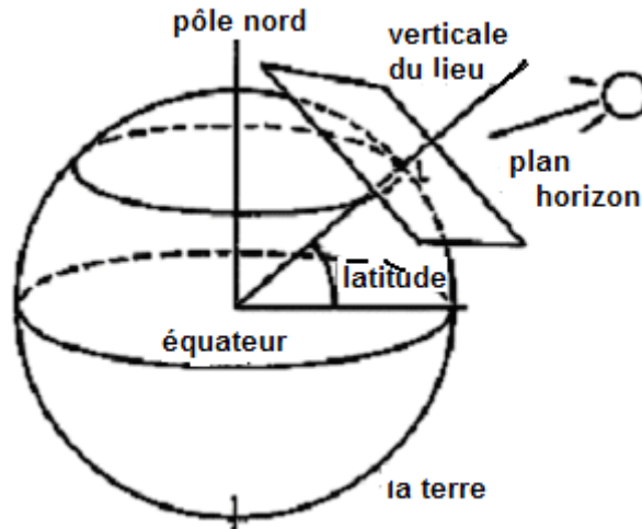
Figure 3- 6 : La latitude d'un lieu. Source : CERMA, 2004.
