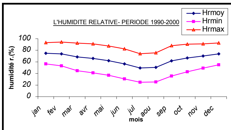
Figure 2-6:Humidité relative (%) période « 1990-2000 »
