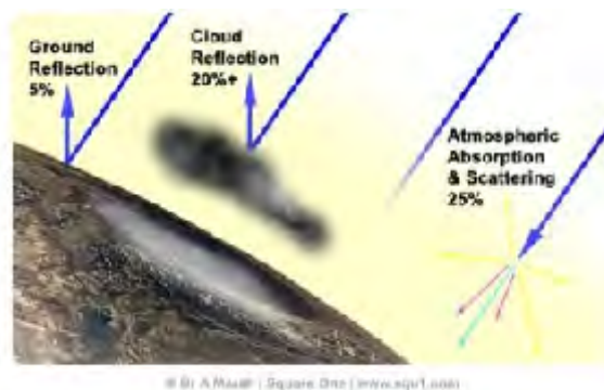
Figure 3- 12 : Effets de l'atmosphère sur l'irradiation solaire
