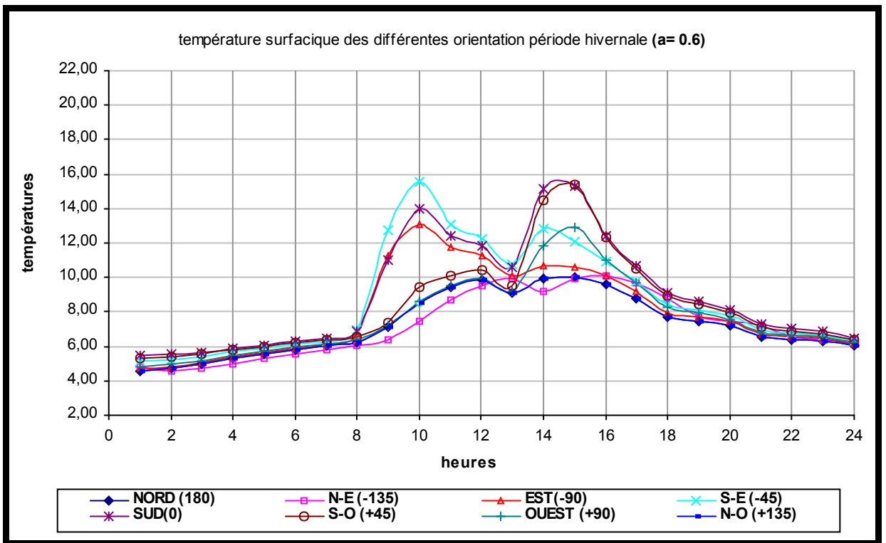
Figure 7-28 : Températures surfaciques des différentes orientations pour une couleur moyenne (période d’hiver)
