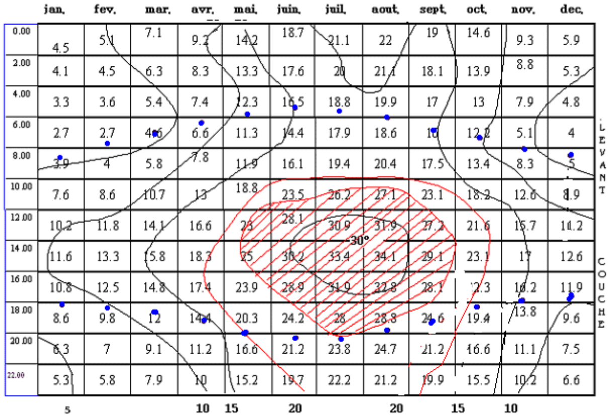
Figure 3- 18 : ISOTHERME DE CONSTANTINE. Source : Auteur.
