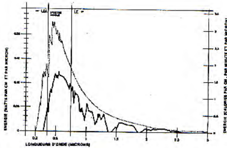
Figure 3-11: Composants du spectre électromagnétique du soleil. Source : Mazria .ed, 1980
