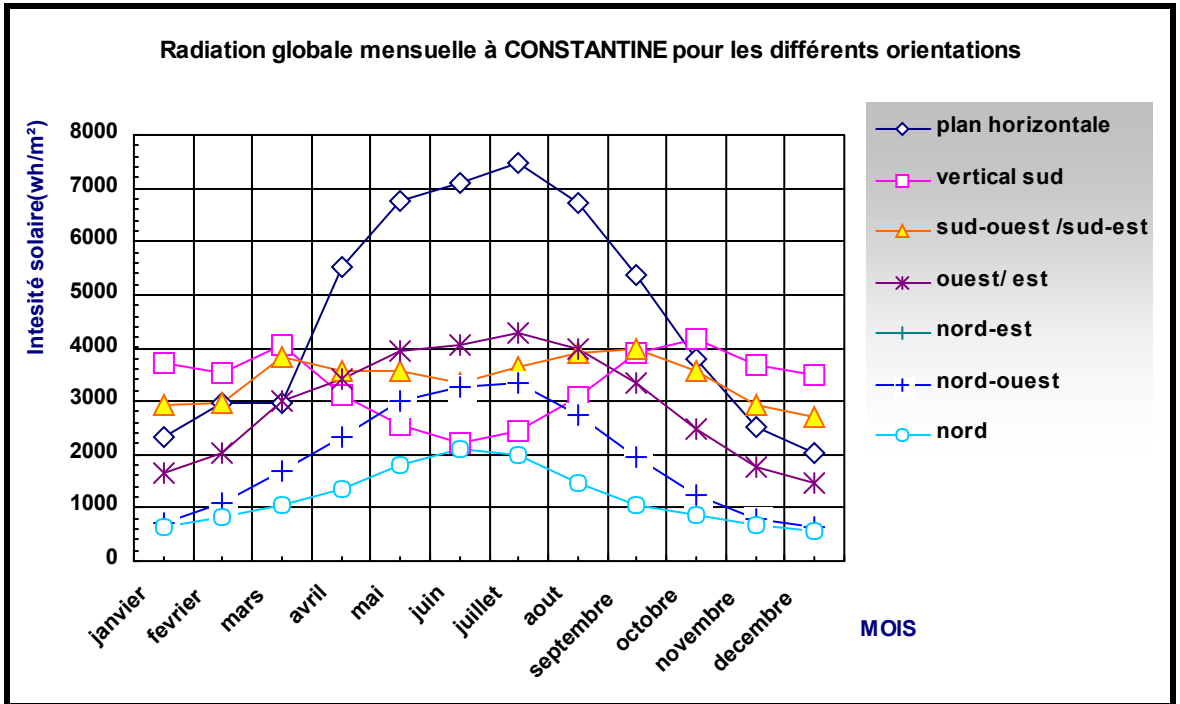
Figure 3-24 : Irradiation globale mensuelle d'une paroi pour différentes orientations « Pour la ville de Constantine » Source : CAPDEROU.1988.
