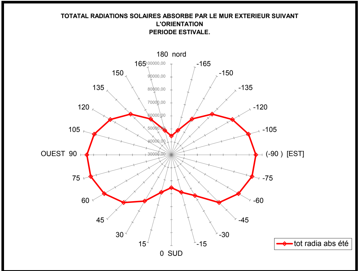
Figure 7-21 : Totale de radiation solaire absorbée par la paroi extérieure en (kJ/m 2 . h) suivant l'orientation. Période estivale.
