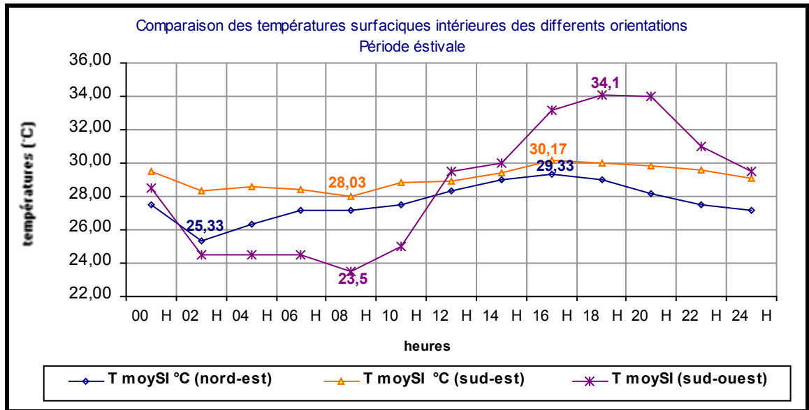
Figure 6-21 : Comparaison des températures surfaciques intérieures des différentes orientations Constantine, 2004 [période d'été]
