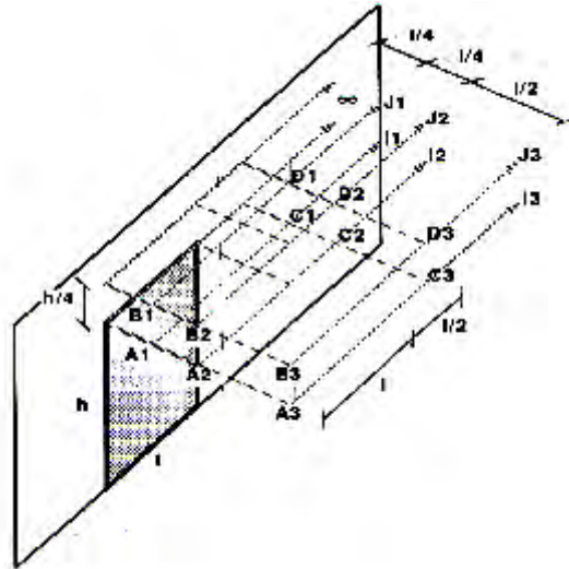
Figure 4-27: Effet de l’auvent. Source : Izard. J.L, 1993
