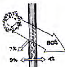
Figure 4-9 : Gain solaire à travers un simple vitrage.
