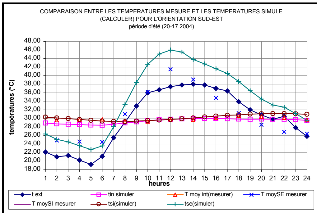
Figure 7-4 : Comparaison des températures surfaciques mesurée et simulée pour sud-est. [Période d'été] journée du 20-07-2004.
