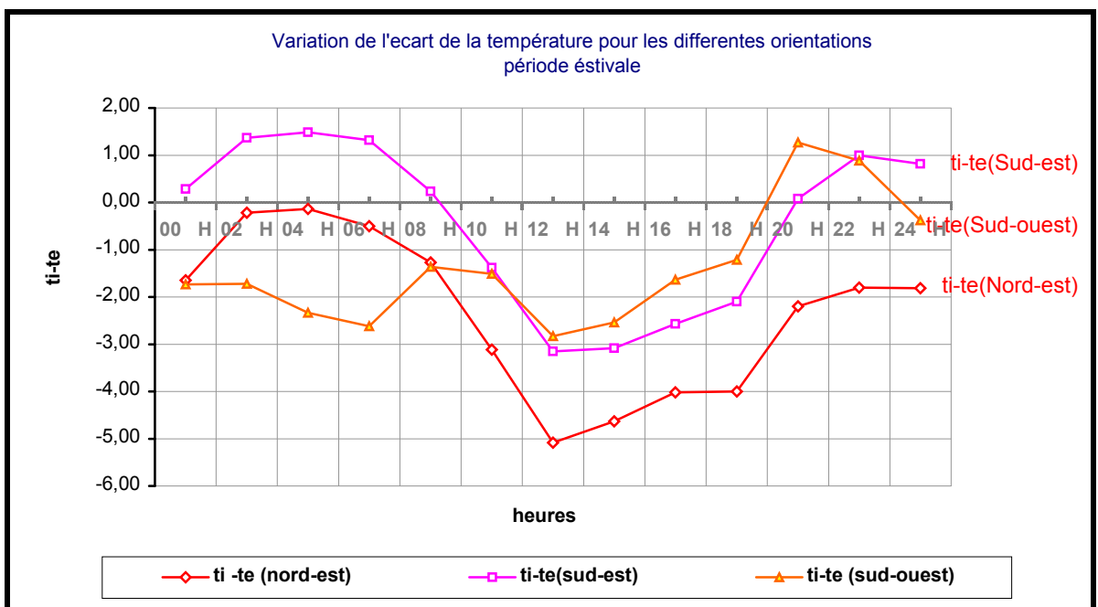
Figure 6-22 : Variation de l'écart de la température pour les différentes orientations [période d'été]
