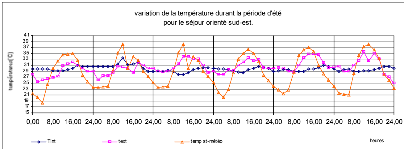
Figure A-7 : variation de la température intérieure durant la période (17/07 à 22/07/2004) séjour orienté à 30 azimuth est.(période d'été)
