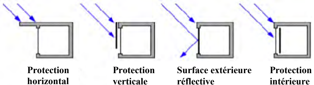
Figure 4- 16 : stratégies d'ombre. Source : MARSH. A, 1981.
