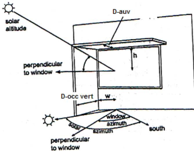
Figure 4-19 : Profondeur et largeur d'une occultation.
