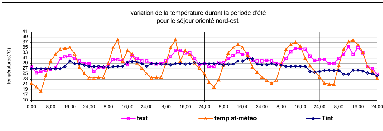
Figure A-8 : : variation de la température intérieure durant la période (17/07 à 22/07/2004) séjour orienté à 120 azimuth est.(période d'été)
