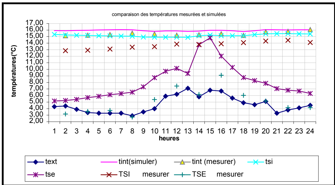
Figure 7-14 : Comparaison des températures surfaciques mesurées et simulées pour l'orientation Sud-ouest. [Période d'hiver] journée du 07-01-2005.
