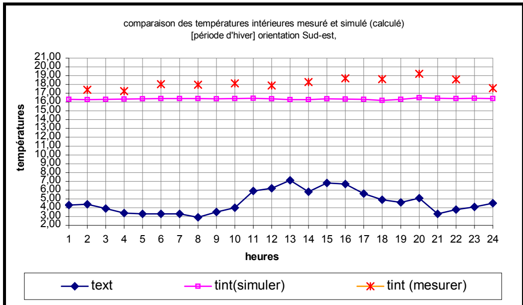
Figure 7-9 : Comparaison des températures intérieures mesurées et simulées pour l'orientation Sud-est. [Période d'hiver] journée du 07-01-2005.
