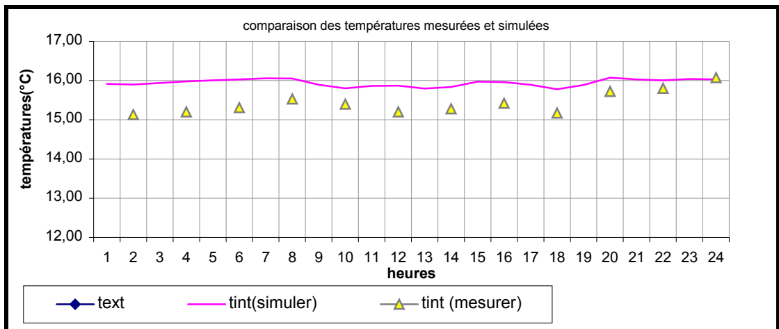
Figure 7-13 : Comparaison des températures intérieures mesurées et simulées pour l'orientation Sud-ouest. [Période d'hiver] journée du 07-01-2005.
