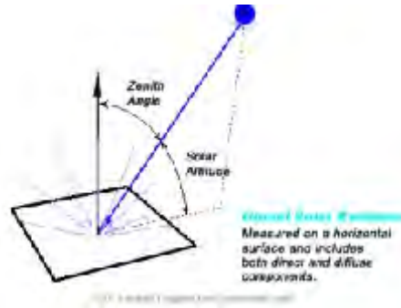
Figure 4-6 : Radiations solaires globales (somme des radiations solaires directes, diffuses et réfléchies.) Source : MARSH, A, 1980.
