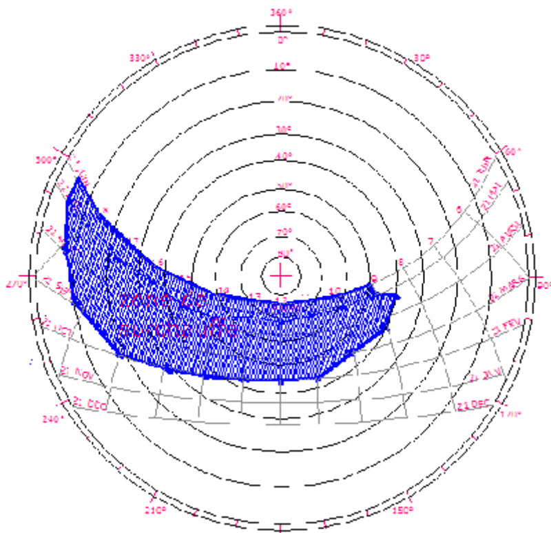
Figure A-6: Zone de surchauffe pour la latitude 36°17'
