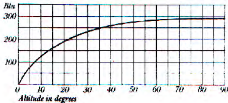
Figure 3-16: Variation du rayonnement direct normal avec la hauteur du soleil.
