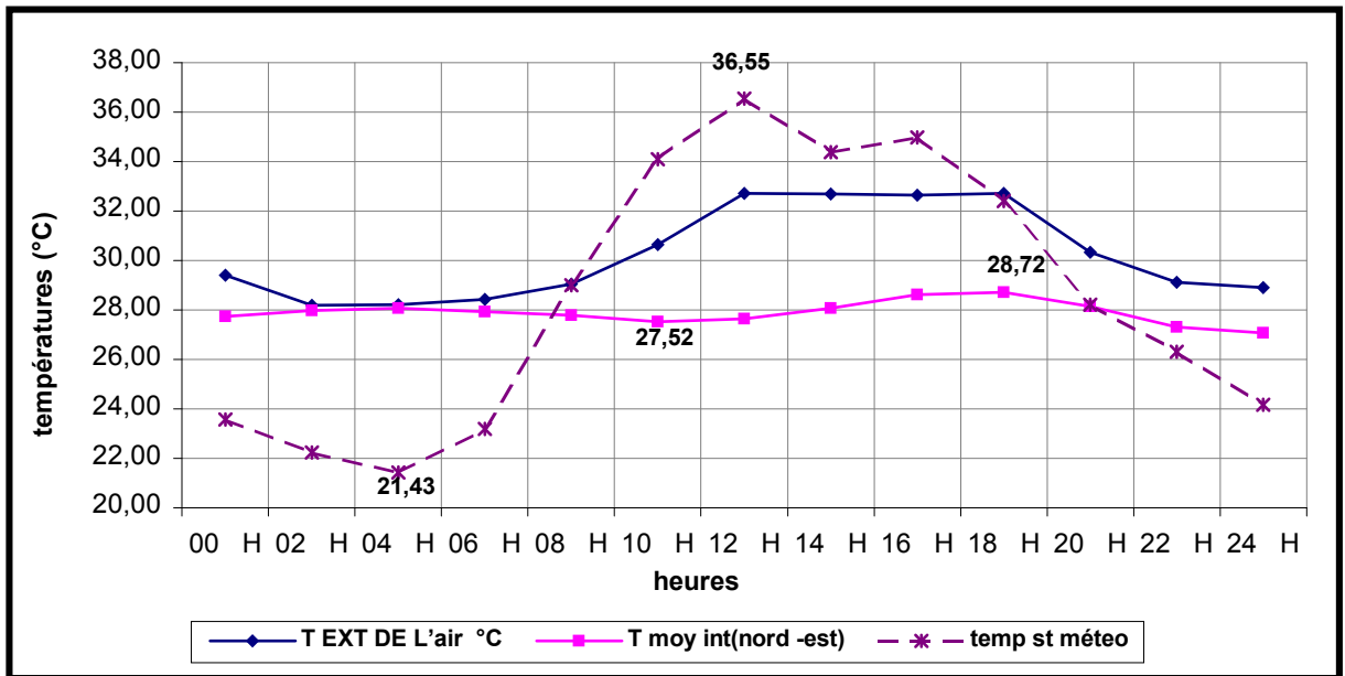
Figure 6-10: Variation de la température intérieure et extérieure, orientation Nord-est. Constantine période d'été.
