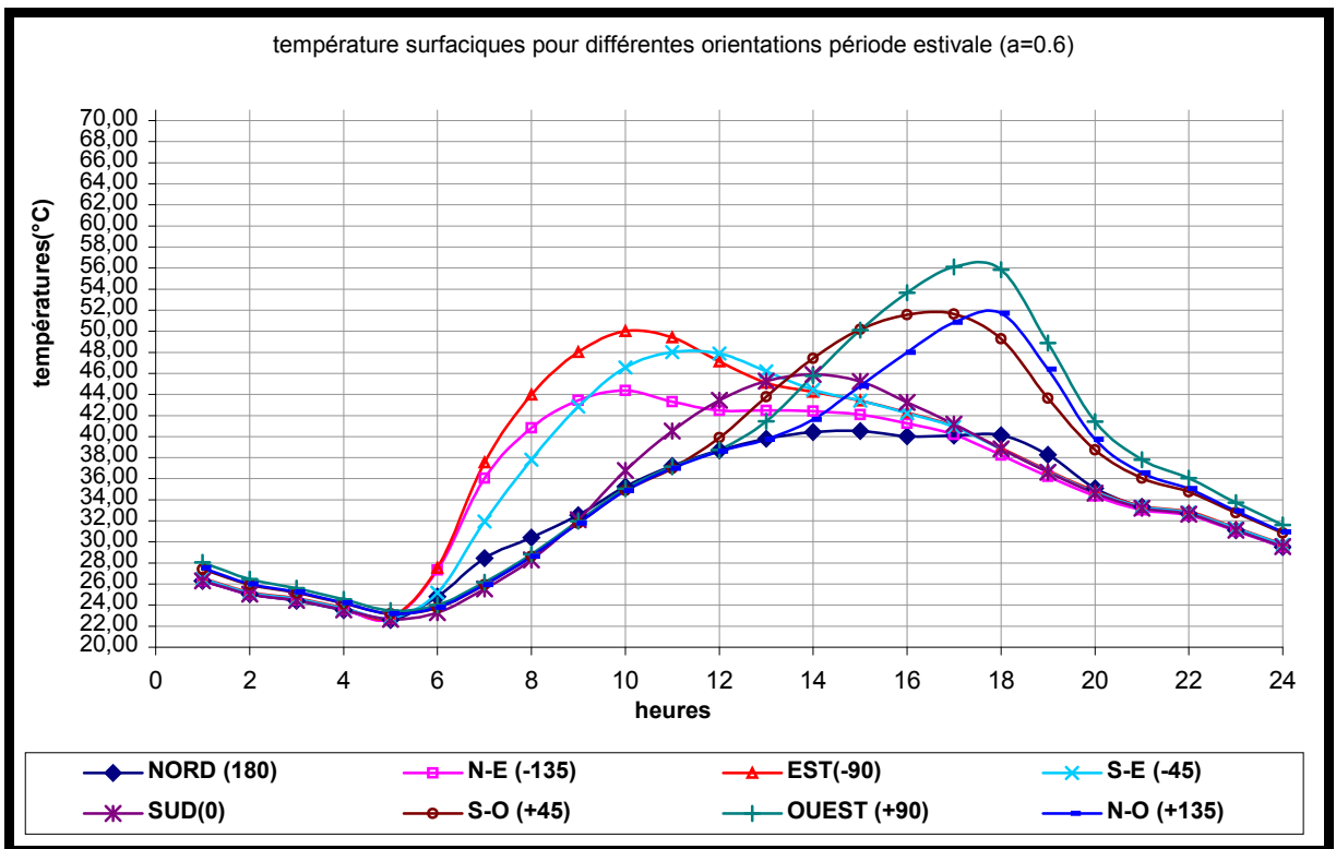
Figure 7-26 : Températures surfaciques des différentes orientations pour une couleur moyenne. (période d'été)
