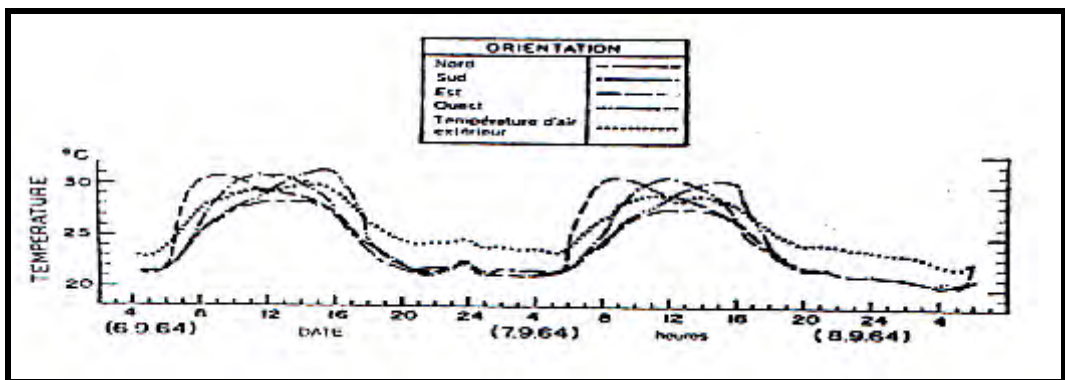
Figure 5-14 : Températures de surfaces externes de murs blancs de différentes orientations.
