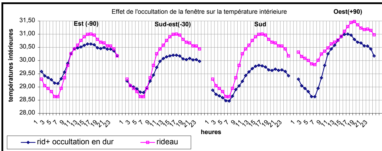
Figure 7-34 : Effet de l'occultation de la fenêtre sur l'abaissement de la température intérieure pour les différentes orientations (période d'été)
