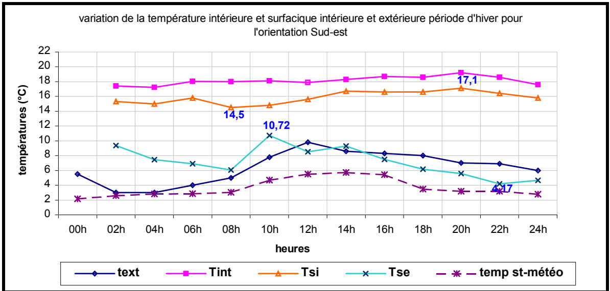
Figure 6-28 : Variation de la température intérieure et surfacique intérieure et extérieure, pour le séjour orienté Sud-est. [Période d’hiver] Constantine, 2004.
