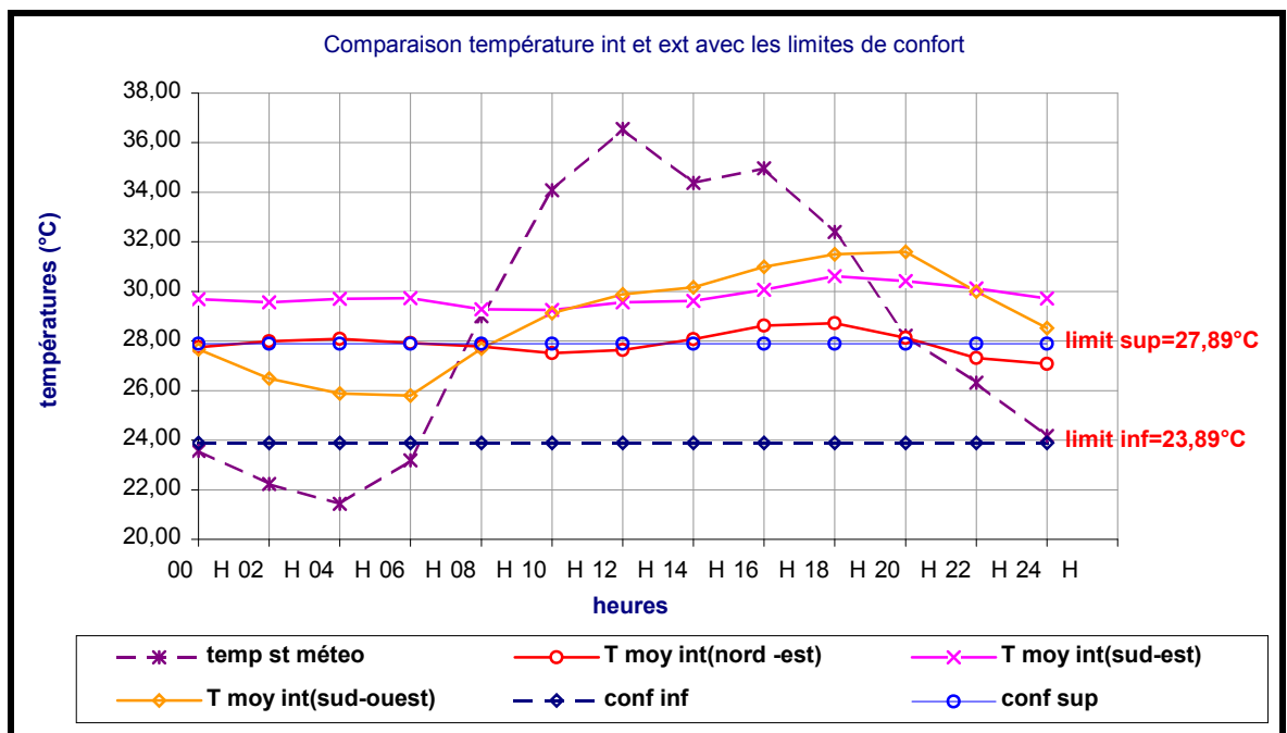
Figure 6-35 : Comparaison des températures Int. et Ext. avec les limites de confort.
