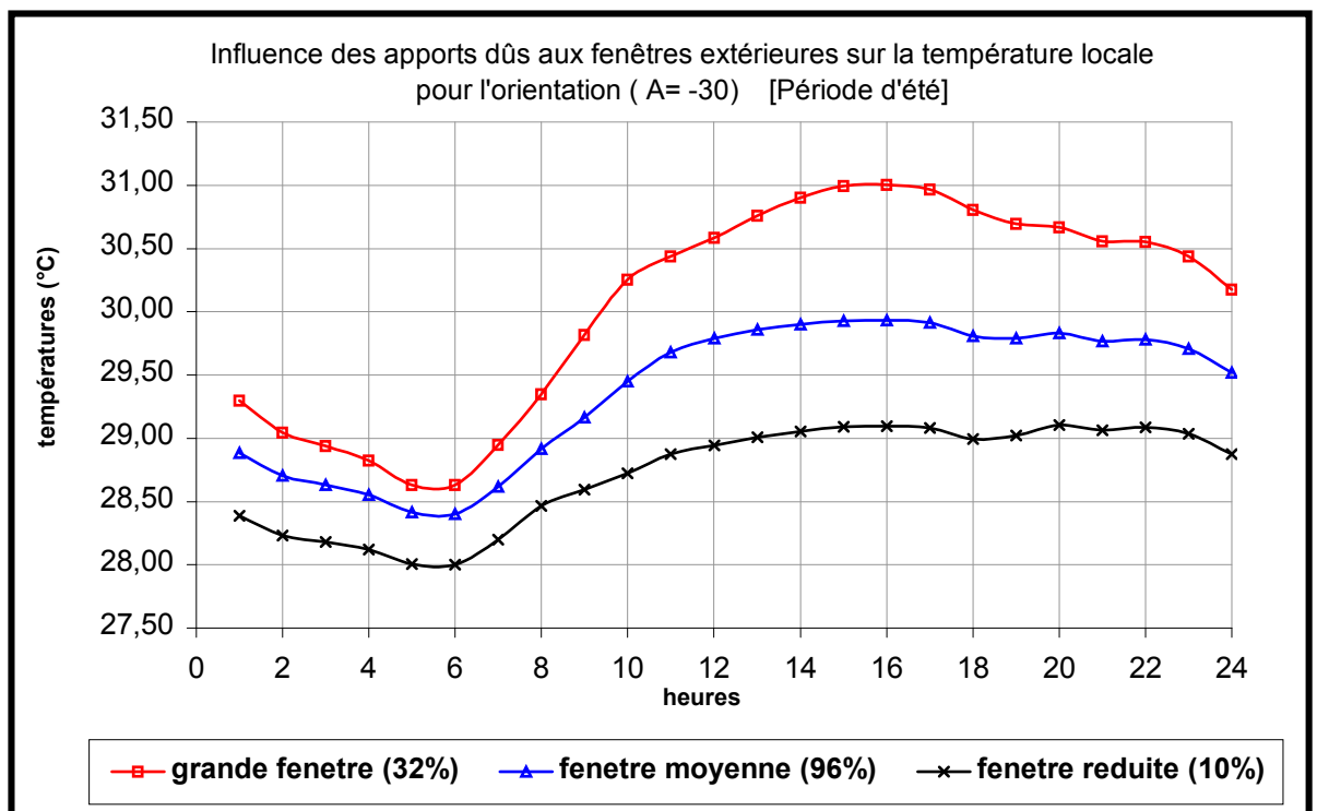
Figure 7-32 : Influence de la taille de la fenêtre sur la température intérieure.
