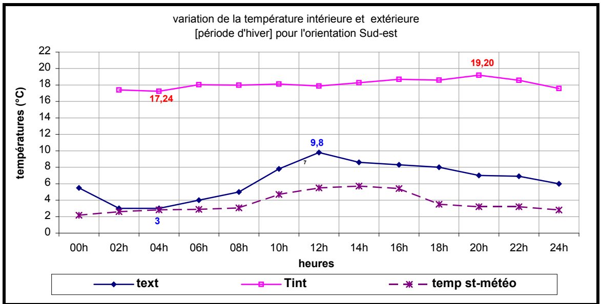
Figure 6-26 : Variation de la température intérieure et extérieure pour le séjour orienté Sud-est. [Période d'hiver] Constantine, 2004.
