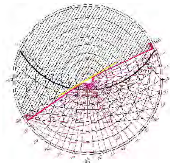
Figure 5-25 : Masque d'ombre de la protection solaire de la fenêtre du séjour SUD-EST.
