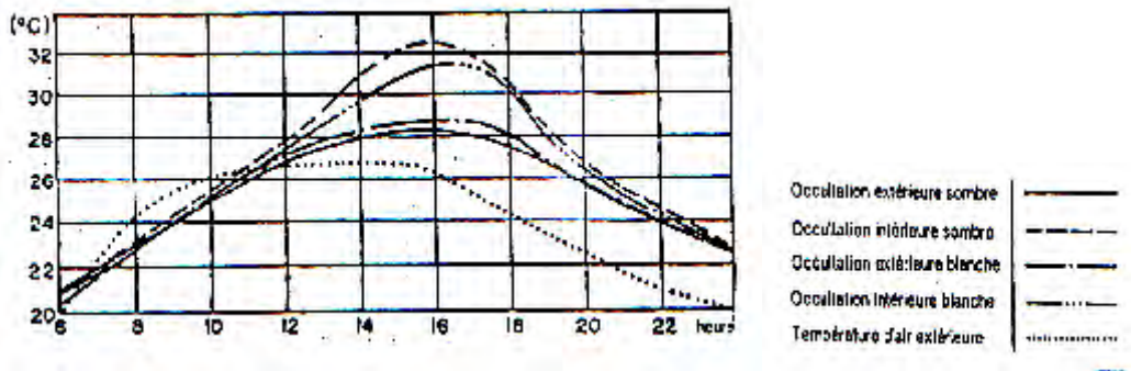
Figure 4-22 : Régimes de températures intérieures pour différents systèmes d'occultation.
