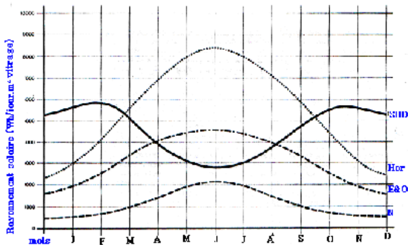
Figure 4-14 : Comparaison entre fenêtres diversement orientées.
