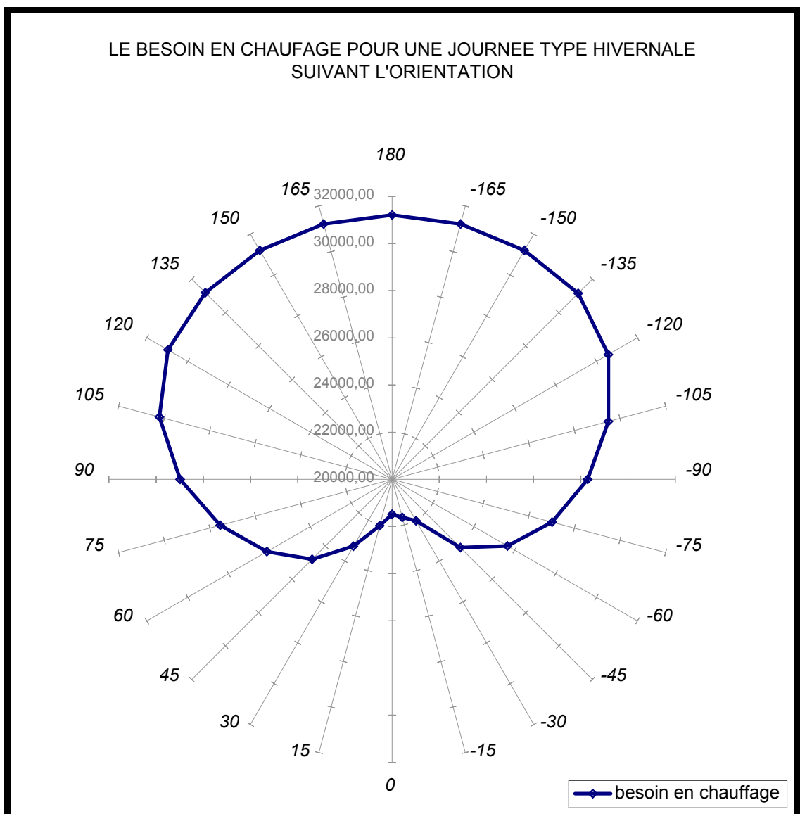
Figure 7-23 : Le besoin en chauffage suivant l'orientation(en kJ).
