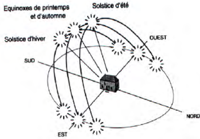
Figure 3- 5 : Trajectoires apparentes du soleil au cours de l'année.
