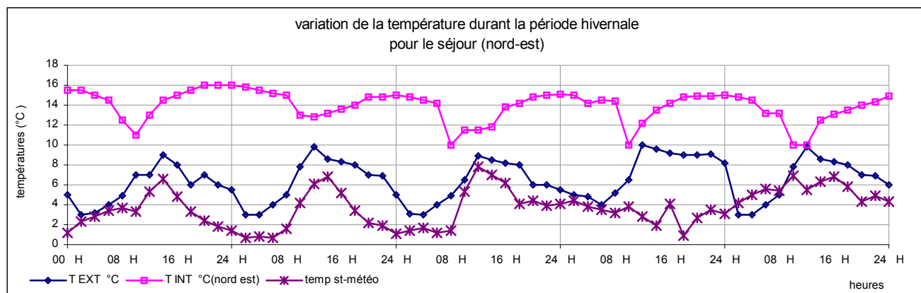
Figure A-9 : variation de la température intérieure durant la période (17/07 à 22/07/2004) séjour orienté à 120 azimuth est.(période d'hiver)
