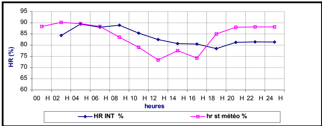
Figure 6-30 : Variation de l'humidité relative dans le séjour orienté sud-ouest. [période d'hiver] Constantine, 2004.
