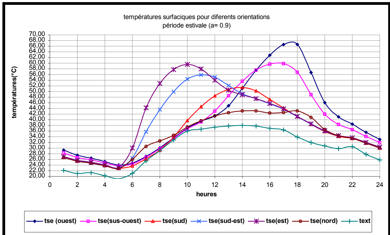
Figure 7-25: Températures surfaciques des différentes orientations pour une couleur sombre (période d'été)
