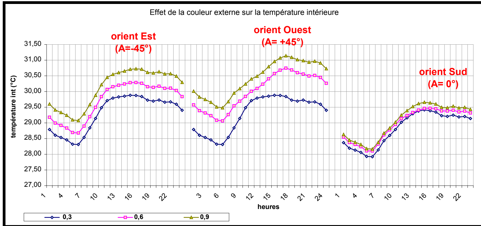
Figure 7-31 : Effet de la couleur sur la température intérieure (pour les orientations Est, Ouest et Sud).
