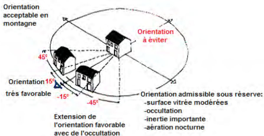
Figure 5-12 : Orientation de la façade principale d'un logement PACA.
