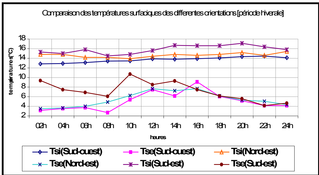
Figure 6-33 : Comparaison des températures surfaciques int. et ext.[ période d’hiver] Constantine, 2004.
