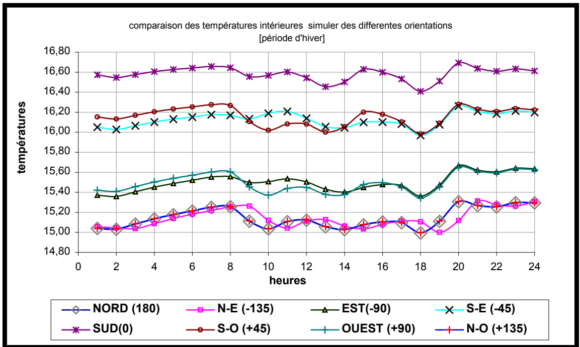
Figure 7-18 : Effet de l'orientation sur la température intérieure [période d'hiver]
