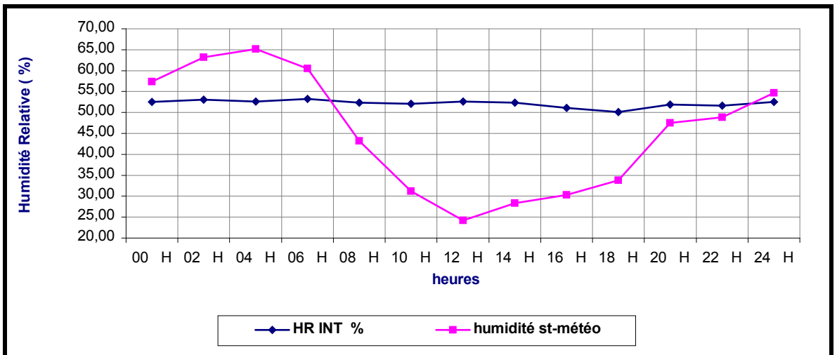
Figure 6-15 : Variation de l'humidité relative intérieure et extérieure du séjour orienté Sud-est. Constantine période d'été.
