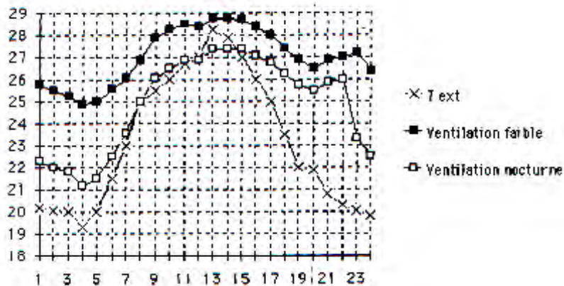
Figure 4-51 : Effet de la ventilation nocturne sur la température d'air intérieure.
