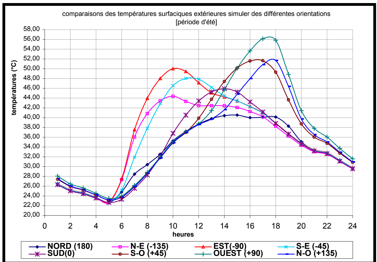
Figure 7-20 : Comparaison des températures surfaciques extérieures simulées pour les différentes orientations (Période d'été).
