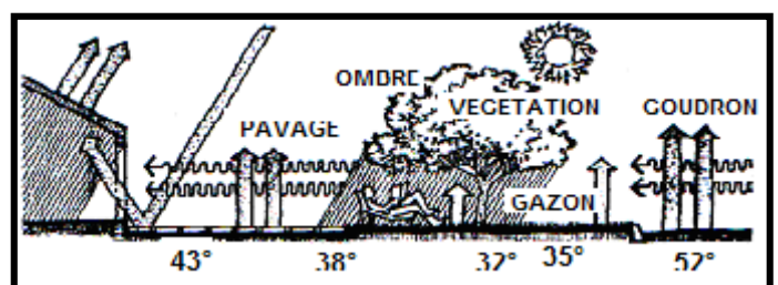
Figure 5-20: Les Températures Autour D'un Bâtiment Et La Nature Des Surfaces Environnantes. Source : KONYA.A 1980
