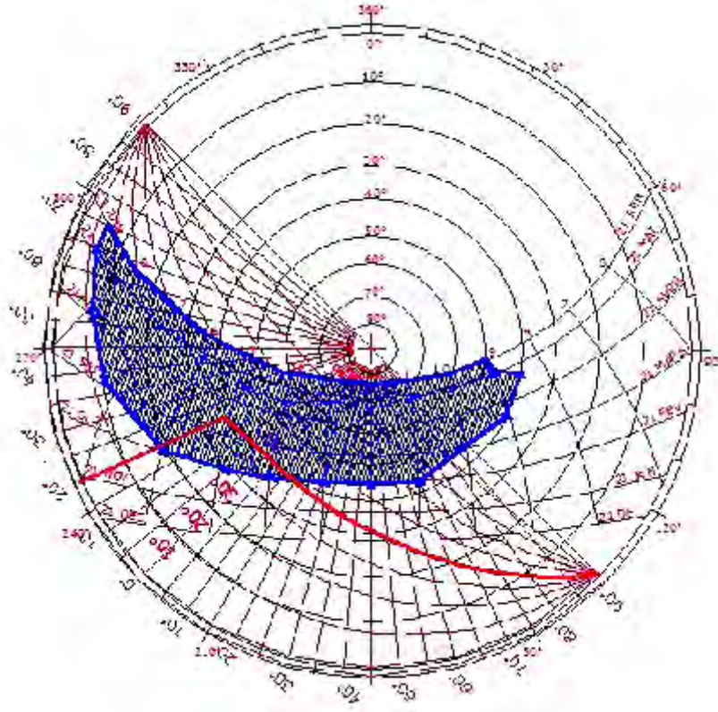
Figure 4-42: Masque d'ombre de la protection solaire de la fenêtre Sud-ouest. Source : Auteur.
