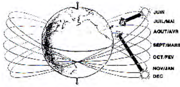
Figure 3-7 : la déclinaison du soleil, telle qu'elle apparaît depuis la terre, le 20 ème jour de chaque mois. Source : MAZRIA, 1981.
