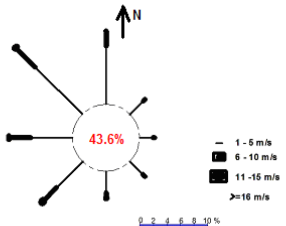
Rose des vents (frequences vents en%) période 1995 - 2004
