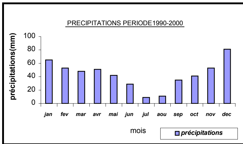
Figure 2-9 : Précipitation en (mm) période (1990-2000)
