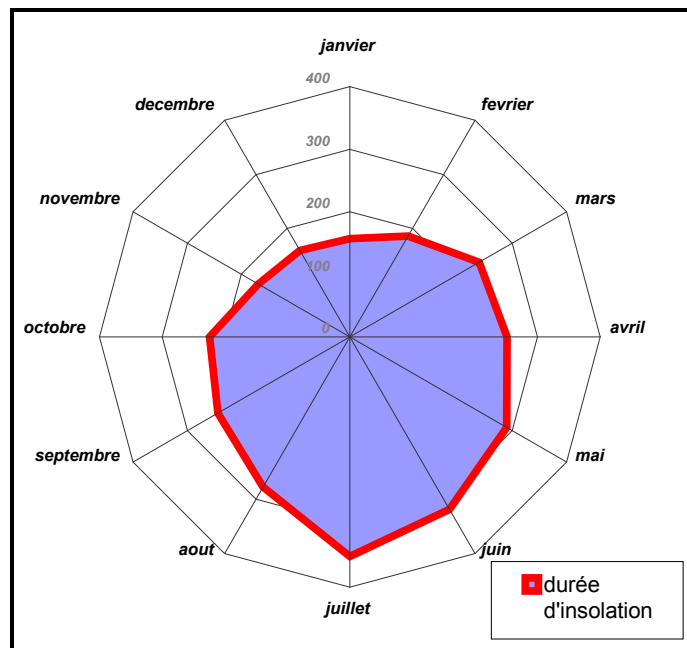
Figure 2-4 : Moyenne mensuelle de la durée d'insolation (en heure). Période de 1994-2003. Source : ONM de Ain el bey de Constantine.
