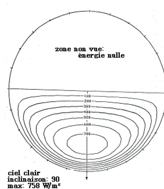
Figure 3-19 : Diagramme énergétique solaire du plan vertical (courbes iso puissance en W/m^2 ). (Indicateur d'irradiation solaire pour une paroi verticale) Source : IZARD.J.L, 1994
