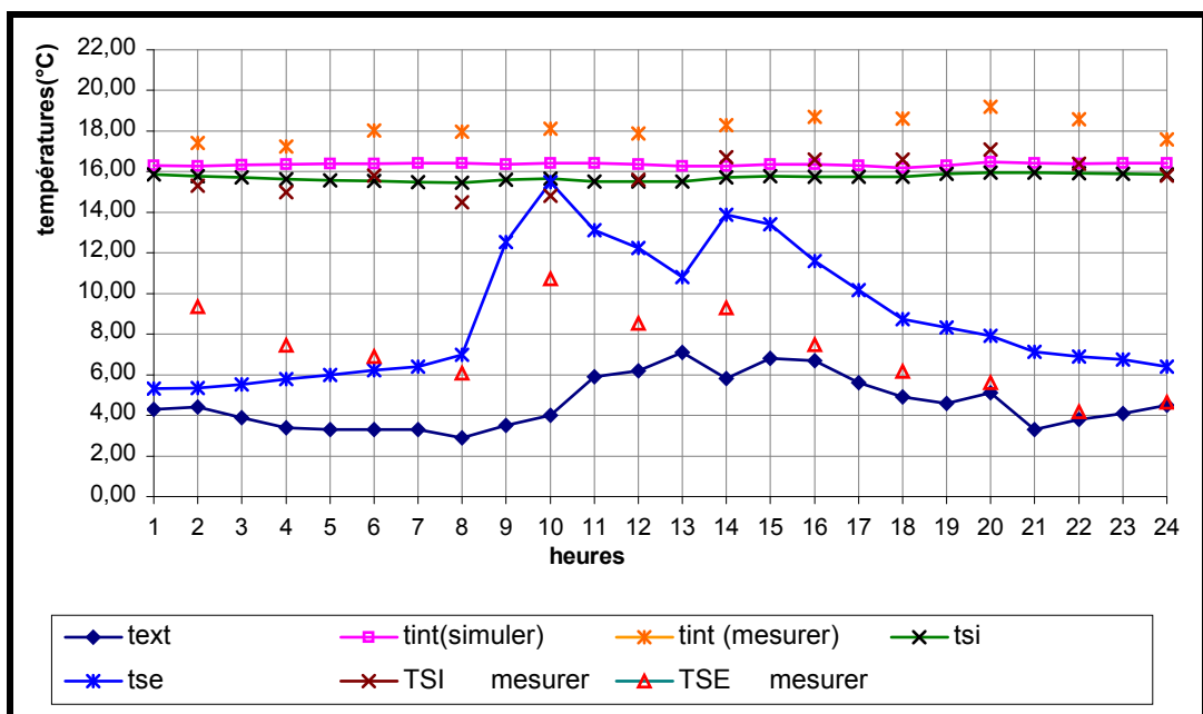
Figure 7-10 : Comparaison des températures intérieures mesurées et simulées pour l'orientation Sud-est. [Période d'hiver] journée du 07-01-2005.
