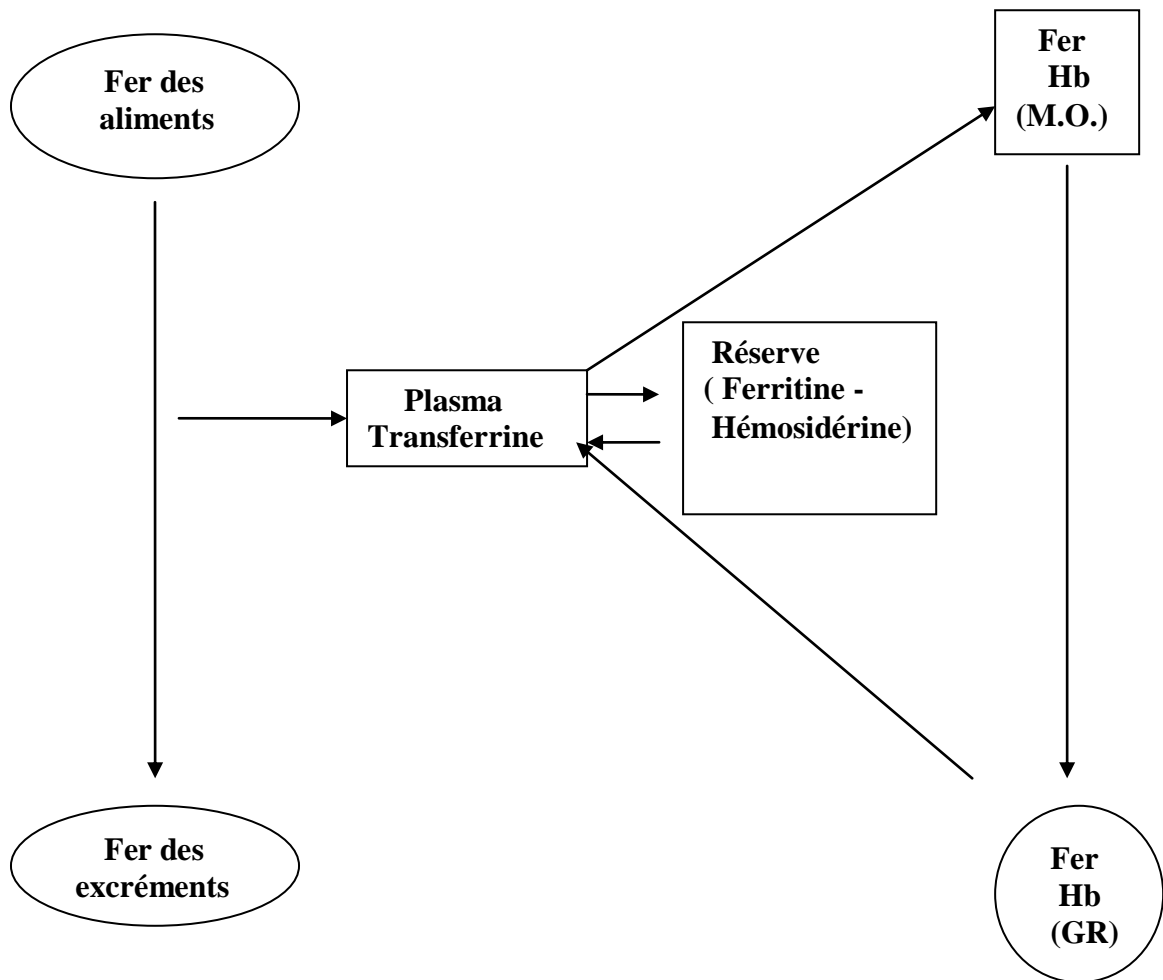
Figure 8 - Schéma simplifié des compartiments du fer (synthèse personnelle)
