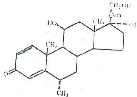
Figure 3 - Structure de la méthylprednisolone
