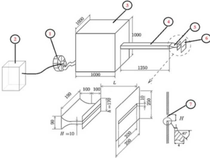
Figure 1 : Dispositif expérimental
