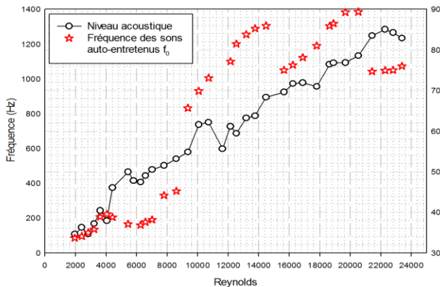
Figure 5 : fréquences et niveaux acoustiques des sons auto-entretenus en fonction du nombre de Reynolds pour L/H=4
