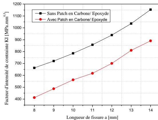
FIGURE 10. Evolution du facteur d'intensité de contrainte en mode I dans une plaque en aluminium fissurée avec et sans réparation par patch.
