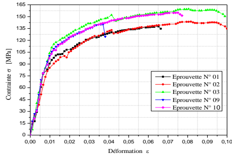
FIGURE 4. Courbe de traction (Contrainte-déformation) pour les éprouvettes mines en aluminium réalisées selon la norme ISO3167.
