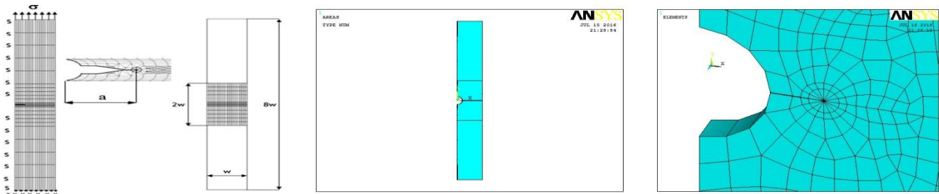
FIGURE 8. Modèle numérique d'une plaque en plaque fissurée non réparée.
