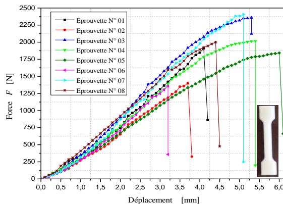
FIGURE 7. Courbes Force-Déplacement pour les éprouvettes en résine.
